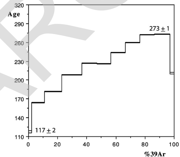
Fig. 26 - Spettro di età apparente Ar/Ar su WM appartenente ad un campione di Gneiss Chiari del Corno Stella milonitico campionato lungo la Linea del Porcile (BERGOMI, 2004).
