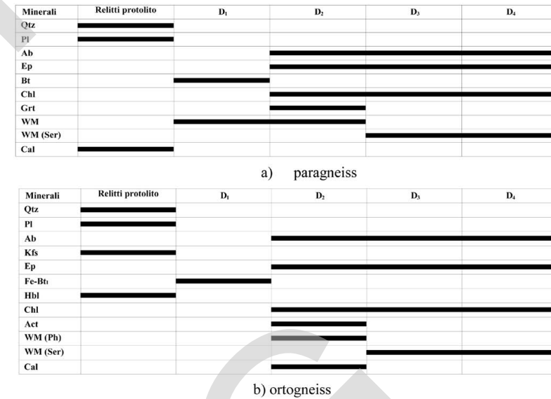
Fig. 23 - Relazioni tra fasi deformative e cristallizzazione metamorfica negli Gneiss del Monte Canale: a) paragneiss; b) ortogneiss. D 1 e D 2 sono fasi pre-alpine, D 3 e D 4 alpine.
