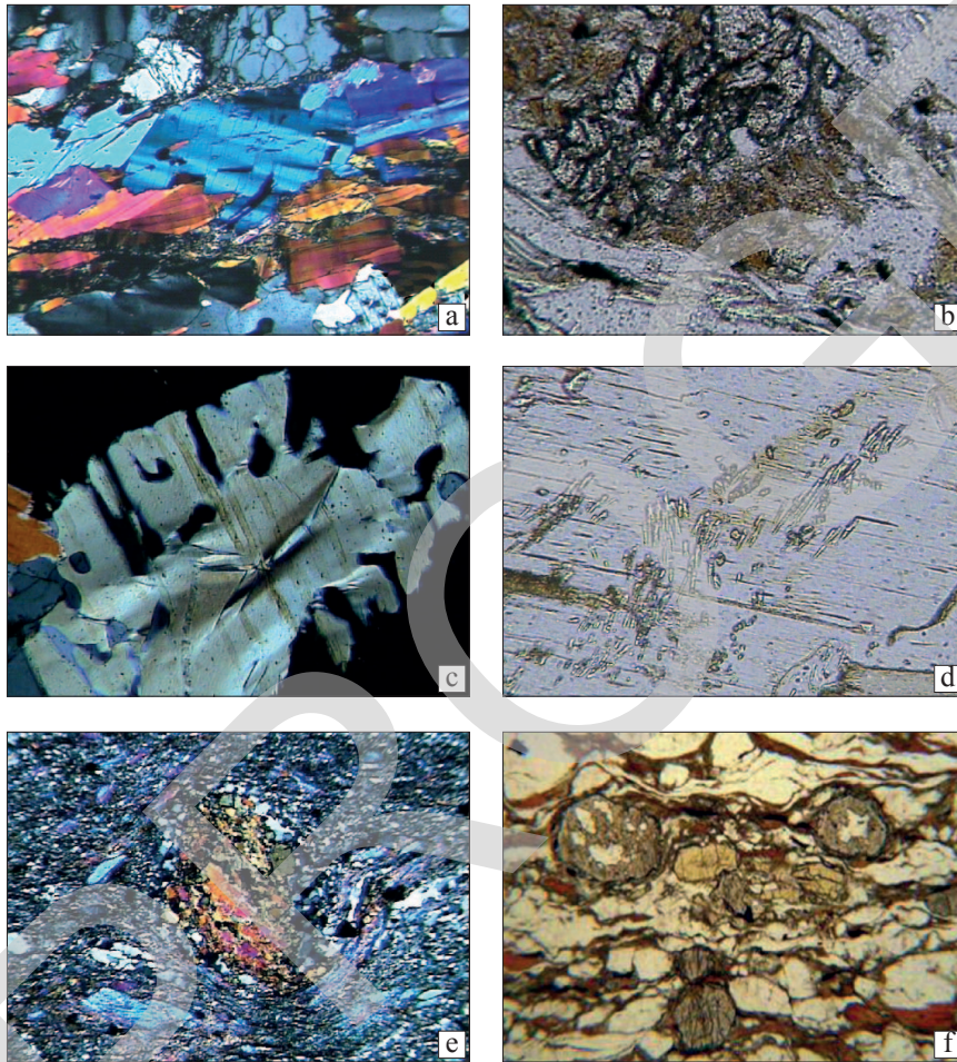
Fig. 5 - Unità degli Gneiss del Monte Tonale – Microfotografie di sezioni sottili: a) Paragneiss kinzigitico. Pol+, 15X - Muscovite cross deformata con relitti di sillimanite. Lungo la strada in sinistra idrografica del Torrente Davaglione, in prossimità di Alpe Arcino (q. 1675 m s.l.m.); b) Protomilonite di paragneiss Pol+, 15X - Granato parzialmente cloritizzato. Dalla clorite si forma biotite nuova. Lungo la strada a Nord di Postalesio in sinistra idrografica del Torrente Caldenno (q. 1000 m s.l.m.); c) Paragneiss kinzigitico Pol+, 15X - Muscovite cross deformata con gocce di quarzo (tipo mirmechite). Lungo la strada in sinistra idrografica Torrente Davaglione, in prossimità di Alpe Arcino (q. 1675 m s.l.m.); d) Paragneiss kinzigitico. Pol+, 20X - Muscovite cross deformata con inclusi di sillimanite relitta. Lungo la strada a Nord di Postalesio in sinistra idrografica Torrente Davaglione, in prossimità di Alpe Arcino (q. 1675 m s.l.m.); e) Milonite di paragneiss. Pol+, 10X - Porfiroclasto di tormalina ricristallizzato. Lungo la strada nel tratto tra Prasomaso e Premachera (q. 1330 m s.l.m.); f) Milonite di micascisto a Bt+Grt+St. Solo pol. 10X. - Lungo la strada in destra idrografica della Val Fontana, a Nord delle Baite della Piana (q. 830 m s.l.m.).
