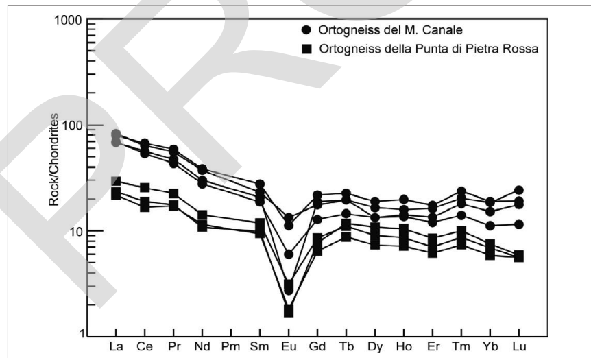
Fig. 3 - Pattern delle REE, normalizzato alla condrite CI (NAKAMURA, 1974) degli ortogneiss occhiali a due miche dell'unità degli Gneiss della Punta di Pietra Rossa (Austroalpino superiore) e degli ortogneiss epidotici dell'unità degli Gneiss del Monte Canale (Austroalpino inferiore) (BERGOMI et alii , 2005).
