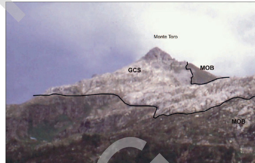
Fig. 12 - Contatto tra Gneiss Chiari del Corno Stella (GCS) e Gneiss di Morbegno (MOB) visto da NW. Versante NE del Monte Toro.
