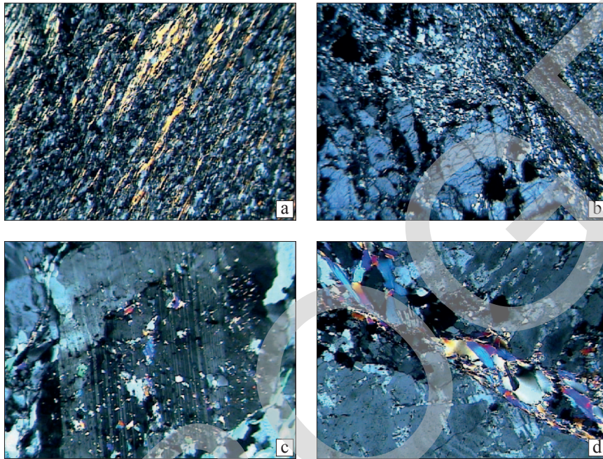
Fig. 4 - Unità degli Gneiss della Punta di Pietra Rossa - Microfotografie di sezioni sottili: a) Milonite di gneiss minuto. Pol+, 10X - Lungo la strada per Sasso, sopra Tresivio, nel tratto tra Prasomaso e Premacher (q. 1370 m s.l.m.); b) Milonite di ortogneiss occhiadino a due miche. Pol+, 15X - Porfiroclasto feldspatico. Val Fontana. c) Ortogneiss occhiadino a due miche. Pol+, 15X - Plagioclasio con zonatura ignea conservata. Lungo la strada a Nord di Regoledo, nel tratto Sogno-Prà Balzar (q. 980 m s.l.m.); d) Ortogneiss occhiadino a due miche. Pol+, 15X - K-feldspato concresciuto con plagioclasio. Lungo la strada a Nord di Regoledo, nel tratto Sogno-Prà Balzar (q. 980 m s.l.m.).
