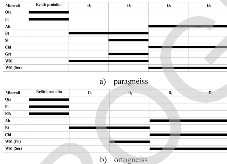
Fig. 22 - Relazioni tra fasi deformative e cristallizzazione metamorfica negli Gneiss della Punta di Pietra Rossa: a) paragneiss; b) ortogneiss. D 1 e D 2 sono fasi pre-alpine, D 3 e D 4 alpine.
