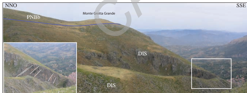
Fig. 40 - Panoramica del contatto stratigrafico tra i calcarei di Piano Battaglia (PNBb) e le sottostanti Dolomie di Isnello (DIS).
