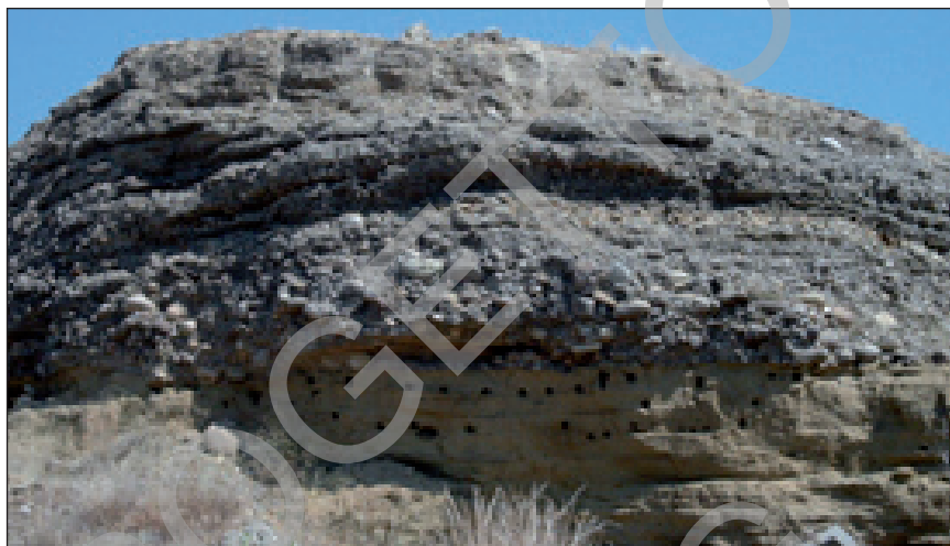
Fig. 56 -Alternanza tra orizzonti di sabbie e ghiaie nei depositi marini del sintema di Buonfornello-Campofelice, subsistema Rocca d'Antoni. Contrada Pestavecchia.
