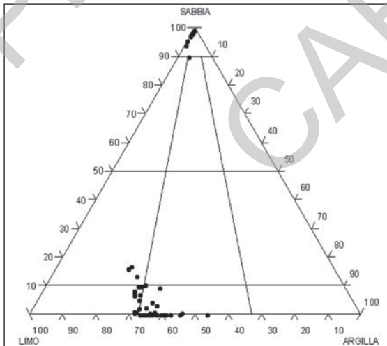
Fig. 65 - Distribuzione secondo il diagramma triangolare di FOLK (1954) dei campioni di sedimenti prelevati nel Golfo di Termini Imerese.
