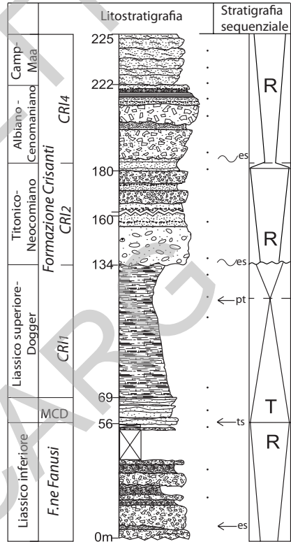
Fig. 35. Sezione colonnare della successione del Castello di Termini Imerese e interpretazione stratigrafico-sequenziale per la ciclicità di primo ordine (da BASILONE, 2000). Legenda, es: superficie di erosione sottomarina; ts: superficie di trasgressione; pt: superficie di massima trasgressione; R: regressione; T: rasgressione; i punti indicano la posizione dei campioni prelevati.
