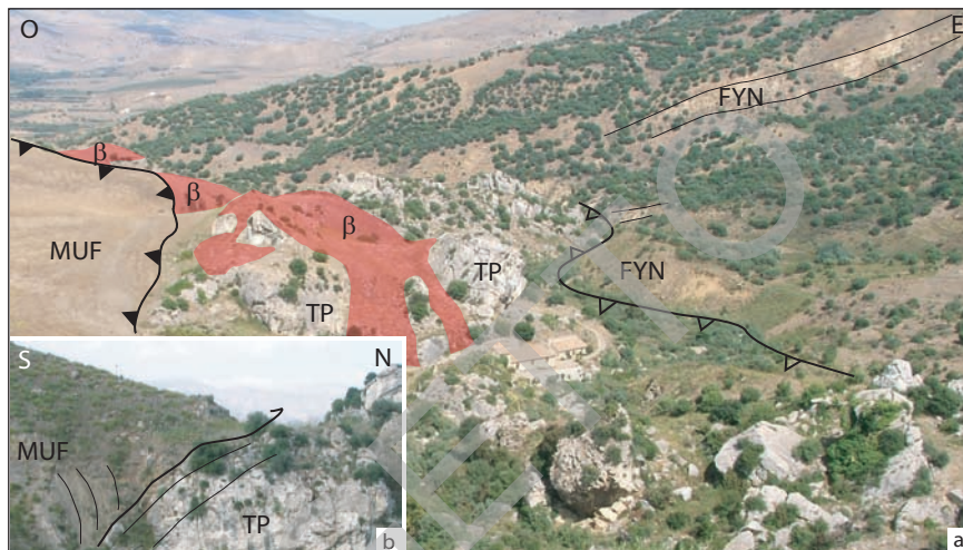
Fig. 74 - Le Rocche (Roccapalumba): a) contatti tettonici tra le successioni carbonatiche della piattaforma Trapanese e le unità strutturali sovrastanti (fysch numidico ad est e Formazione Mufara ad ovest); i depositi di piattaforma sono dissezionati da faglie dirette mesozoiche lungo le quali risalgono filoni magmatici ( \beta ). b) Particolare del sovrascorrimento delle unità permo-triassiche sui depositi di piattaforma del Dogger-Malm.
