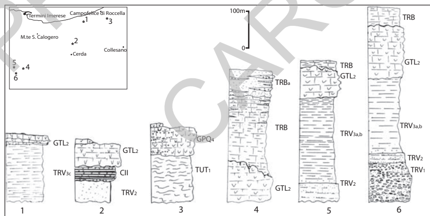
Fig. 47 - Sezioni stratigrafiche di successioni messiniano-plioceniche affioranti in due aree del Foglio. Area costiera F. Imera - F. Roccella: 1 - sezione di C.da Pestavecchia; 2 - sezione di Cozzo Marmaro; 3 - sezione di C.da Gatto. Area di Pizzo Bosco: 4 - sezione di Pizzo Bosco (fianco SE); 5 - sezione di Cozzo Bianco-Cozzo Scavuzzo; 6 - sezione di Cozzo Scorusa.
