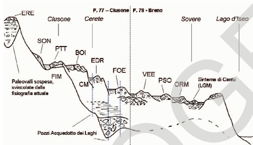
Fig. 17 - Schema dei rapporti stratigrafici fra le unità dell'anfiteatro della Val Borlezza.
