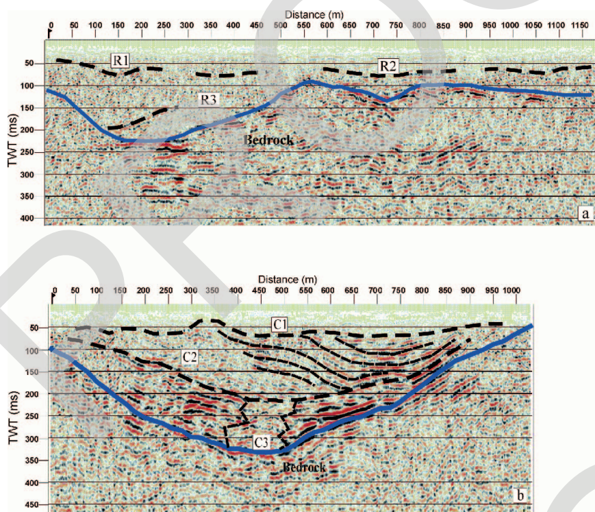
Fig. 10 - Profili sismici e loro interpretazione. In alto: profilo di Rovetta (elemento a in Fig. 9). In basso: profilo di Fiorine (elemento b in Fig. 9). In entrambi i profili il N è a sinistra (da DE FRANCO et alii , 2004).
