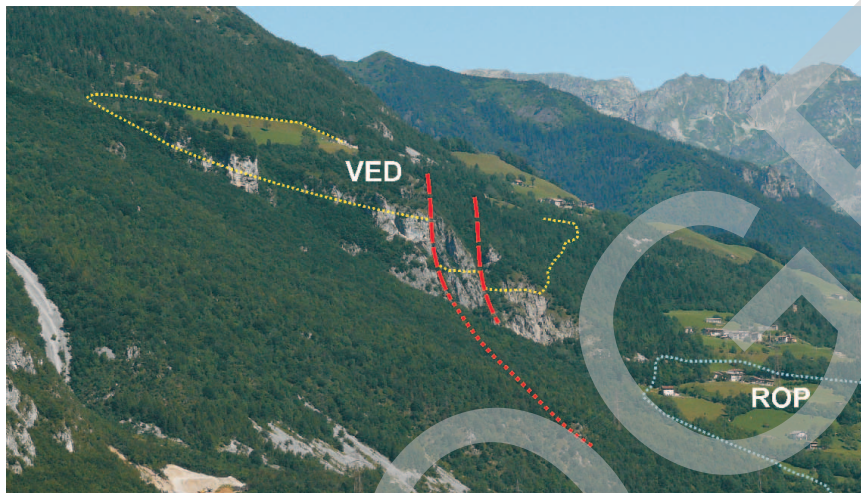
Fig. 18 – Versante orientale del M. Secco: il piastrone dei conglomerati del Vendulo (VED) evidenzia un paleofondovalle sospeso, troncato dalla valle attuale e dislocato da piani di scivolamento gravitativo (in rosso). Il conglomerato di Groppino (ROP) è successivo rispetto alla dislocazione principale da esso suturata (foto C. Ferliga).
