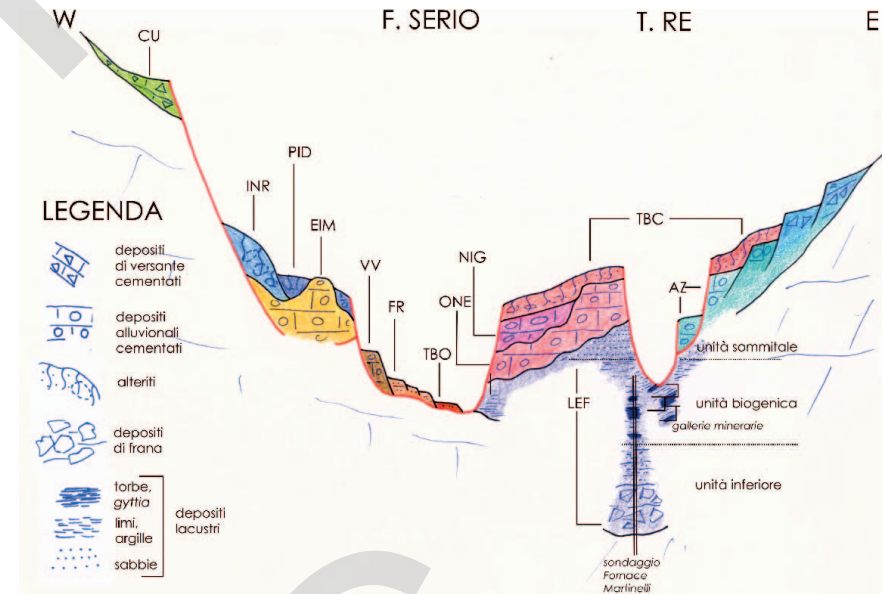
Fig. 22 - Schema dei rapporti stratigrafici fra le unità affioranti nella valle principale a S di Ponte Costone. Scala verticale maggiore rispetto a quella orizzontale.
