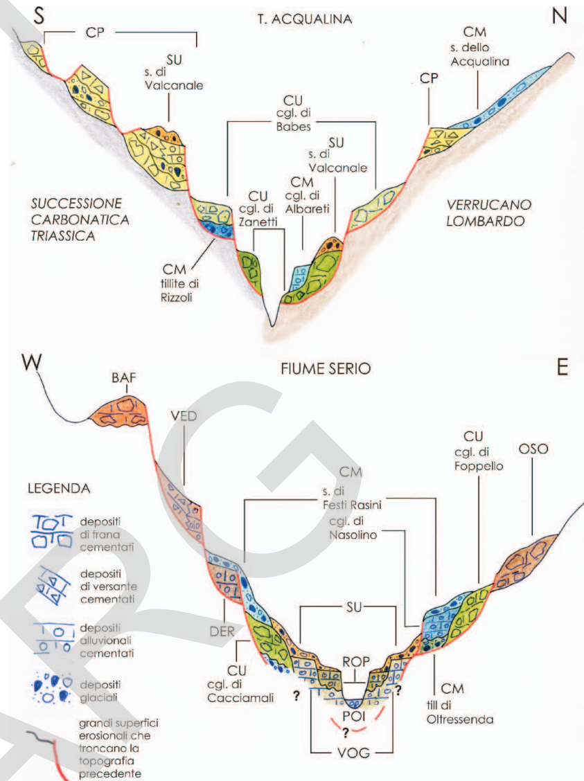
Fig. 19 - Schema dei rapporti stratigrafici fra le unità affioranti nella valle principale a N di Ponte Costone: a) valle del T. Acqualina e asse seriano (in basso). Il conglomerato di Groppino, descritto entro la successione dell'anfiteatro del Serio (3.4.12) ove presenta precise relazioni geometrico-stratigrafiche con le altre unità, viene mantenuto distinto anche entro la valle quale "livello marker" di aggancio fra successioni di eventi non altrimenti correlabili tra loro. Scala verticale maggiore rispetto a quella orizzontale.
