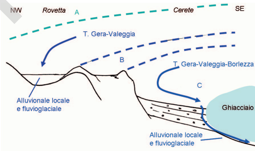
Fig. 8 – Schema delle relazioni fra fronte glaciale, depositi alluvionali locali e fluvio-glaciali camuni desunte dai dati di terreno. A) fase in cui il ghiacciaio colmava tutta l'area; B) fasi in cui il ghiacciaio si affacciava sulla piana di Clusone e la sua piana fluvio-glaciale scendeva verso il Serio; C) fasi in cui il ghiacciaio si attestava in Val Borlezza e sia il drenaggio locale sia le acque di fusione trovavano deflusso verso il Lago d'Iseo, incanalandosi presumibilmente alla base del ghiacciaio stesso. (ridisegnato, da FERLIGA, 2007a).
