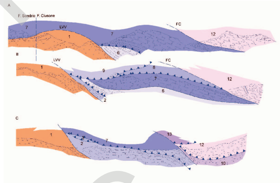
Fig. 25 – A fronte: schema tettonico del Foglio 077-Clusone: sono riconoscibili le unità strutturali inferiori, intermedie e superiori costituite a loro volta da diverse unità tettoniche minori (identificate con numeri). Sopra: nei profili geologici semplificati sono ricostruiti i rapporti tra le principali unità tettoniche riconosciute.
