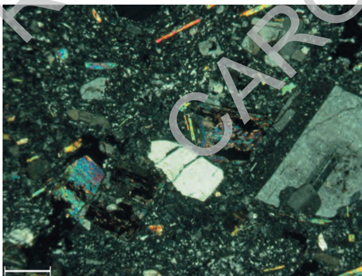
Fig. 43 - Formazione di Monte Macaone. Lava riodacitica. Associazione di plagioclasto, quarzo e biotiti in fondo microcristallino con orientamento fluidale. Microfoto a polarizzatori incrociati (scala di riferimento 675 \mu\text{m} ).
