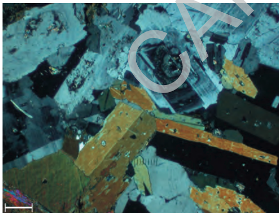
Fig. 70 - Diorite appartenente alla tonalite del Monte Monoccola (TMX). La microfotografia a polarizzatori incrociati mette in evidenza la struttura fanerocristallina ipidiomorfa della roccia, ricca di biotite con orneblenda, plagioclasio labradoritico, quarzo e scarso feldspato alcalino (scala di riferimento 350 µm).
