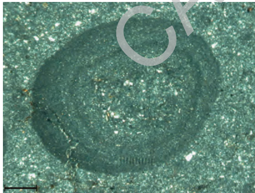
Fig. 34 - Cineriti con lapilli di accrezione a morfologia tondeggianti e zonazione concentrica a grana variabile. Microfoto a polarizzatori incrociati (scala di riferimento 675 \mu\text{m} ).
