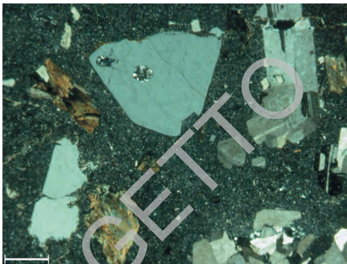
Fig. 42 - Formazione di Monte Macaone. Lava dacitica. Struttura porfirica con fenocristalli di quarzo, plagioclasti, biotite in fondo microgranulare cristallino. Microfoto a polarizzatori incrociati (scala di riferimento 125 \mu\text{m} ).
