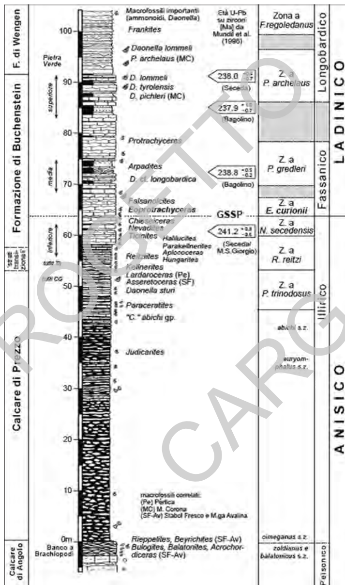
Fig. 107 - Colonna stratigrafica sintetica del Triassico medio esposta lungo l'alveo del Fiume Càffaro presso Romantera (Bagolino). La sigla GSSP indica il livello stratigrafico del "chiodo d'oro" della base del piano Ladinico (modificata da BRACK et alii, 2005). La denominazione delle sottozone (s.z.) per l'Anisico è da MONNET et alii (2008).
