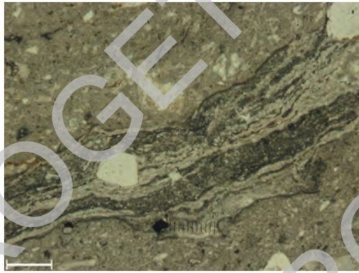
Fig. 33 - Fiamme pomicee rinsaldate orientate lungo la direzione del flusso piroclastico. Microfoto a polarizzatori paralleli (scala di riferimento 125 \mu\text{m} ).
