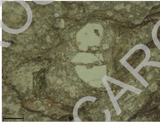
Fig. 37 - Membro di Val Dorizzo - Litofacies piroclastica. Quarzo fratturato e dislocato. Microfoto a polarizzatori paralleli (scala di riferimento 400 \mu\text{m} ).
