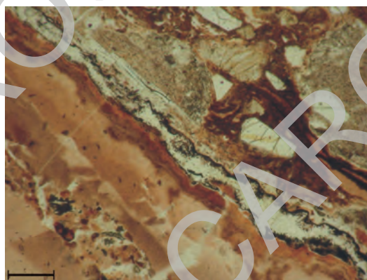
Fig. 58 - Ciottolo di selce nel conglomerato del Verrucano Lombardo a tetto della litozona superiore della vulcanite di Auccia a Punta dell'Auccia. Tali selci di origine idrotermale sono abbondanti negli ultimi episodi vulcanici della litozona superiore della vulcanite di Auccia. Microfoto a polarizzatori paralleli (scala di riferimento 675 \mu\text{m} ).
