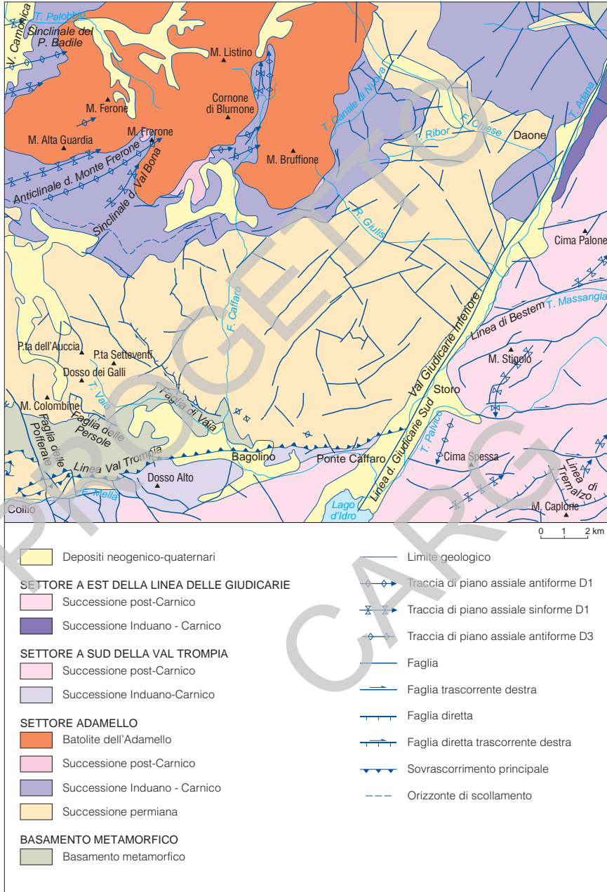
Fig. 92 - Schema tettonico del Foglio 079-Bagolino.
