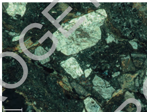
Fig. 38 - Membro di Val Dorizzo - Litofacies piroclastica. Plagioclasti idiomorfi associati a biotiti deformate. Microfoto a polarizzatori incrociati (scala di riferimento 400 µm).
