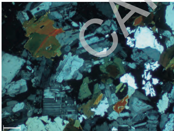
Fig. 69 - Tonalite del Lago della Vacca (LGV). Microfotografia a polarizzatori incrociati. Struttura granulare ipidiomorfa con abbondanti plagioclasti labradoritico-andesinici associati a biotite, orneblenda e quarzo (scala di riferimento 350 µm).
