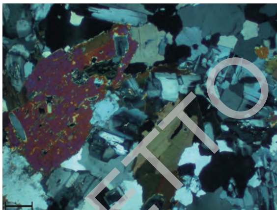
Fig. 67 - Tonalite del Monte Alfa Guardia (TMG). Microfotografia a polarizzatori incrociati. Struttura granulare ipidiomorfa con abbondanti plagioclasti labradoritico-andesinici associati a biotite, ortoclasti, quarzo e K-feldspato interstiziale (scala di riferimento 350 \mu\text{m} ).
