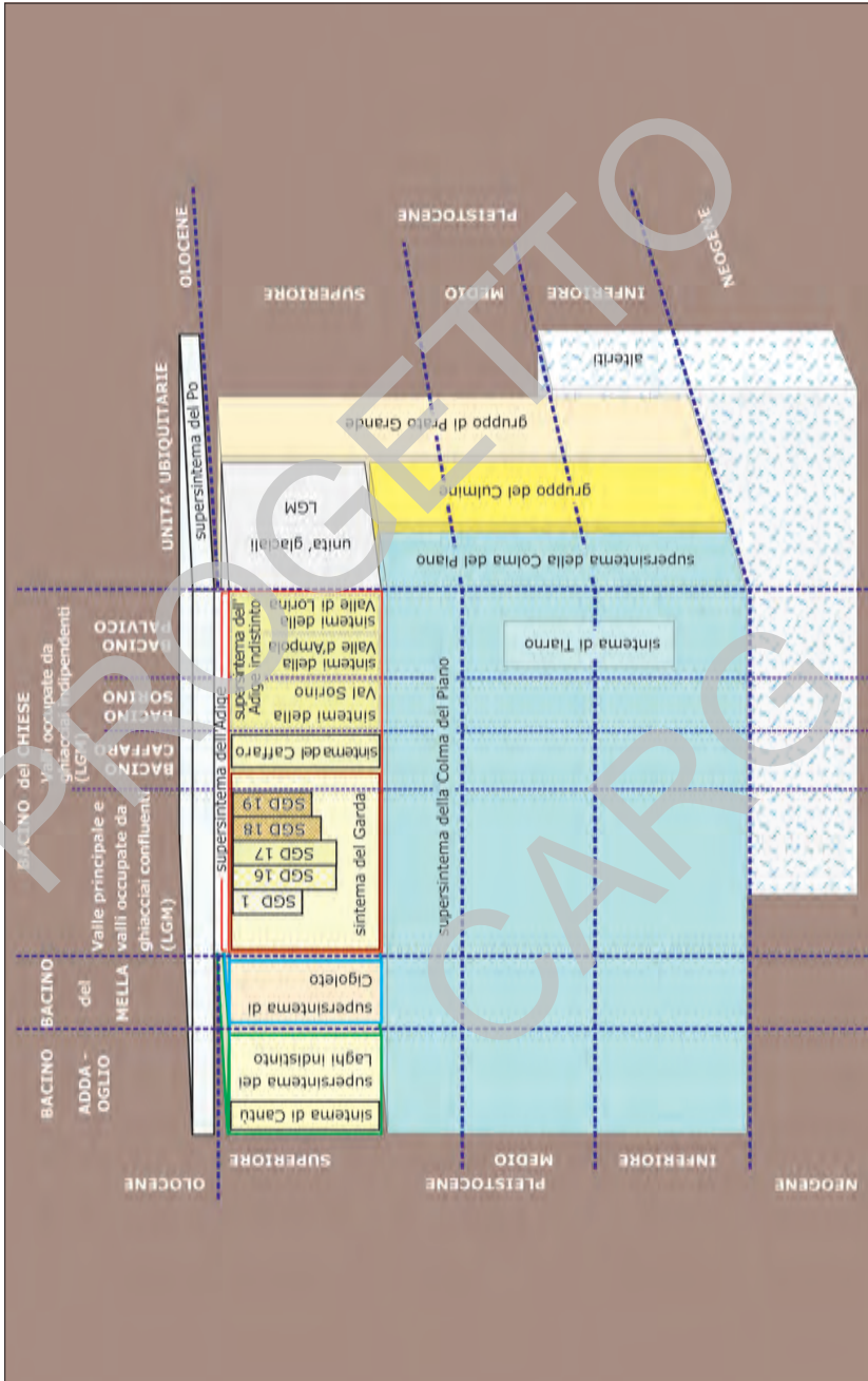
Fig. 77 - Schema dei rapporti stratigrafici delle unità continentali neogenico-quaternarie presenti entro il Foglio 079-Bagolino.
