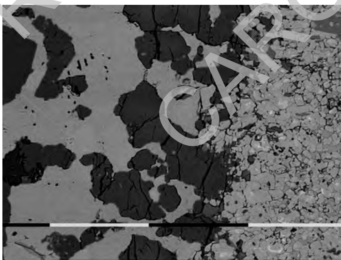
Fig. 76 - Breccia del Pissalat (BPA). Microfotografia SEM, scala di riferimento 0,1 mm. Dettaglio della fascia a silicati con cristalli di forsterite in calcite (lato destro) e associazione di granuli di diopside, calcite e tremolite (lato sinistro).
