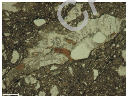
Fig. 39 - Litozona delle peliti con pomici. Visione generale, presenza di pomici inglobate da matrice pelitica microcristallina. Microfoto a polarizzatori paralleli (scala di riferimento 675 µm).
