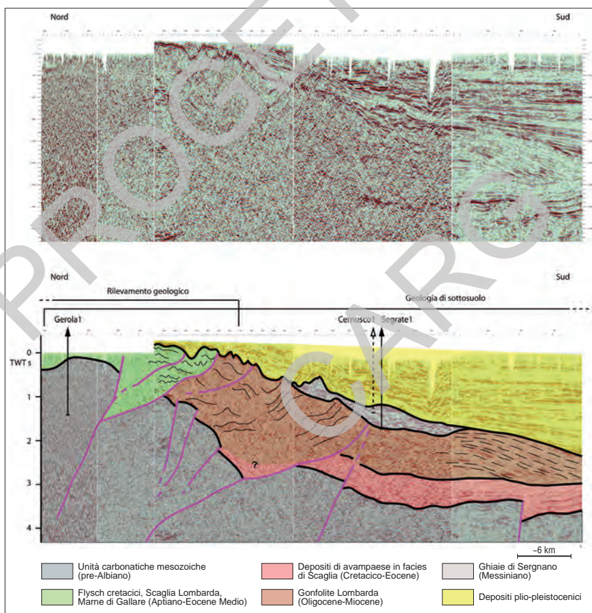
Fig. 4 - Sezione sismica esemplificativa dello stile strutturale presente nel settore orientale del Foglio 096-Seregno (per gentile concessione di ENI).
