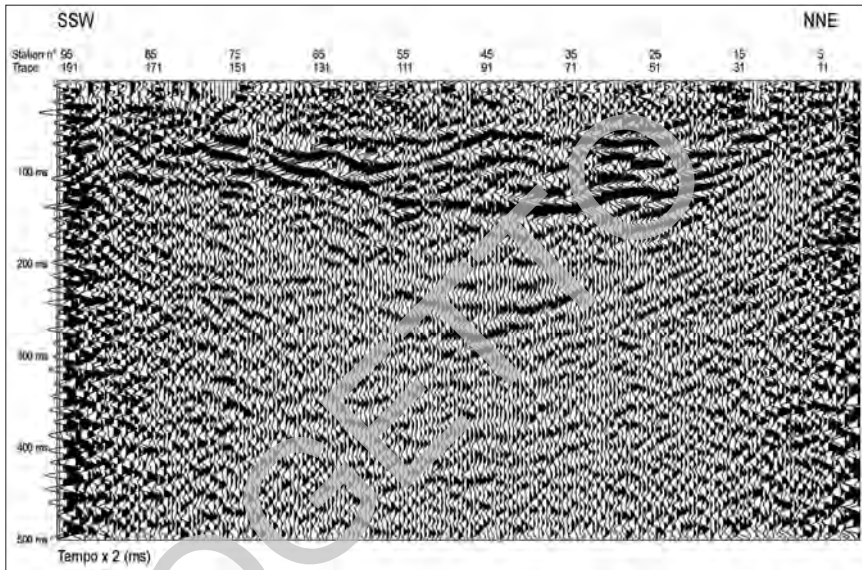
Fig. 6a - Profilo sismico a riflessione lungo la Linea 1b, che evidenzia un profilo paleovallivo colmato da due corpi lenticolari sovrapposti.
