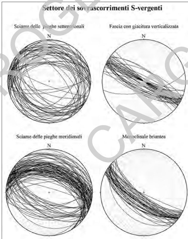
Fig. 31 - Proiezione stereografica equiareale (emisfero inferiore) delle giaciture S_0 misurate nel Settore dei sovrascorrimenti S-vergenti.
