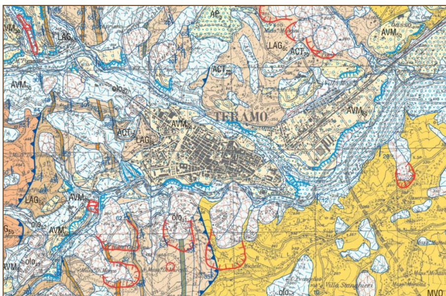
Figura 2.6.8 – Stralcio del Foglio 339 "Teramo" della Carta geologica d'Italia in scala
