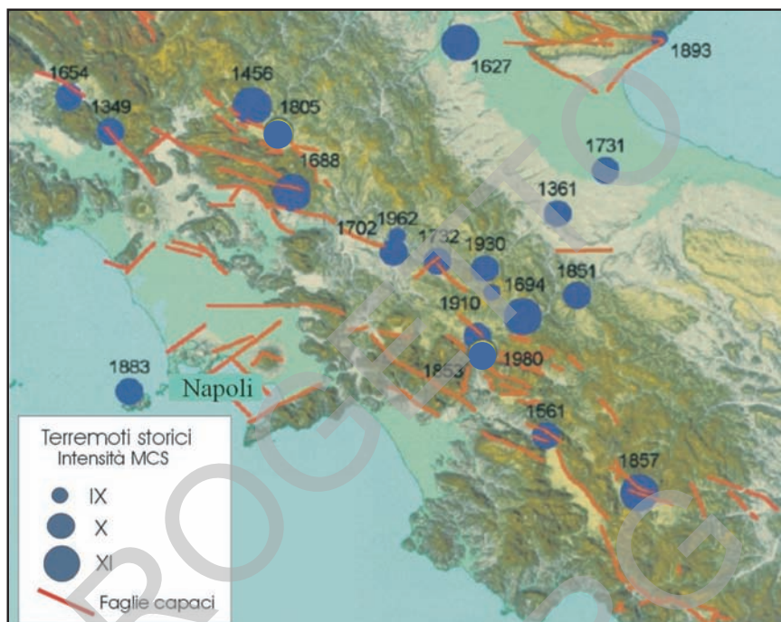
Fig. 41 - Epicentri dei terremoti storici lungo la fascia dell'Appennino Meridionale con I > IX MCS e rappresentazione delle faglie capaci (dati derivanti dal CPTI, 1999 e dal data base ITHACA, MICHETTI et alii, 2000)
