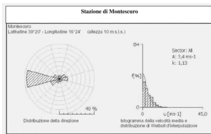
Figura 13.2 Distribuzione della direzione e istogramma della velocità del vento
