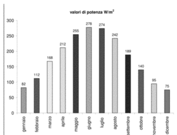
Figura 13.6 - Valori di potenza media mensile
