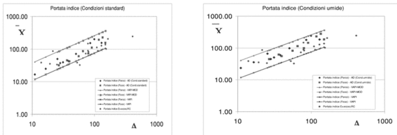
Figura 14.4-Inviluppo delle portate indici calcolate con la procedura VAPI e con il modello di trasformazione afflussi-deflussi nell'ipotesi di condizioni molto umide del suolo
