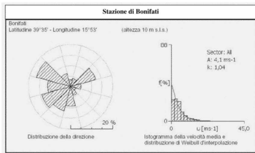
Figura 13.1 Distribuzione della direzione e istogramma della velocità del vento
