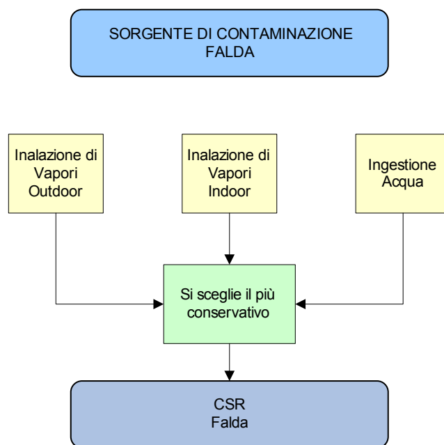
Figura 4.9 - Criterio di cumulazione dovuto a più vie d'esposizione per la falda
