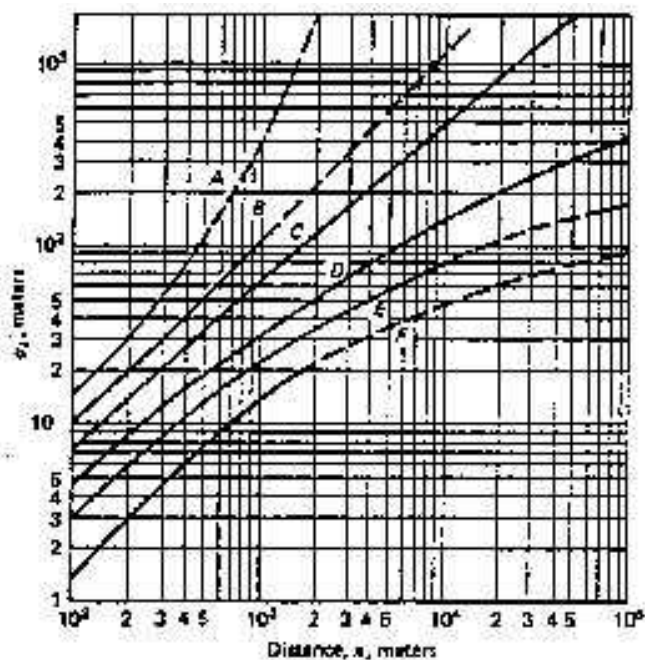
Figura 3.13: Coefficiente di dispersione trasversale
