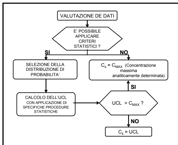
Figura 3.5: Criterio per la selezione della concentrazione rappresentativa alla sorgente ( C_s )
