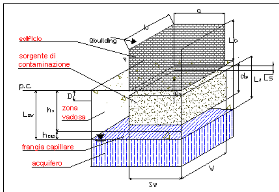
Figura 3.14: MCS: sorgente di contaminazione nel suolo insaturo ed edificio fuori terra
