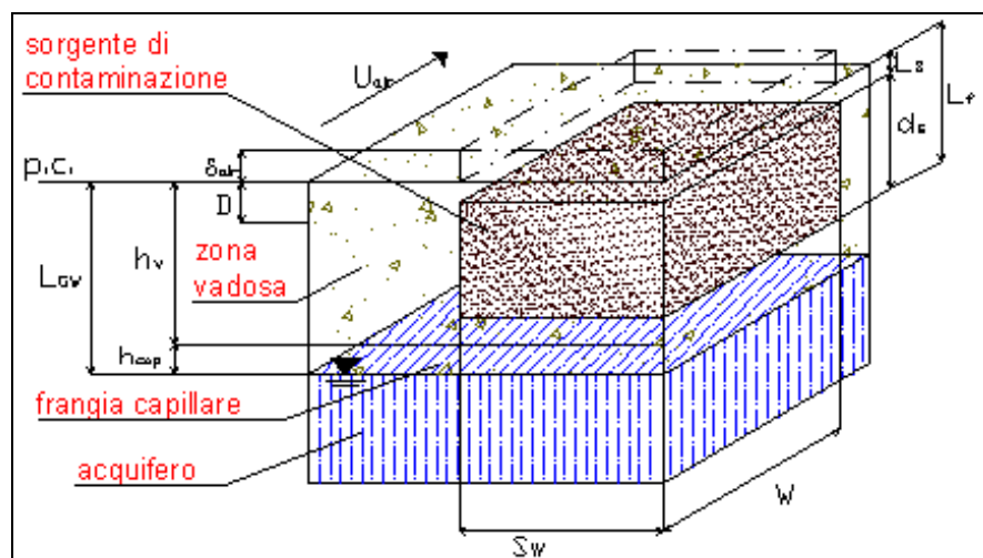
Figura 3.10: MCS: sorgente di contaminazione nel suolo insaturo
