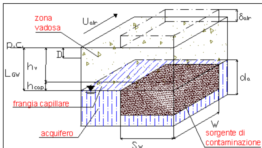
Figura 3.11: MCS: sorgente di contaminazione nel suolo saturo
