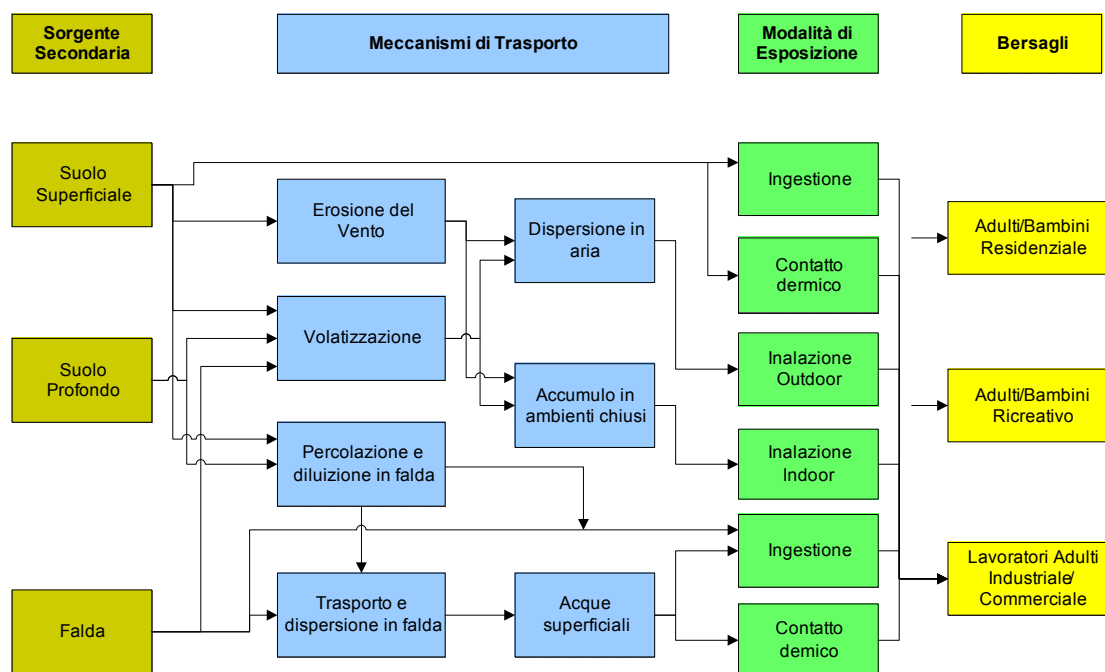
Figura 3.1: Definizione del modello concettuale: diagramma di flusso
