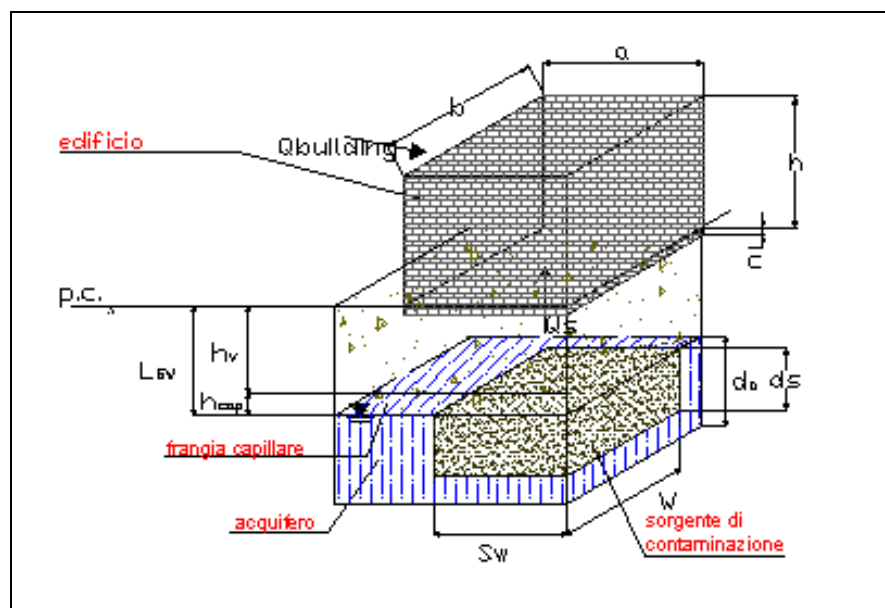
Figura 3.17: MCS: sorgente di contaminazione nel suolo saturo ed edificio parzialmente interrato
