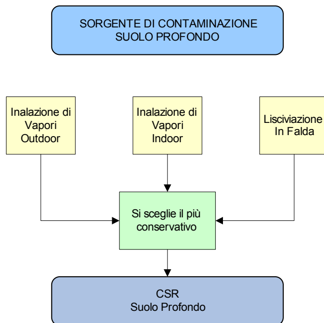
Figura 4.8 - Criterio di cumulazione dovuto a più vie d'esposizione per il suolo profondo
