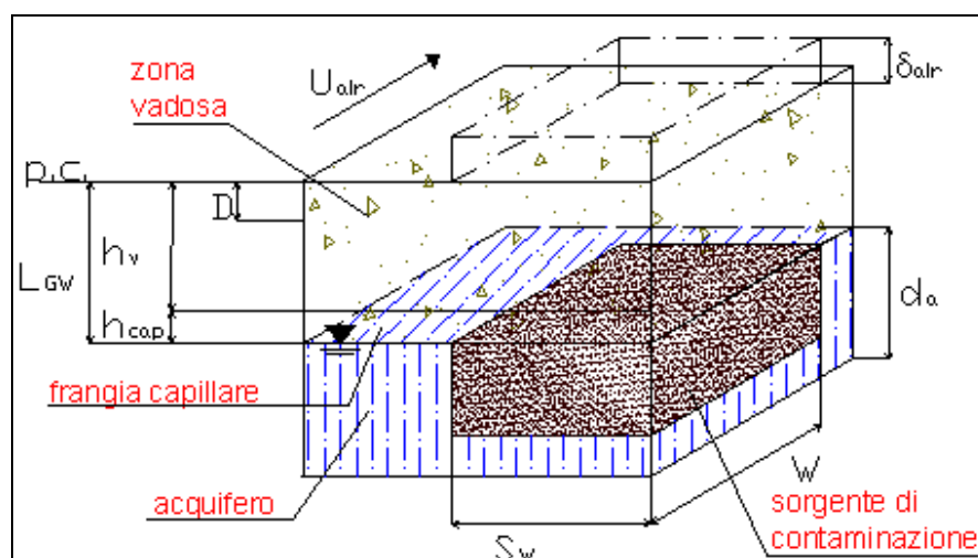
Figura 3.3: Geometria del sito e della sorgente di contaminazione in zona satura.
