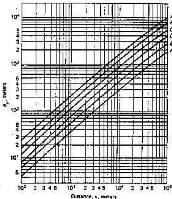
Figura 3.12 Coefficiente di dispersione verticale
