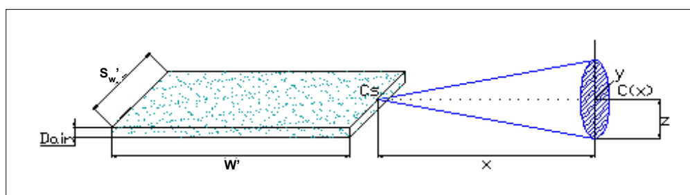
Figura 3.22: Modello gaussiano di dispersione in atmosfera
