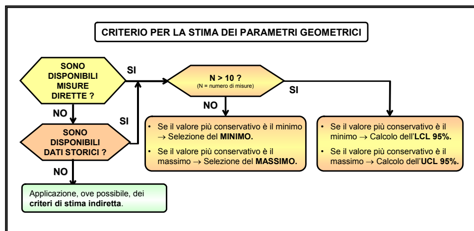
Figura 3.4: Procedura per la stima dei parametri geometrici.
