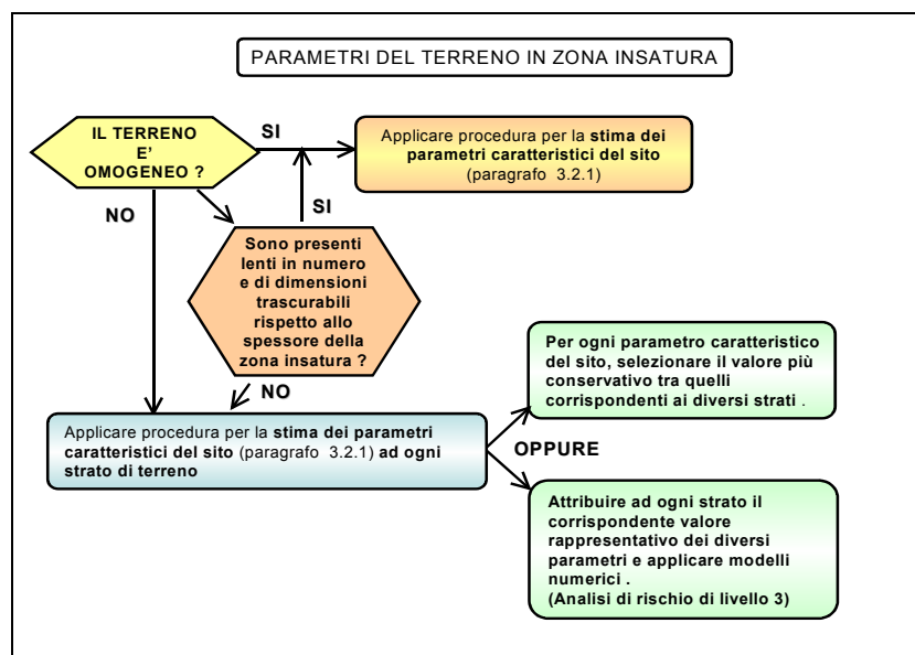
Figura 3.8: Procedura per i parametri della zona insatura.
