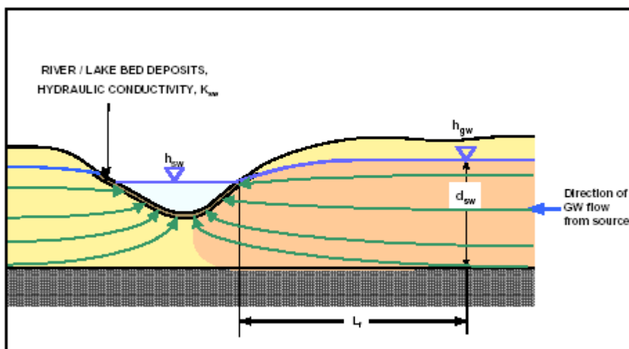
Figura 3.18: Schema per il calcolo della cadente piezometrica falda-corpo idrico ricevente
