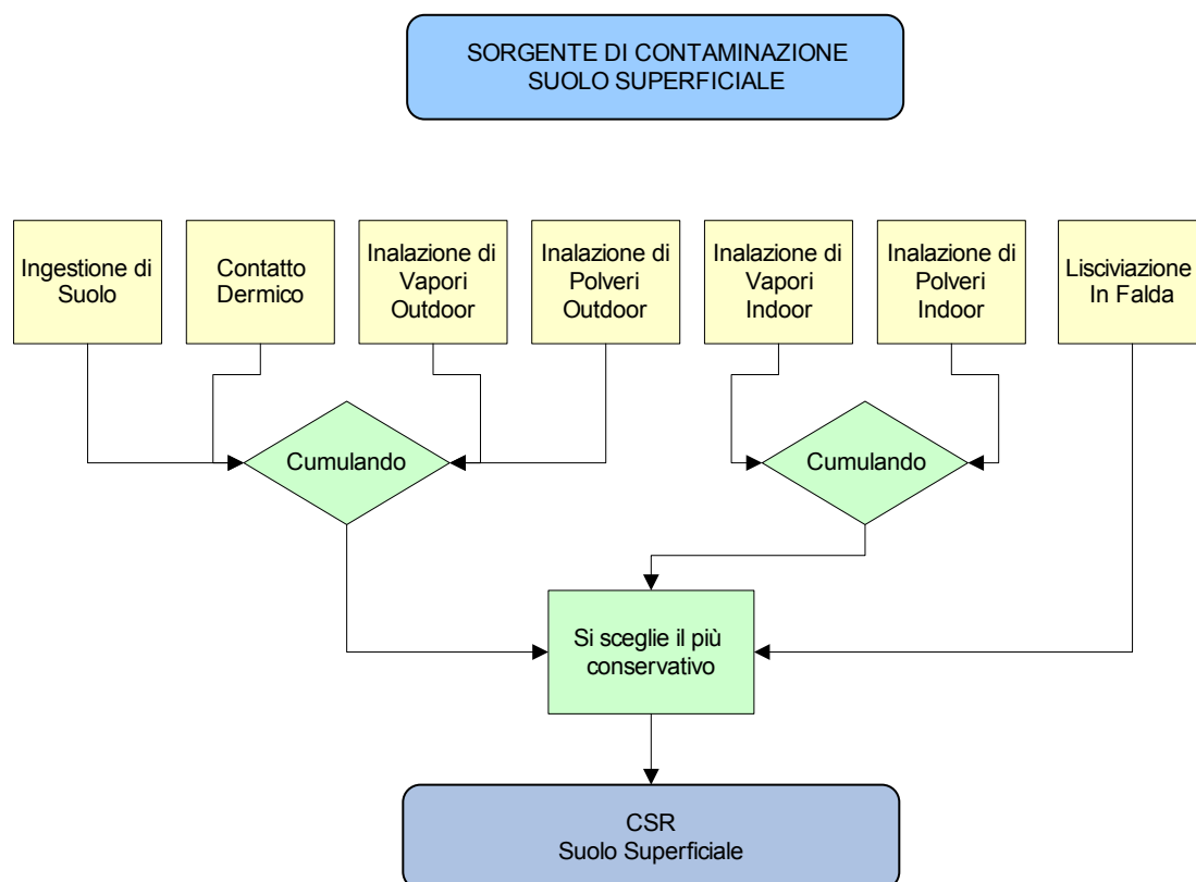
Figura 4.7: Criterio di cumulazione dovuto a più vie d'esposizione per il suolo superficiale
