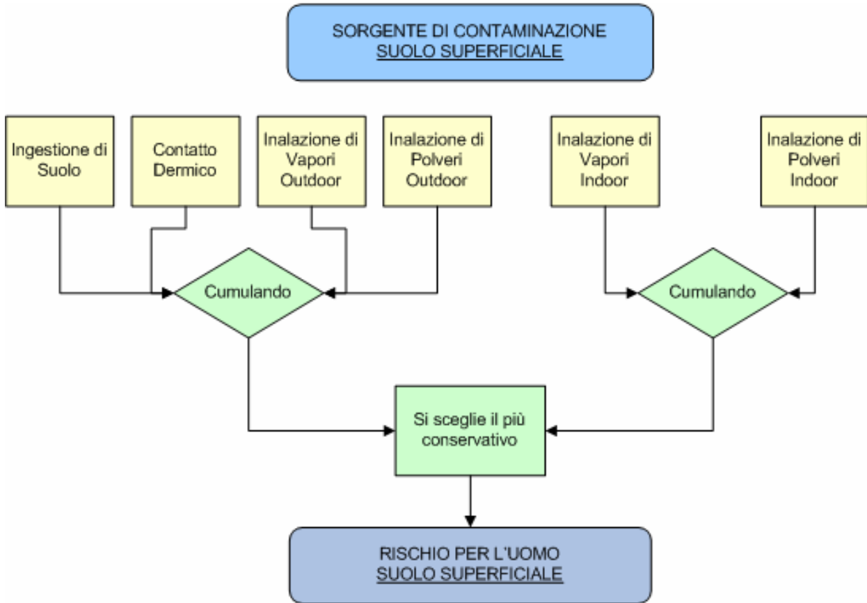
Figura 4.2 – Criterio di calcolo del rischio individuale dovuto a più vie di esposizione per suolo superficiale
