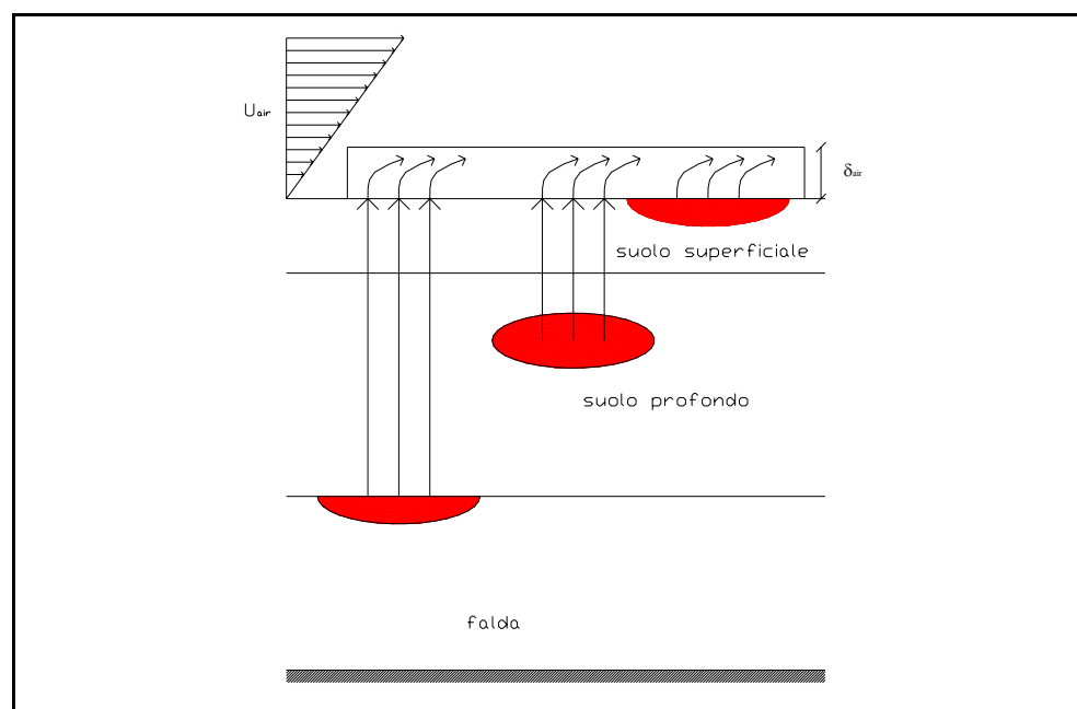
Figura 3.21: Volatilizzazione di vapori in ambienti aperti (outdoor)
