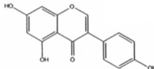
ISOFLAVONE (Genistein) Mol. Wt.: 270
