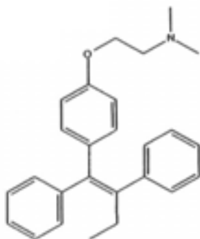
TAMOXIFEN Mol. Wt.: 372
