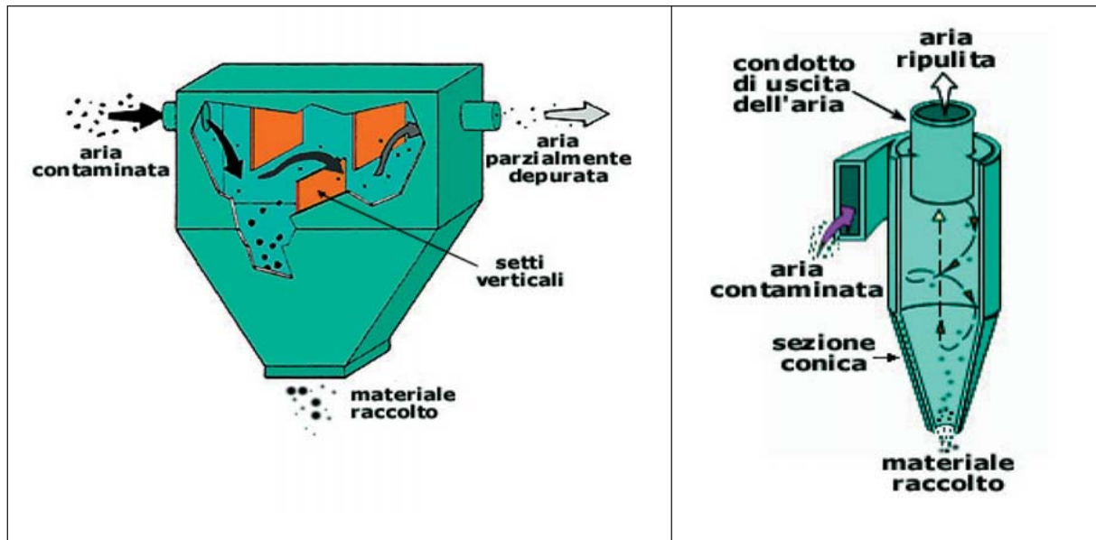
Figura 6.1: Camera a deposizione
