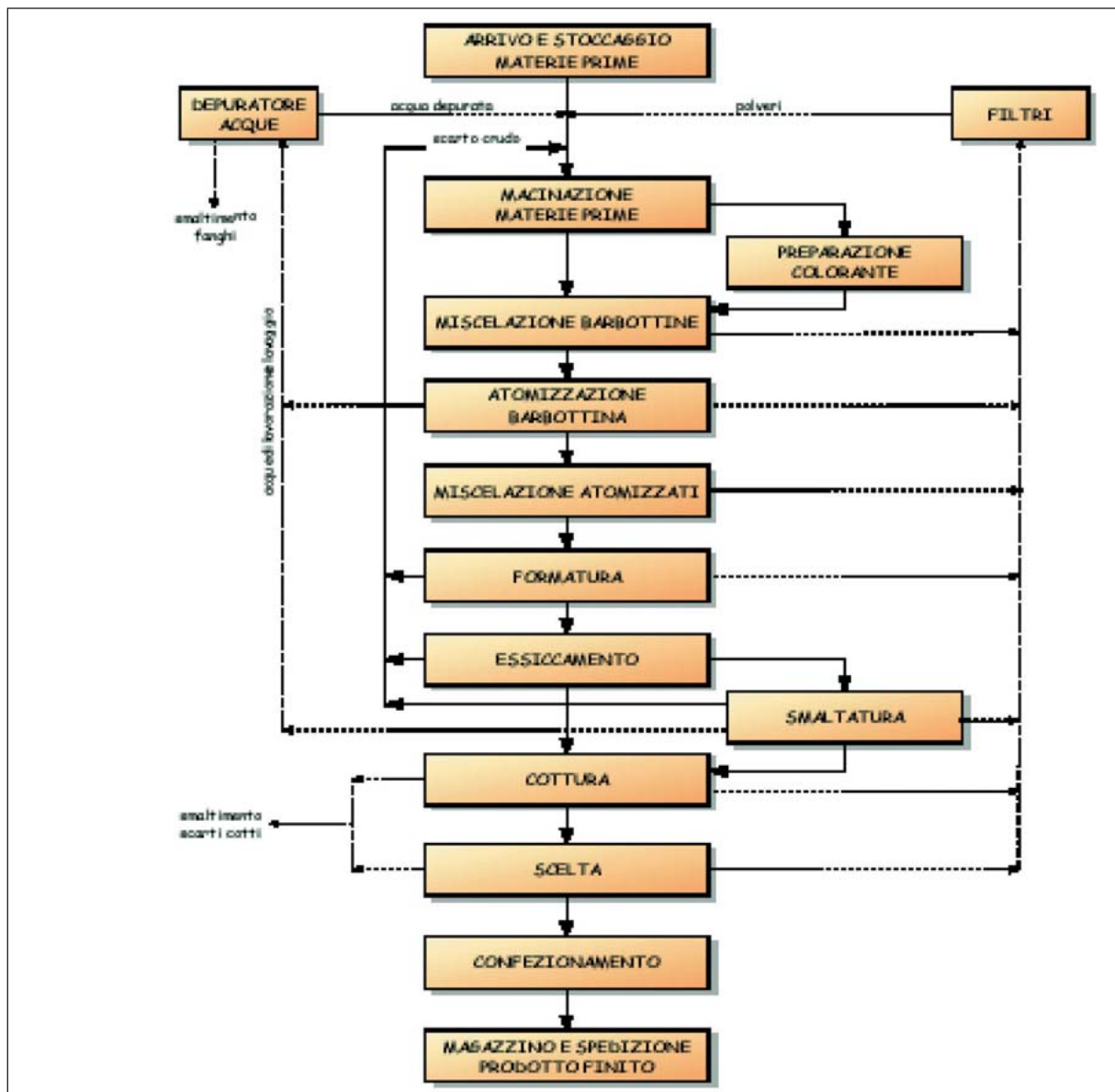
Figura 2.6: Diagramma di flusso del comparto ceramico
