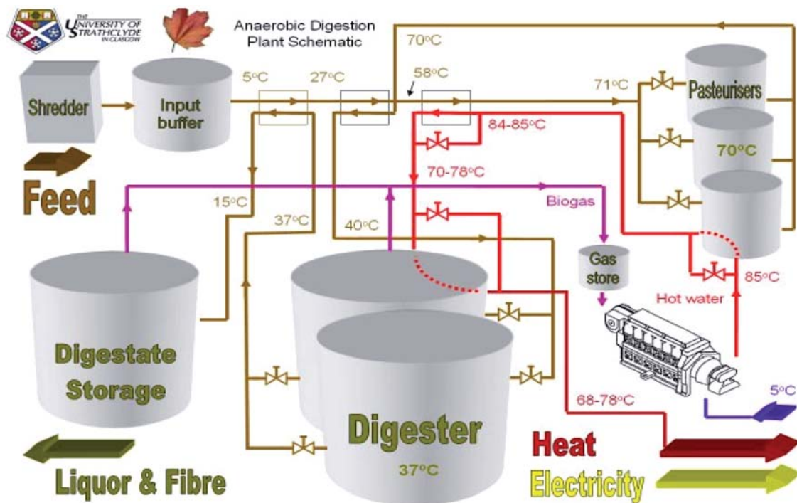
Figura 1 - Schema particolareggiato di un impianto di digestione
