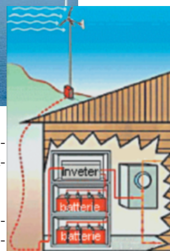
Figura 20. Piccolo impianto eolico
