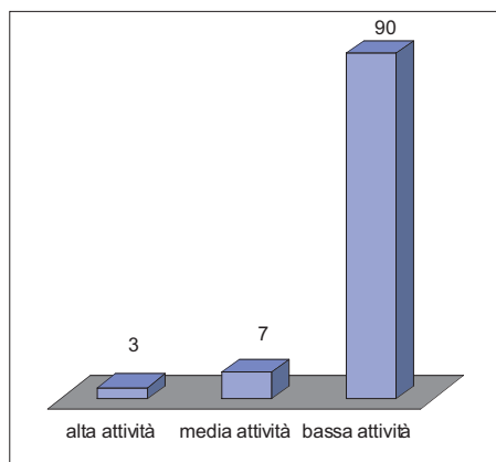
Figura 39. Rifiuti radioattivi per una centrale nucleare da 1000MW (m 3 all'anno)
