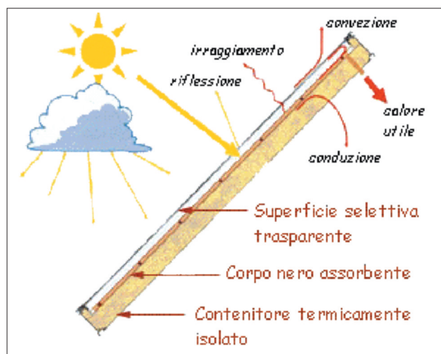
Figura 5. Schema collettore piano
