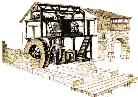
Figura 23. Primi mulini ad acqua
