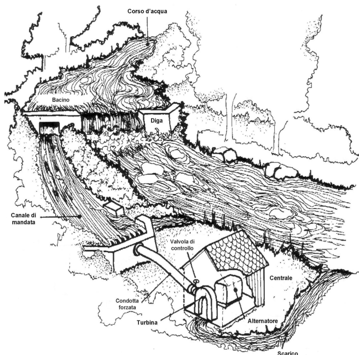
Figura 24. Schema-tipo di installazione idroelettrica
