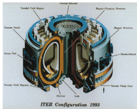
Figura 41. Schema di un apparecchio sperimentale per ottenere la fusione nucleare tramite confinamento magnetico
