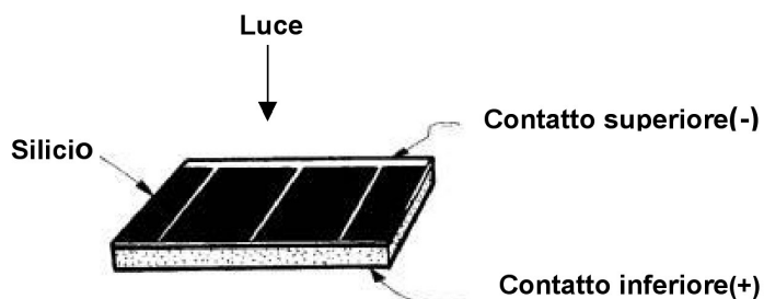
Figura 10. Conformazione esteriore di una cellula fotovoltaica. Il contatto superiore identifica il morsetto negativo del componente, quello inferiore corrisponde al polo positivo del generatore di tensione.
