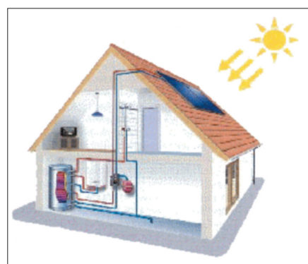
Figura 6. Impianto termosolare. Tutti gli edifici che dispongono di uno spazio soleggiato (tetto inclinato, tetto terrazato, giardino, ecc.) possono essere dotati di un impianto solare per la produzione di acqua calda sanitaria.
