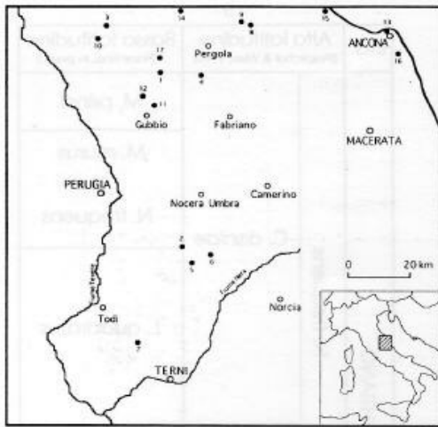
Fig. 3 - Ubicazione delle sezioni citate nel testo: 1) Valdorbia; 2) Pale; 3) Infernaccio, Presale e Piobbico; 4) Fonte Avellana; 5) Monte Serrone; 6) Monte Civitella; 7) Pozzale; 8) Torrente Bosso; 9) Fonte Giordano; 10) S.S. Apecchiese; 11) Gola del Bottaccione; 12) Valle della Contessa; 13) Monte Conero; 14) Montebello d'Urbino; 15) Senigallia; 16) Camerano; 17) Moria.
