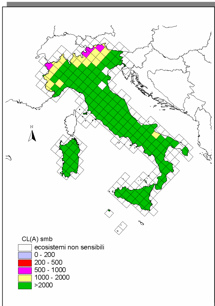
Mappa dei carichi critici di acidità (equivalenti di idrogeno x ettaro x anno), calcolata con la metodologia del bilancio chimico di massa riportata nel Manuale dei carichi critici.
