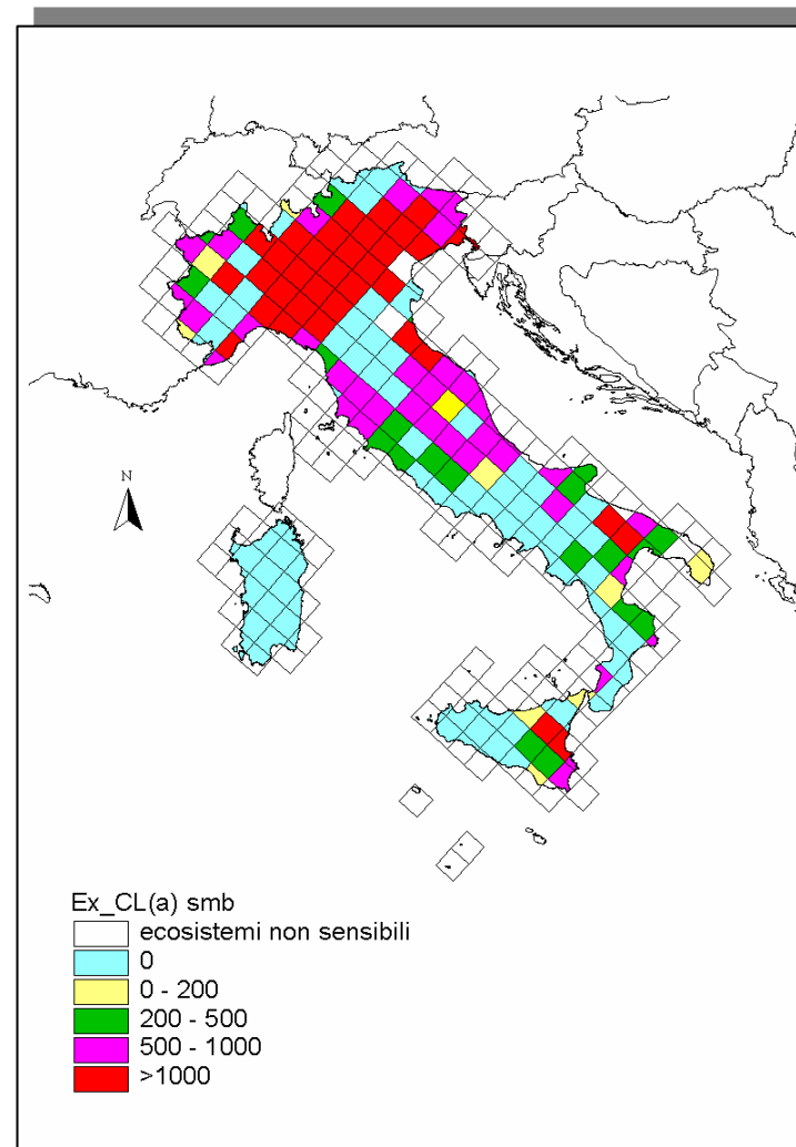
Mappa delle eccedenze di acidità (equivalenti di idrogeno x ettaro x anno). Le deposizioni sono calcolate su dati EMEP riferiti al 1999.
