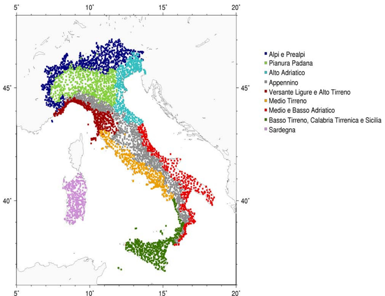
Figura 9.1: L'Italia divisa in nove aree climatiche.
