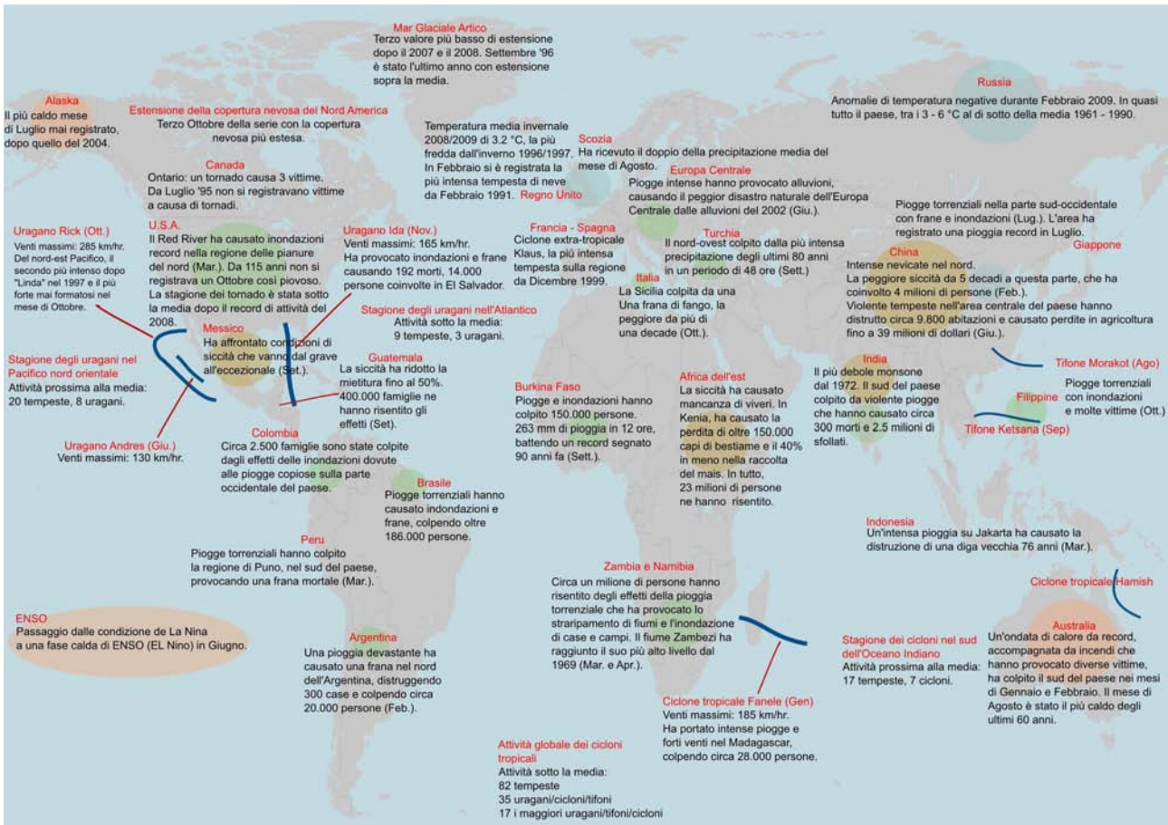
Figura 2.2: Sintesi delle principali anomalie climatiche globali verificatesi nel corso del 2009. Fonte: NOAA .
