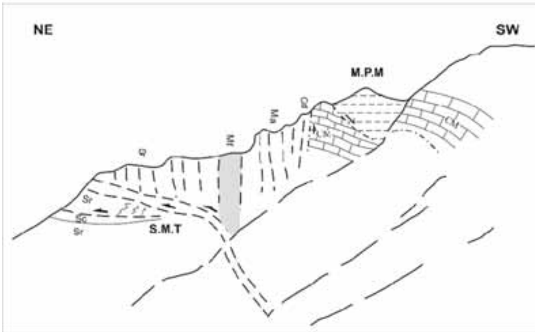
Figure 3.14 - Panoramic view of the Sibillini Mts thrust, looking towards Pizzo di Meta Mt.. CM (Calcere Massiccio); Cd (Calcari Diasprini); Ma (Maiolica); Mf (Fucoidi); Sr (Scaglia Rossa); Sc (Scaglia cinerea).
