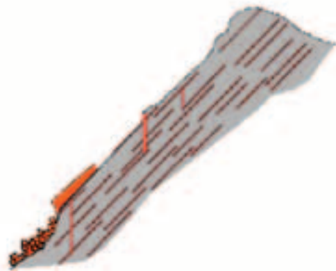
Figure 31 - Images from the "Progetto Geositi": The Colle delle Finestre Landslide (Artwork by Baggio, 2001).
