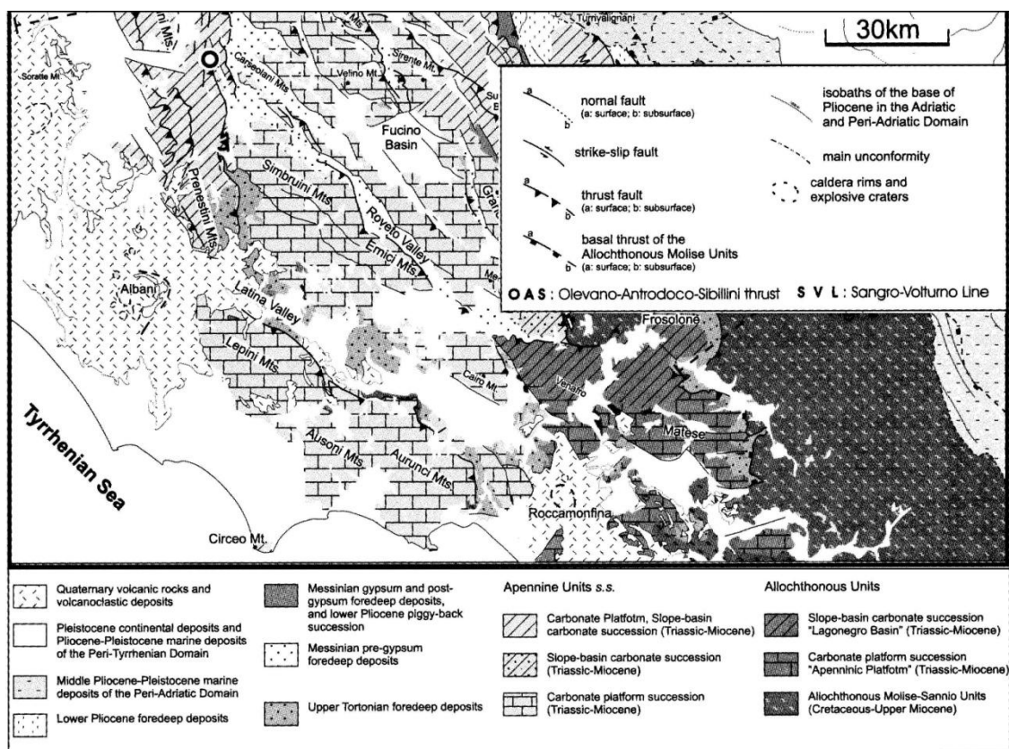
Fig. 12 – Carta geologico-strutturale, da Calamita F. et alii (2006), modificata.
