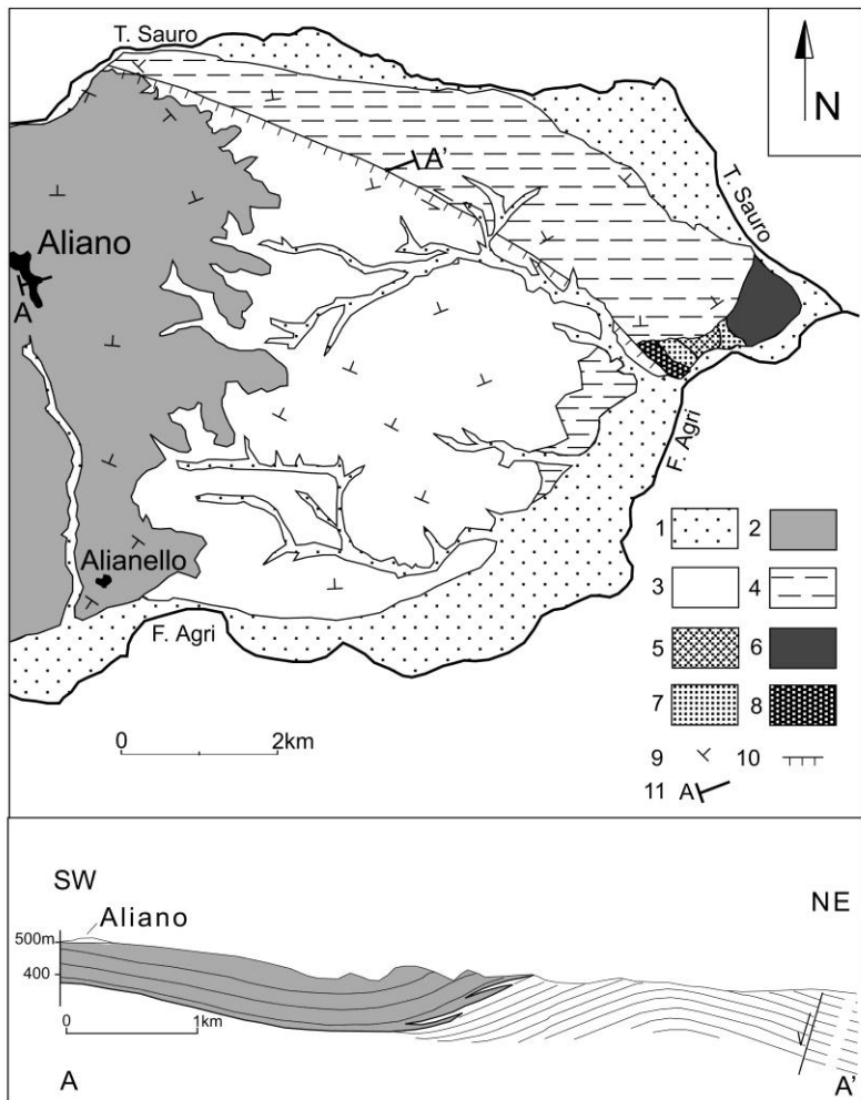
Fig. 5 – Carta e sezione geologica dell'area orientale di Aliano. 1 - Depositi alluvionali attuali e recenti. 2 - Sabbie di Aliano - Ciclo del Sauro (Pliocene sup.-Pleistocene inf.). 3 - Argille grigio-azzurre - Ciclo del Sauro (Pliocene sup.-Pleistocene inf.). 4 - Argille grigio-azzurre - Ciclo di Caliandro (Pliocene medio-sup.). 5 - Marne arenacee di Serra Cortina (Langhiano inf.-Serravalliano). 6 - Arenarie di Corleto (Oligocene sup.-Miocene inf.). 7 - Argille varicolori superiori (Oligocene). 8 - Formazione di Monte Sant'Arcangelo (Cretaceo sup.-Eocene). 9 - Giacitura degli strati. 10 - Faglia. 11 - Traccia sezione.
