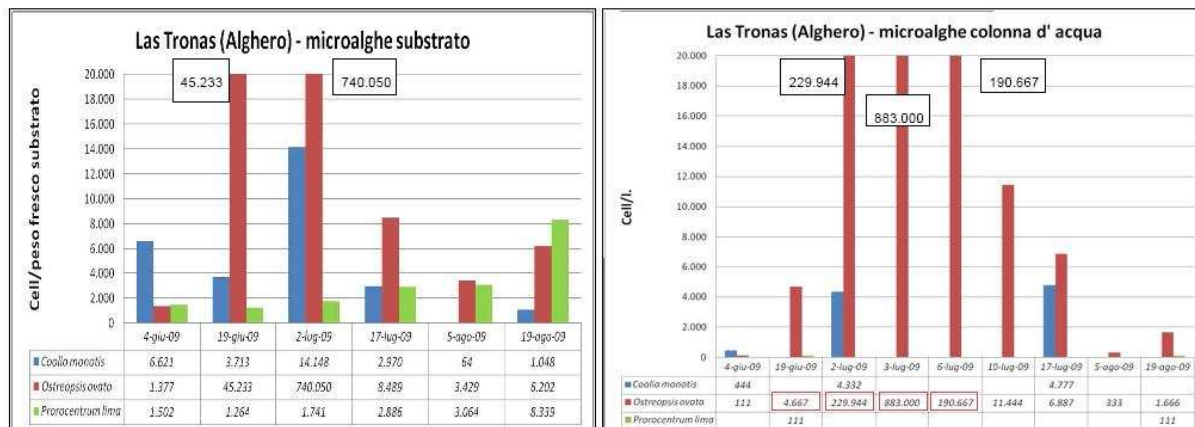
Figure 12.4 e 12.5 – Concentrazioni delle microalghe su substrato e in colonna d'acqua
