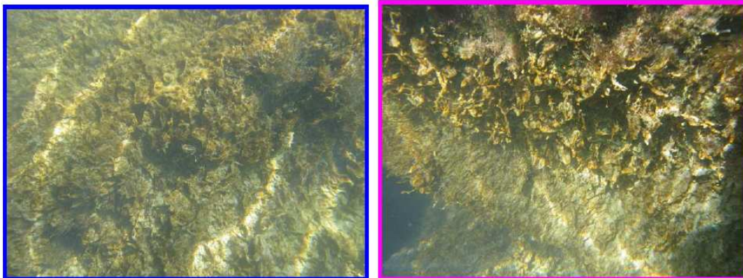
Figure 14.16, 14.17 – Litorale Pisano: mucillagine su substrato
