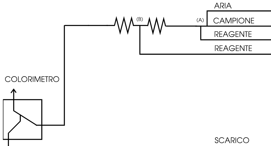
Fig. 5 - Manifold per il dosaggio di \text{PO}_4 .
