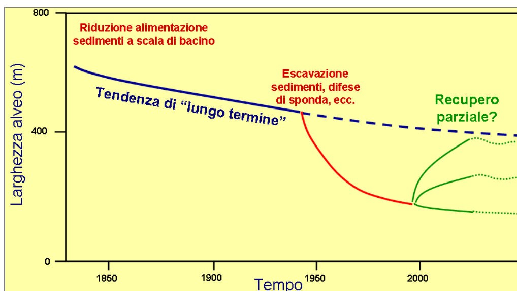
Figura 3.1 – Schema evolutivo delle larghezze osservate in alcuni tratti del F. Magra. (Modificato da RINALDI et al., 2008 ): sovrapposizione del trend di lungo termine, legato a variazioni di produzione di sedimenti a scala di bacino, con il trend determinato dalla fase di maggiore di disturbo legata all'escavazione di sedimenti, e successivo parziale recupero morfologico.
