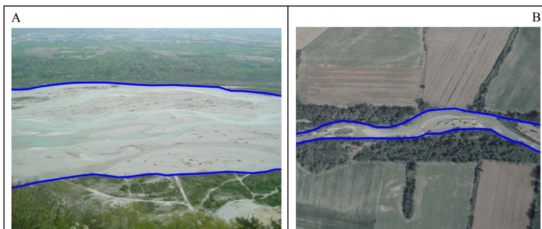
Figura 4.6 – Delimitazione dell'alveo per corsi d'acqua sufficientemente larghi (larghezza > 30 m).
