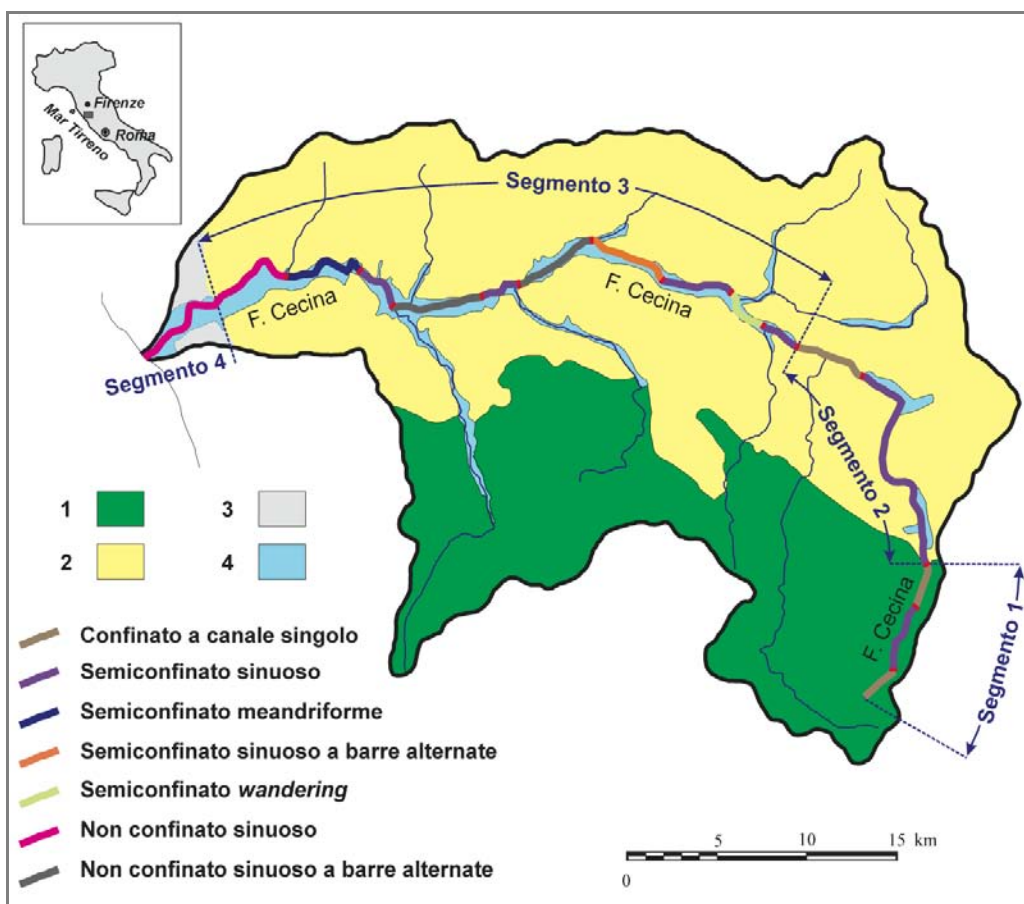
Figura 4.29 – Esempio di suddivisione dei segmenti del Fiume Cecina in tipologie sulla base di confinamento e morfologia.
