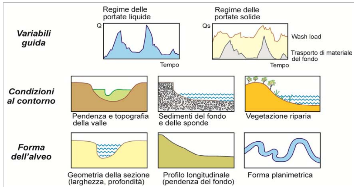
Figura 2.7 – La forma di un alveo alluvionale come risultato dell'interazione tra variabili guida e condizioni al contorno.
