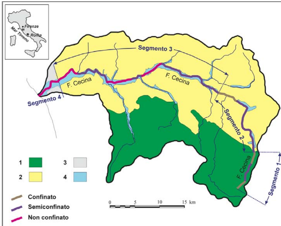
Figura 4.4 – Esempio di suddivisione dei segmenti del Fiume Cecina in base al confinamento. (A seguito di questo STEP sono stati individuati preliminarmente i tratti: 1: Unità collinare-montuosa; 2: unità collinare; 3: unità di pianura costiera; 4: depositi alluvionali).
