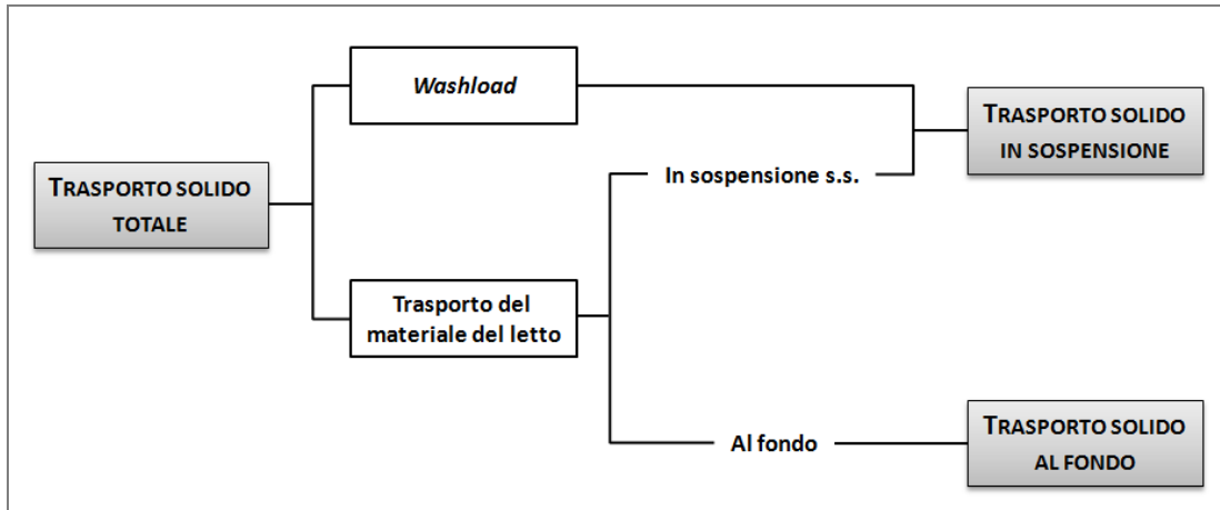
Figura 2.12 – Tipologie di trasporto solido.
