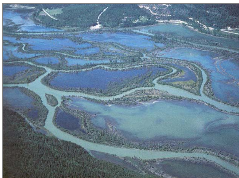
Figura 4.16 – Alveo anastomizzato. Si riconoscono i canali e le isole inondate a seguito di un evento di piena.
