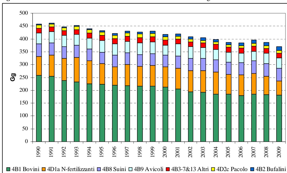
Figura 3.1 - Serie storica delle emissioni nazionali di ammoniaca dall'agricoltura dal 1990 al 2009
