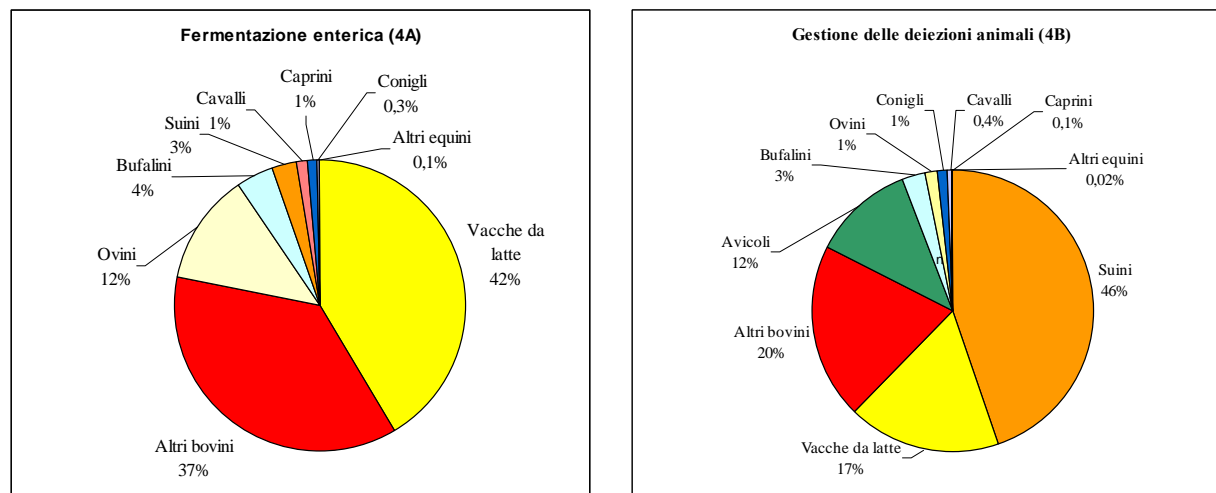
Figura 3.6 - Ripartizione delle emissioni nazionali di metano per 4 A 4 B e per categoria zootecnica, anno 2009
