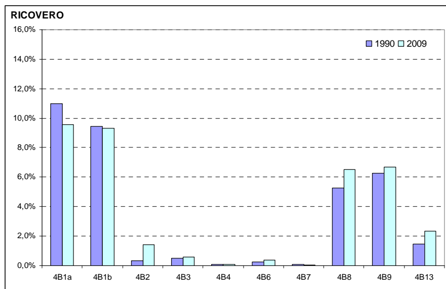
Figura 3.2 – Ripartizione delle emissioni nazionali di ammoniaca per la categoria 4B per fasi e per categoria zootecnica
