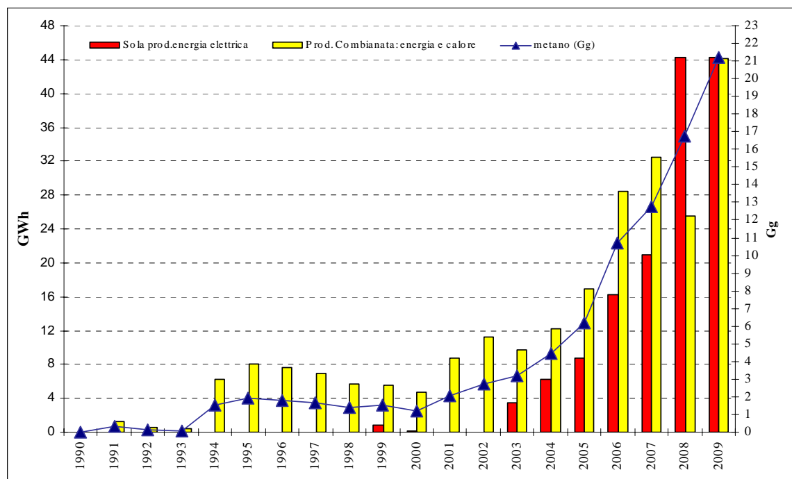
Figura 2.2 - Serie storica della produzione lorda di biogas e quantità di metano recuperato dalle deiezioni animali dal 1990 al 2009
