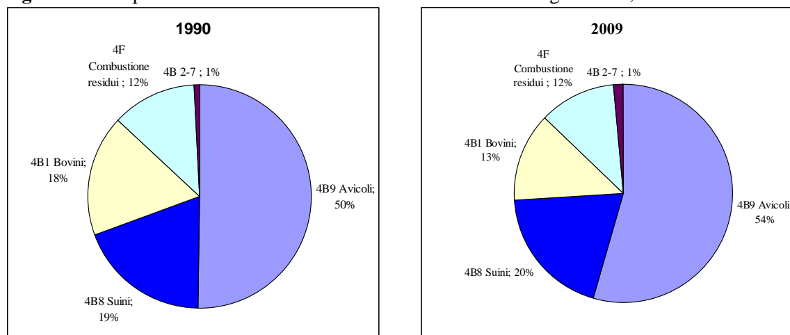
Figura 3.9 – Ripartizione delle emissioni nazionali di PM10 dall'agricoltura, anno 1990 e 2009
