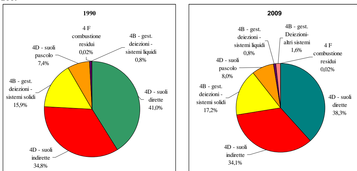
Figura 3.7 – Ripartizione delle emissioni nazionali di protossido di azoto dall'agricoltura, anni 1990 e 2009
