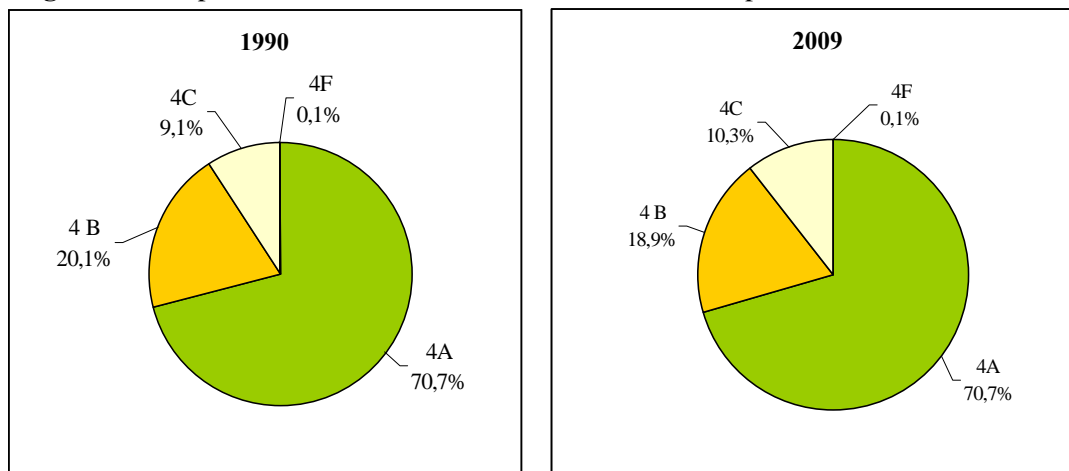
Figura 3.5 - Ripartizione delle emissioni nazionali di metano per fonti emissive, anni 1990 e 2009
