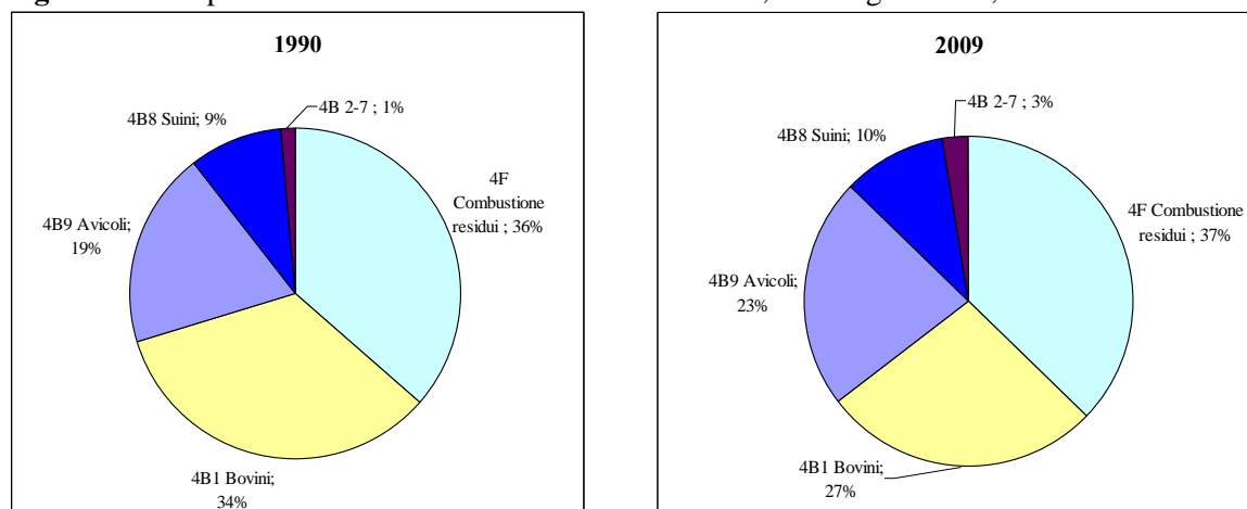
Figura 3.8 – Ripartizione delle emissioni nazionali di PM2,5 dall'agricoltura, anno 1990 e 2009
