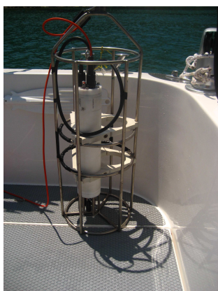
Figura 4.1 – Sonda parametrica
