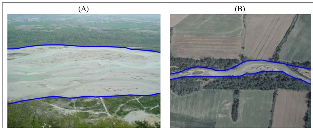
Figura 4.6 – Delimitazione dell'alveo per corsi d'acqua sufficientemente larghi (larghezza > 30 m). Le linee blu rappresentano le sponde dell'alveo. (A) Esempio relativo a un tratto del fiume Togliamento; (B) Esempio relativo a un tratto del fiume Cecina.
