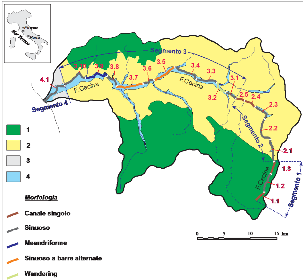
Figura 4.24 – Fase di suddivisione iniziale: esempio relativo al fiume Cecina. A conclusione della Fase 1 sono stati individuati 19 tratti. I tratti 2.1, 2.2 e 2.3 derivano dalla suddivisione di un precedente tratto sulla base di forti variazioni dell'indice di confinamento (ovvero della larghezza della pianura), mentre i tratti 2.4 e 2.5 derivano dalla confluenza di un importante affluente. 1: unità collinare-montuosa; 2: unità collinare; 3: unità di pianura costiera; 4: depositi alluvionali.
