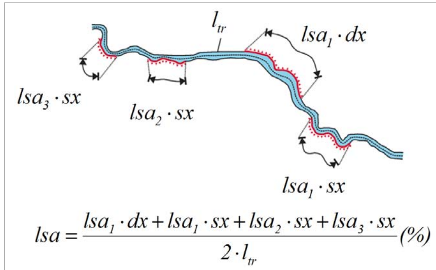
Figura 9.2 – Misura della Lunghezza di sponde in arretramento ( lsa ).
