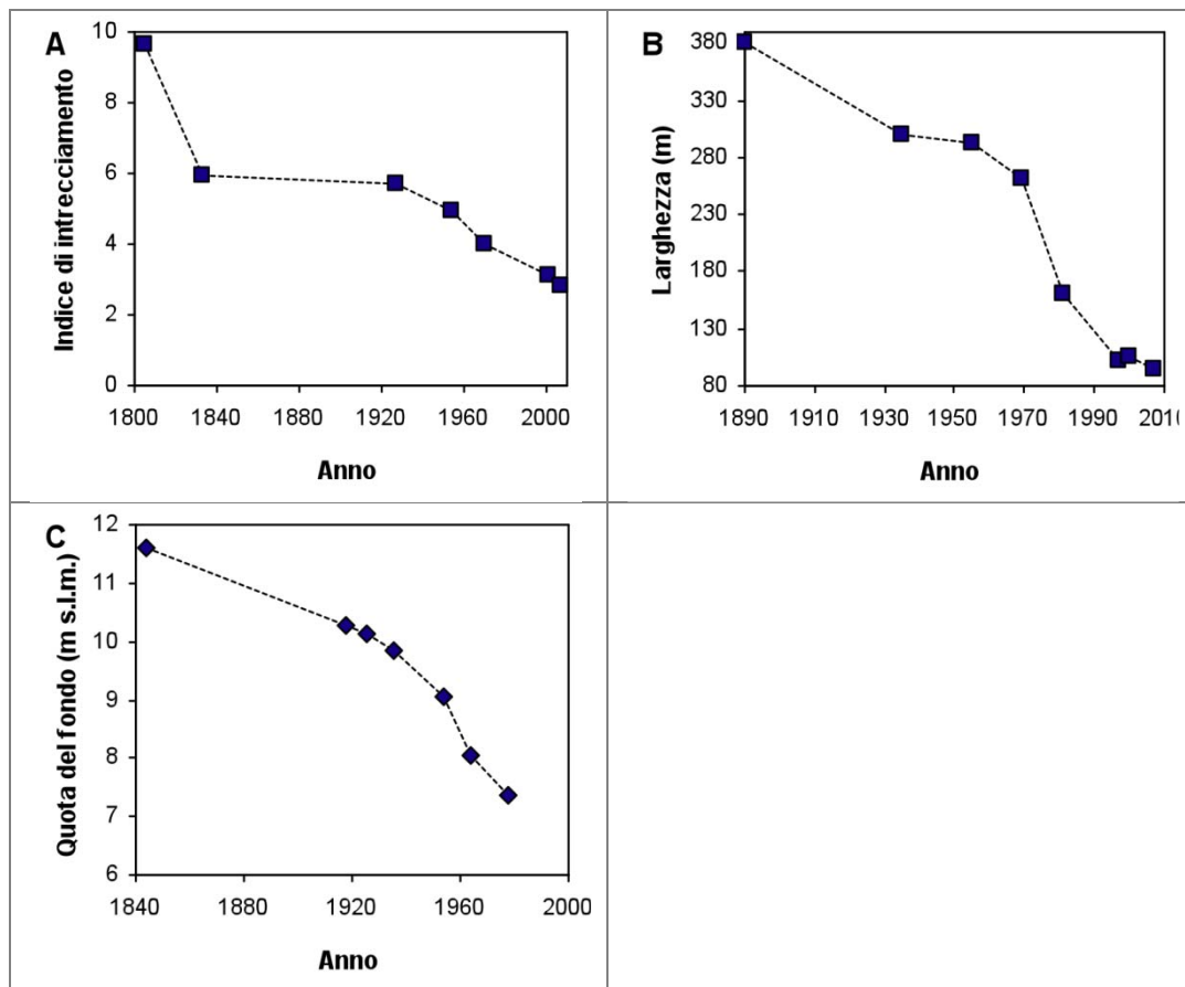
Figura 6.2 – Variazioni in una sezione o tratto. A: Variazioni dell'indice di intrecciamento in un tratto del Fiume Tagliamento nel corso degli ultimi 200 anni; B: Variazioni della larghezza in un tratto del Fiume Panaro (modificato da RINALDI et al., 2008a ). C: Variazioni di quota del fondo in una sezione del Fiume Arno (modificato da RINALDI & SIMON, 1998 ).
