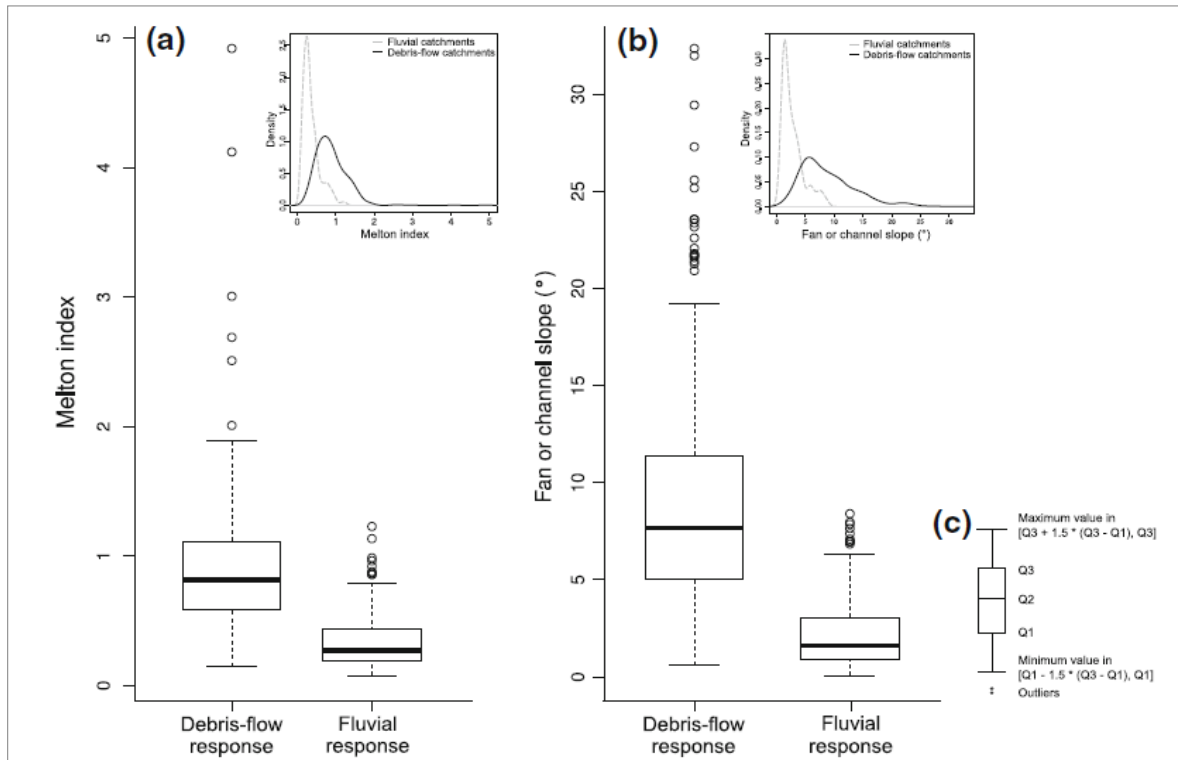
Figura A 7.2 – Distribuzione del numero di Melton (a) e dell’inclinazione del conoide (o del letto lungo il conoide, b) nei bacini da colata ( debris flow ) e da trasporto al fondo ( fluvial ). I bacini da piena di detrito sono stati fatti ricadere in questa analisi nei bacini di tipo “ fluvial ”. Il riquadro (c) spiega il significato dei grafici: Q2 rappresenta la mediana, Q1 e Q3 il 25° e 75° quartile rispettivamente, e gli estremi i valori minimi e massimi escludendo gli outlier. Da BERTRAND et al. (2013) .
