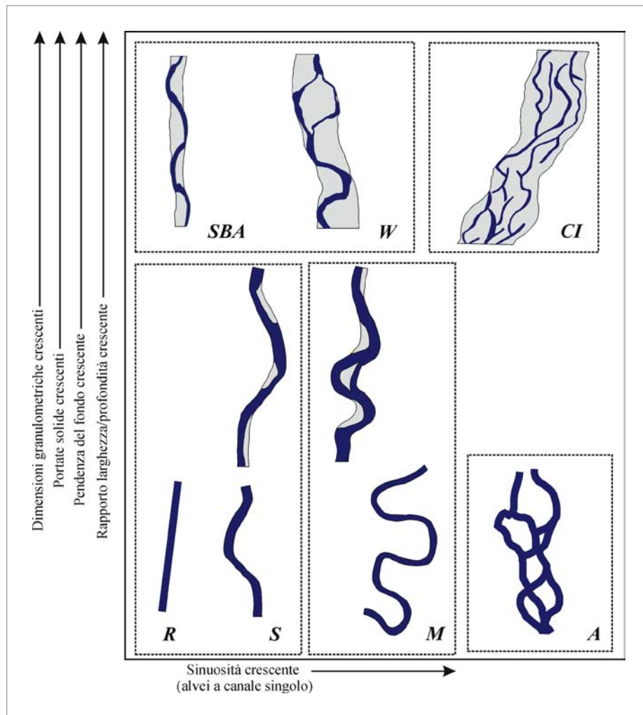
Figura 4.18 – Morfologie fluviali e relazioni con i principali parametri di controllo (modificato da RINALDI, 2003 ). R : Rettilineo; S : Sinuoso; M : Meandri; A : Anabranching; SBA : Sinuoso a barre alternate; W : Wandering; CI : Canali intrecciati.
