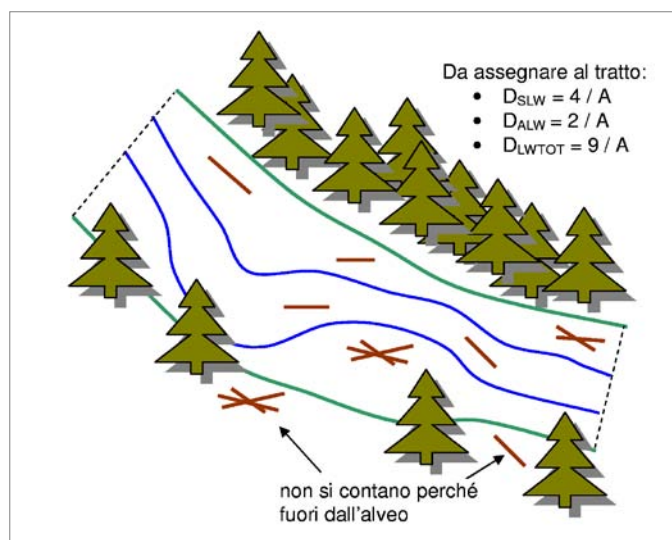
Figura 9.7 – Esempio di conteggio di LW nel sito di monitoraggio, delimitato a monte e a valle dalle linee nere tratteggiate. La linea verde continua simboleggia il limite superiore dell'alveo (sponde), mentre quella blu l'alveo di magra. I segmenti marroni rappresentano tronchi con dimensioni > 1 m in lunghezza e > 0.1 in diametro (LW). Si evidenzia come gli elementi presenti nella piana inondabile non vengano considerati, mentre non si fa differenza tra quelli giacenti su barriere o nel canale di magra. La superficie di alveo ( A ) da misurare ed utilizzare per il calcolo della densità areale di LW è quella compresa tra le linee verdi.
