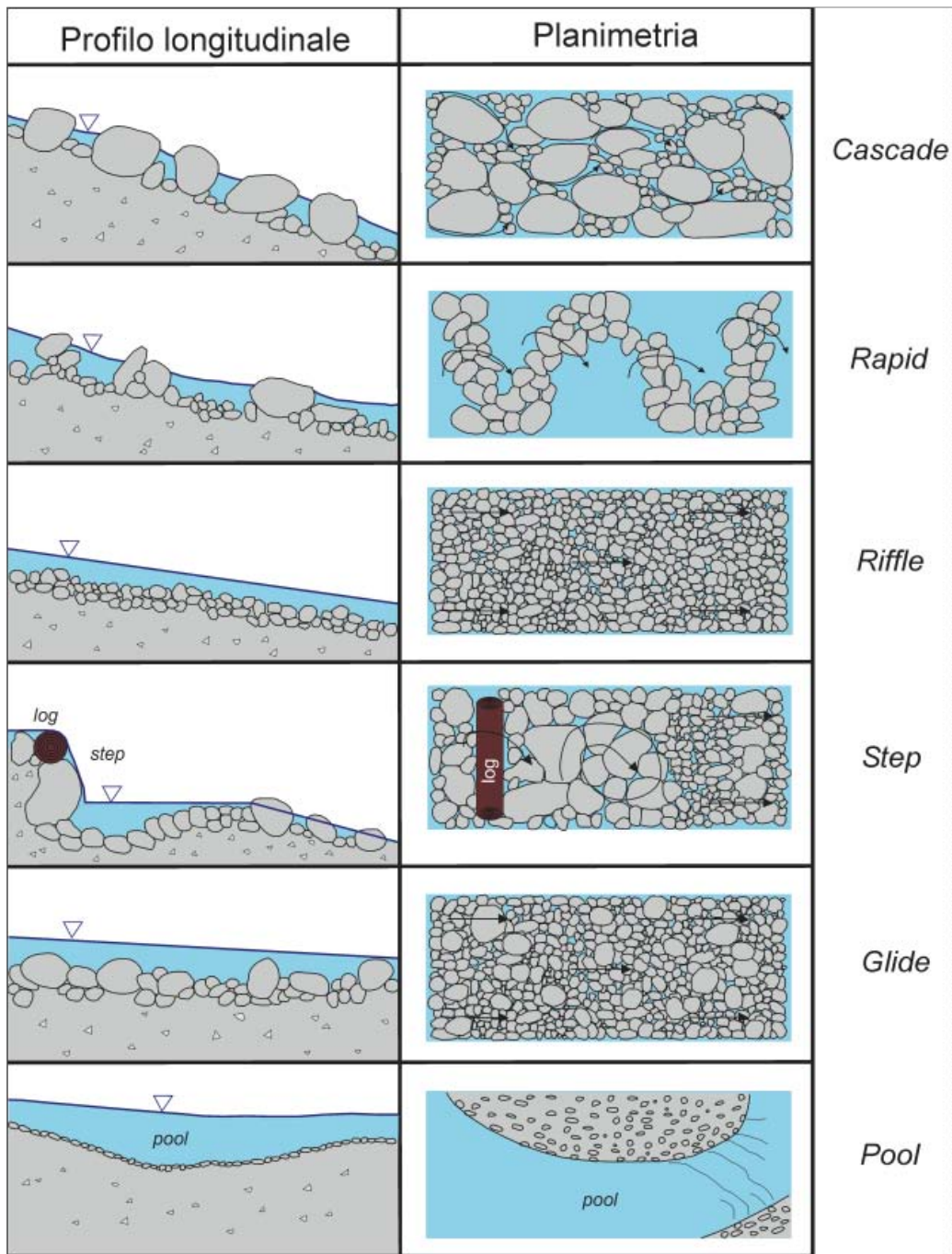
Figura 4.25 – Principali morfologie a scala di unità in alvei alluvionali a pendenza e levata (modificato da HALWAS & CHURCH, 2002 ). Questa classificazione non prevede i “run”, unità di raccordo tra step e pools con caratteristiche idrodinamiche molto simili a quelle delle glide , ma di dimensioni minori.
