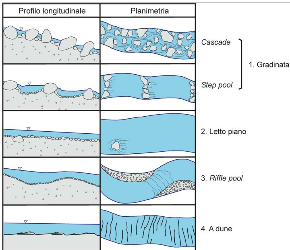
Figura 4.29 – Morfologie di alvei a fluviali a scala di dettaglio ( modificato da MONTGOMERY & BUFFINGTON, 1997 ).
