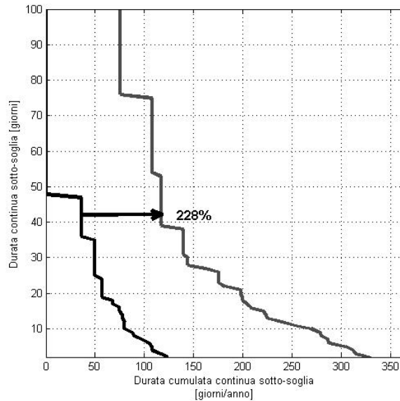
Figura A4.5 - Esempio di calcolo dell'alterazione media della durata degli eventi di stress (eventi di habitat disponibile sotto-soglia) per la specie barbo ( Barbus sp. ) per il F. Taro a Piane di Carniglia (Parma). Le curve di durata dell'habitat disponibile sotto-soglia (CDS) vengono calcolate per le condizioni non alterate (linea di colore nero) e alterate (linea di colore grigio).
