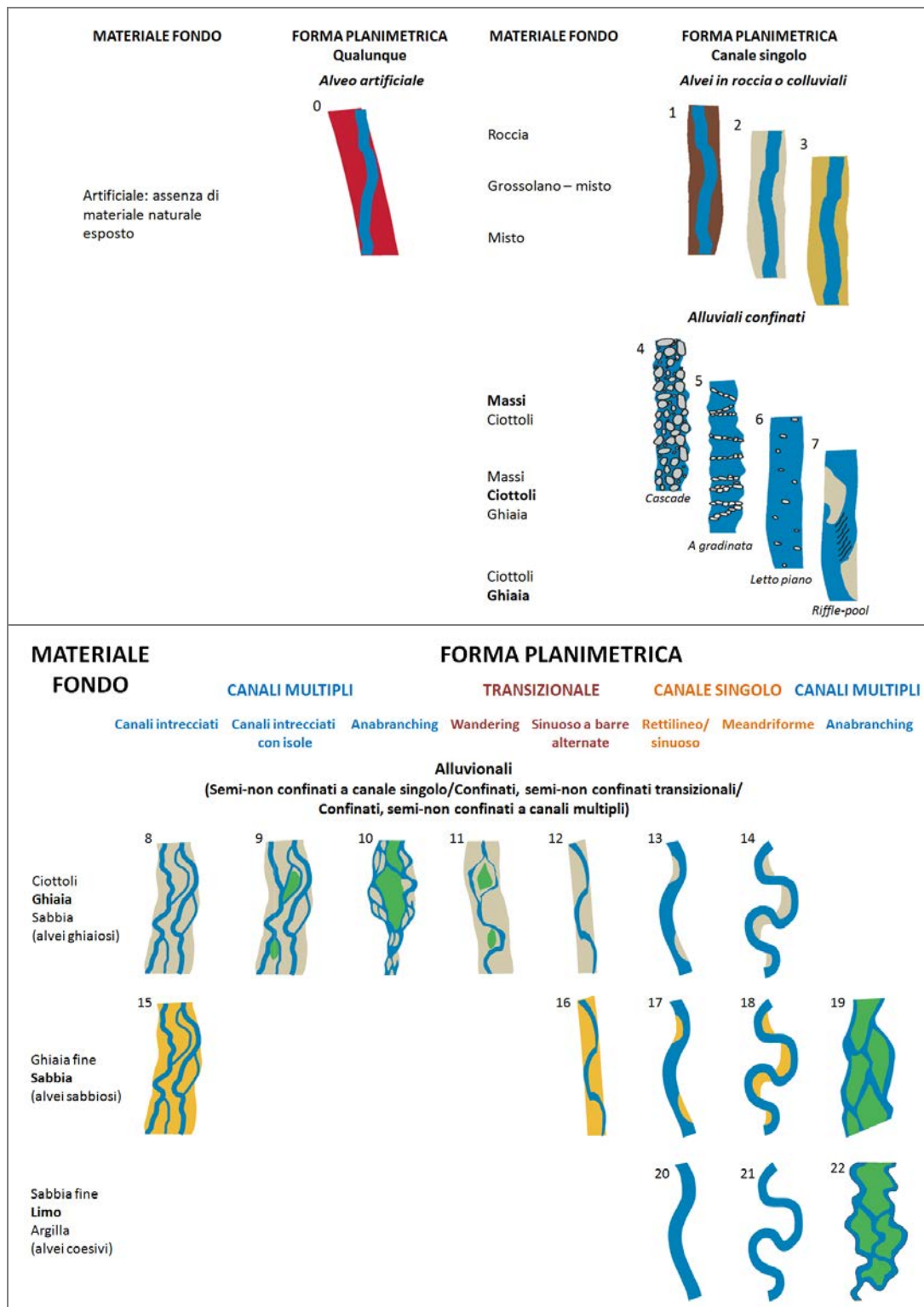
Figura 1.4 - Classificazione estesa delle tipologie morfologiche dei corsi d'acqua ( Extended River Typology ; modificato da Rinaldi et al., 2016 ). Alvei artificiali. (0) A fondo artificiale. Alvei confinati a canale singolo. (1) In roccia; (2) colluviale a sedimenti grossolani - misti; (3) colluviale a sedimenti misti; (4) cascade ; (5) a gradinate; (6) letto piano; (7) riffle-pool . Alvei alluvionali semiconfinati o non confinati a canale singolo, confinati/semi-/non confinati transizionali o a canali multipli. (8) A canali intrecciati ghiaioso; (9) a canali intrecciati con isole; (10) anabranching ghiaioso (equiv. ai tipi 3, 5 o 6 secondo Nanson & Knighton (1996) ); (11) wandering ; (12) sinuoso a barre alternate ghiaioso; (13) rettilineo-sinuoso ghiaioso; (14) meandriforme ghiaioso; (15) a canali intrecciati sabbioso; (16) sinuoso a barre alternate sabbioso; (17) rettilineo-sinuoso sabbioso; (18) meandriforme sabbioso; (19) anabranching sabbioso (equiv. ai tipi 2 o 4 secondo Nanson & Knighton (1996) ); (20) rettilineo-sinuoso limoso; (21) meandriforme limoso; (22) anastomizzato (equiv. al tipo 1 secondo Nanson & Knighton (1996) ).
