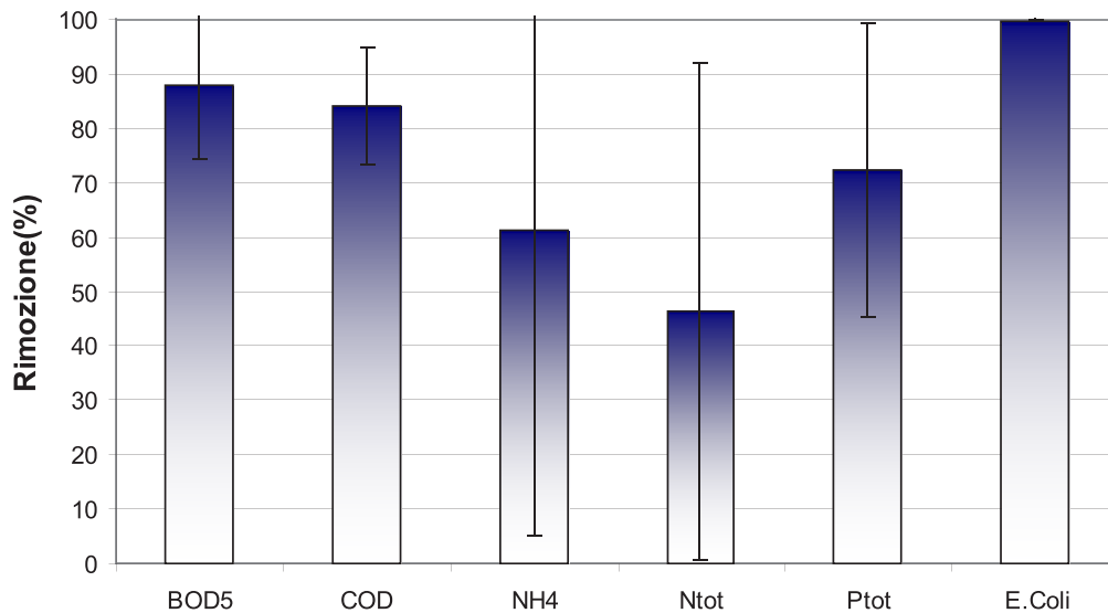
Impianto Azienda agrituristica "Baggiolino"-Comune di Scandicci (FI) Rese depurative - (dati: 2002-2003)
