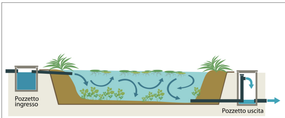
Figura 3 – Rappresentazione schematica di un sistema a flusso libero
