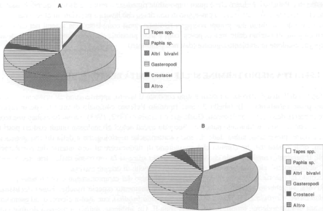
Fig. 25: Composizione, in numero (A) e in peso (B), della cattura con turbosoffiante in Rivola C.
