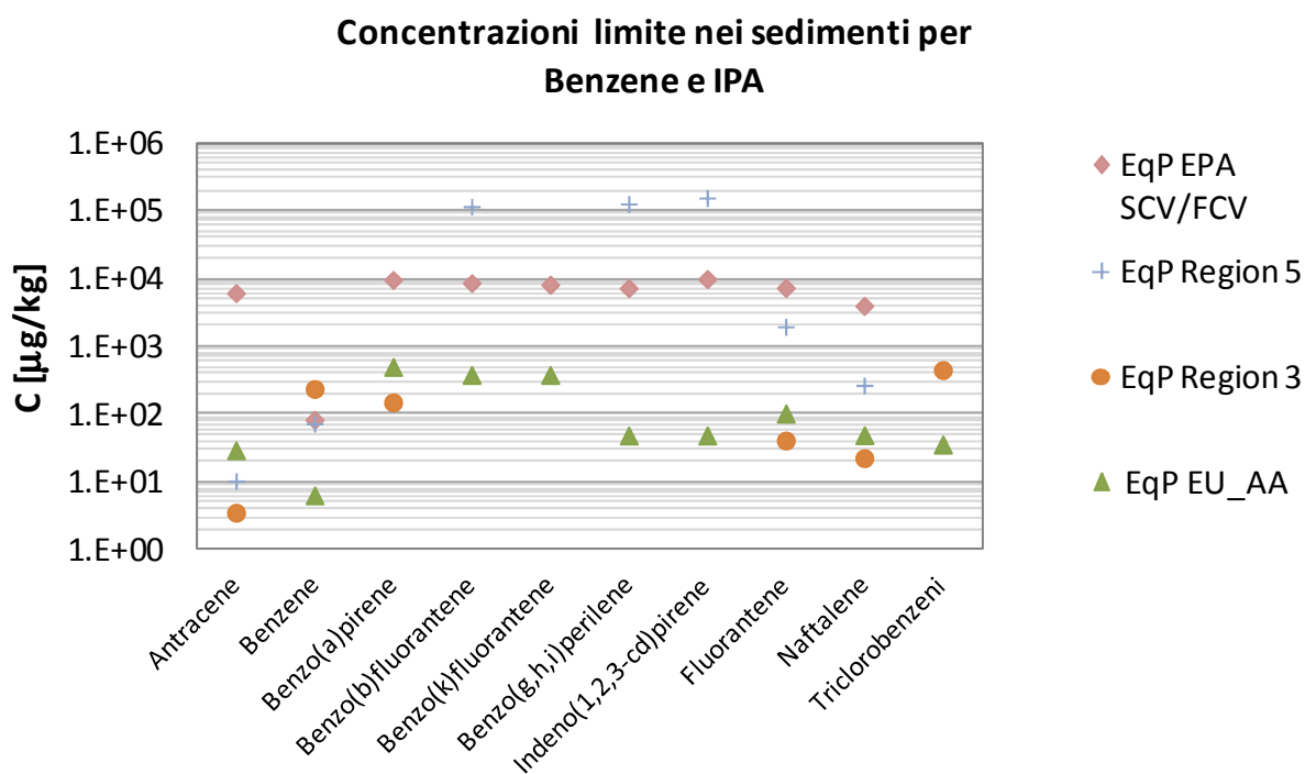
Figura 3.26: Confronto tra i valori di SQG calcolati a partire dagli standard di qualità fissati dalla direttiva 105/2008 (EU_AA), quelli calcolati dagli standard di qualità delle acque statunitensi (EPA SCV/FCV, EPA Region 3/5)
