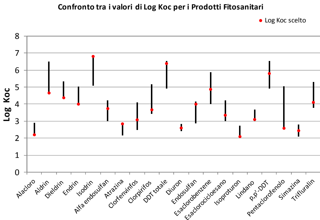
Figura 3.17: Valore di Koc scelto e range di variabilità del Koc tra tutti i riferimenti ed equazioni considerati per i fitosanitari
