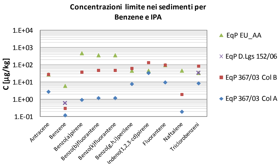
Figura 3.23: Confronto tra i valori di SQG calcolati a partire da diversi standard di qualità delle acque superficiali italiani e dagli standard di qualità fissati dalla direttiva 105/2008 (EU_AA) per benzene ed IPA
