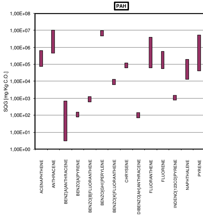
Figura 3.47: Variazione dei valori degli SQG per gli IPA per le diverse specie
