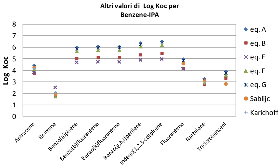
Figura 3.13: confronto tra i valori di Koc proposti da Sabljic et al.(1995), Karichoff (1981) e Karichoff e Long (1995) e quelli calcolati con le equazioni riportate in Tabella 3.1 per benzene ed IPA
