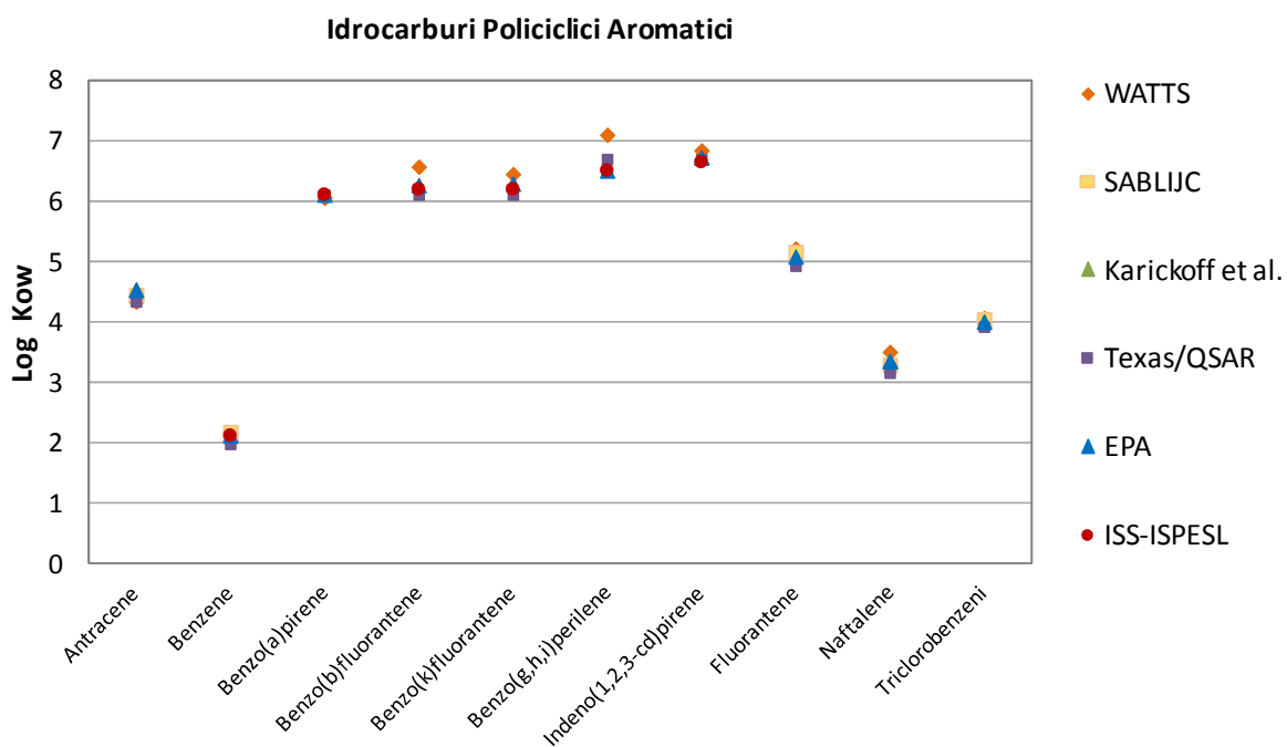
Figura 3.1: Kow per la classe dei composti policiclici aromatici
