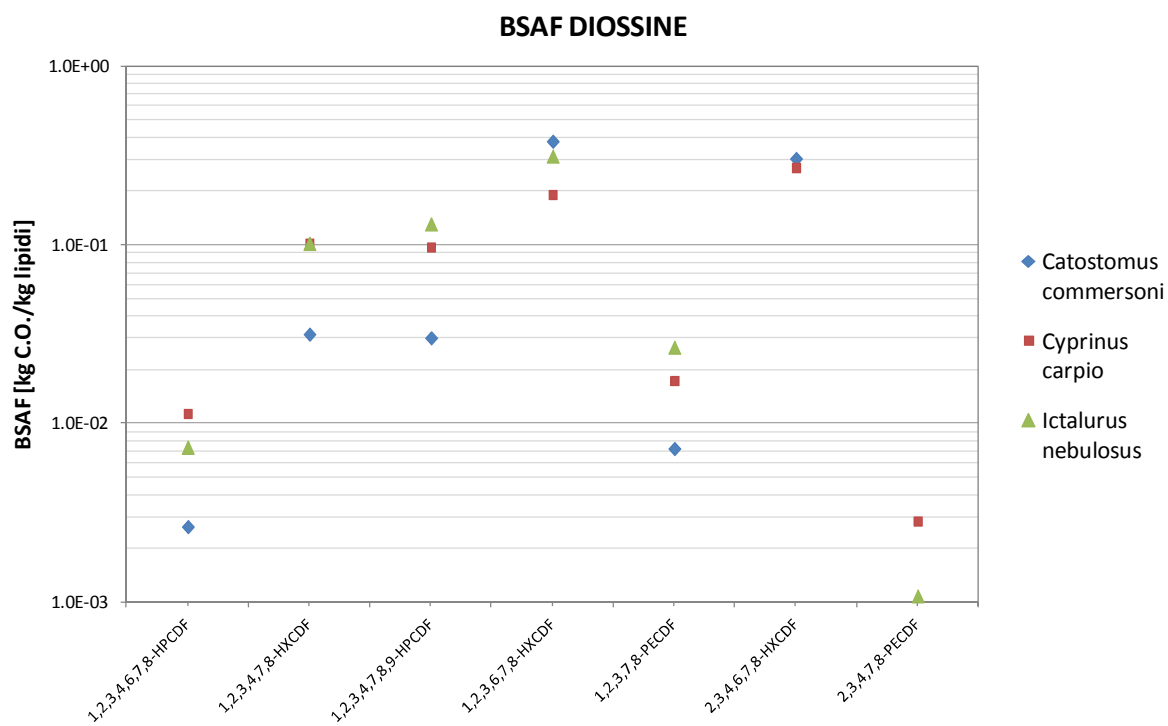
Figura 3.34: Valori di BSAF per i furani relativi a 3 specie di pesci
