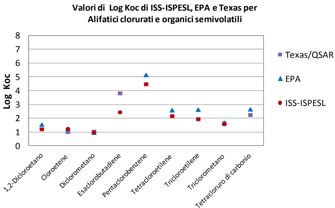
Figura 3.9: Confronto tra i valori di Koc proposti da ISS-ISPEL, EPA e Texas per i alifatici clorurati e organici semivolatili
