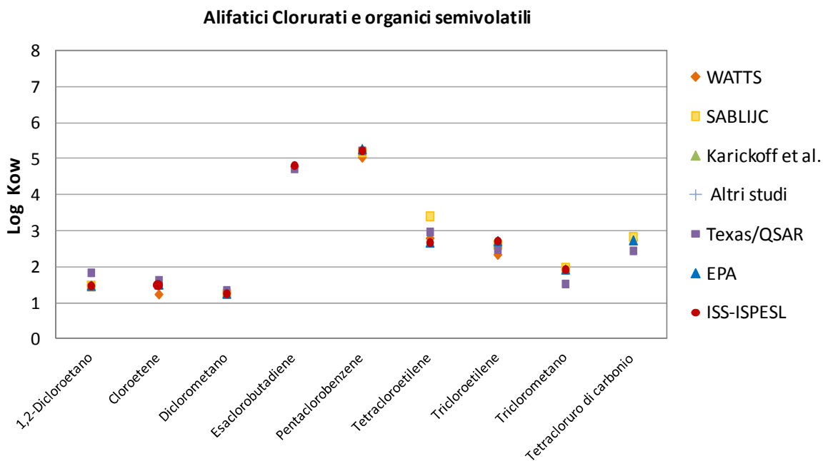
Figura 3.3: Valori di Kow per la classe dei composti clorurati
