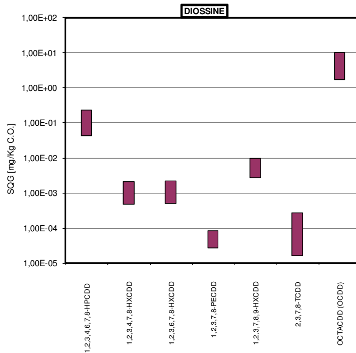
Figura 3.45: Variazione dei valori degli SQG per le diossine per le diverse specie
