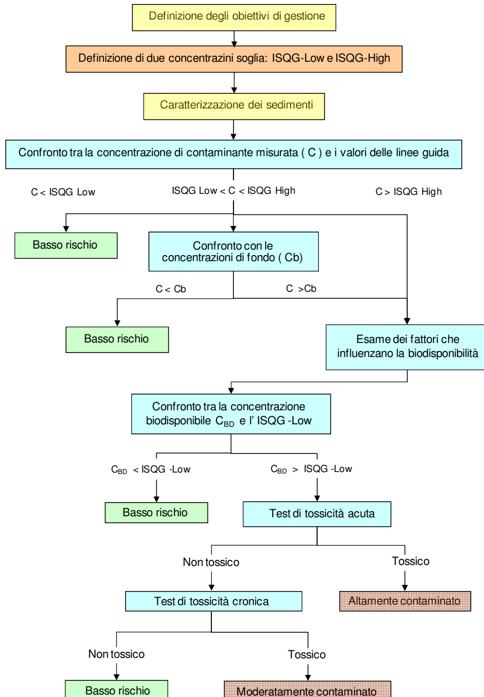
Figura 1.4: Albero decisionale utilizzato nella definizione degli SQG in Australia e Nuova Zelanda
