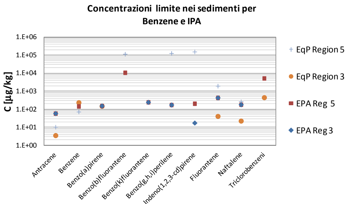
Figura 3.29: Confronto tra i valori di SQG calcolati a partire dagli standard di qualità delle acque statunitensi (EqP Region 3/5) e valori standard sui sedimenti statunitensi (EPA Region 3/5) per benzene ed IPA
