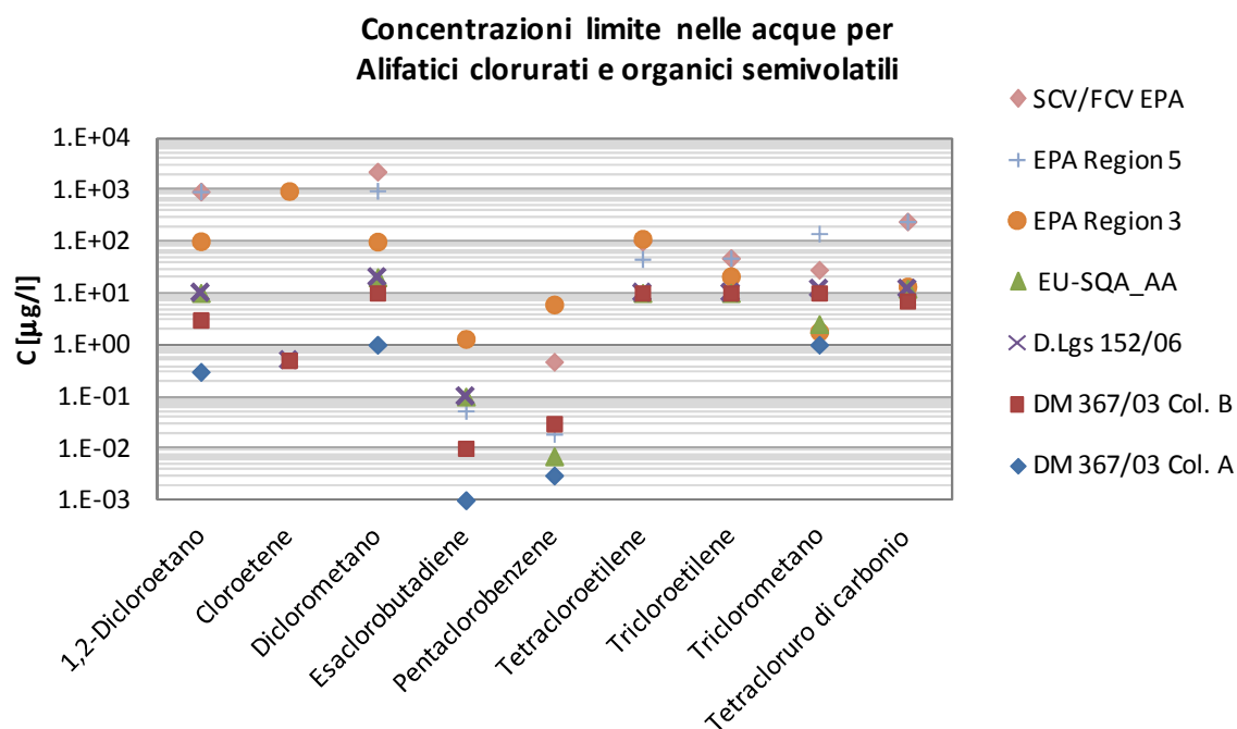
Figura 3.22: Standard di qualità delle acque nazionali ed internazionali per alifatici clorurati e organici semivolatili
