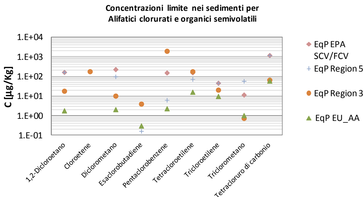
Figura 3.28: Confronto tra i valori di SQG calcolati a partire dagli standard di qualità fissati dalla direttiva 105/2008 (EU_AA), quelli calcolati dagli standard di qualità delle acque statunitensi (EPA SCV/FCV), e valori standard sui sedimenti statunitensi (EPA Region 3/5) per alifatici clorurati e organici semivolatili
