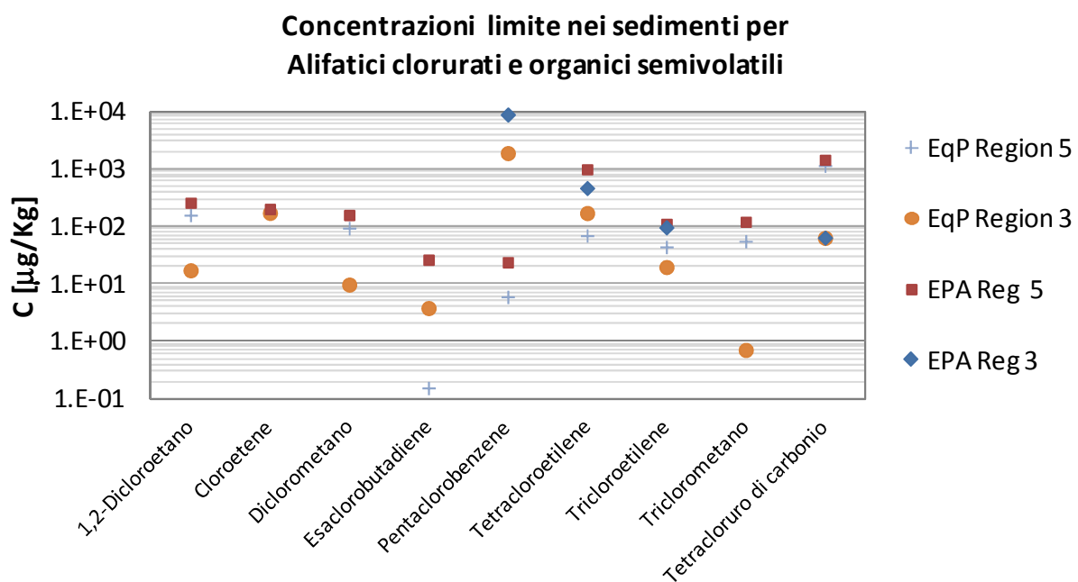
Figura 3.31: Confronto tra i valori di SQG calcolati a partire dagli standard di qualità delle acque statunitensi (EqP Region 3/5) e valori standard sui sedimenti statunitensi (EPA Region 3/5) per alifatici clorurati e organici semivolatili
