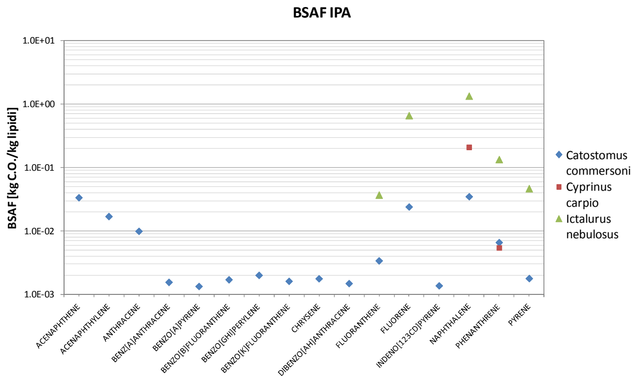
Figura 3.36: Valori di BSAF per gli IPA relativi a 3 specie di pesci
