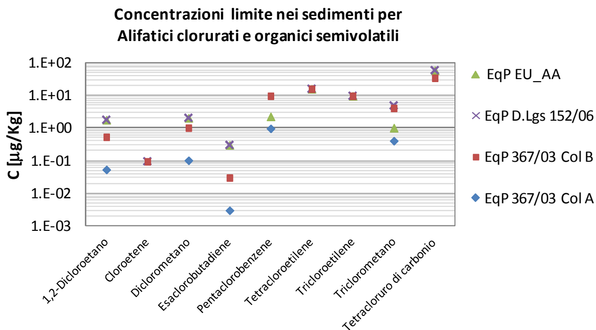
Figura 3.25: Confronto tra i valori di SQG calcolati a partire da diversi standard di qualità delle acque superficiali italiani e dagli standard di qualità fissati dalla direttiva 105/2008 (EU_AA) per alifatici clorurati e organici semivolatili
