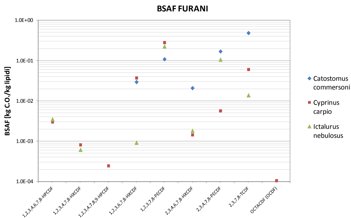
Figura 3.33: Valori di BSAF per i furani relativi a 3 specie di pesci
