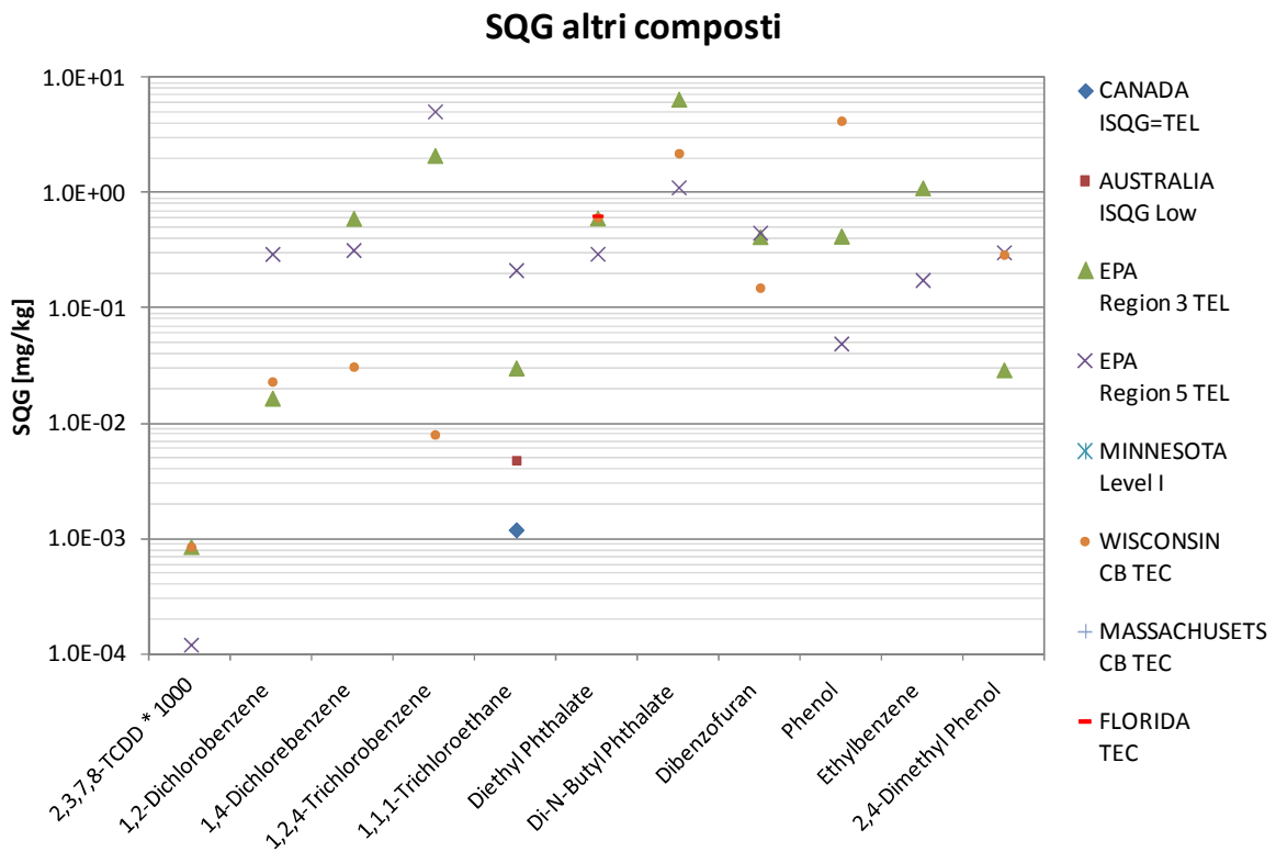
Figura 1.8: Confronto tra i valori inferiori degli SQG relativi ad alcuni contaminanti definiti nelle diverse giurisdizioni
