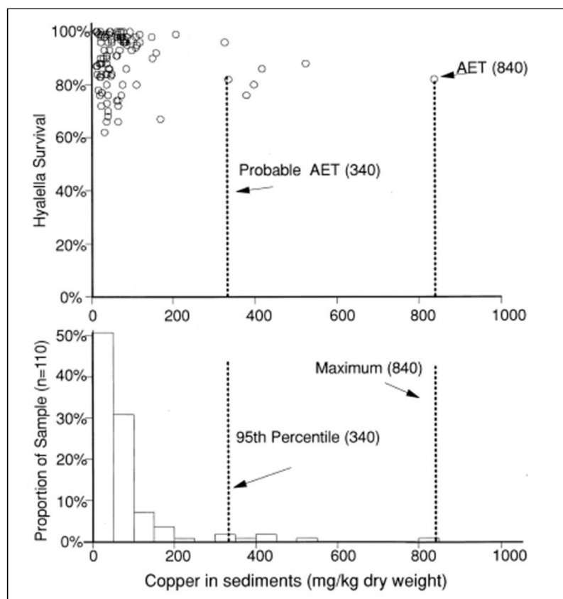
Figura 2.2: Esempio di derivazione grafica del valore di PAET per le concentrazioni di rame nei sedimenti da dati relativi alla sopravvivenza dell'anfipode Hyalella Azteca .
