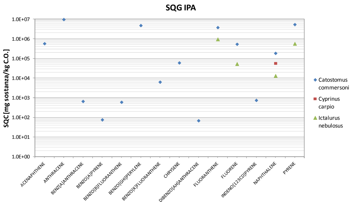
Figura 3.42: Valori di SQG per gli IPA relativi a 3 specie di pesci
