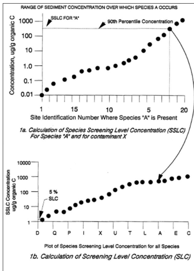
Figura 2.1: Esempio di calcolo delle concentrazioni del livello di screening per una sostanza generica (A)
