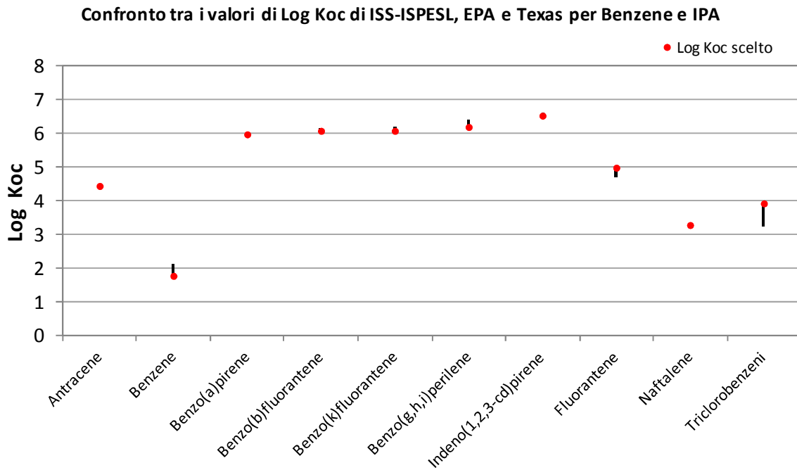
Figura 3.10: Valore di Koc scelto e range di variabilità del Koc tra database ISS-ISPEL, EPA e Texas per benzene ed IPA
