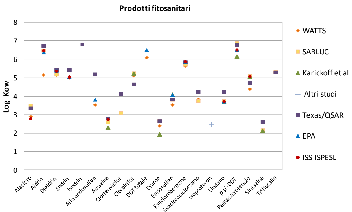
Figura 3.2: Valori di Kow per la classe dei prodotti fitosanitari
