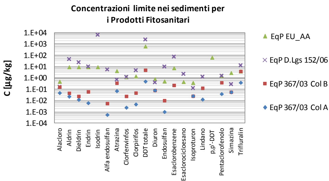
Figura 3.24: Confronto tra i valori di SQG calcolati a partire da diversi standard di qualità delle acque superficiali italiani e dagli standard di qualità fissati dalla direttiva 105/2008 (EU_AA) per i fitosanitari
