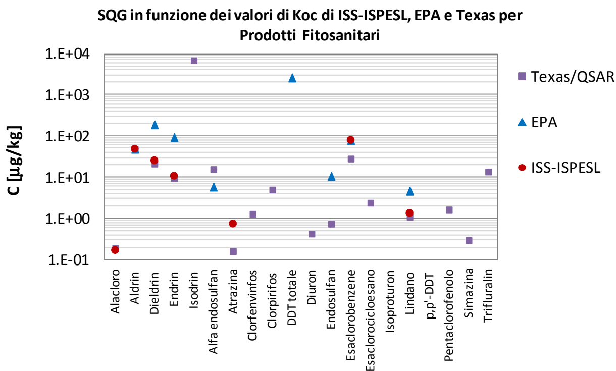
Figura 3.19: Confronto tra i valori di SQG calcolati utilizzando i valori di Koc proposti da ISS-ISPEL, EPA e Texas per i fitosanitari. Standard di qualità delle acque utilizzato: D. Lgs. 152/06
