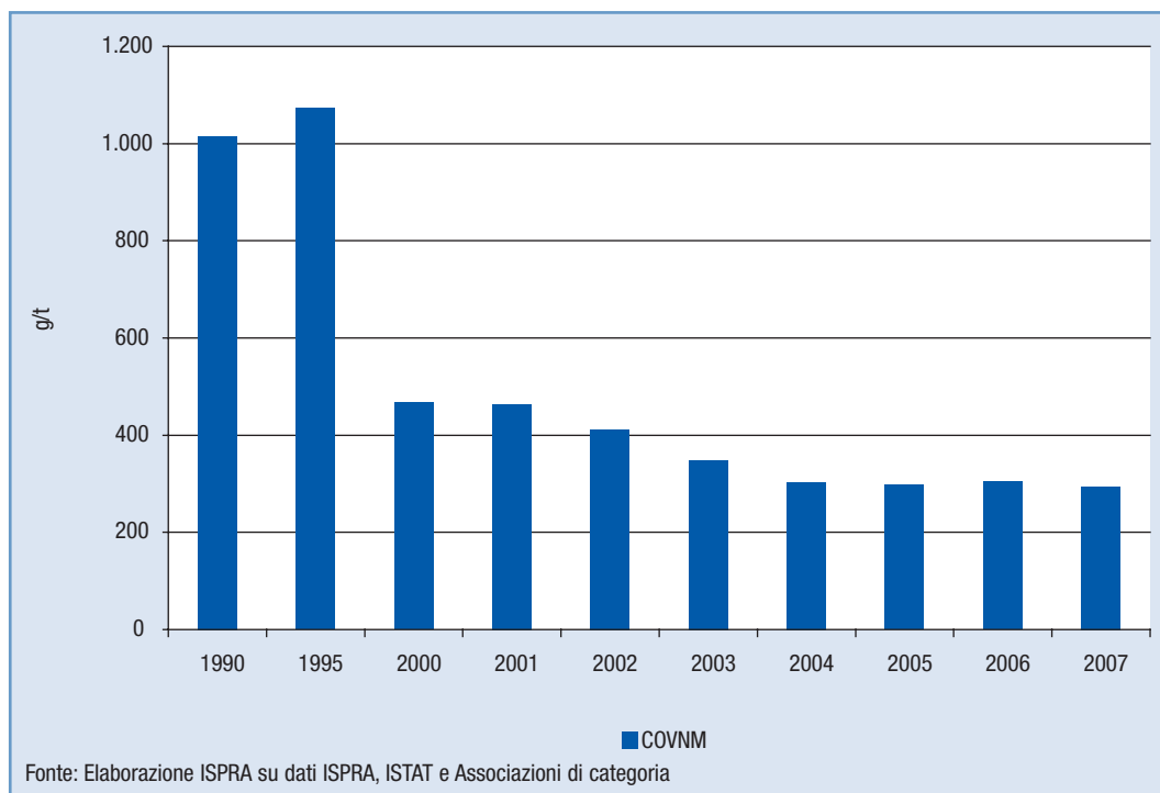
Figura 5.3: Emissioni specifiche di COVNM nell'industria chimica
