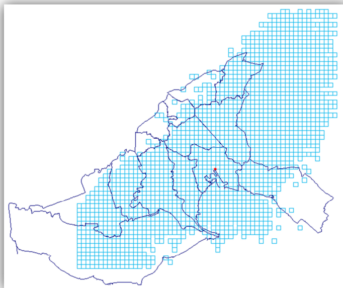
Figura 12: Modello di dispersione l'area di dispersione dell'NO 2 prodotto esclusivamente dalla centrale termoelettrica A2A di Monfalcone con concentrazioni > 0,5 µg/m 3
