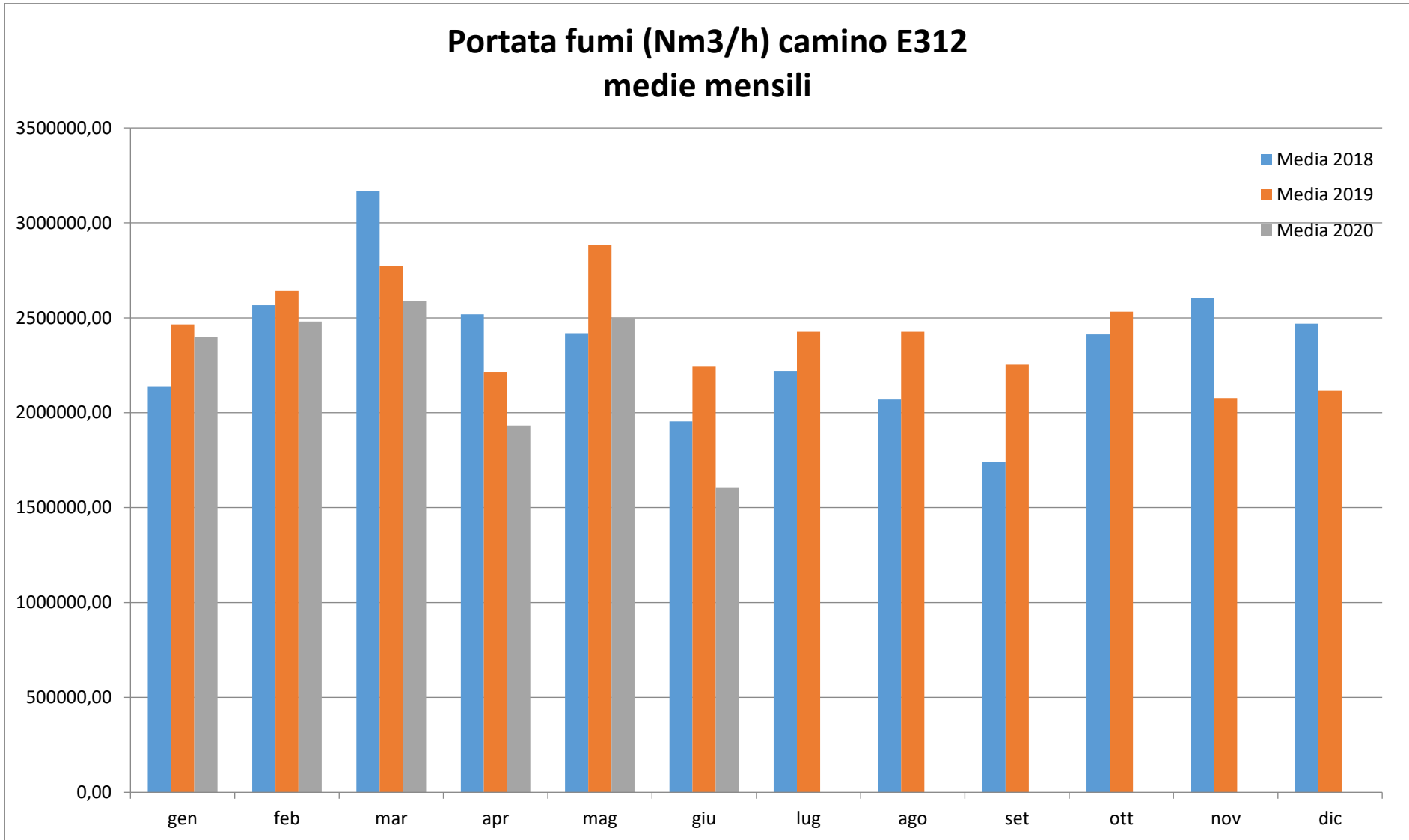
Figura 8. Esercizio Camino E312 Area Agglomerato, periodo gennaio 2018 – giugno 2020
