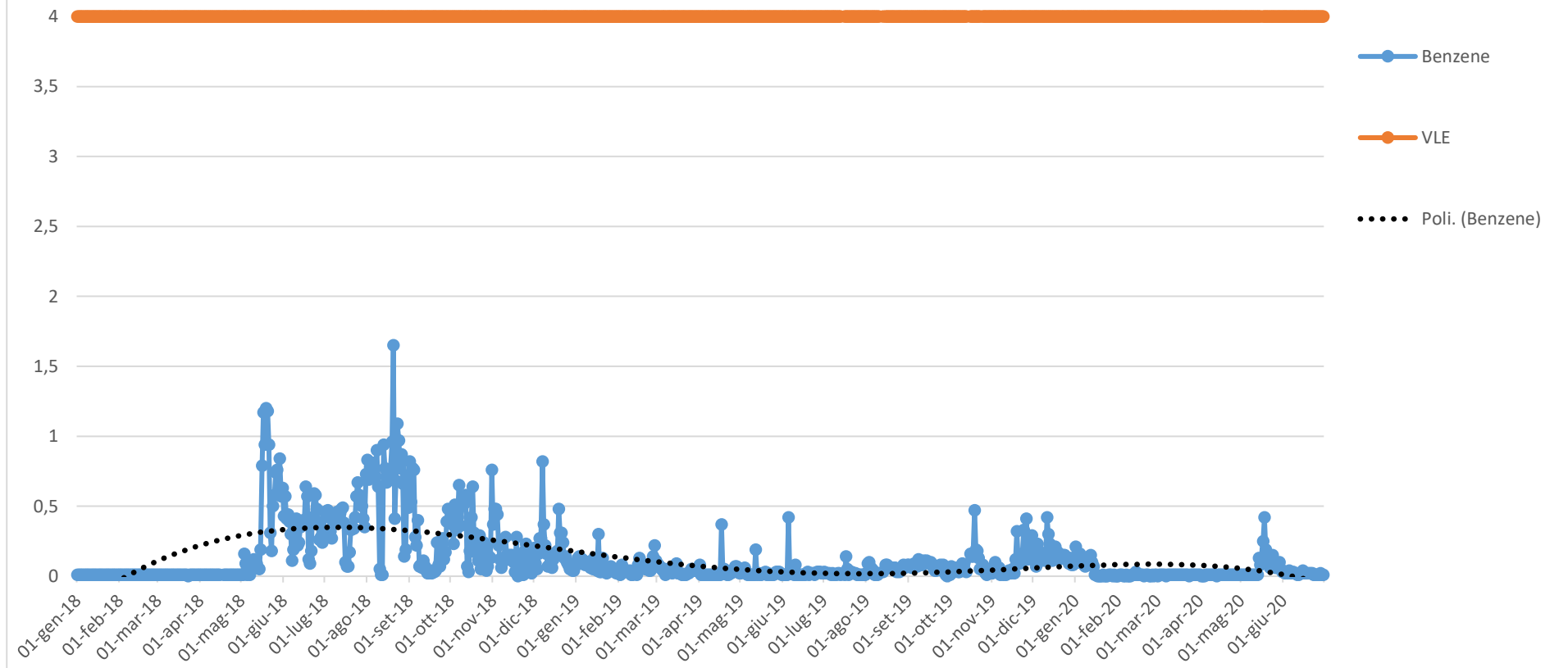
FIG. 7 – Trend Benzene camini cokefazione
