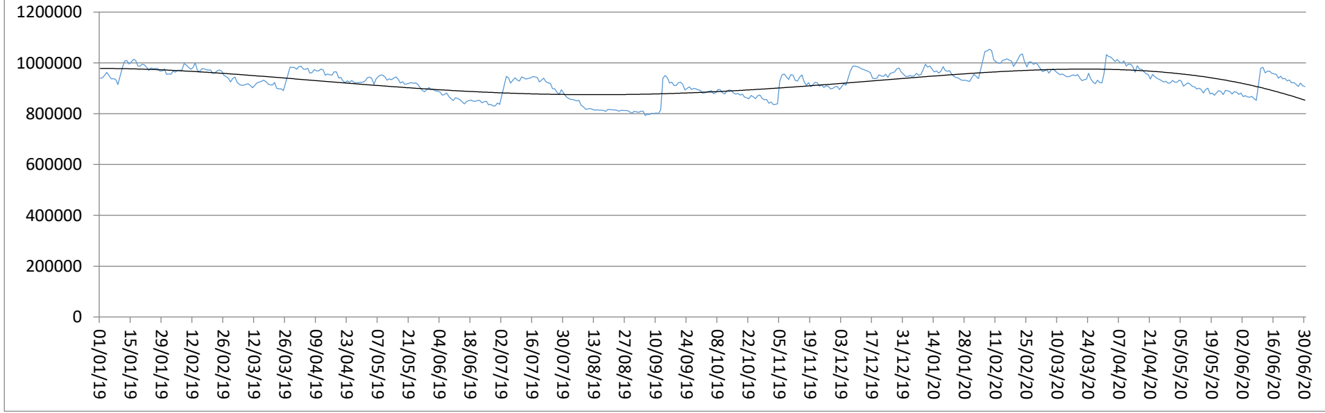
Portata Fumi (Nm3/h) camino E102B - Anni 2019-2020
