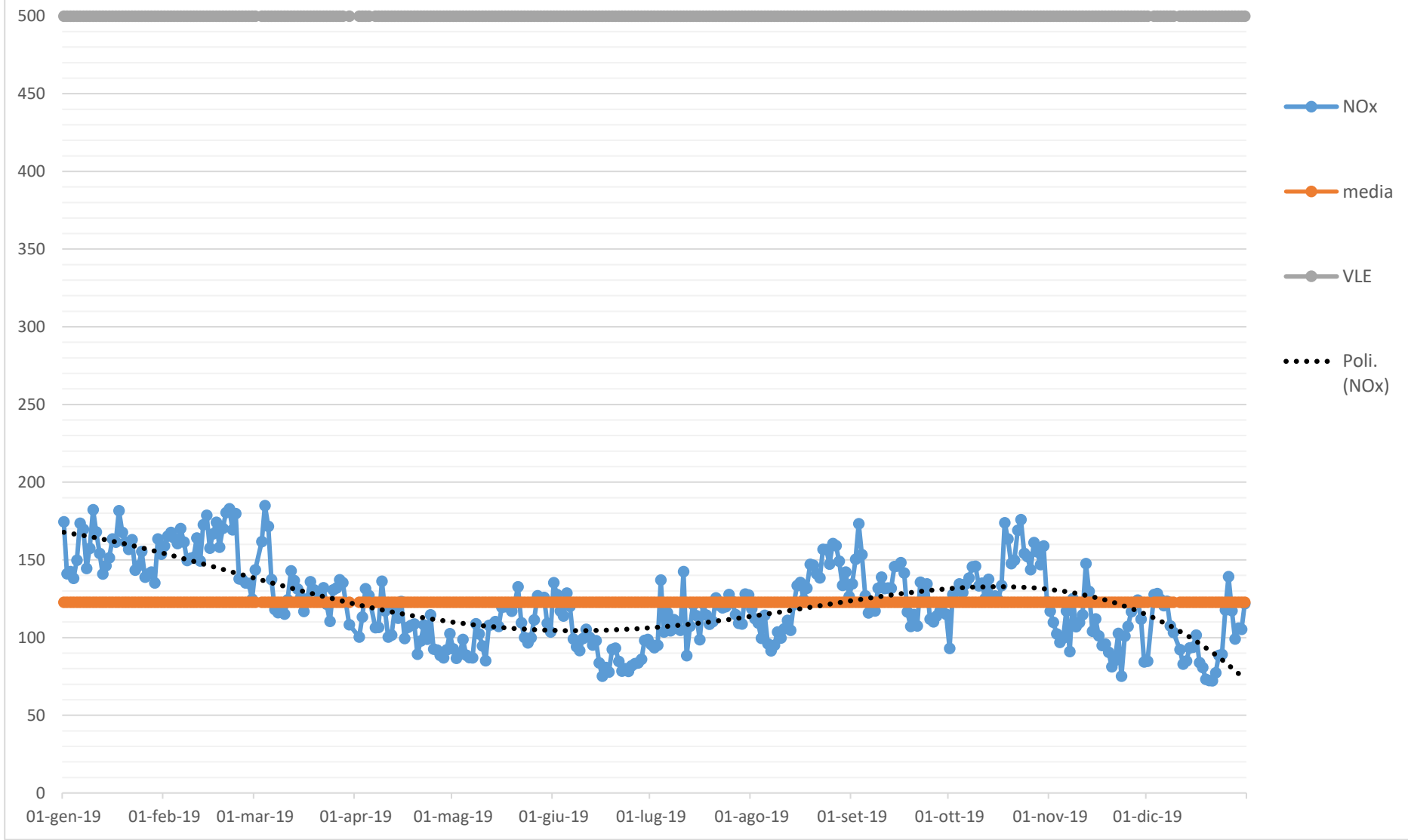
Concentrazione di NOx (mg/Nm3, media giornaliera) camino E426 cokeria - ANNO 2019
