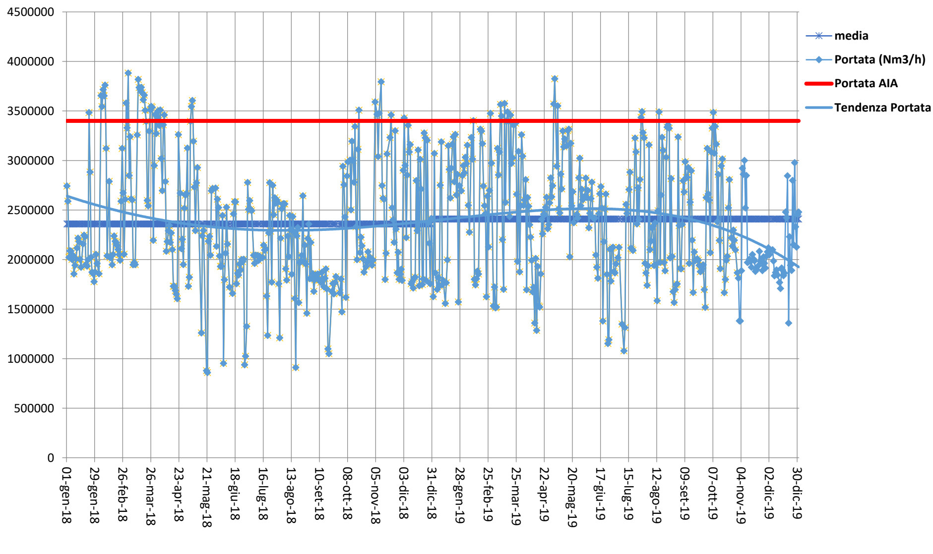
Portata fumi (Nm3/h) - Camino E312 - Anni 2018 - 2019
