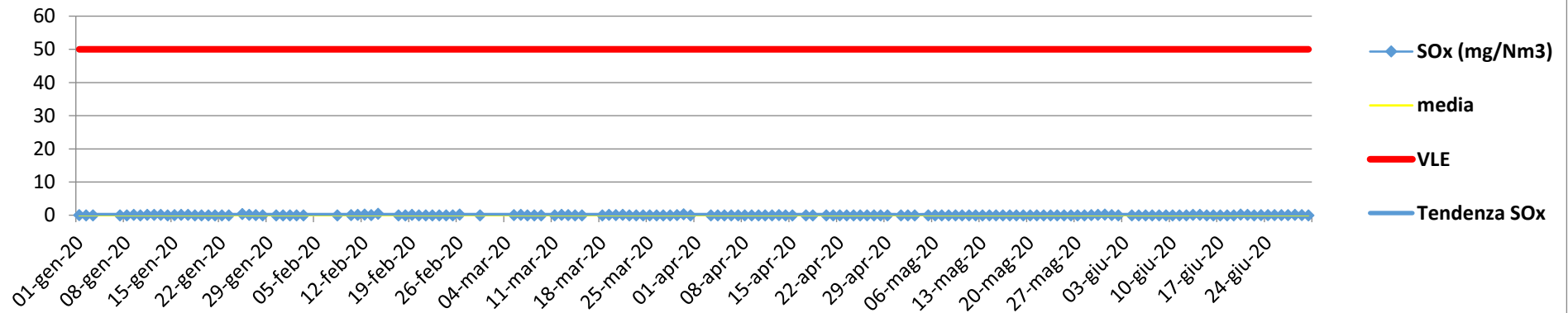
Concentrazione SOx (mg/Nm3) camino E325 - Anno 2020
