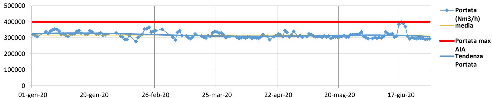
Portata fumi (Nm3/h) camino E325 - Anno 2020
