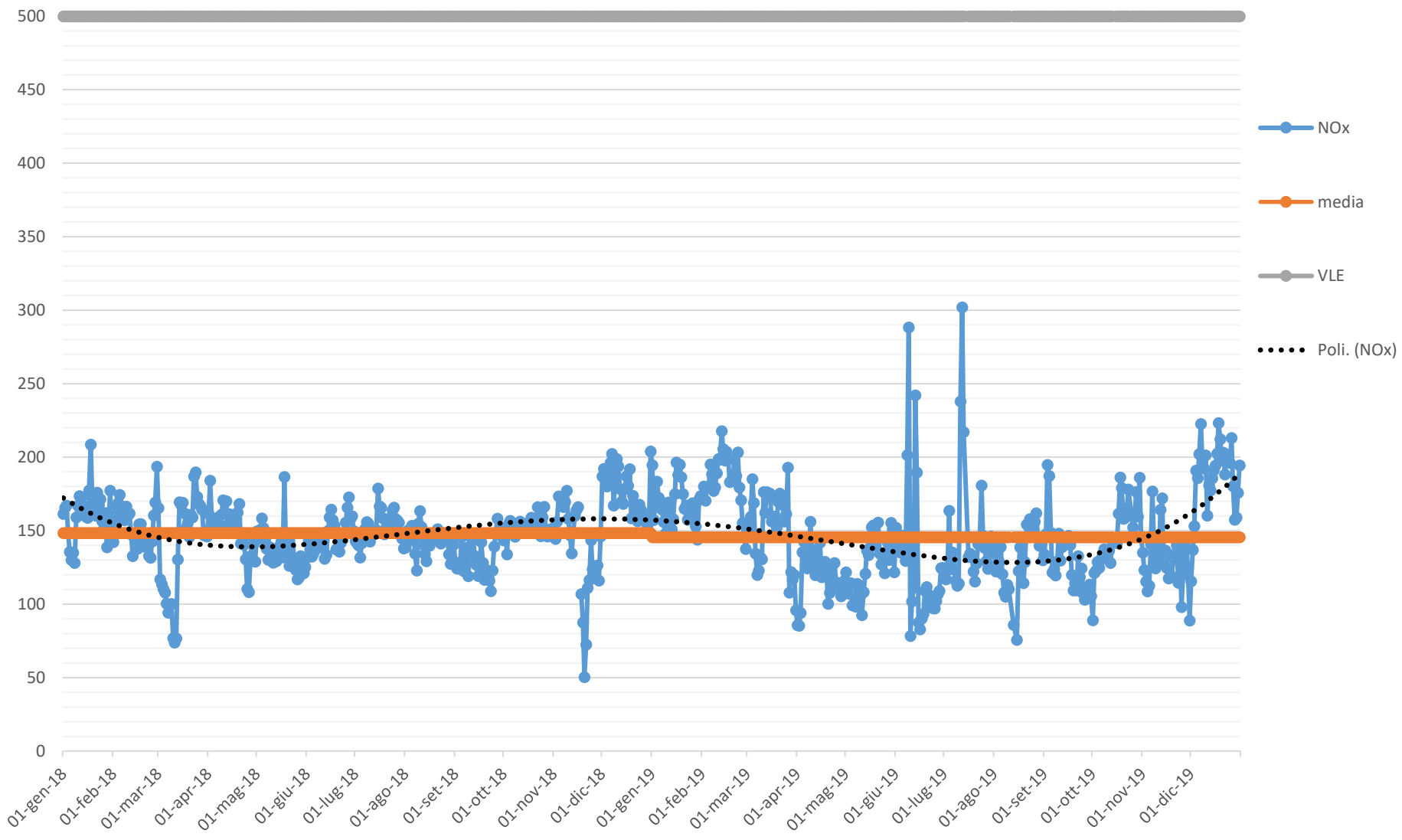
Concentrazione NOx (mg/Nm3, media giornaliera) camino E428 cokeria - ANNI 2018-2019
