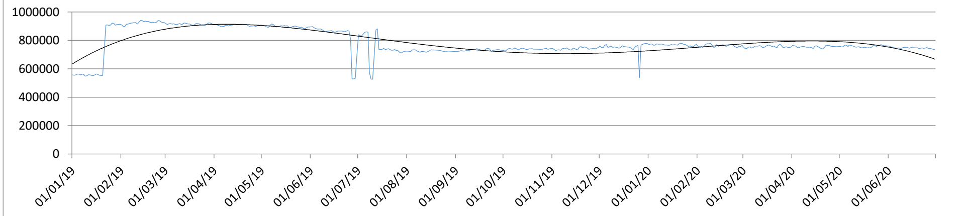
Portata Fumi (Nm3/h) camino E109 - Anni 2019-2020
