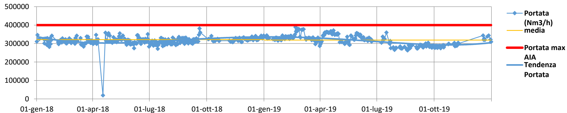
Portata fumi (Nm3/h) camino E325 - Anni 2018-2019
