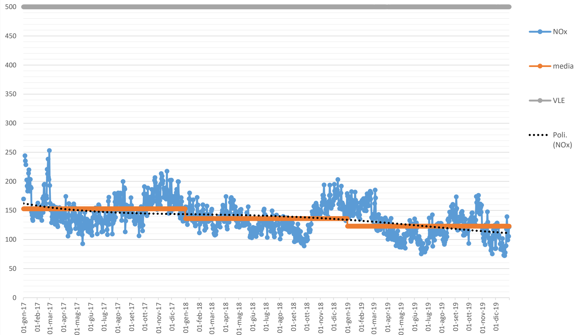
Concentrazione di NOx (mg/Nm3, media giornaliera) camino E426 cokeria-ANNI 2017-2018- 2019
