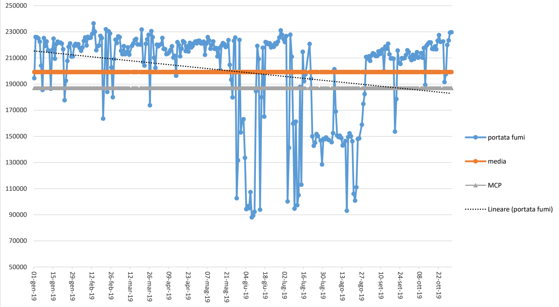
Portata fumi (Nm3/h) camino 4 (E424) cokeria - anno 2019
