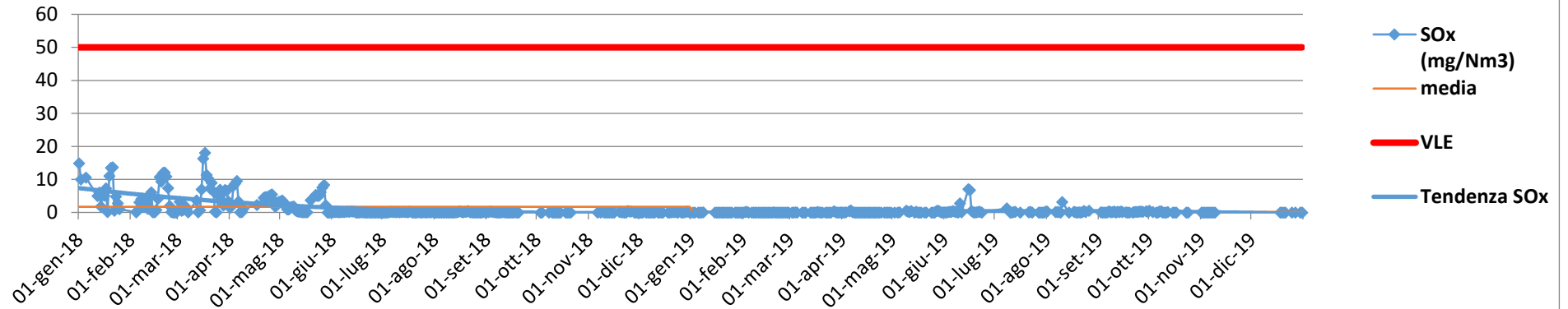
Concentrazione SOx (mg/Nm3) camino E325 - Anni 2018-2019
