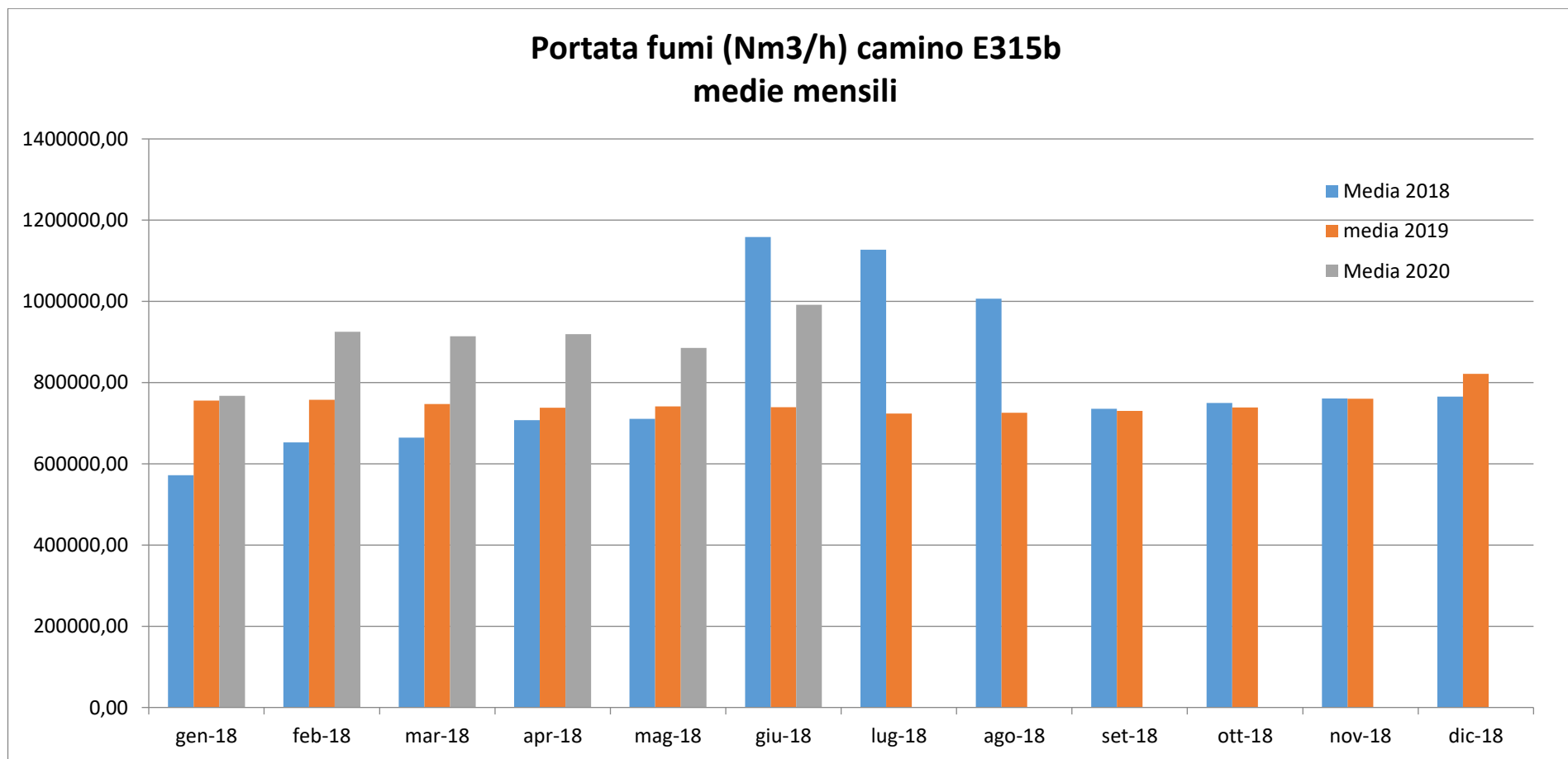
Figura 10. Esercizio Camino E315b Area Agglomerato, periodo gennaio 2018 – giugno 2020
