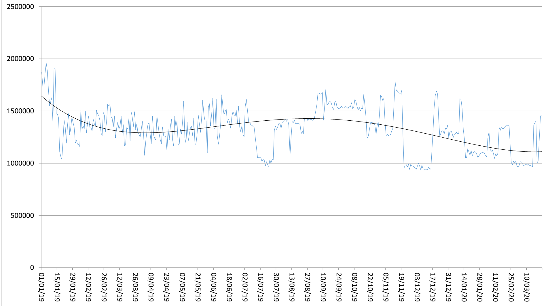
Portata Fumi (Nm 3 /h) camino E525B - Anni 2019-2020
