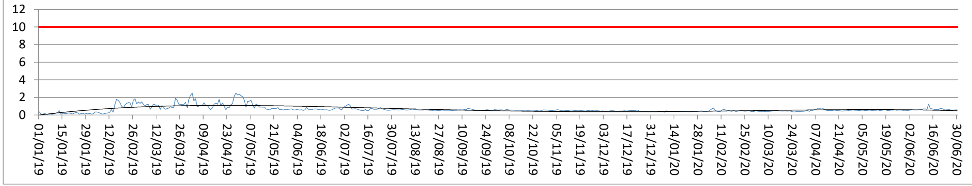
Polveri (mg/Nm3) camino E102B - Anni 2019-2020
