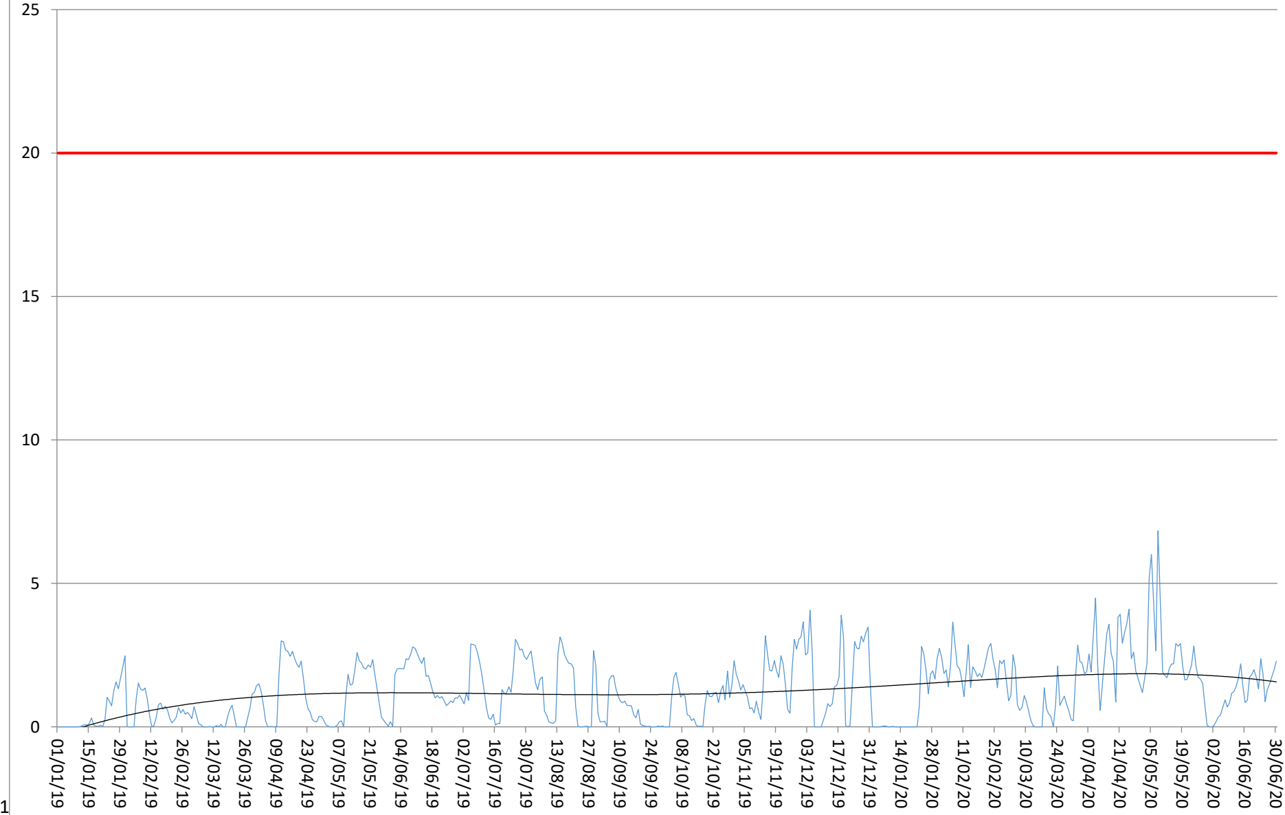
NOx (mg/Nm3) camino E551B - Anni 2019-2020
