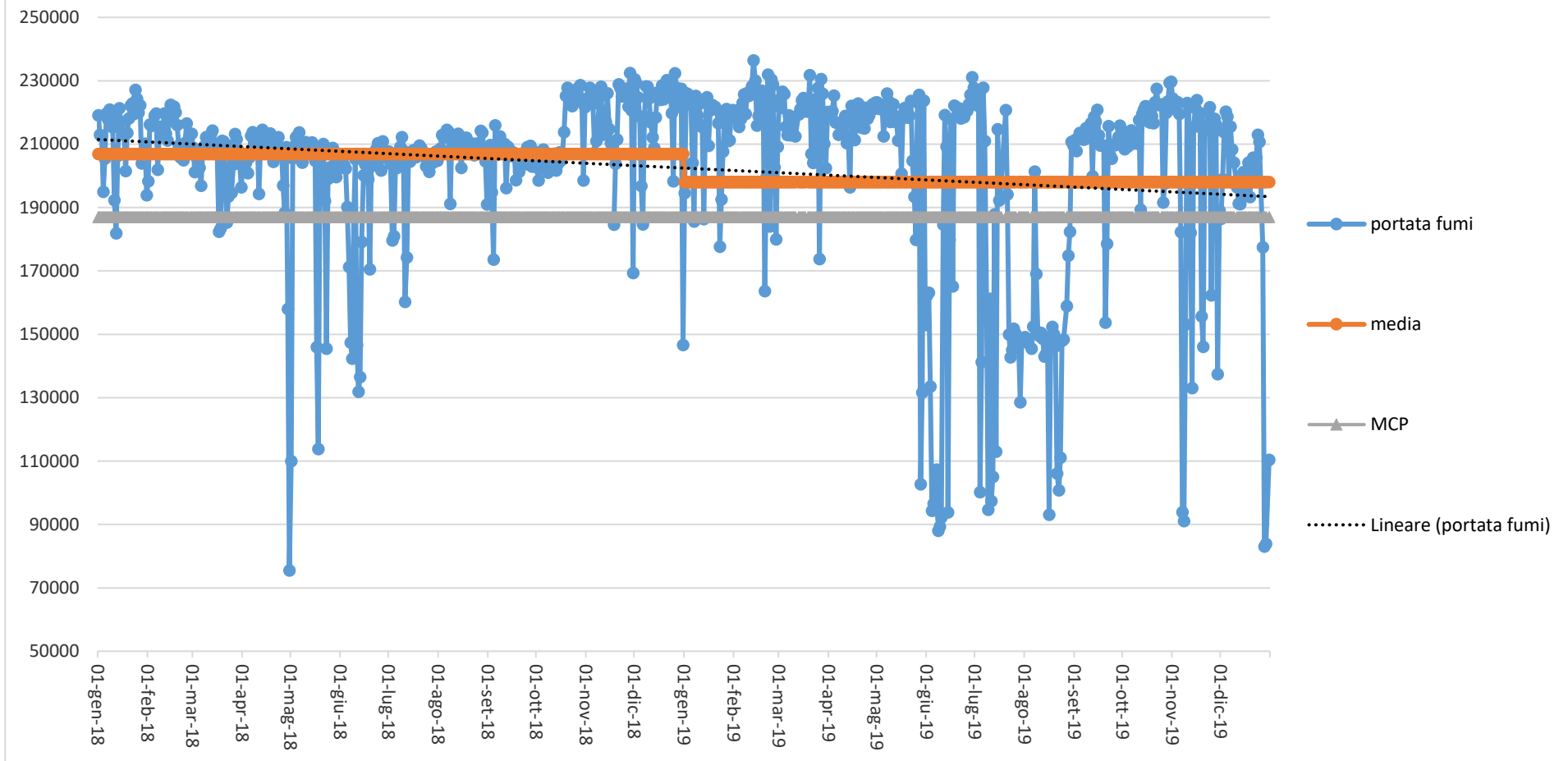
Portata fumi (Nm 3 /h) camino 4 (E424) cokeria - anni 2018-2019
