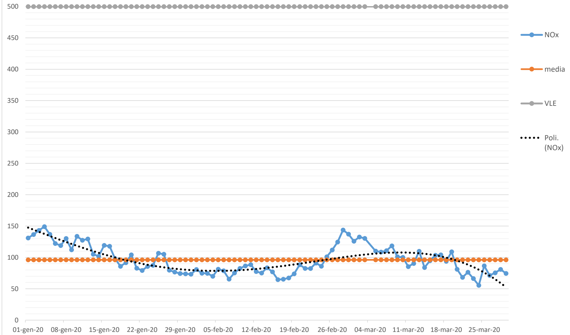
Concentrazione di NOx (mg/Nm3, media giornaliera) camino E426 cokeria - ANNO 2020
