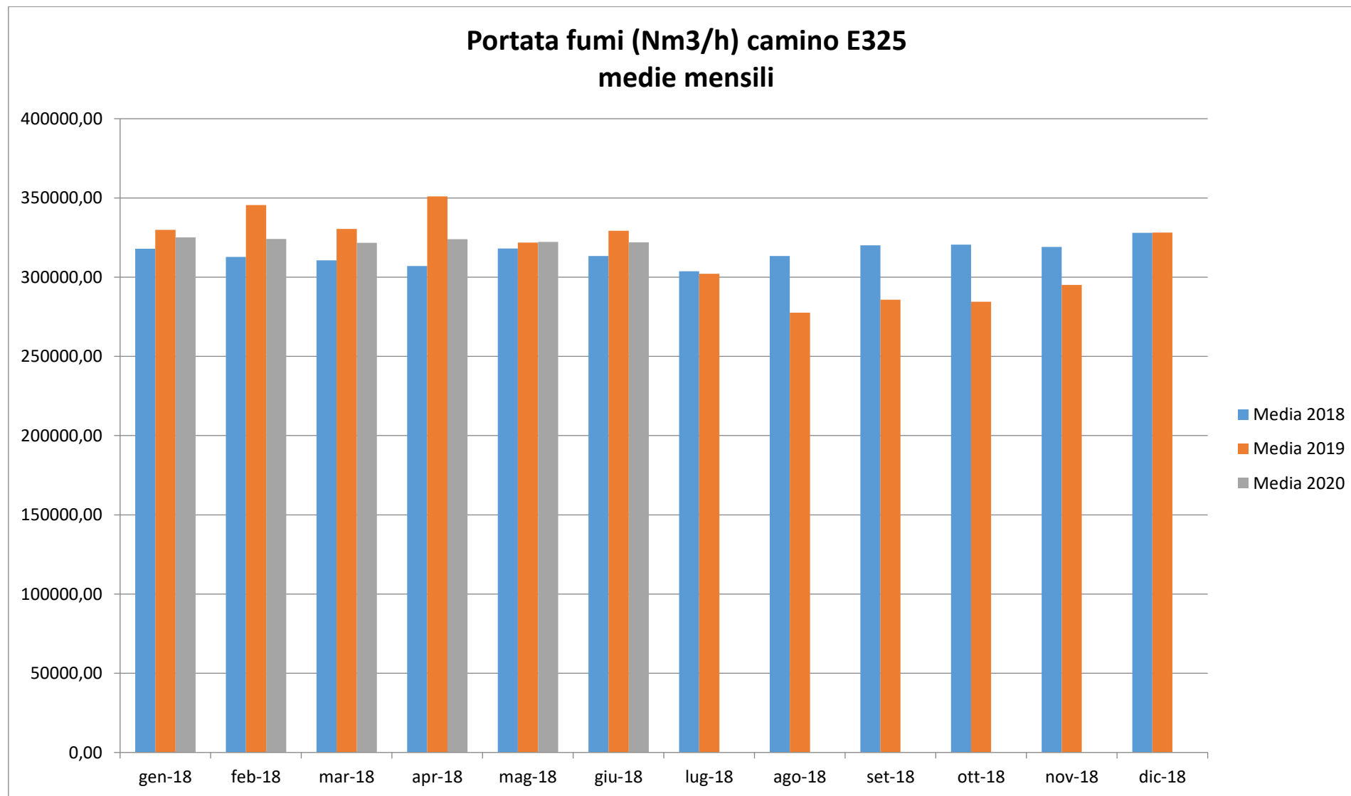
Figura 12. Esercizio Camino E325 Area Agglomerato, periodo gennaio 2018 – giugno 2020
