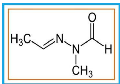
Figura 79. Formula di struttura della Giromitrina 66 [Arrangiamento grafico di C. Siniscalco - © - Archivio GMEM - AMB]
