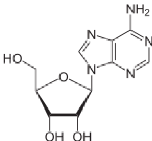
Figura 8. Formula di struttura dell'Adenosina 17 [Arrangiamento grafico di C. Siniscalco - © - Archivio GMEM - AMB]
