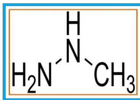
Figura 80. Formula di struttura della Monometilidrazina 67 [Arrangiamento grafico di C. Siniscalco - © - Archivio GMEM - AMB]
