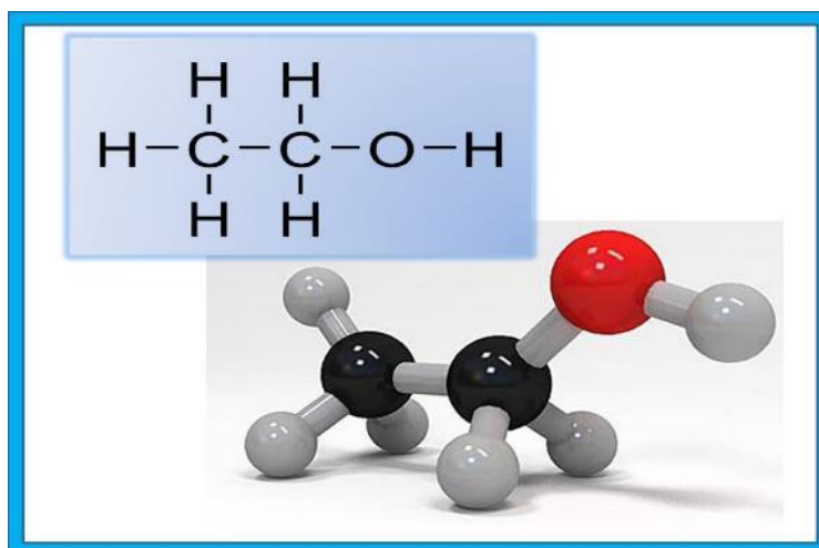
Figura 53. Immagini della formula dell'alcol etilico o etanolo 51 [Arrangiamento grafico di C. Siniscalco - © - Archivio GMEM - AMB]
