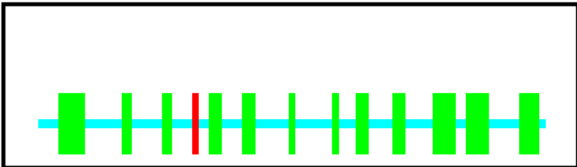
Figura 12. Struttura della proteina monomerica Clitocypin 19 [Arrangiamento grafico di C. Siniscalco - © - Archivio GMEM - AMB]
