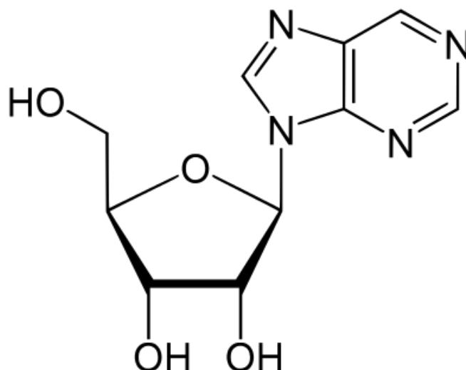
Figura 6. Formula di struttura della Nebularina 16 [Arrangiamento grafico di C. Siniscalco - © - Archivio GMEM - AMB]
