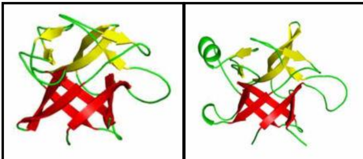
Figura 13. Esempio della struttura cristallina di due peptidasi 20 [Arrangiamento grafico di C. Siniscalco - © - Archivio GMEM - AMB]
