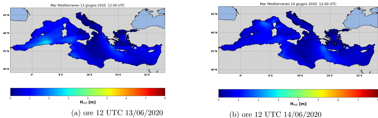
Figura 1: MCWAF ISPRA - altezza significativa ( H_{m0} ) Mar Mediterraneo
