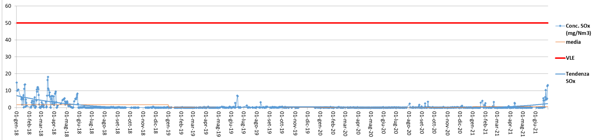
Concentrazione SOx (mg/Nm3) camino E325 - Anni 2018-2019-2020-2021
