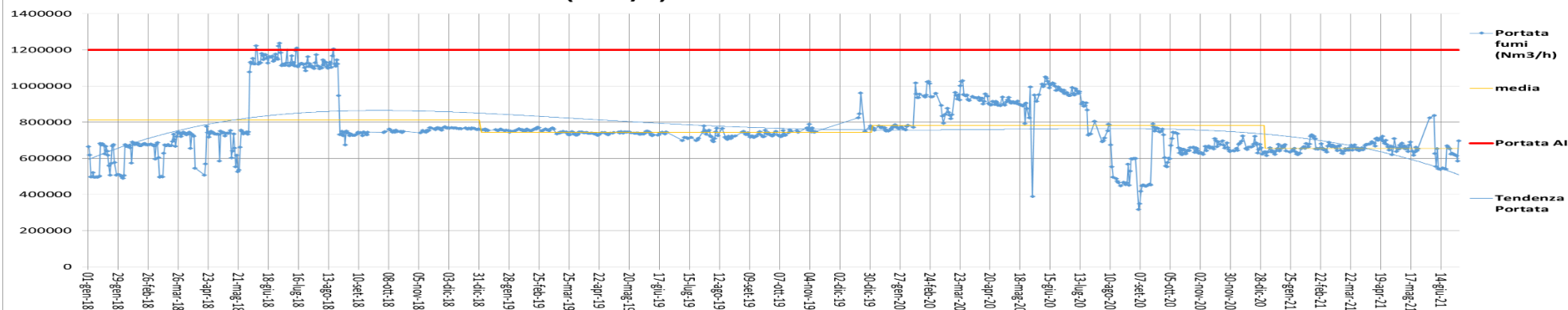
Portata fumi (Nm3/h) camino E315b - Anni 2018-2019-2020-2021
