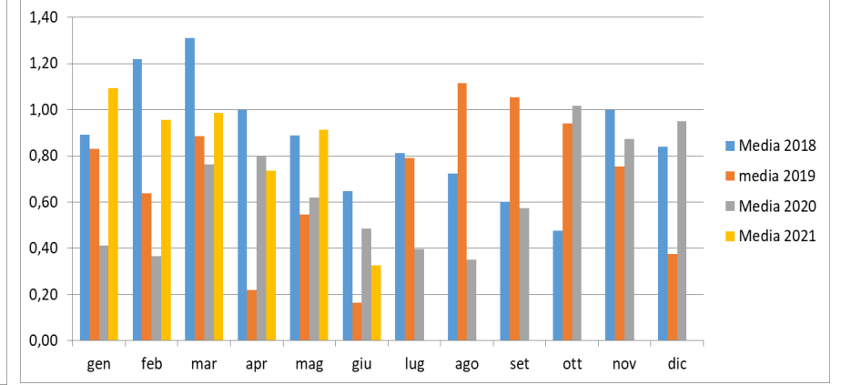
Concentrazione polveri (mg/Nm3) camino E325 medie mensili
