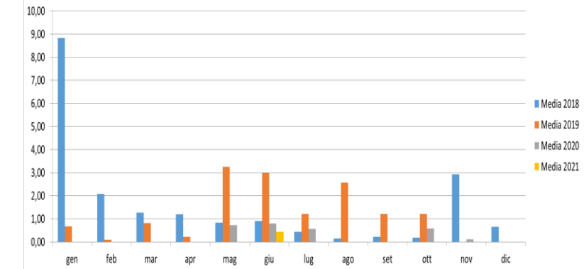
Concentrazione SOx (mg/Nm3) camino E315b medie mensili
