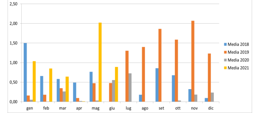
Concentrazione polveri (mg/Nm3) camino E315b medie mensili
