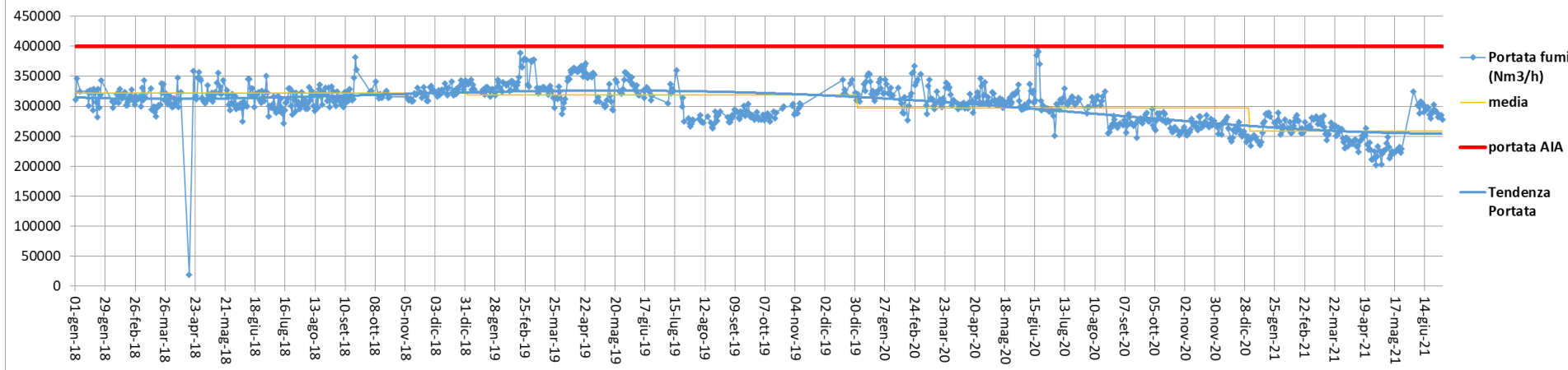
Portata fumi (Nm3/h) camino E325 - Anni 2018-2019-2020-2021
