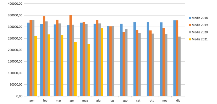
Portata fumi (Nm3/h) camino E325 medie mensili
