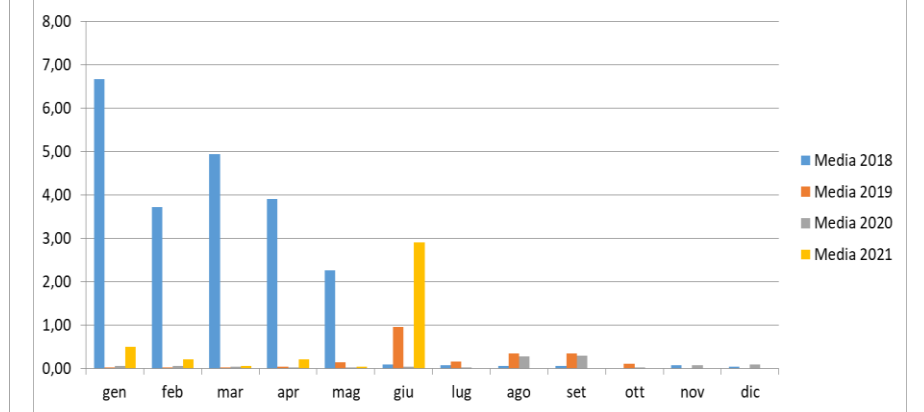
Concentrazione SOx (mg/Nm3) camino E325 medie mensili
