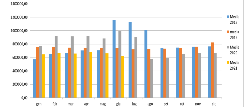
Portata fumi (Nm3/h) camino E315b medie mensili
