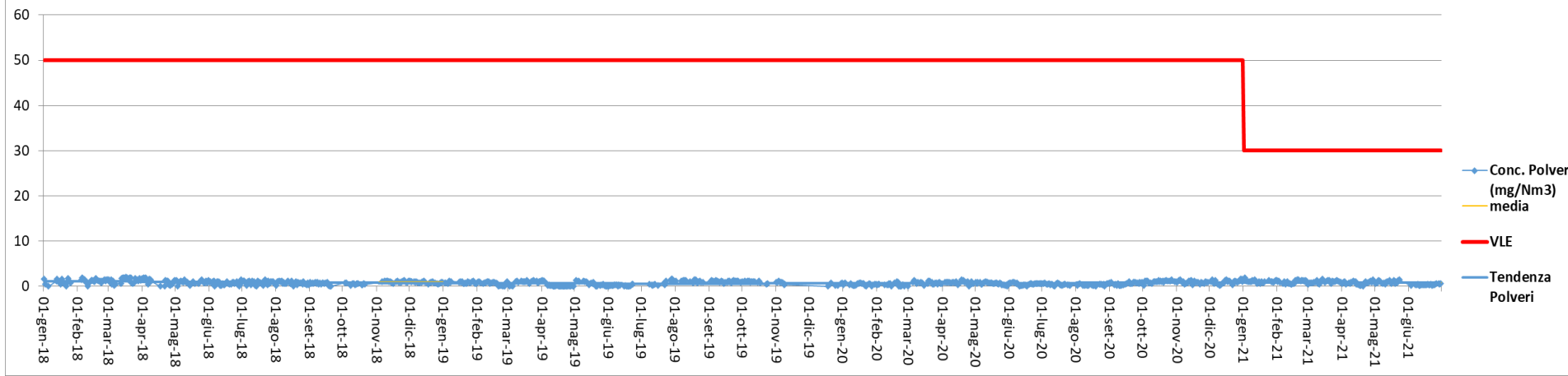
Concentrazione polveri (mg/Nm3) camino E325 - Anni 2018-2019-2020-2021
