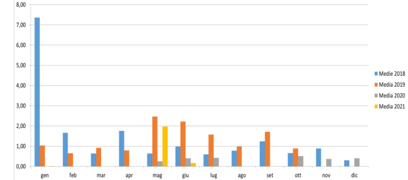
Concentrazione NOx (mg/Nm3) camino E315b medie mensili
