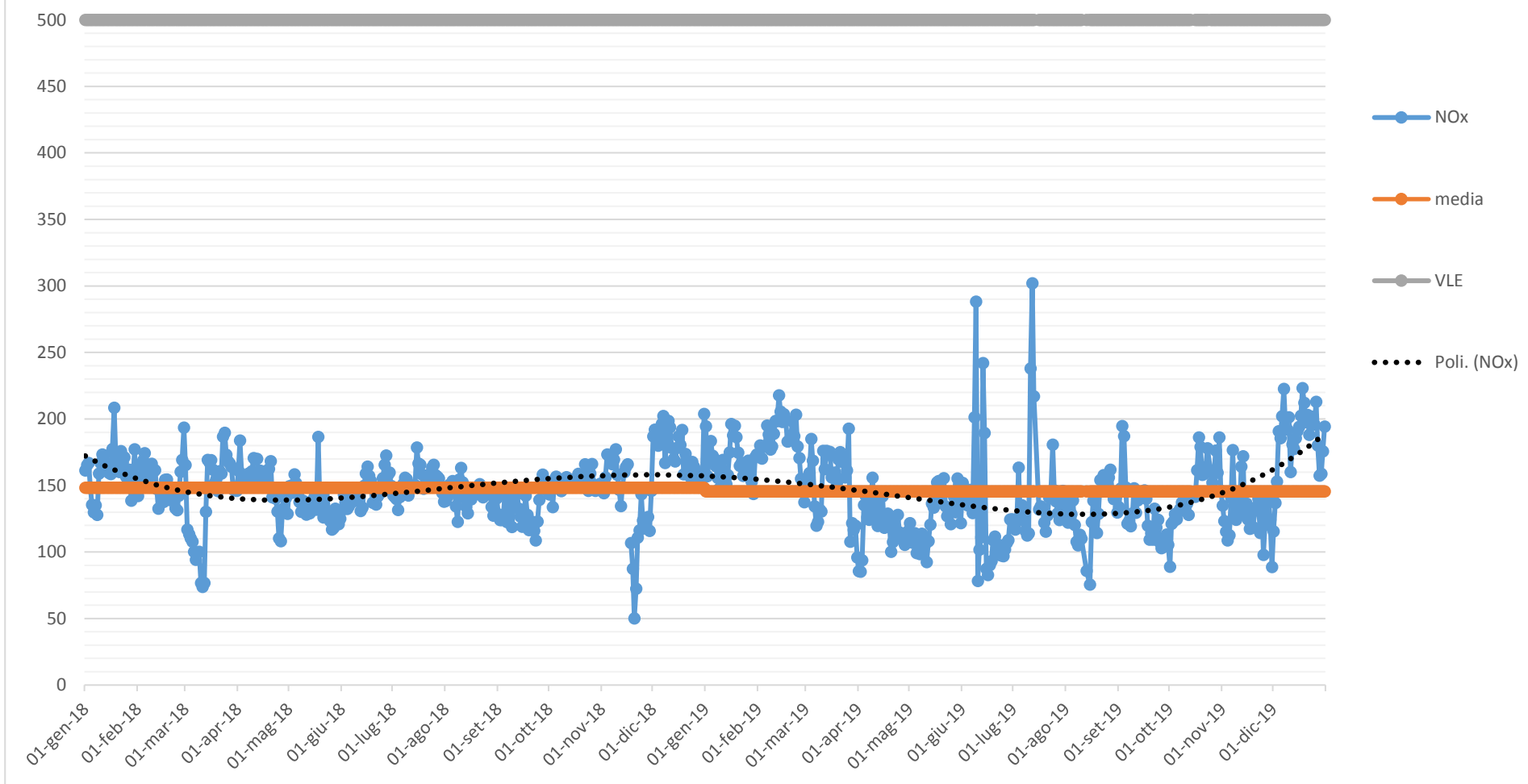
Concentrazione NOx (mg/Nm3, media giornaliera) camino E428 cokeria - ANNO 2018-2019
