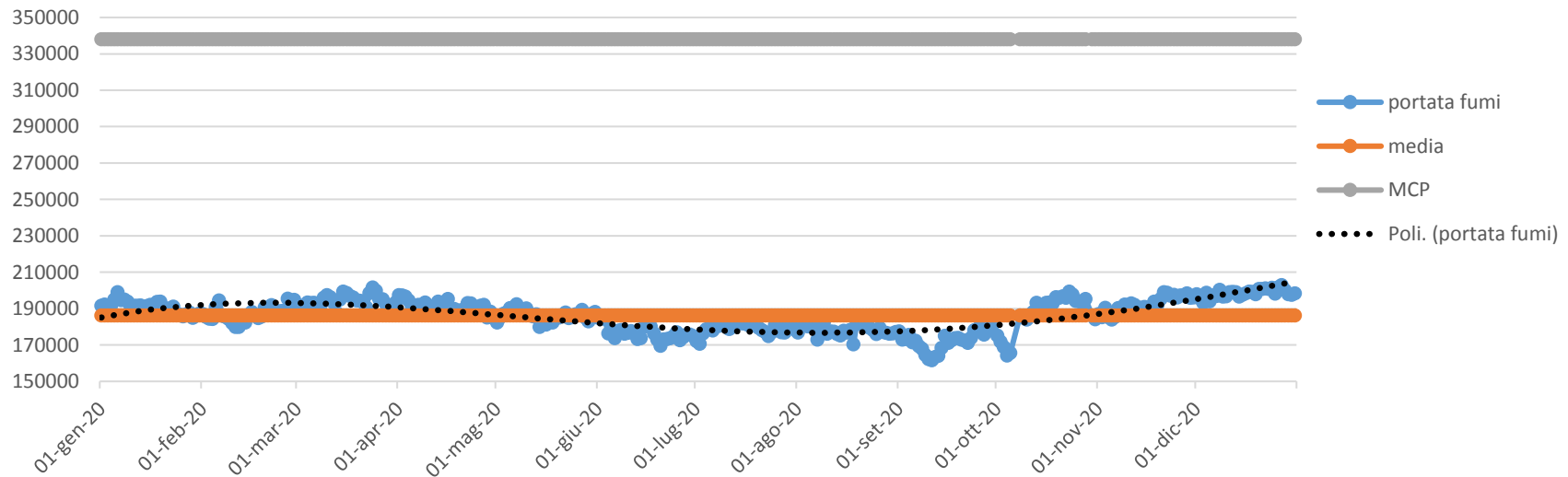
Portata fumi (Nm3/h) camino E436 cokeria - anno 2020
