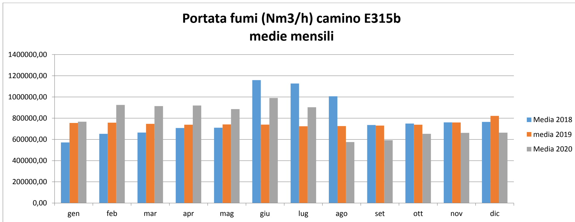
Figura 10. Esercizio Camino E315b Area Agglomerato, periodo gennaio 2018 – dicembre 2020
