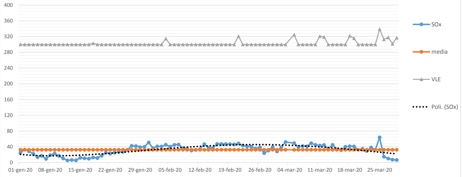
Concentrazione SOx (mg/Nm3, media giornaliera) camino E426 - ANNO 2020
