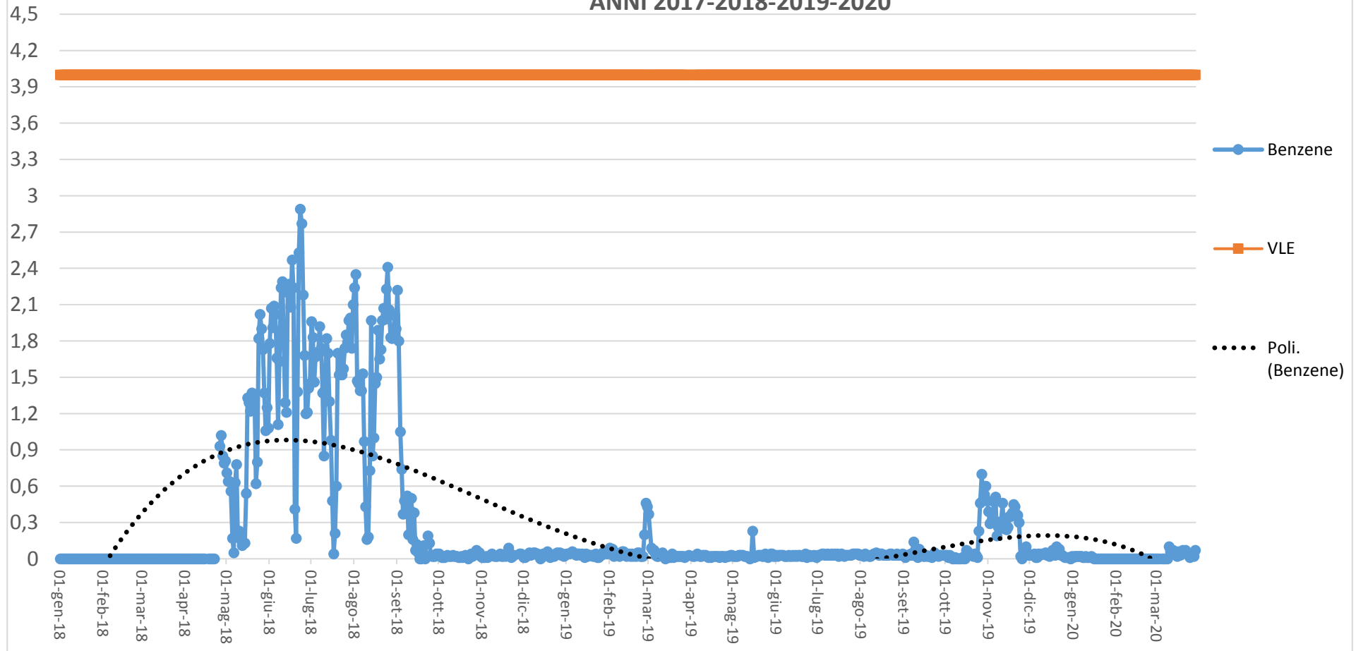
Concentrazione Benzene (mg/Nm 3 , media giornaliera) camino E426 ANNI 2017-2018-2019-2020
