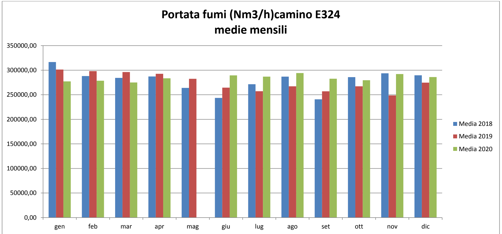
Figura 11. Esercizio Camino E324 Area Agglomerato, periodo gennaio 2018 – dicembre 2020
