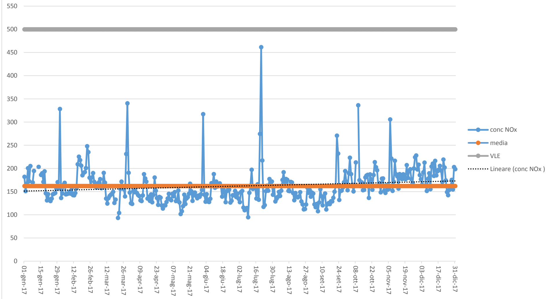
Concentrazione NOx (mg/Nm3, media giornaliera) camino E424 cokeria - ANNO 2017
