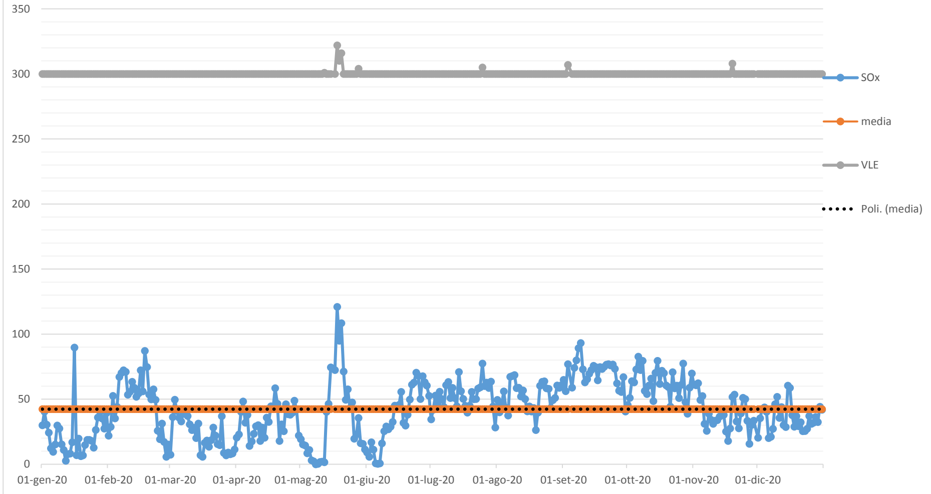
Concentrazione SOx (mg/Nm3, media giornaliera) camino E428 -ANNO 2020
