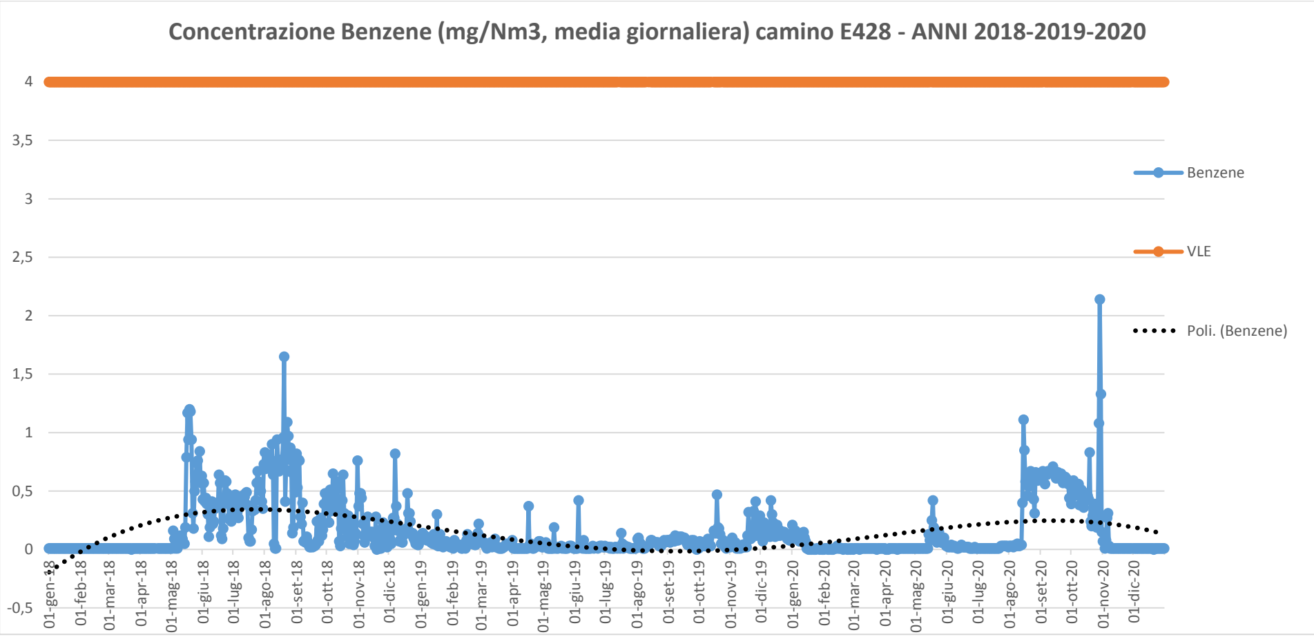
FIG. 7 – Trend Benzene camini cokefazione
