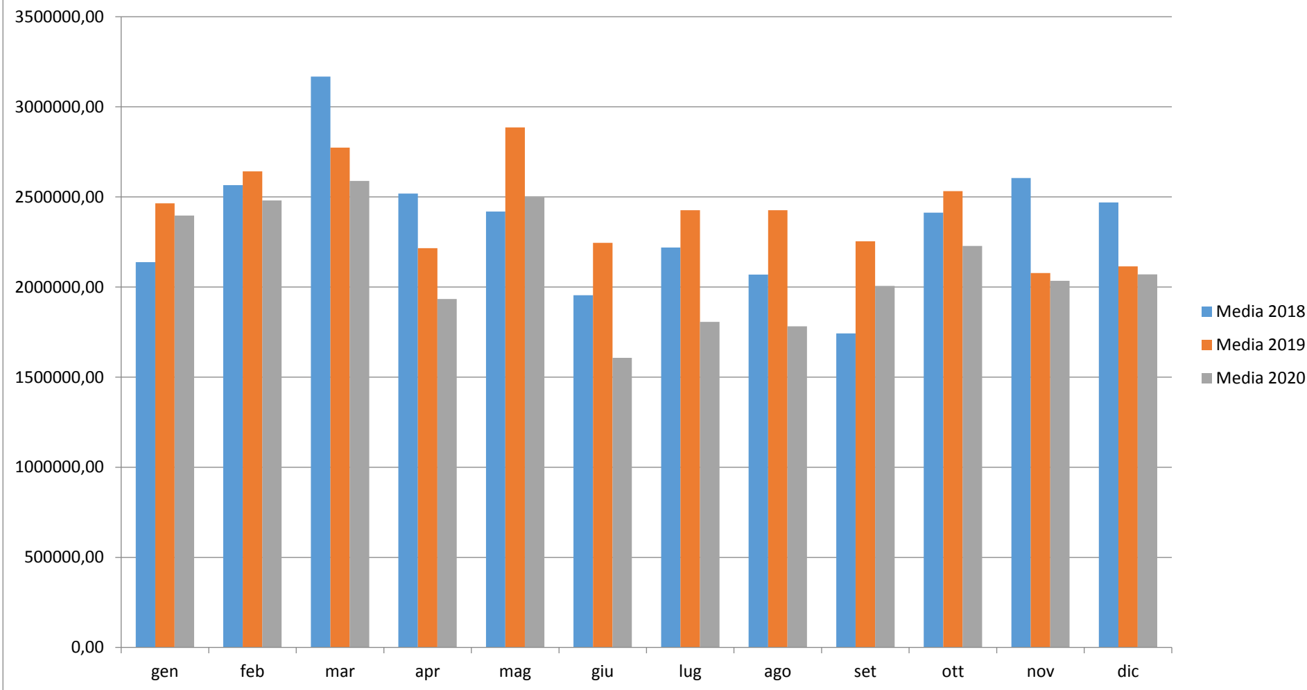
Figura 8. Esercizio Camino E312 Area Agglomerato, periodo gennaio 2018 – dicembre 2020
