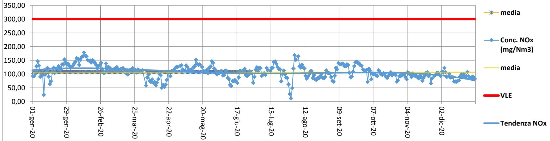
Concentrazione NOx (mg/Nm3) - camino E312 - Anno 2020
