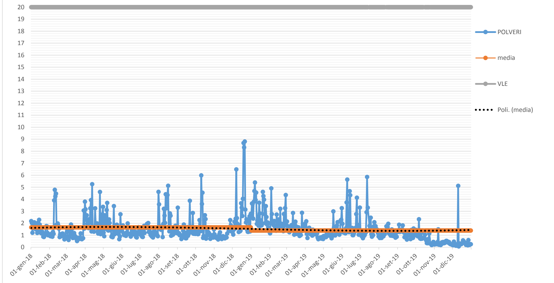
Concentrazione polveri (mg/Nm3, media giornaliera) camino E428 - ANNO 2018/2019
