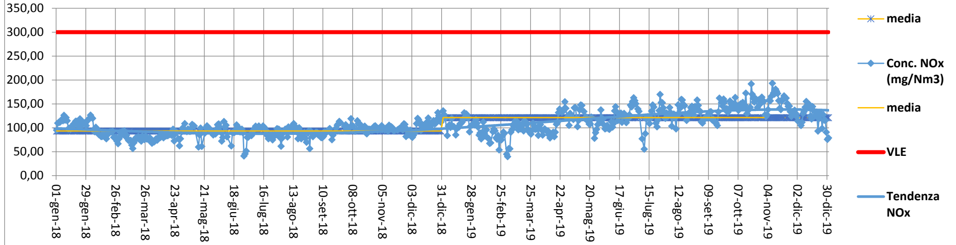
Concentrazione NOx (mg/Nm3) - camino E312 - Anni 2018 - 2019
