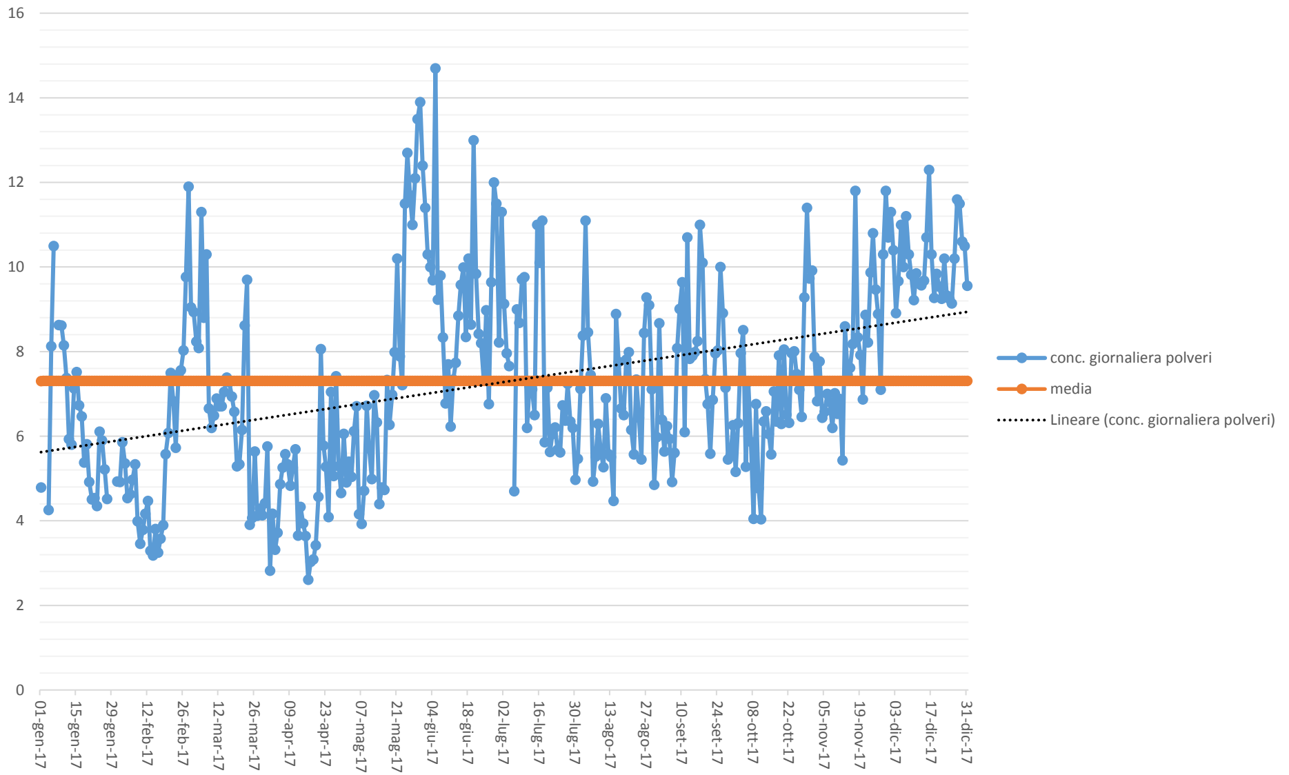
Concentrazione polveri (mg/Nm3, media giornaliera) camino E426 - ANNO 2017
