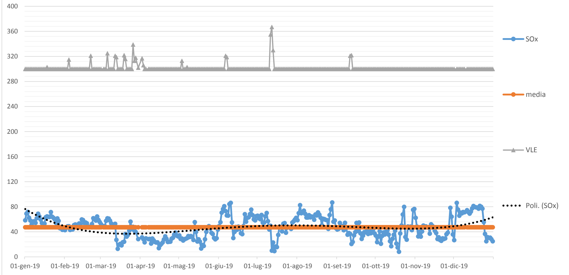
Concentrazione SOx (mg/Nm3, media giornaliera) camino E426 - ANNO 2019
