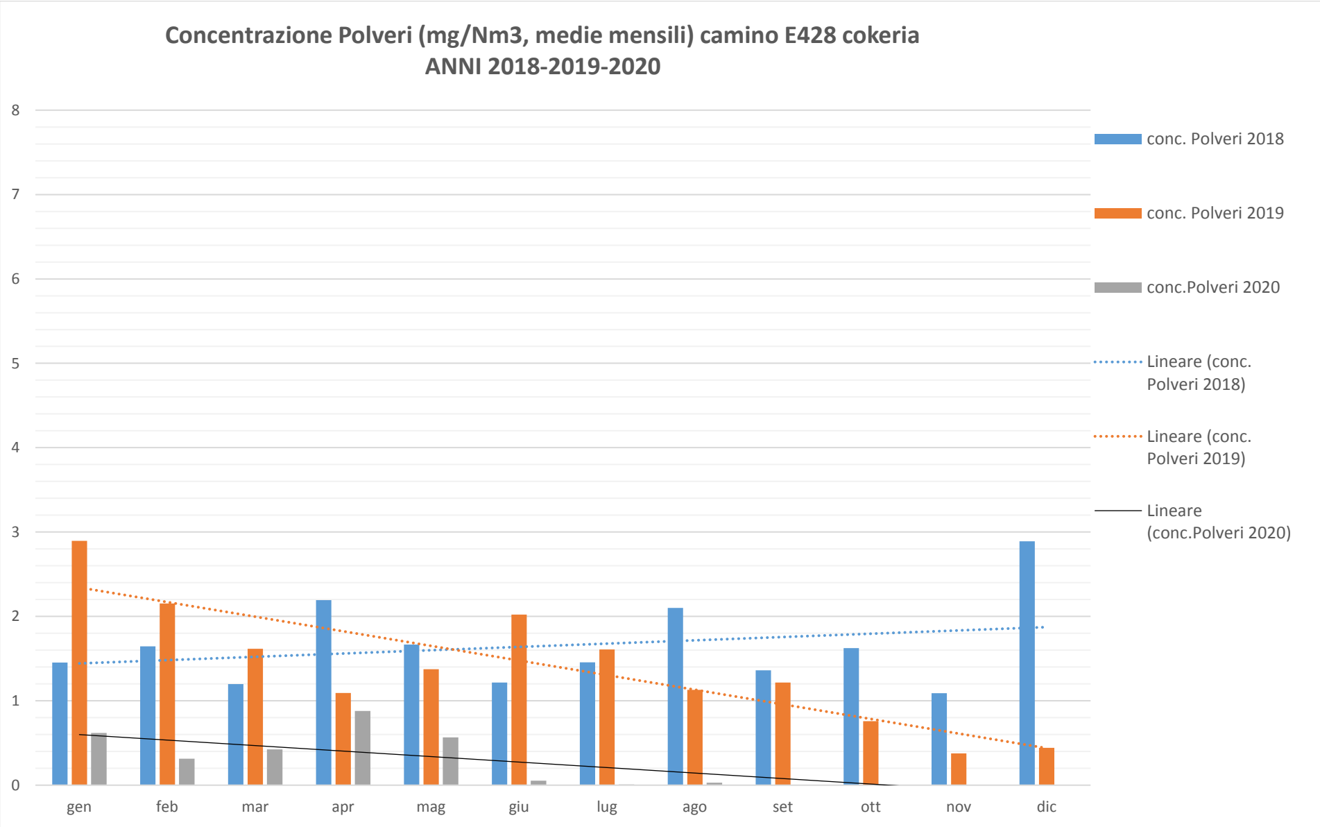
FIG. 3 – Camino E428 - COKEFAZIONE
