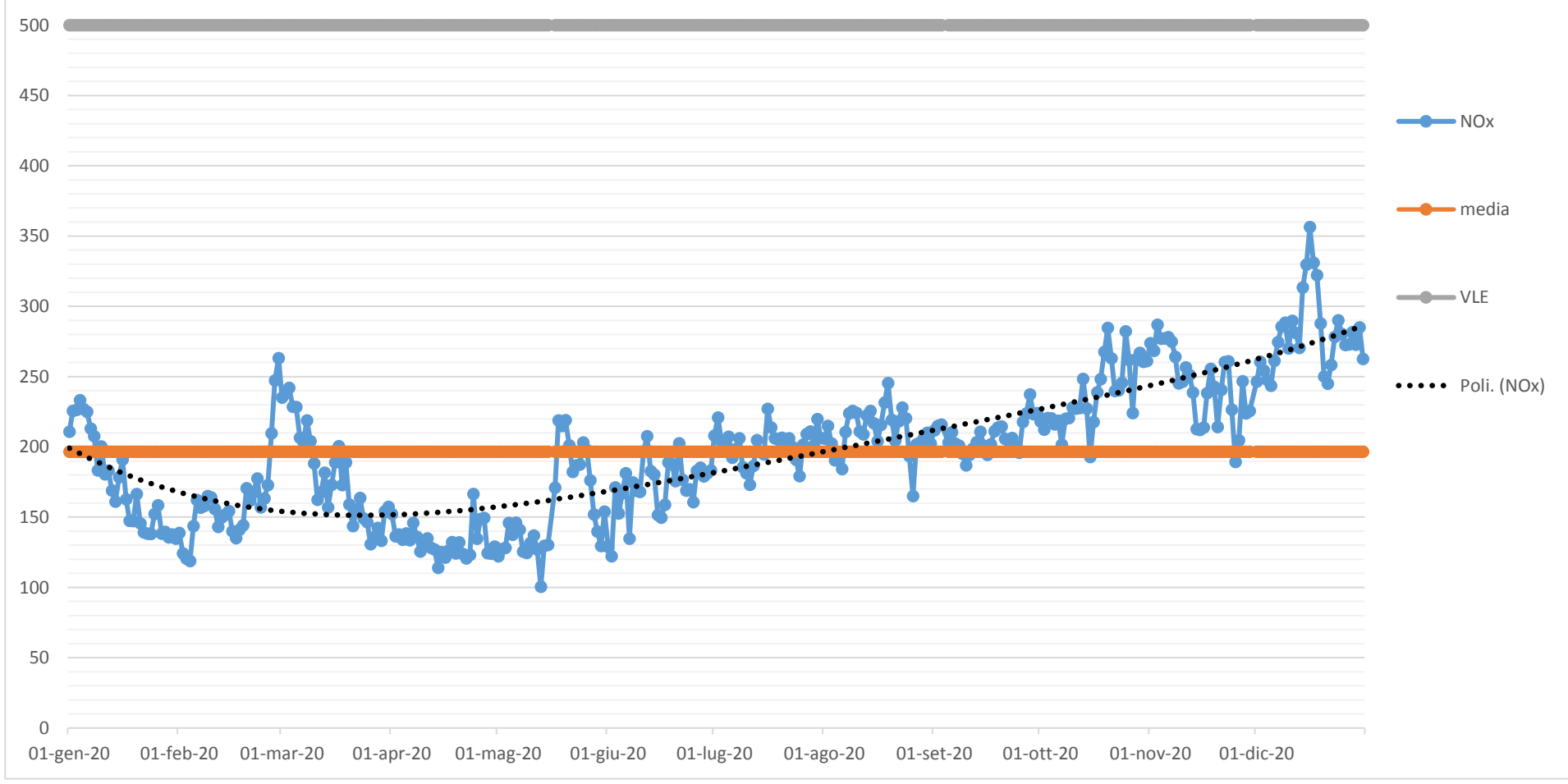
Concentrazione NOx (mg/Nm3, media giornaliera) camino E428 cokeria - ANNO 2020
