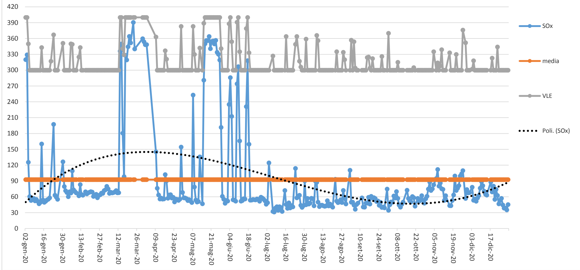
Concentrazione SOx (mg/Nm3, media giornaliera) camino E424 - ANNO 2020
