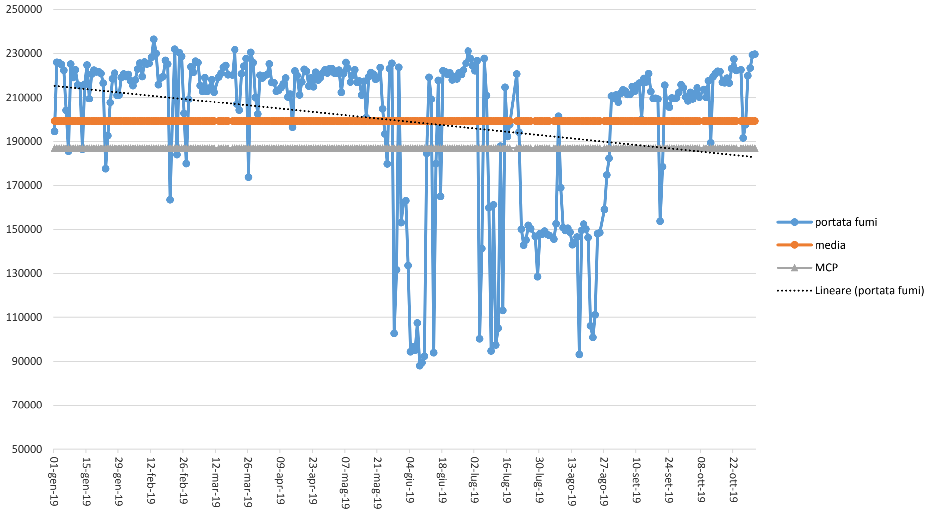
Portata fumi (Nm 3 /h) camino 4 (E424) cokeria - anno 2019
