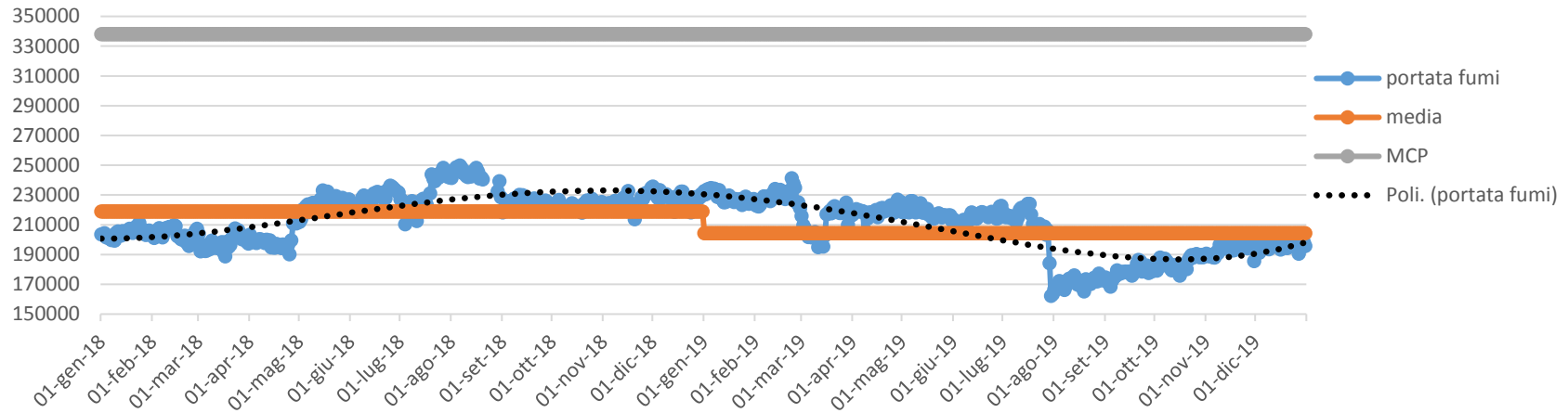
Portata fumi (Nm3/h) camino E436 cokeria - anno 2018/19
