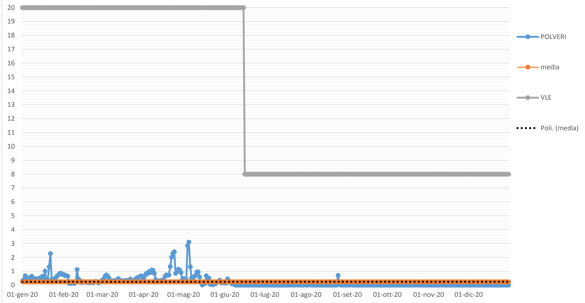
Concentrazione polveri (mg/Nm3, media giornaliera) camino E428 - ANNO 2020
