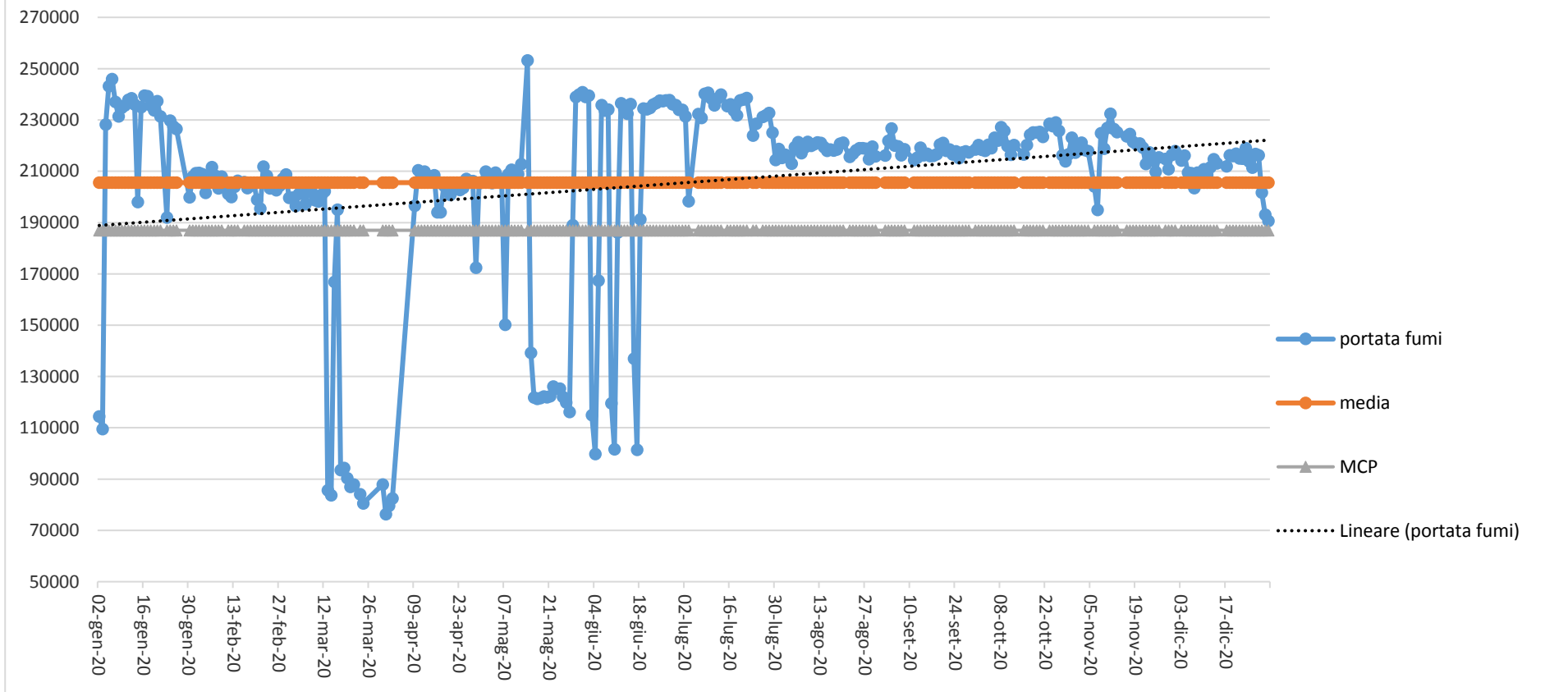
Portata fumi (Nm3/h) camino 4 (E424) cokeria - anno 2020
