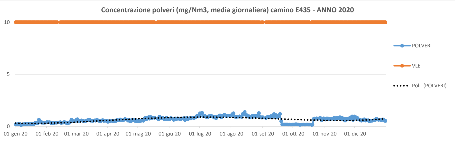
FIG. 4 – Camino E435 – SFORNAMENTO COKE
