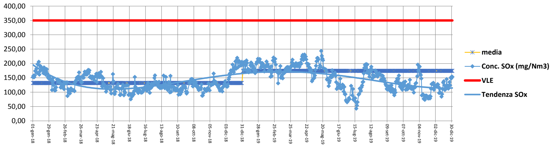
Concentrazione SOx (mg/Nm3) - Camino E312 - Anni 2018 - 2019
