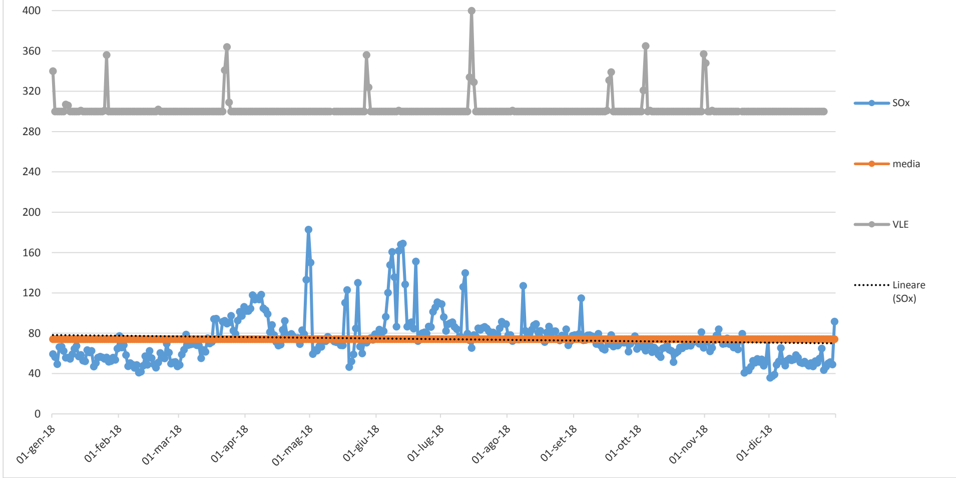
Concentrazione SOx (mg/Nm3, media giornaliera) camino E424 - ANNO 2018
