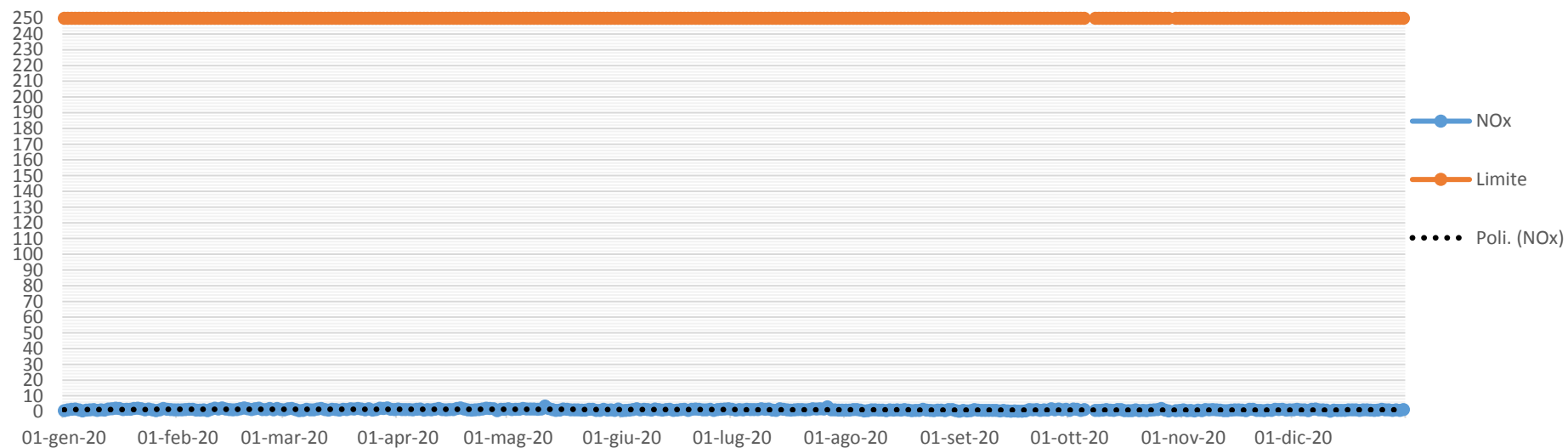
Concentrazione di NOx (mg/Nm3, media giornaliera) camino E436 cokeria - ANNO 2020
