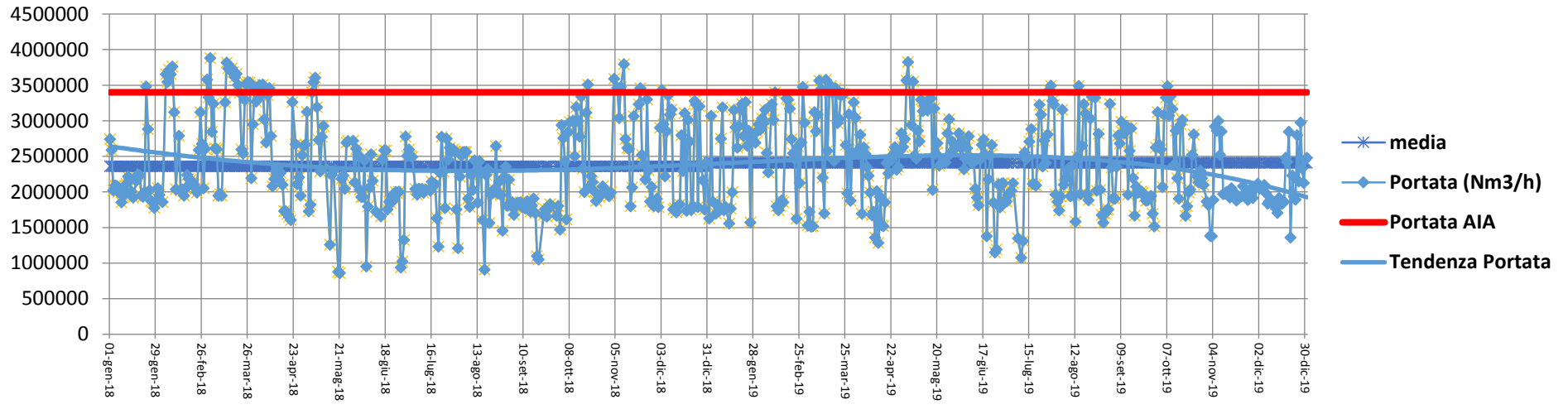
Portata fumi (Nm3/h) - Camino E312 - Anni 2018 - 2019
