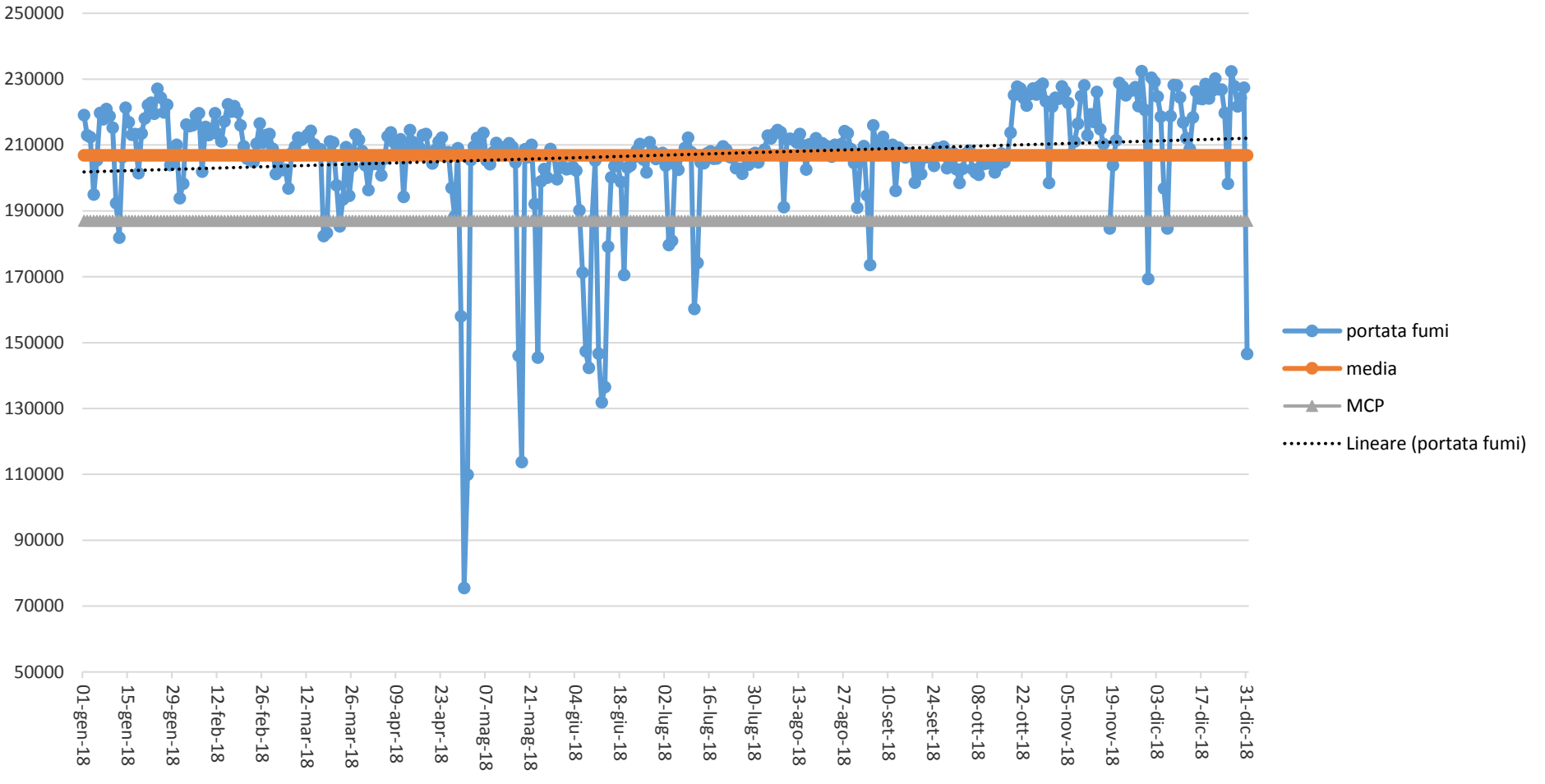
Portata fumi (Nm3/h) camino 4 (E424) cokeria - anno 2018
