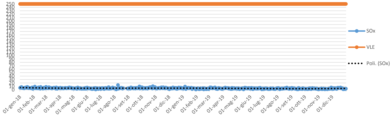
Concentrazione SOx (mg/Nm3, media giornaliera) camino E436 - ANNO 2018/19
