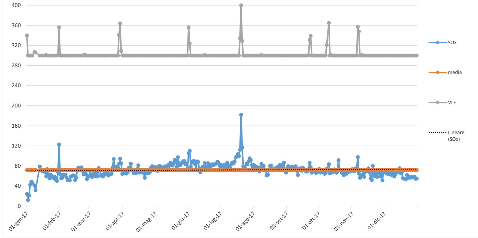
Concentrazione SOx (mg/Nm3, media giornaliera) camino E424 - ANNO 2017
