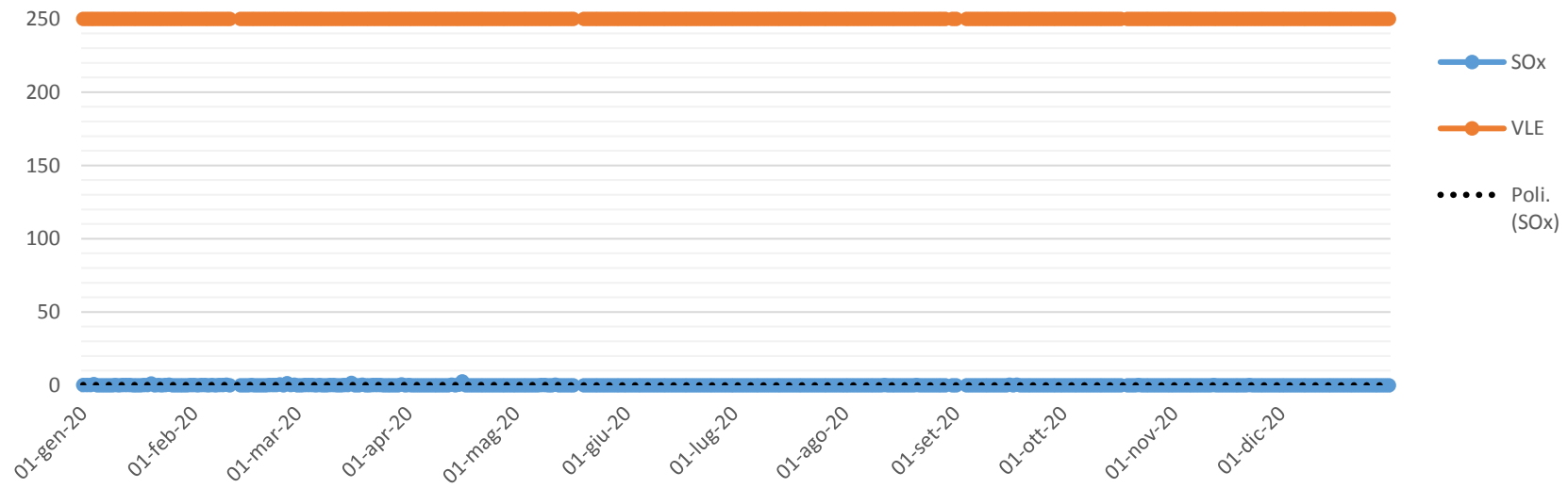
Concentrazione SOx (mg/Nm3, media giornaliera) camino E435 - ANNO 2020
