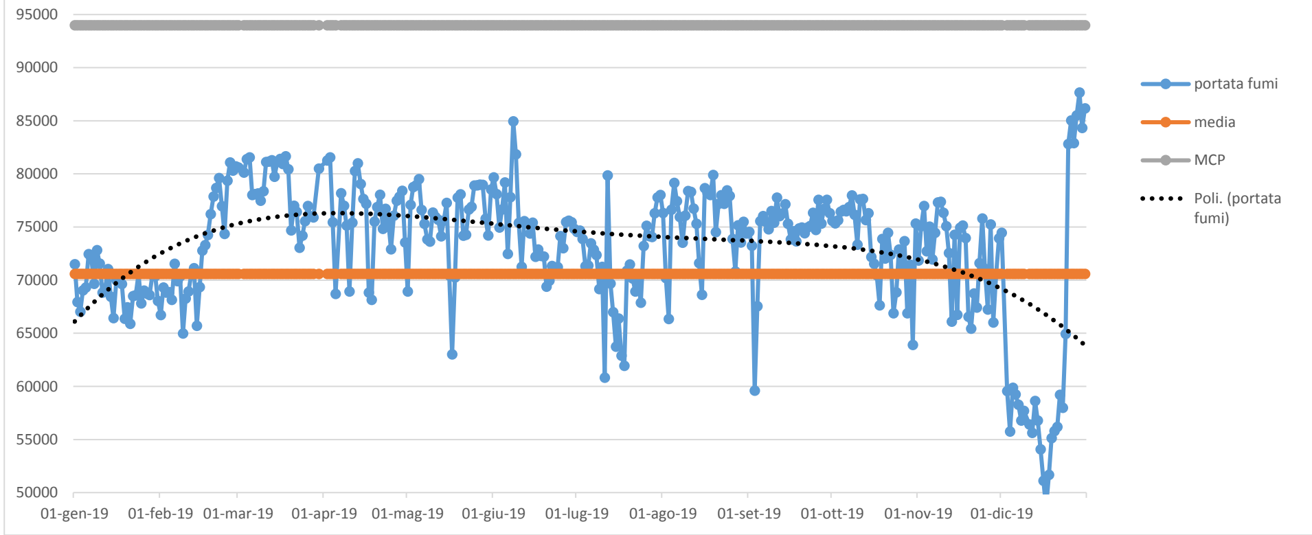
Portata fumi (Nm3/h) camino (E426) cokeria - anno 2019
