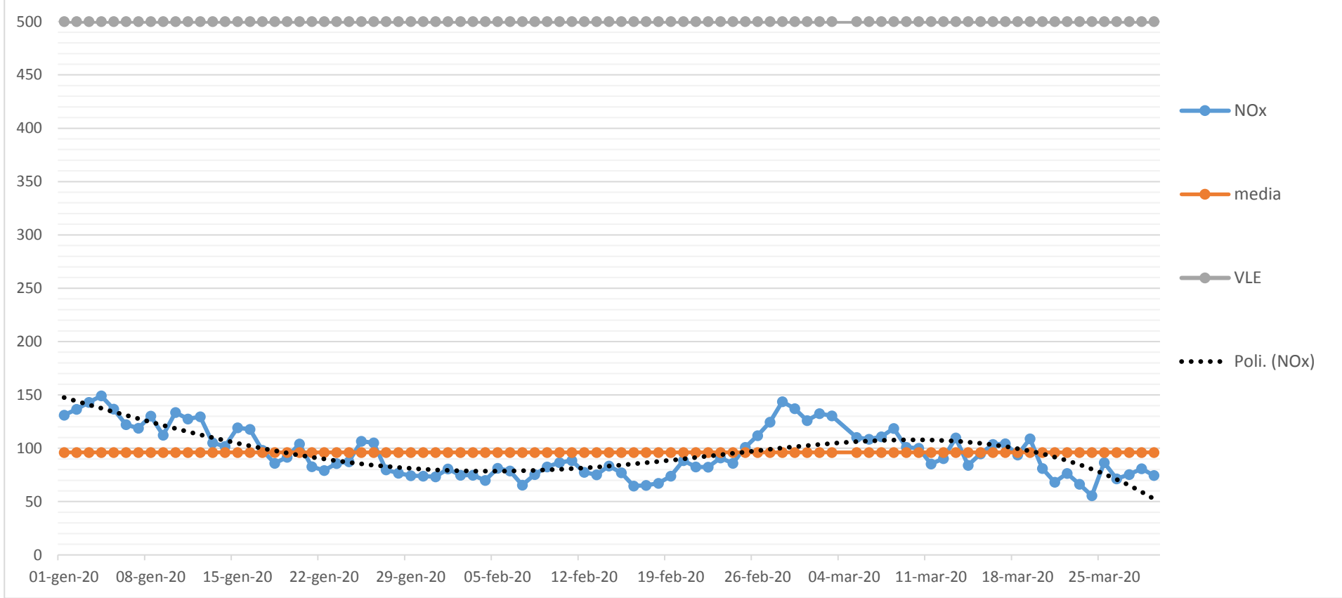
Concentrazione di NOx (mg/Nm3, media giornaliera) camino E426 cokeria - ANNO 2020
