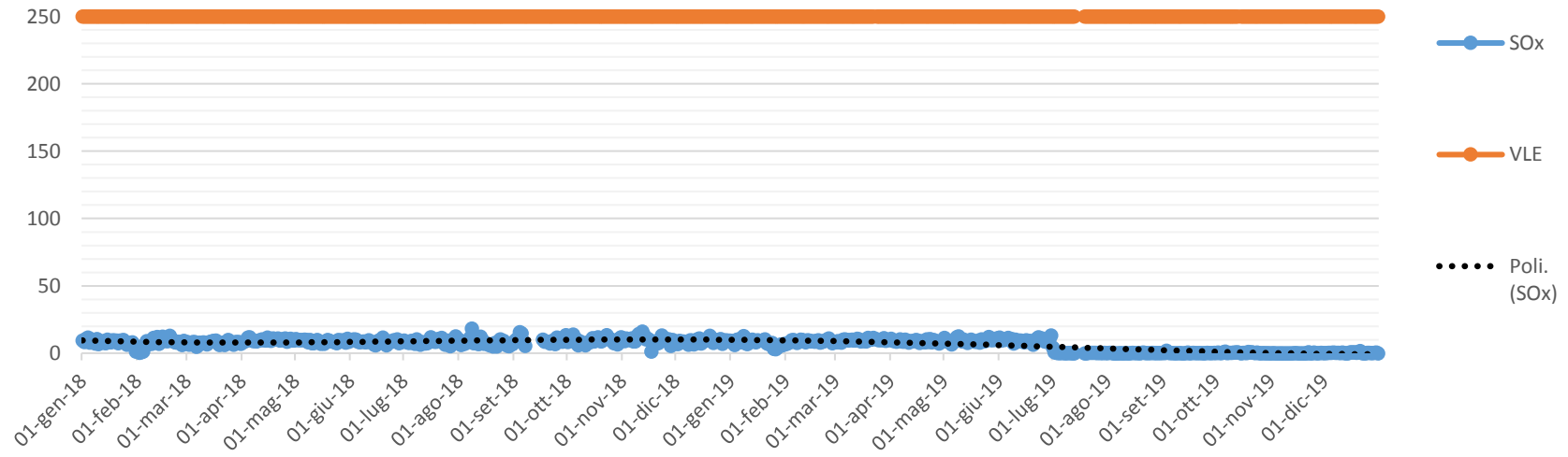
Concentrazione SOx (mg/Nm3, media giornaliera) camino E435 - ANNO 2018/19
