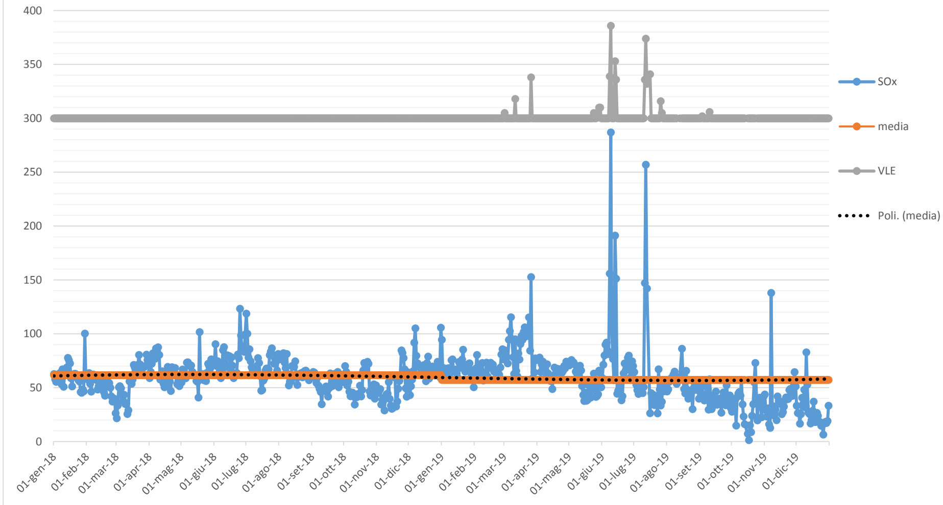
Concentrazione SOx (mg/Nm3, media giornaliera) camino E428 -ANNO 2018/19
