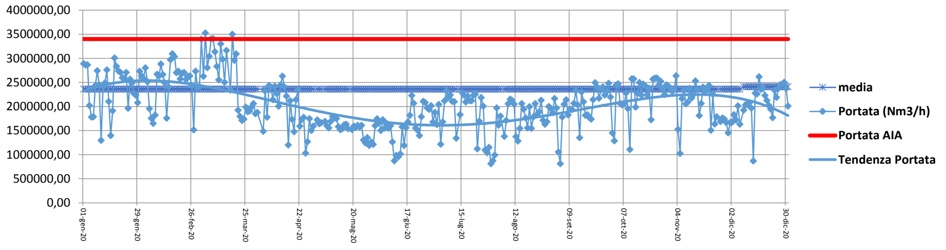
Portata fumi (Nm3/h) - Camino E312 - Anno 2020
