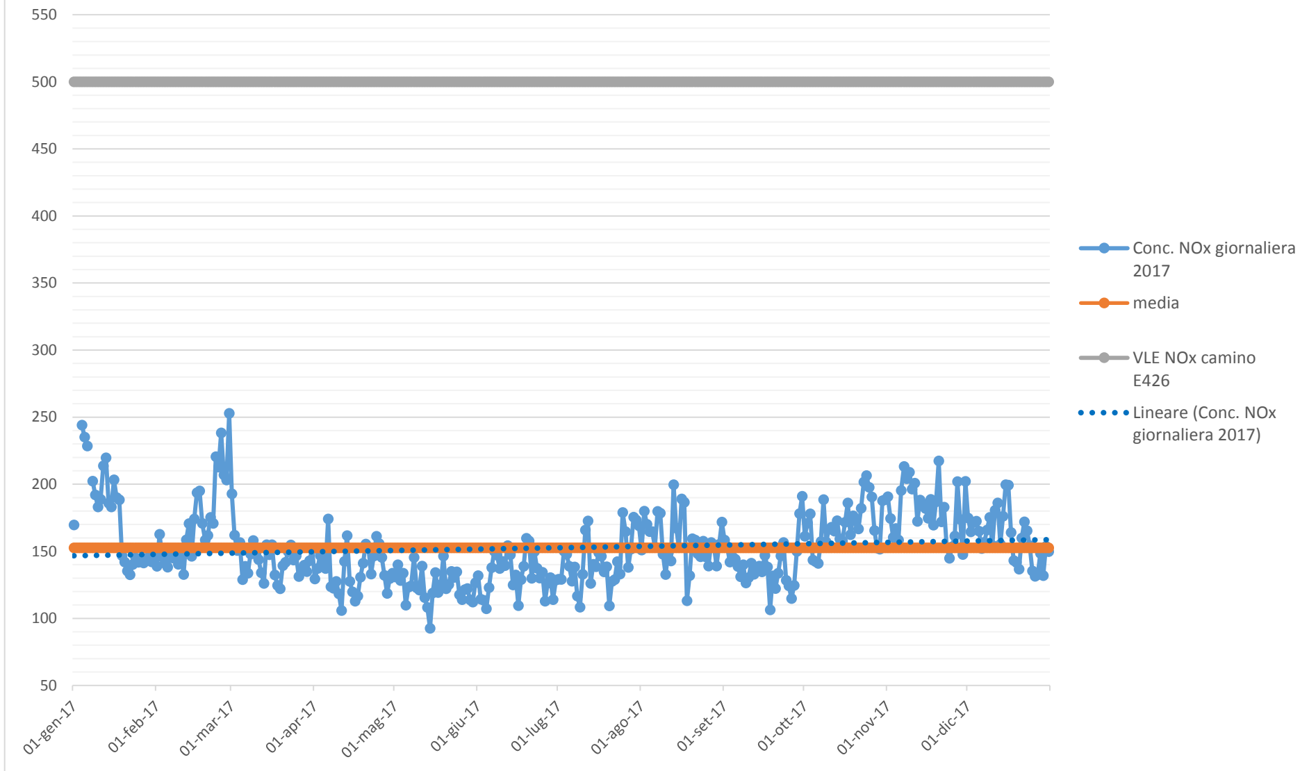
Concentrazione NOx (mg/Nm3, media giornaliera) camino E426 cokeria - ANNO 2017
