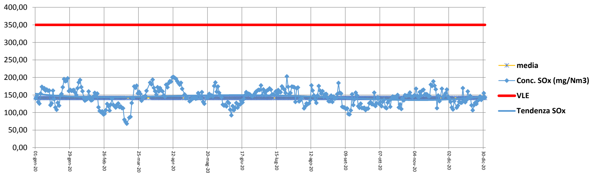
Concentrazione SOx (mg/Nm3) - Camino E312 - Anno 2020
