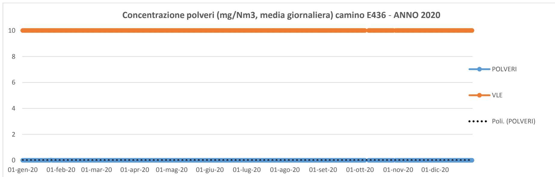
FIG. 5 – Camino E436 – SFORNAMENTO COKE
