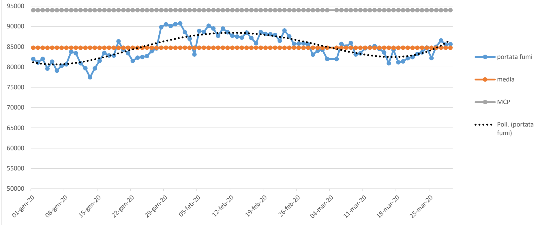
Portata fumi (Nm3/h) camino (E426) cokeria - anno 2020
