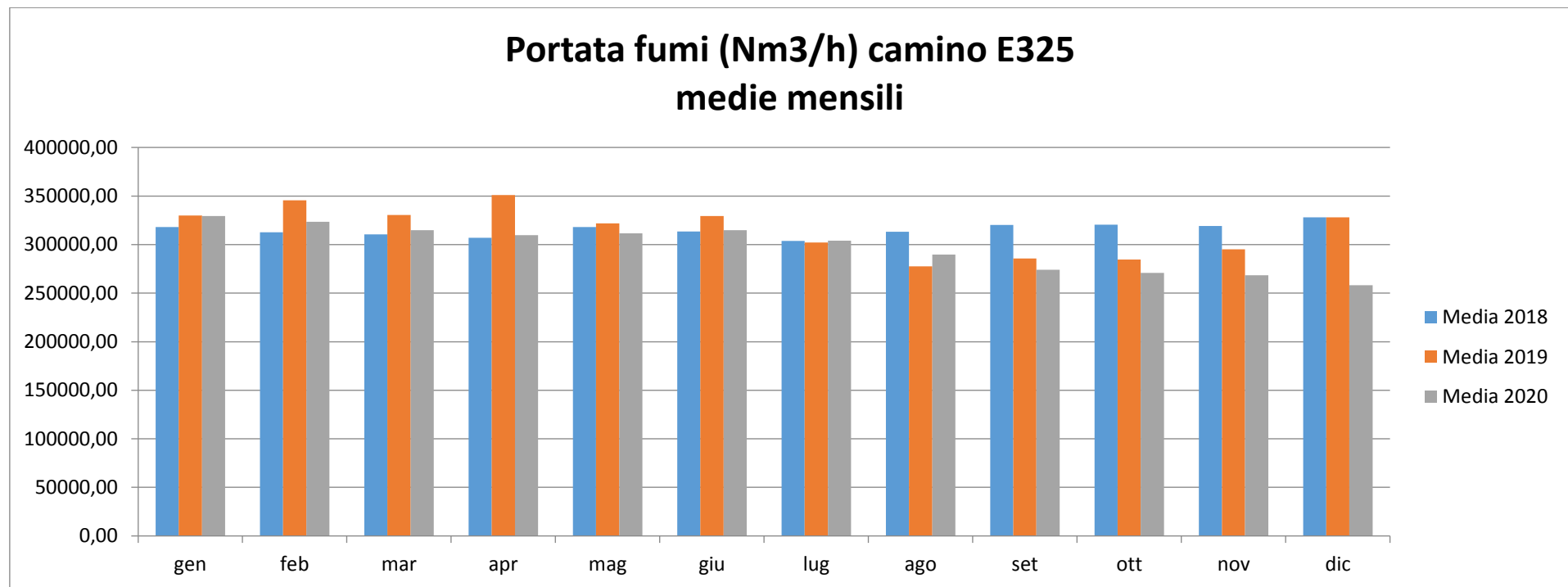
Figura 12. Esercizio Camino E325 Area Agglomerato, periodo gennaio 2018 – dicembre 2020
