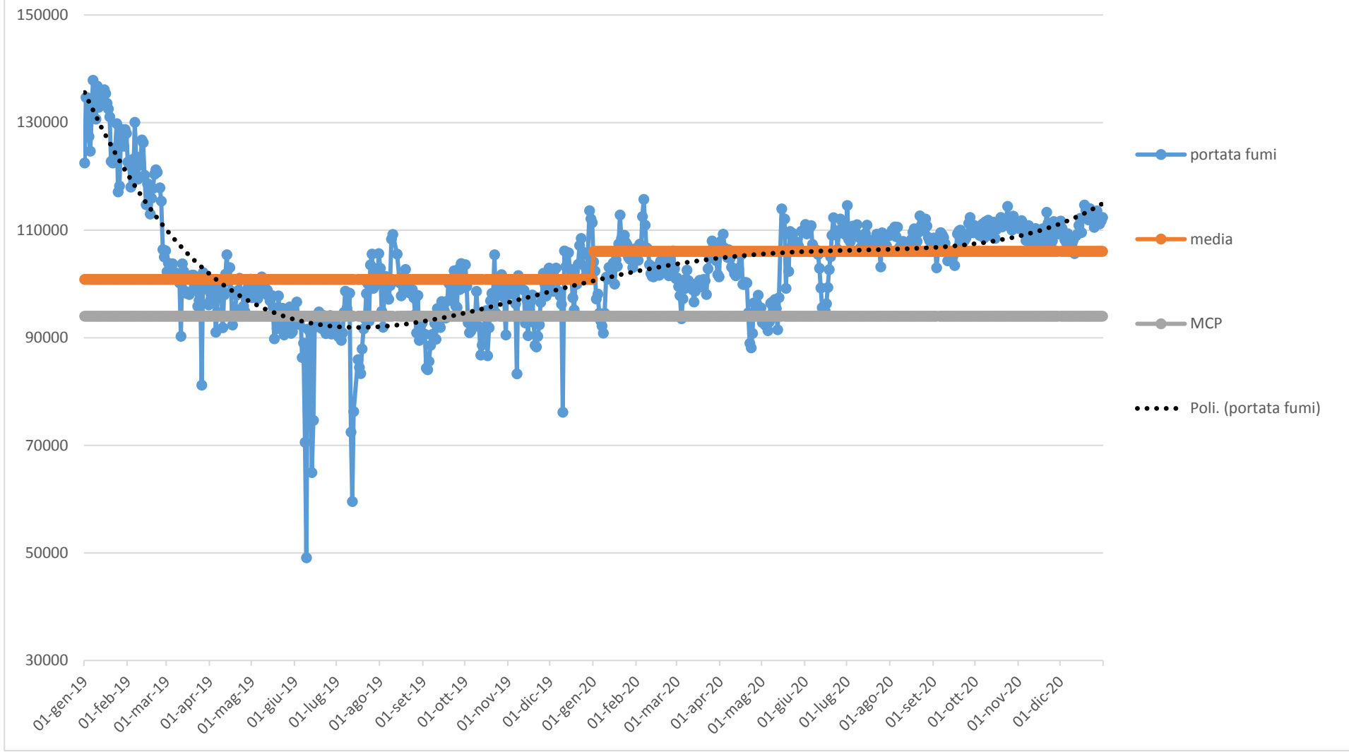
Portata fumi (Nm3/h) camino (E428) cokeria - anno 2019/2020
