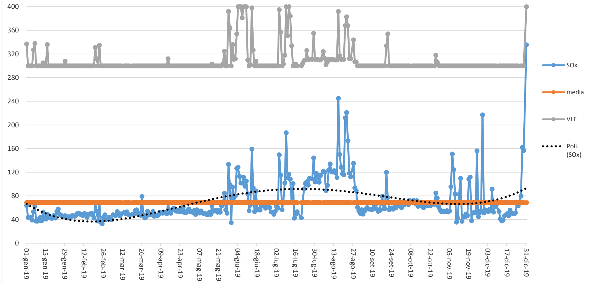
Concentrazione SOx (mg/Nm3, media giornaliera) camino E424 - ANNO 2019
