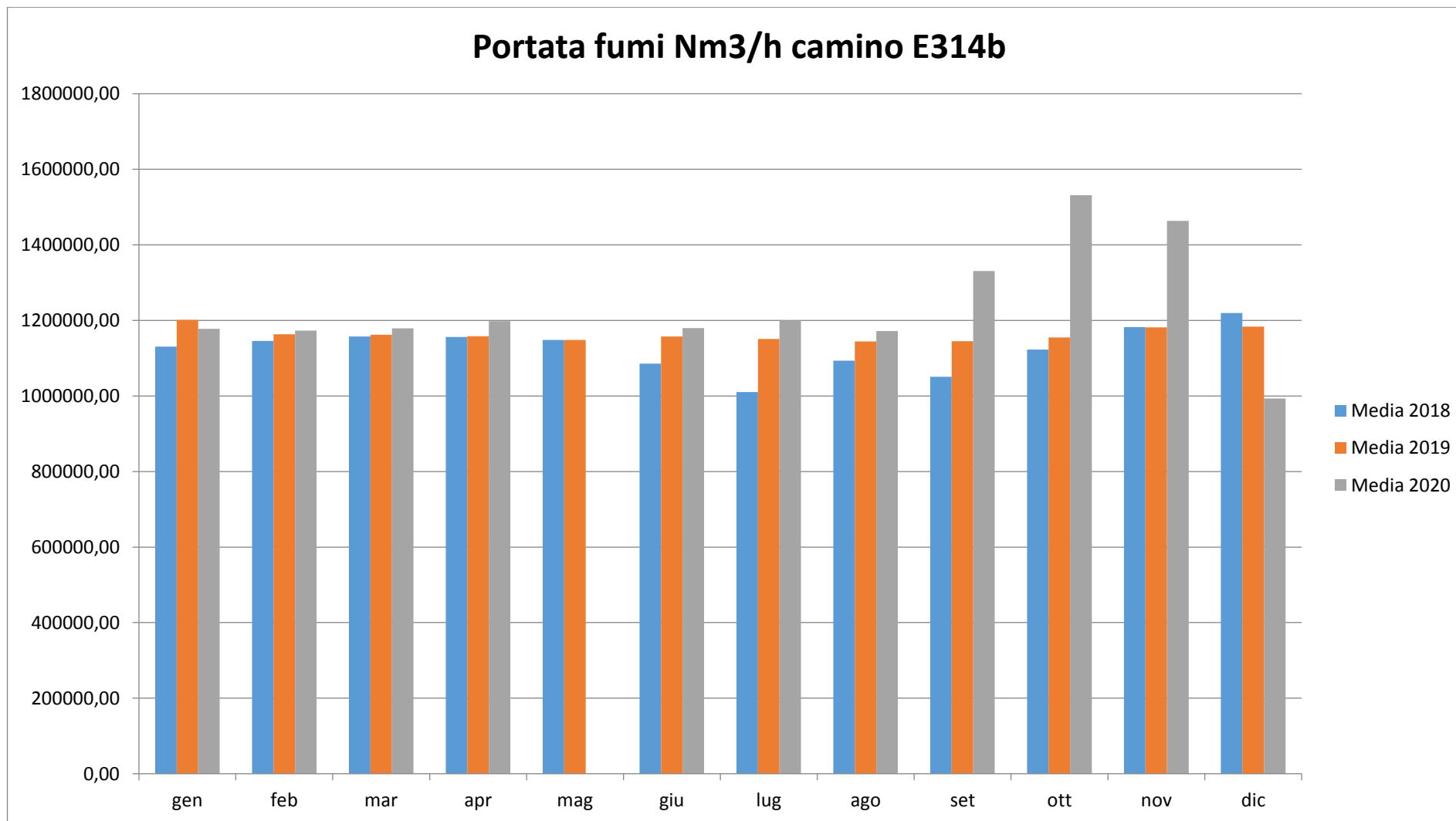
Figura 9. Esercizio Camino E314b Area Agglomerato, periodo gennaio 2018 – dicembre 2020
