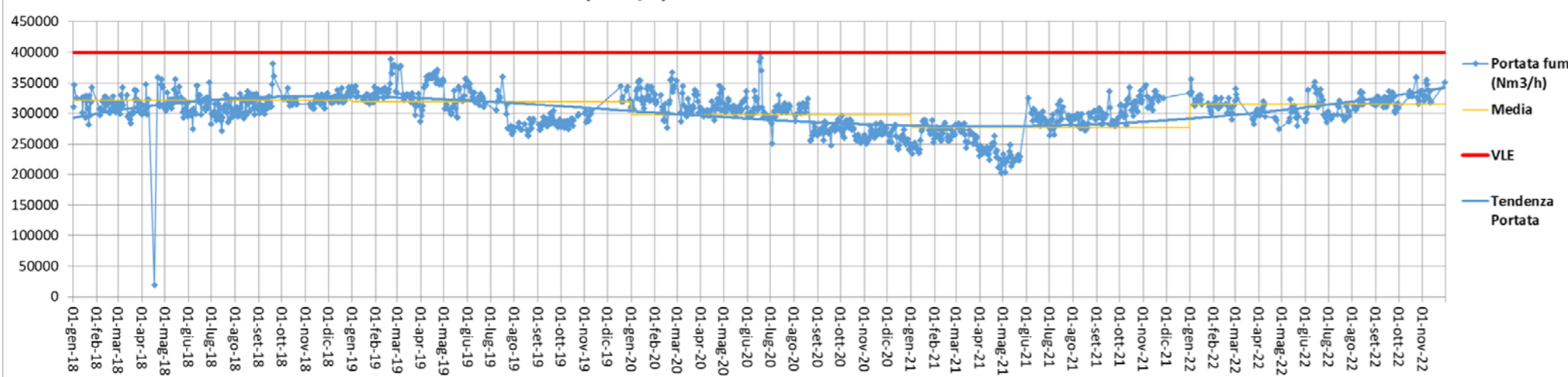
Portata fumi (Nm3/h) camino E325 - Anni 2018-2019-2020-2021-2022
