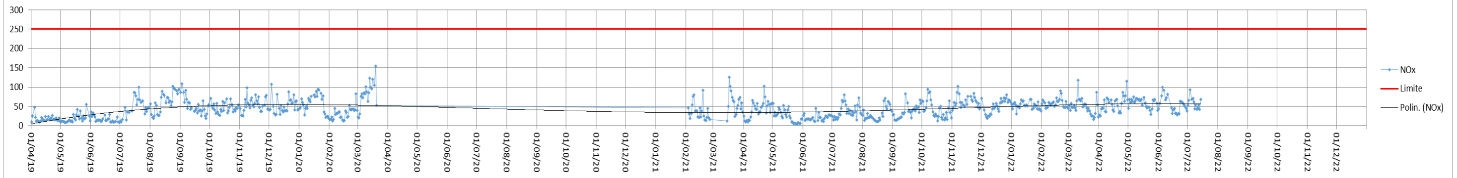
NOx (mg/Nm3) camino E135
