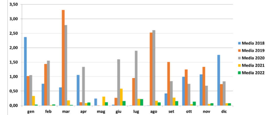
Concentrazione polveri mg/Nm3 camino E314b
