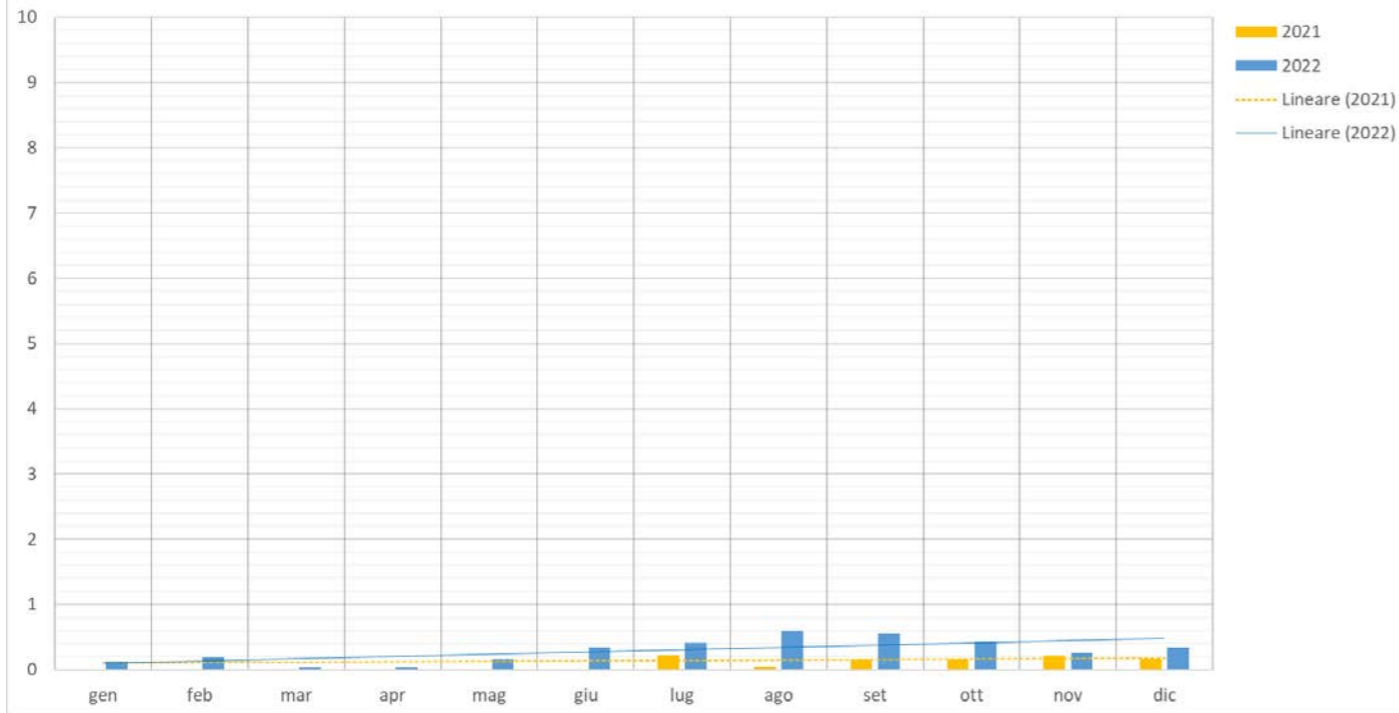
Concentrazione Polveri (mg/Nm3, medie mensili) camino E437 cokeria ANNI 2021-2022
