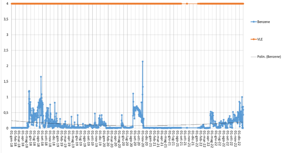
Concentrazione Benzene (mg/Nm3, media giornaliera) camino E428 ANNI 2018-2019-2020-2021-2022
