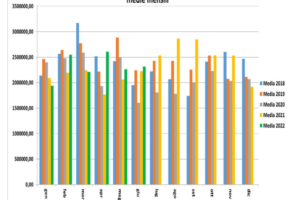
Portata fumi (Nm3/h) camino E312 medie mensili
