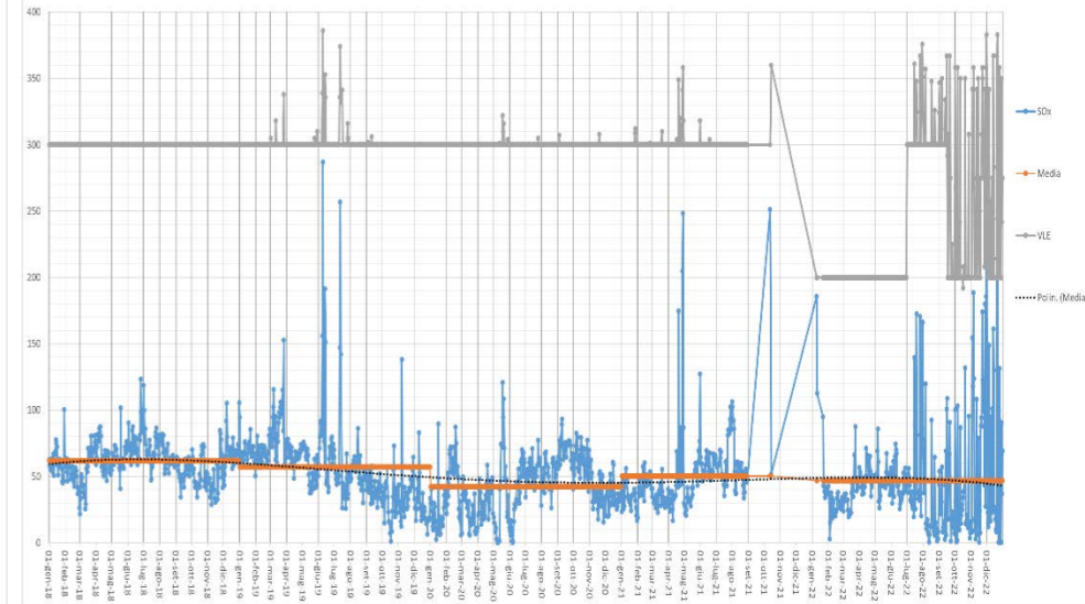
Concentrazione SOx (mg/Nm3, media giornaliera) camino E428 - ANNO 2018 - 2019 - 2020-2021-2022
