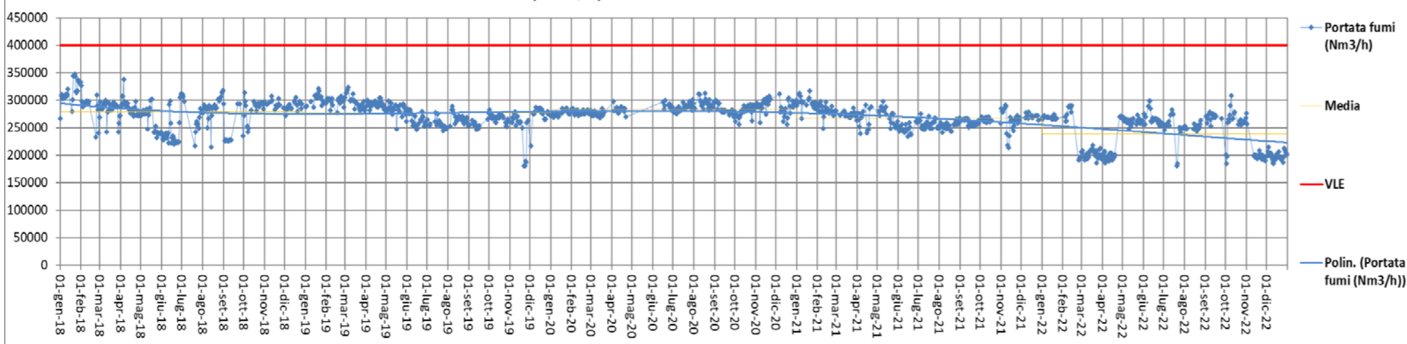
Portata fumi (Nm3/h) camino E324 - Anni 2018-2019-2020-2021-2022
