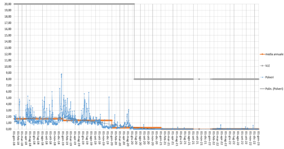
Concentrazione polveri (mg/Nm3, media giornaliera) camino E428 ANNO 2018-2019-2020-2021-2022
