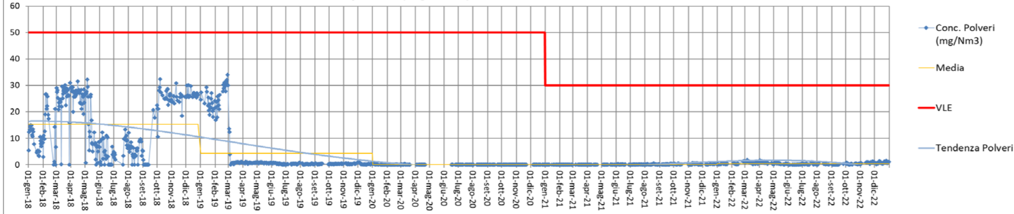
Concentrazione polveri (mg/Nm3) camino E324 - Anni 2018-2019-2020-2021-2022
