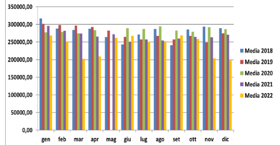
Portata fumi (Nm3/h)camino E324 medie mensili
