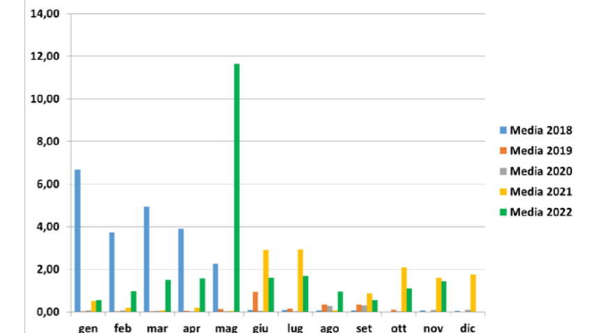
Concentrazione SOx (mg/Nm3) camino E325 medie mensili
