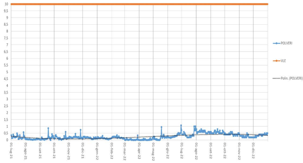
Concentrazione polveri (mg/Nm3, media giornaliera) camino E437 ANNO 2021-2022
