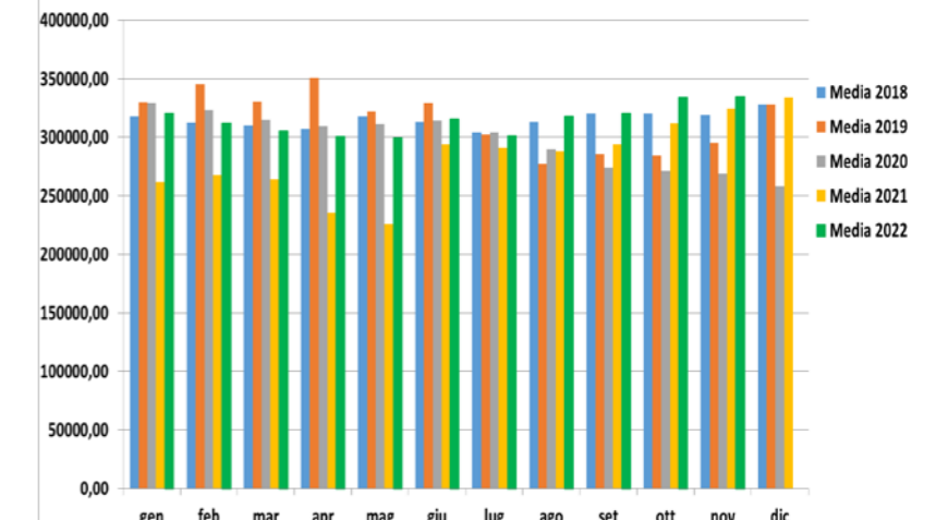
Portata fumi (Nm3/h) camino E325 medie mensili
