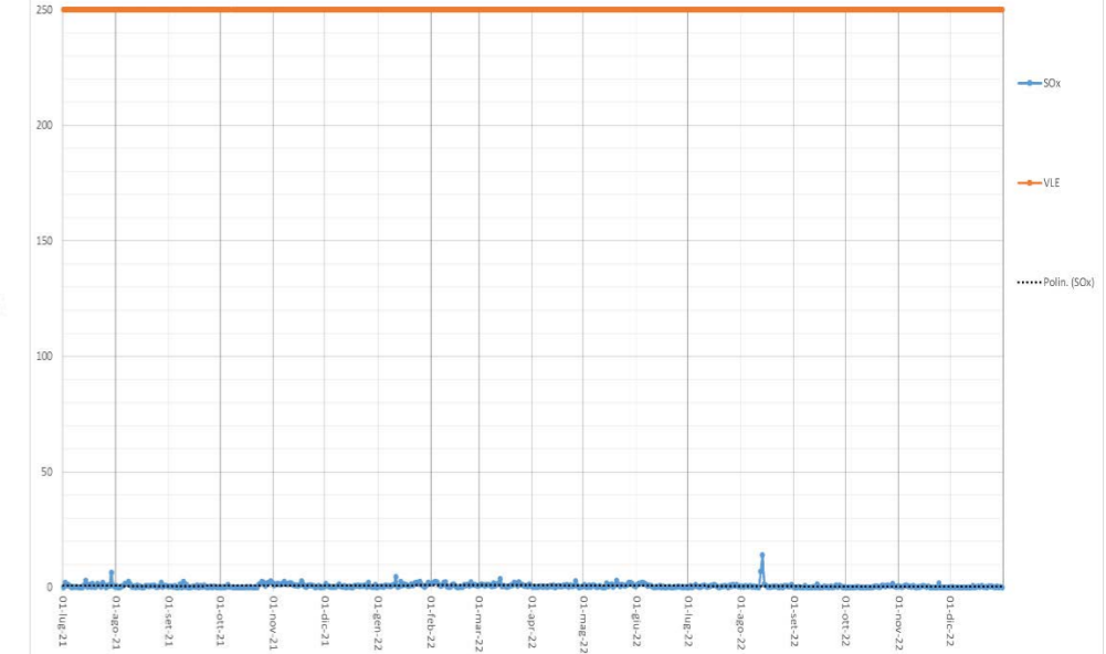
Concentrazione SOx (mg/Nm3, media giornaliera) camino E437 ANNO 2021-2022
