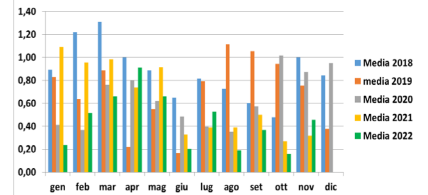
Concentrazione polveri (mg/Nm3) camino E325 medie mensili
