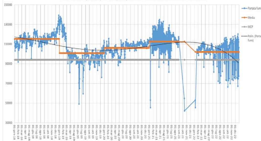
Portata fumi (Nm3/h) camino(E428) cokeria - anno 2018-2019-2020-2021-2022
