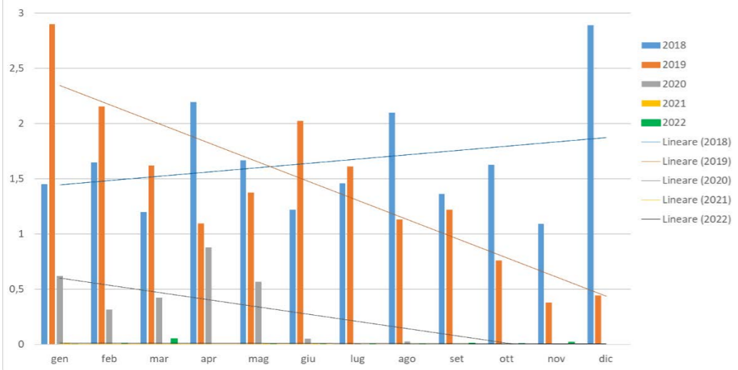
Concentrazione Polveri (mg/Nm3, medie mensili) camino E428 cokeria ANNI 2018-2019-2020-2021-2022
