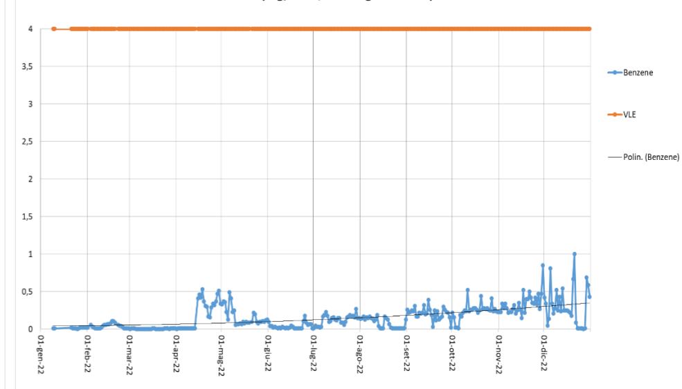
Concentrazione Benzene (mg/Nm3, media giornaliera) camino E428 - ANNO 2022
