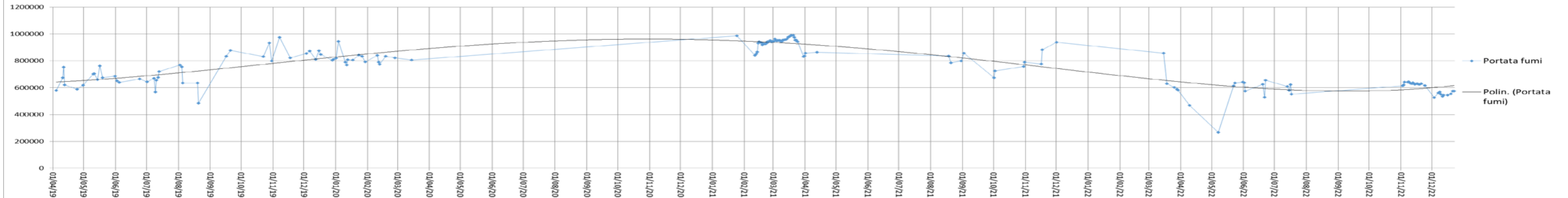
Portata Fumi (Nm3/h) camino E525
