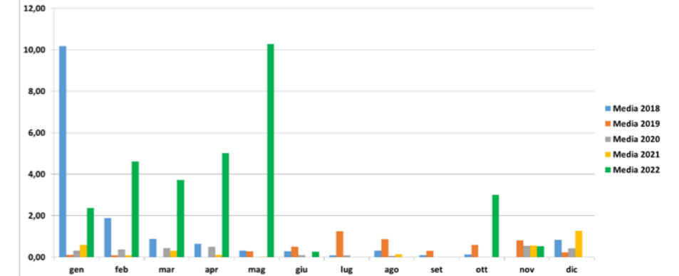
Concentrazione SOx mg/Nm3 camino E314b
