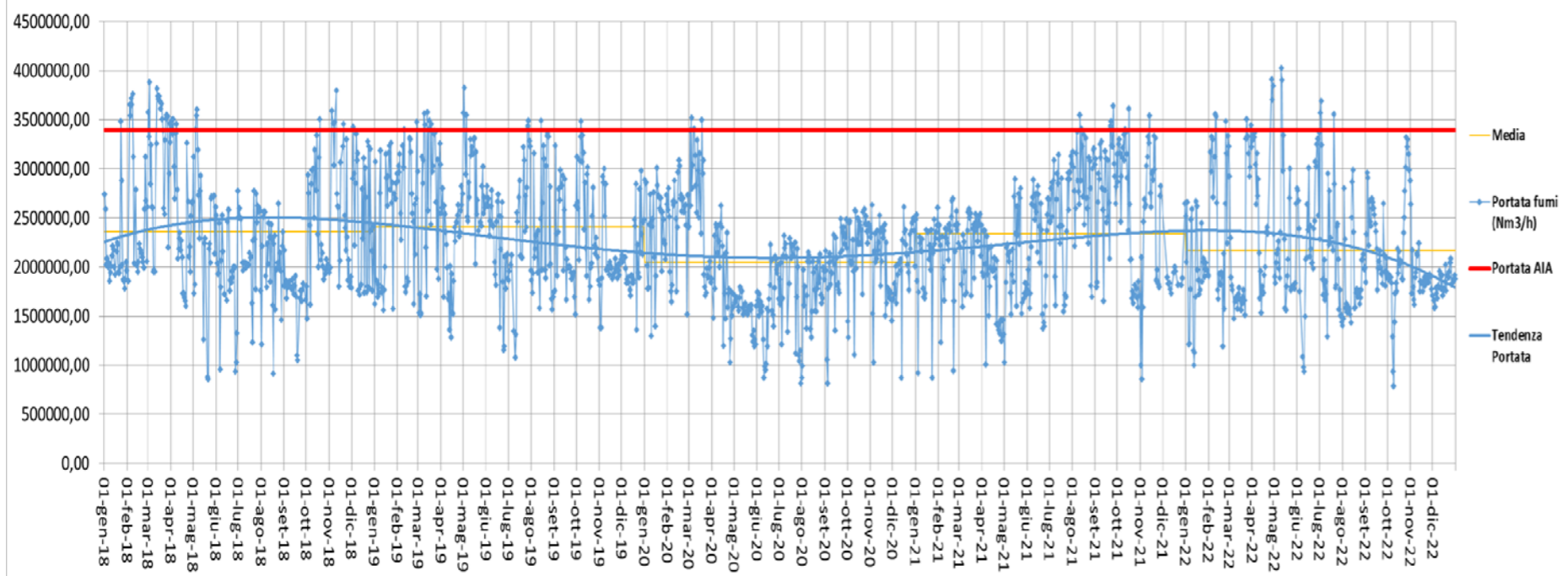
Portata fumi (Nm3/h) - Camino E312 - Anni 2018 - 2019 - 2020 - 2021 - 2022
