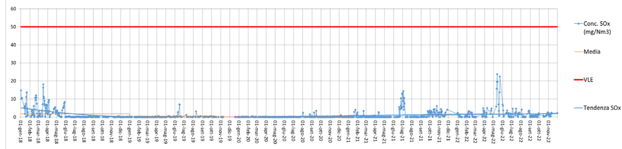
Concentrazione SOx (mg/Nm3) camino E325 - Anni 2018-2019-2020-2021-2022
