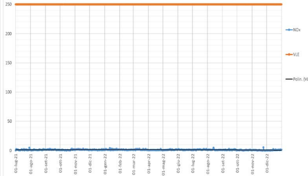
Concentrazione di NOx (mg/Nm3, media giornaliera) camino E437 cokeria ANNO 2021-2022
