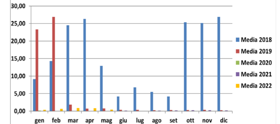
Concentrazione polveri (mg/Nm3) camino E324 medie mensili
