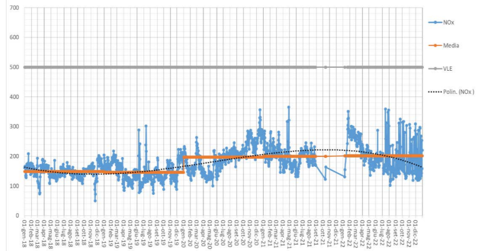
Concentrazione NOx (mg/Nm3, media giornaliera) camino E428 cokeria ANNO 2018-2019-2020-2021-2022
