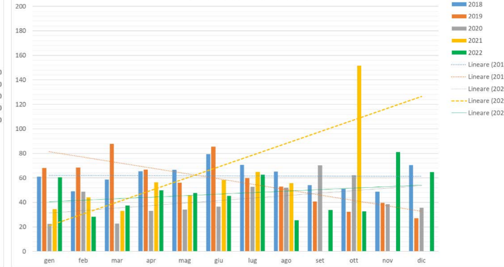
Concentrazione SOx (mg/Nm3, medie mensili) camino E428 cokeria ANNI 2018-2019-2020-2021-2022
