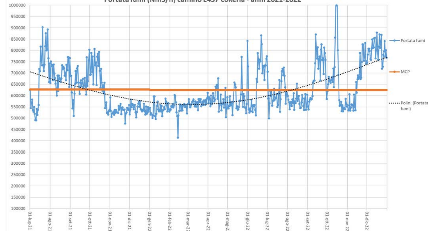
Portata fumi (Nm3/h) camino E437 cokeria - anni 2021-2022
