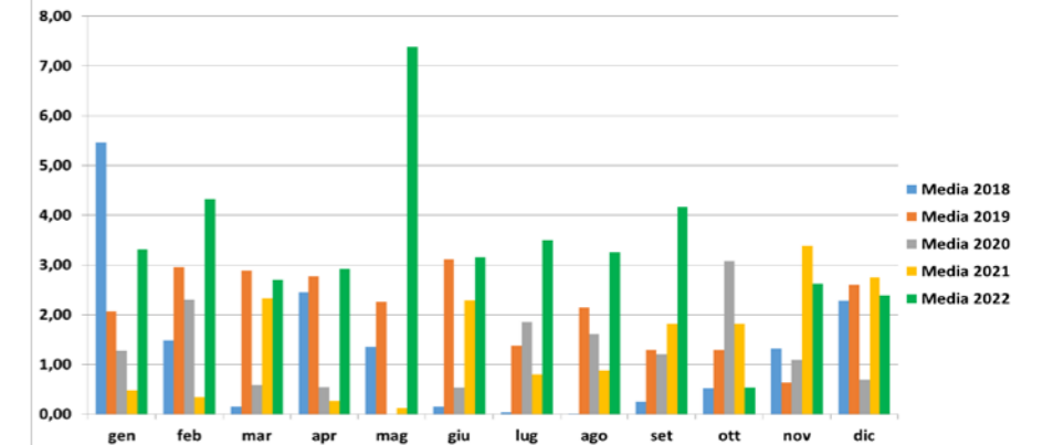
Concentrazione NOx mg/Nm3 camino E314b
