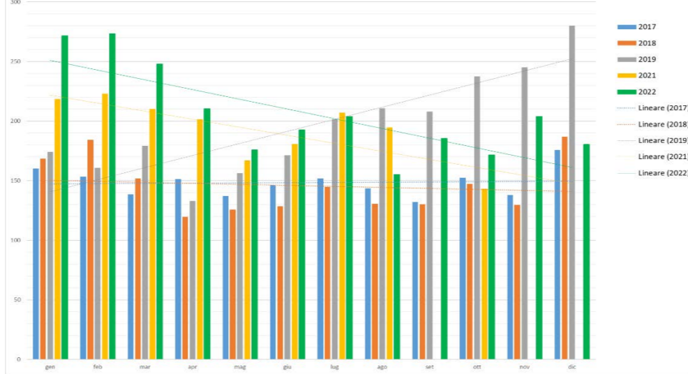
Concentrazione NOx (mg/Nm3, medie mensili) camino E428 cokeria ANNI 2018-2019-2020-2021-2022
