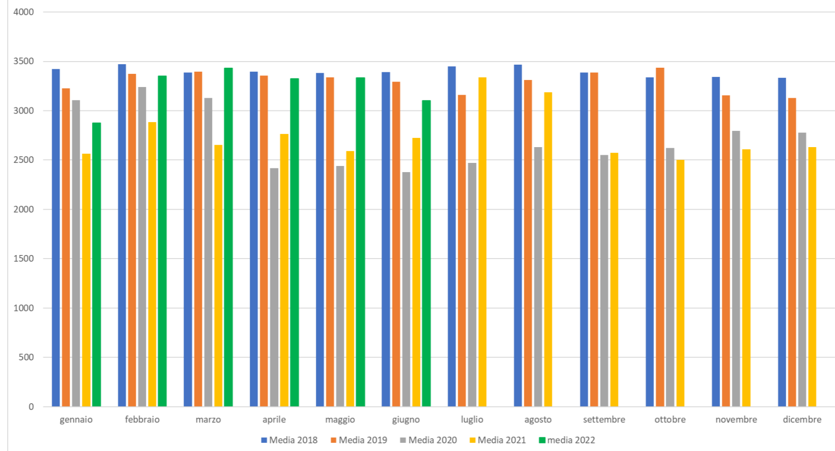
Produzione media mensile cokeria (tonns) anno 2018-2019-2020-2021-2022 (I semestre)
