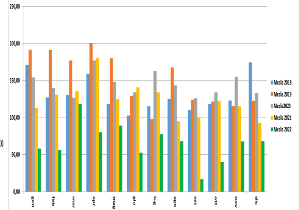
Concentrazione SOx (mg/Nm3) camino E312 medie mensili
