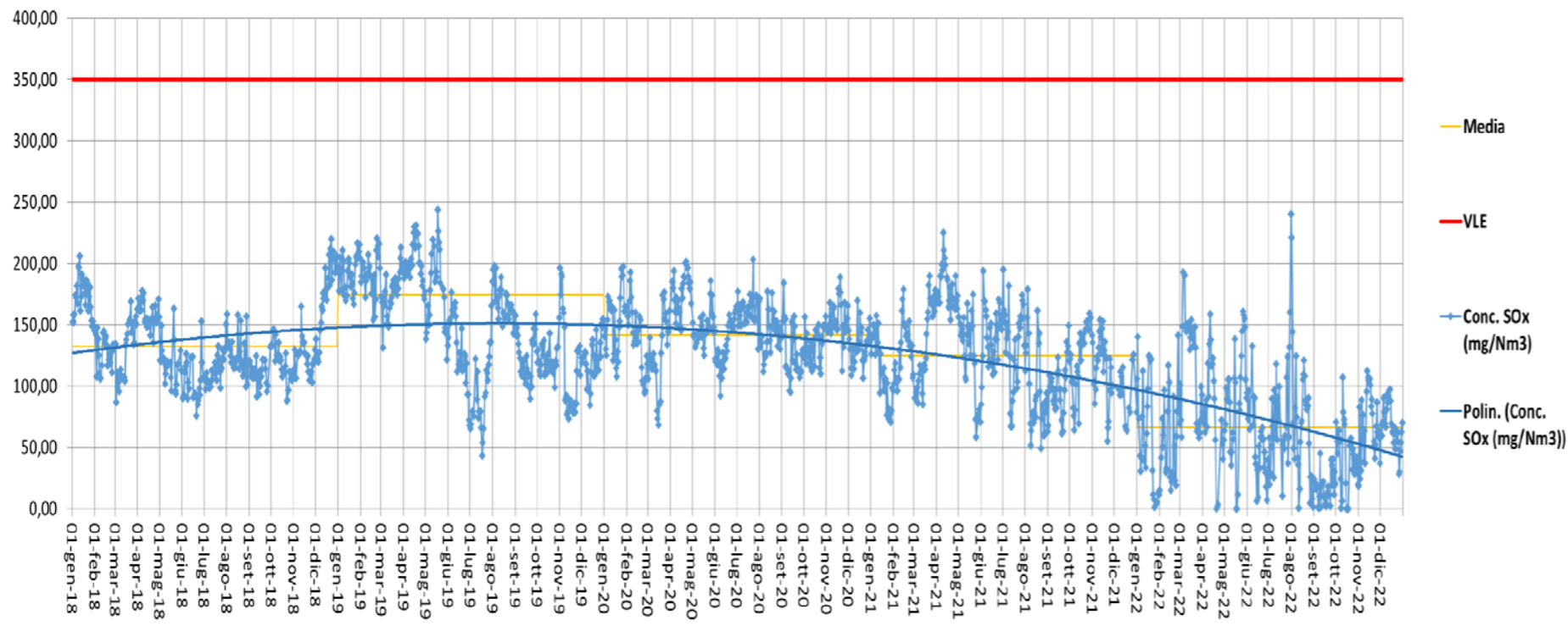
Concentrazione SOx (mg/Nm3) - Camino E312 - Anni 2018 - 2019 - 2020 - 2021 - 2022
