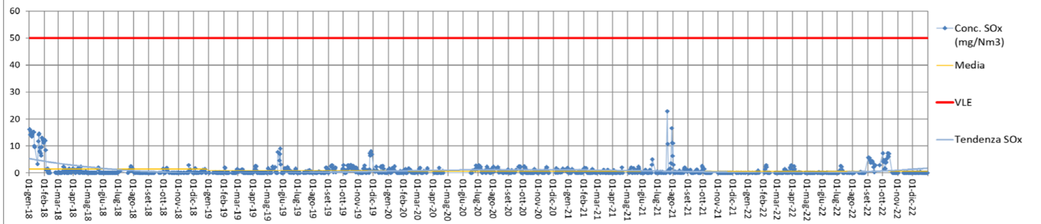
Concentrazione SOx (mg/Nm3) camino E324 - Anni 2018-2019-2020-2021-2022
