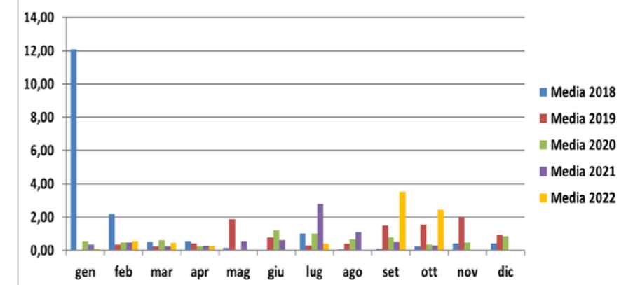
Concentrazione SOx (mg/Nm3) camino E324 medie mensili
