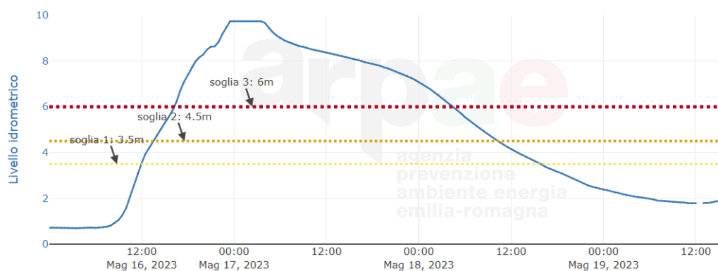
Figura 8 - Idrogramma di piena registrato alla stazione idrometrica di Faenza sul Lamone. FONTE ARPAE Emilia Romagna
