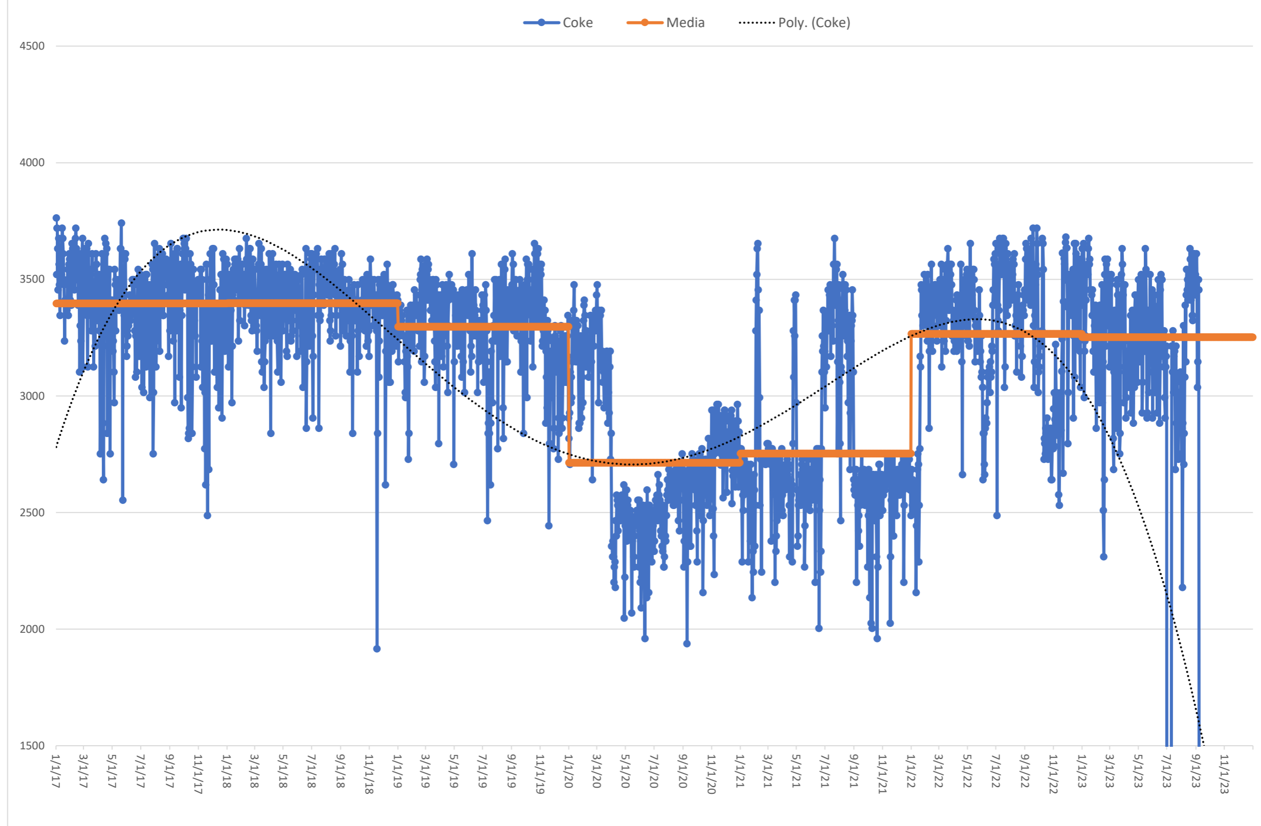
Produzione giornaliera (tonns) cokeria anno anno 2017-2018-2019-2020-2021-2022 -2023)
