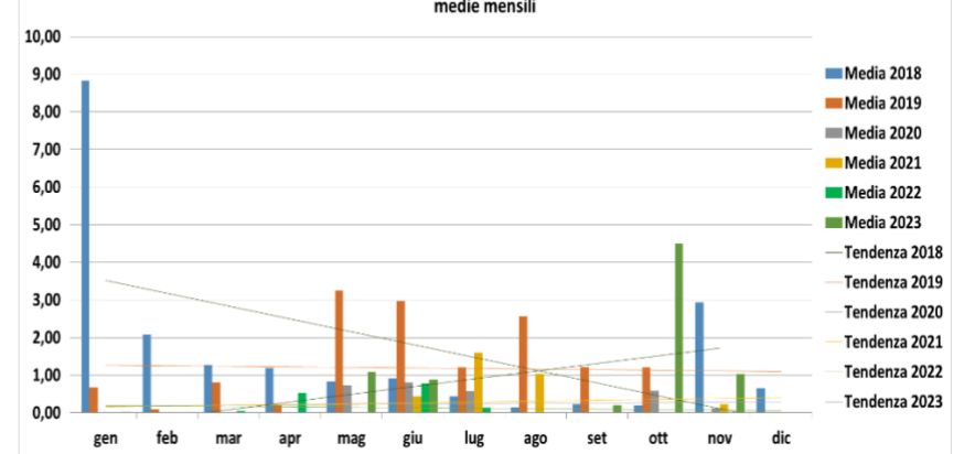
Portata fumi (Nm 3 /h) camino E315b Agglomerato medie mensili
