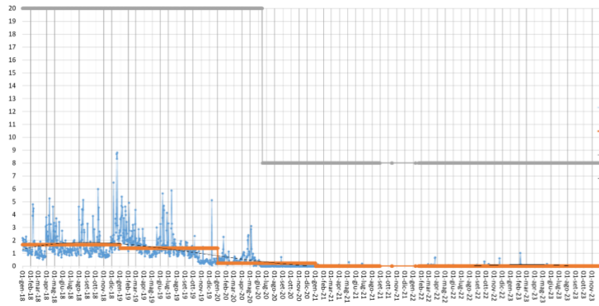
Concentrazione Polveri (mg/Nm3, medie mensili) camino E428 cokeria
