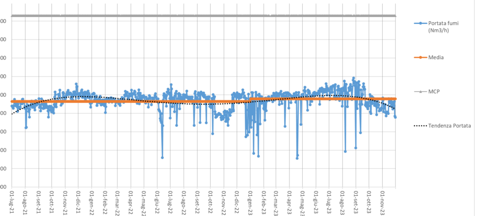
Portata fumi (Nm3/h) camino E425 cokeria
