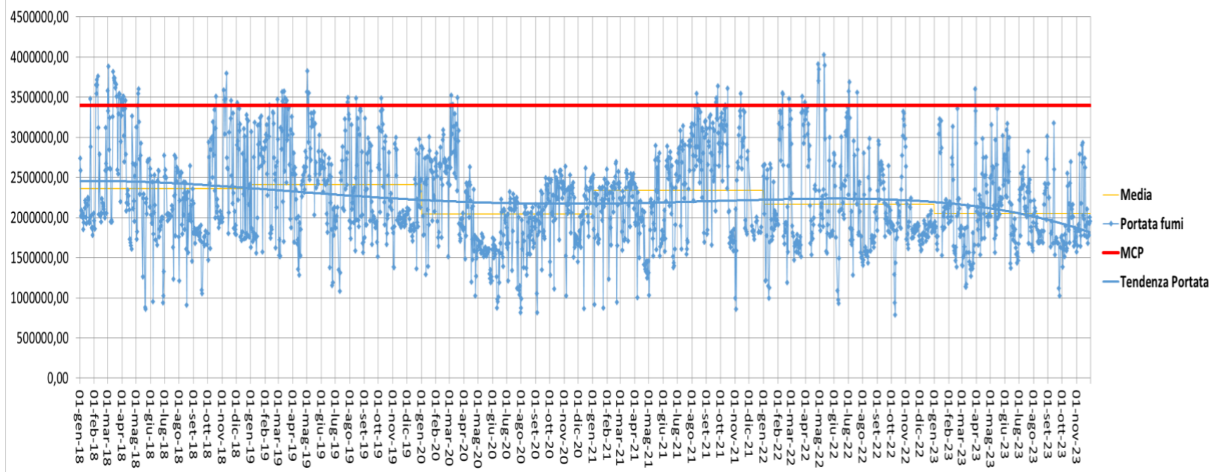
Portata fumi (Nm3/h) - Camino E312 Agglomerato
