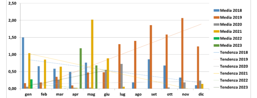
Concentrazione polveri (mg/Nm 3 ) camino E315b Agglomerato medie mensili
