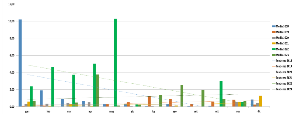
Concentrazione SOx mg/Nm3 camino E314b Agglomerato medie mensili
