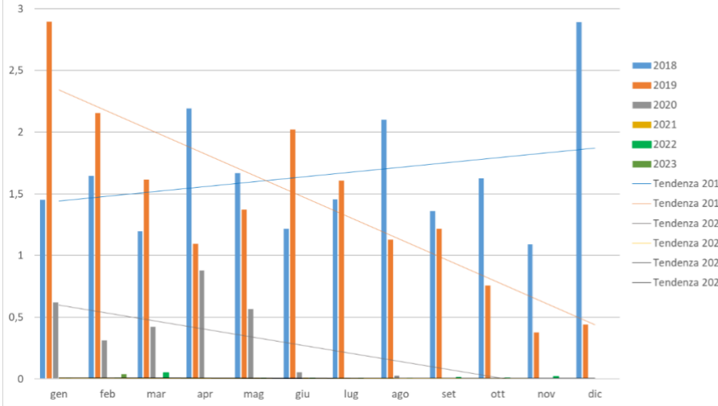
Concentrazione Polveri (mg/Nm3, medie mensili) camino E428 cokeria
