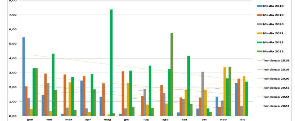
Concentrazione NOx mg/Nm3 camino E314b Agglomerato medie mensili
