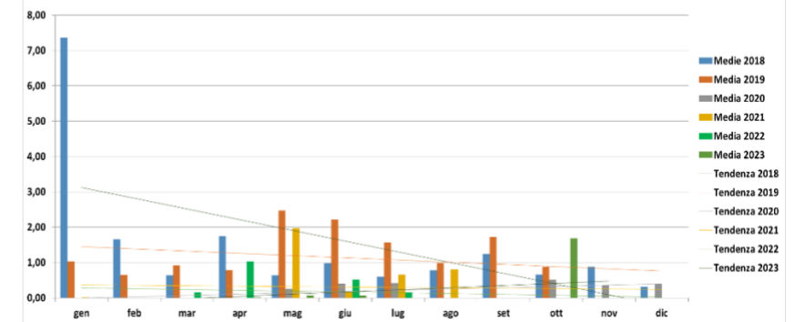
Concentrazione SOx (mg/Nm 3 ) camino E315b Agglomerato medie mensili
