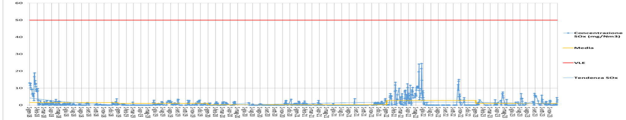
Concentrazione SOx (mg/Nm3) camino E314b Agglomerato
