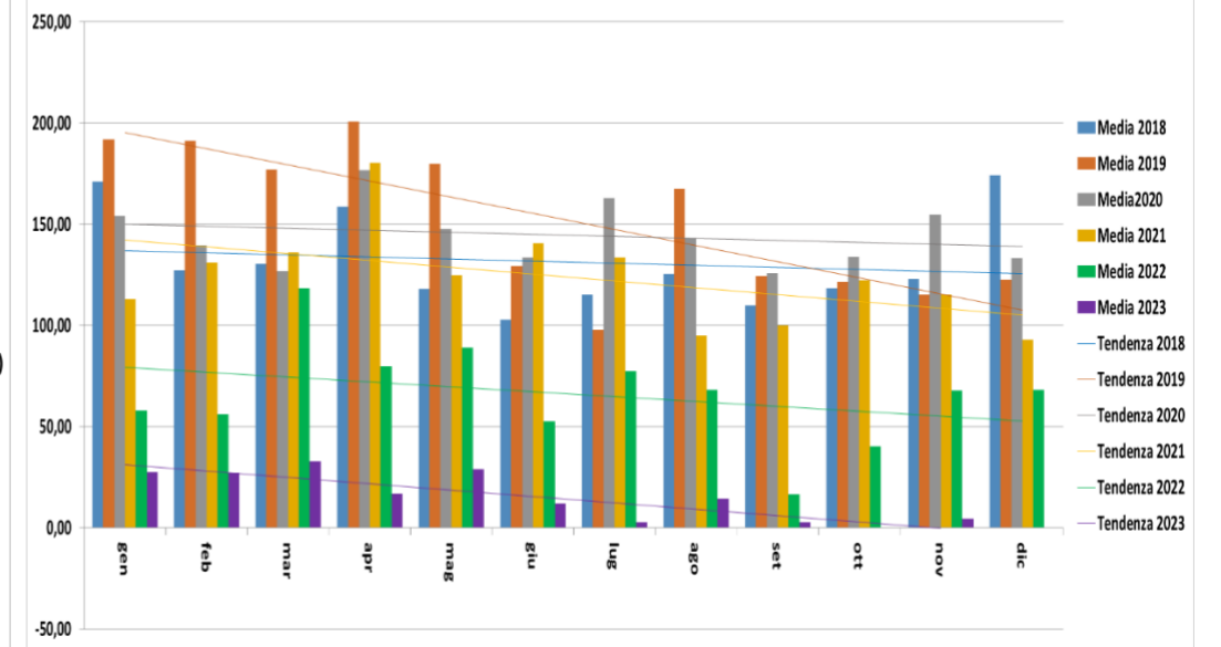
Concentrazione SOx (mg/Nm3) camino E312 Agglomerato medie mensili
