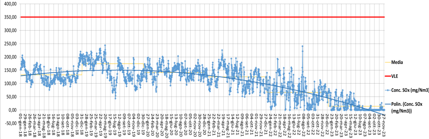
Concentrazione SOx (mg/Nm3) - Camino E312 Agglomerato
