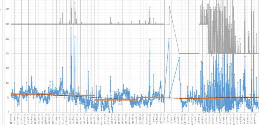
Concentrazione SOx (mg/Nm3, medie mensili) camino E428 cokeria
