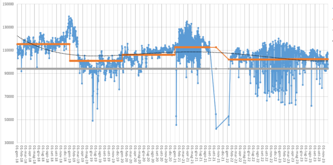
Portata fumi (Nm3/h) camino(E428) cokeria
