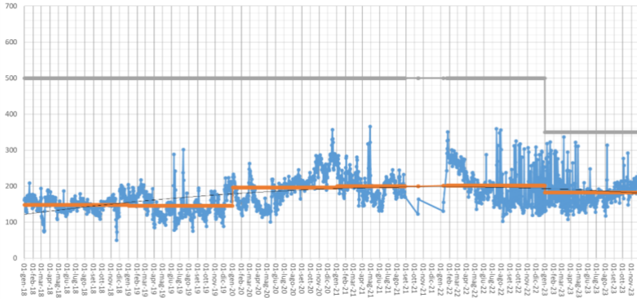
Concentrazione NOx (mg/Nm3, medie mensili) camino E428 cokeria
