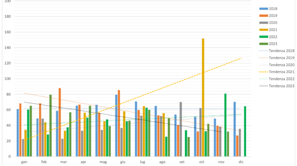
Concentrazione Benzene (mg/Nm3, media giornaliera) camino E428 cokeria
