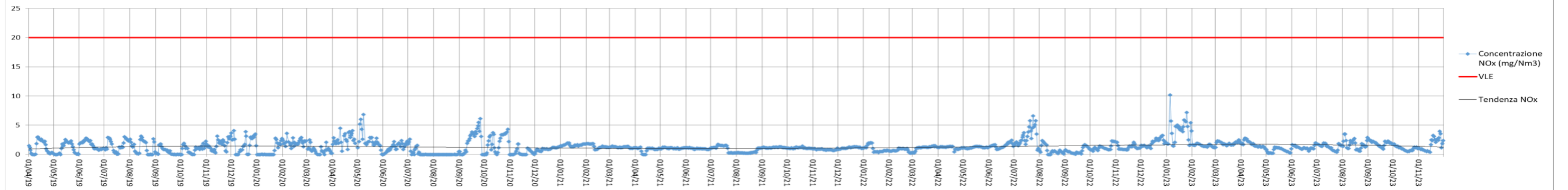
Concentrazione NOx (mg/Nm3) camino E551B
