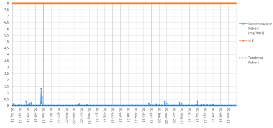
Concentrazione polveri (mg/Nm3, media giornaliera) camino E425 cokeria
