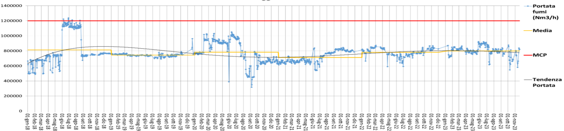
Portata fumi (Nm 3 /h) camino E315b Agglomerato
