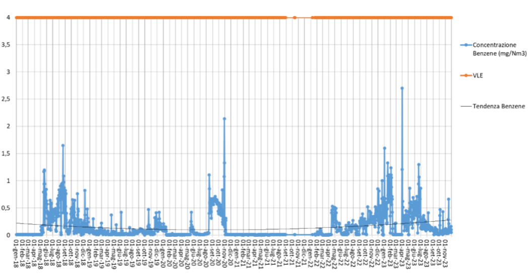
Concentrazione Benzene (mg/Nm3, media giornaliera) camino E428 cokeria
