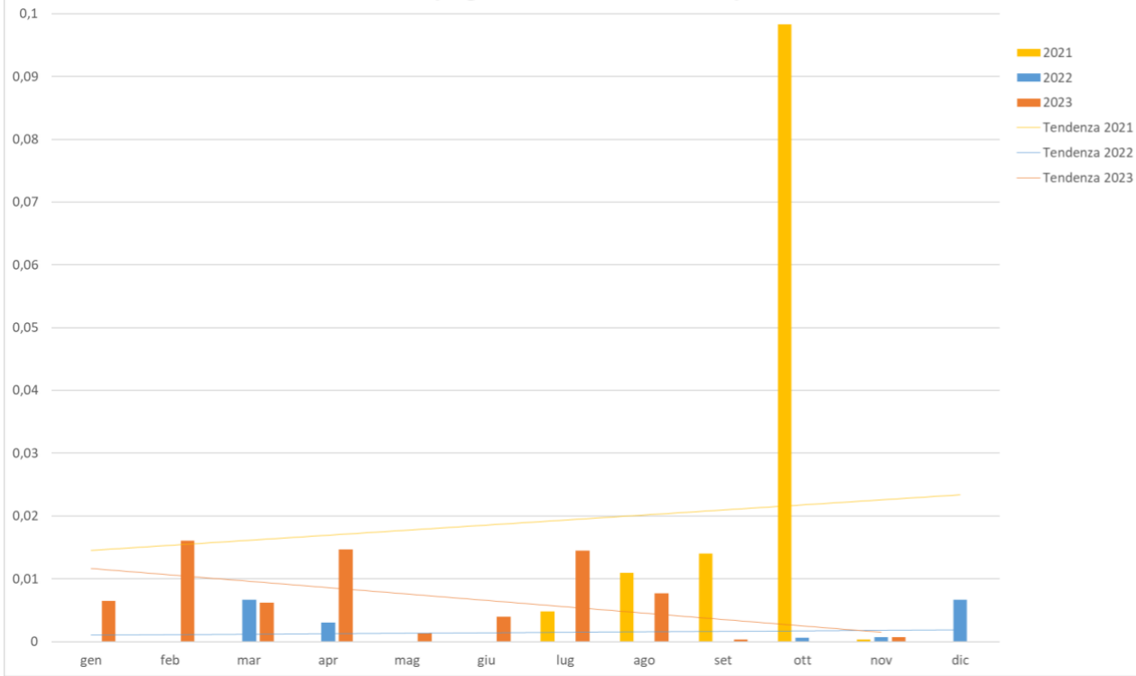
Concentrazione Polveri (mg/Nm3, medie mensili) camino E425 cokeria
