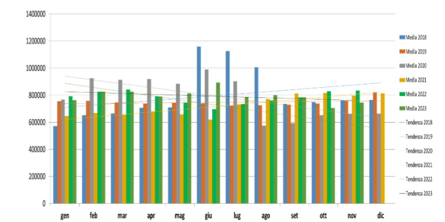
Portata fumi (Nm 3 /h) camino E315b Agglomerato medie mensili
