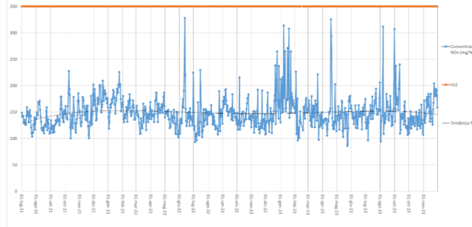
Concentrazione di NOx (mg/Nm3, media giornaliera) camino E425 cokeria
