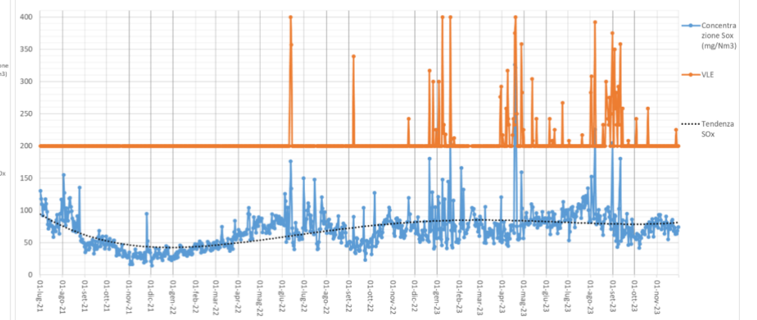
Concentrazione SOx (mg/Nm3, media giornaliera) camino E425 cokeria
