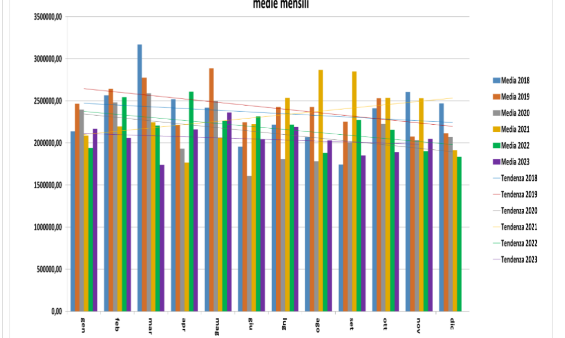
Portata fumi (Nm3/h) camino E312 Agglomerato medie mensili
