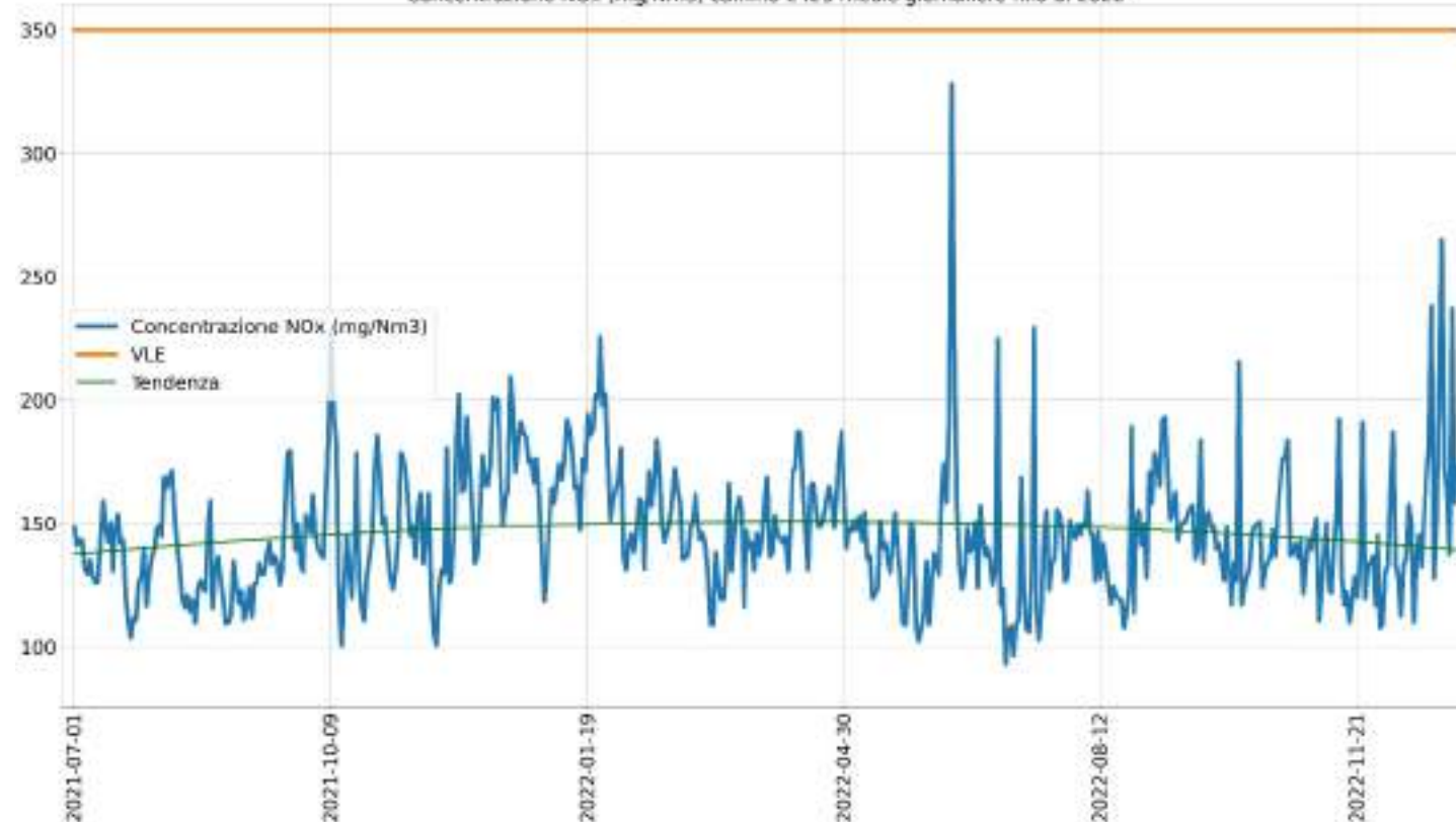
Concentrazione NOx (mg/Nm3) camino E425 medie giornaliere fino al 2022
