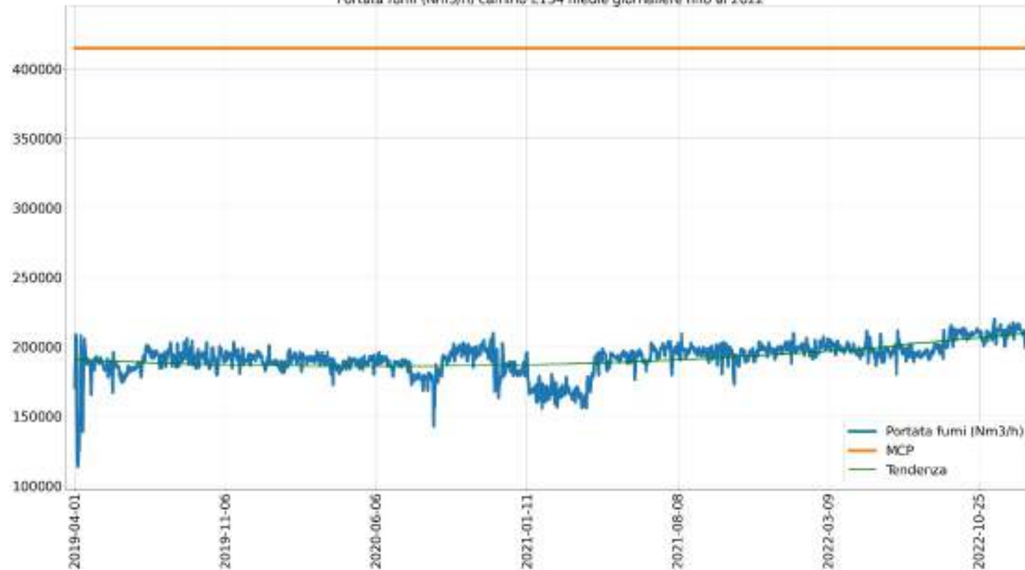
Portata fumi (Nm 3 /h) camino E134 medie giornaliere fino al 2022
