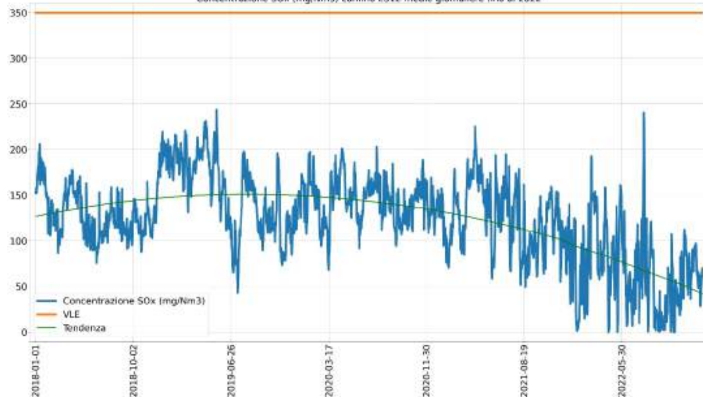
Concentrazione SOx (mg/Nm3) camino E312 medie giornaliere fino al 2022
