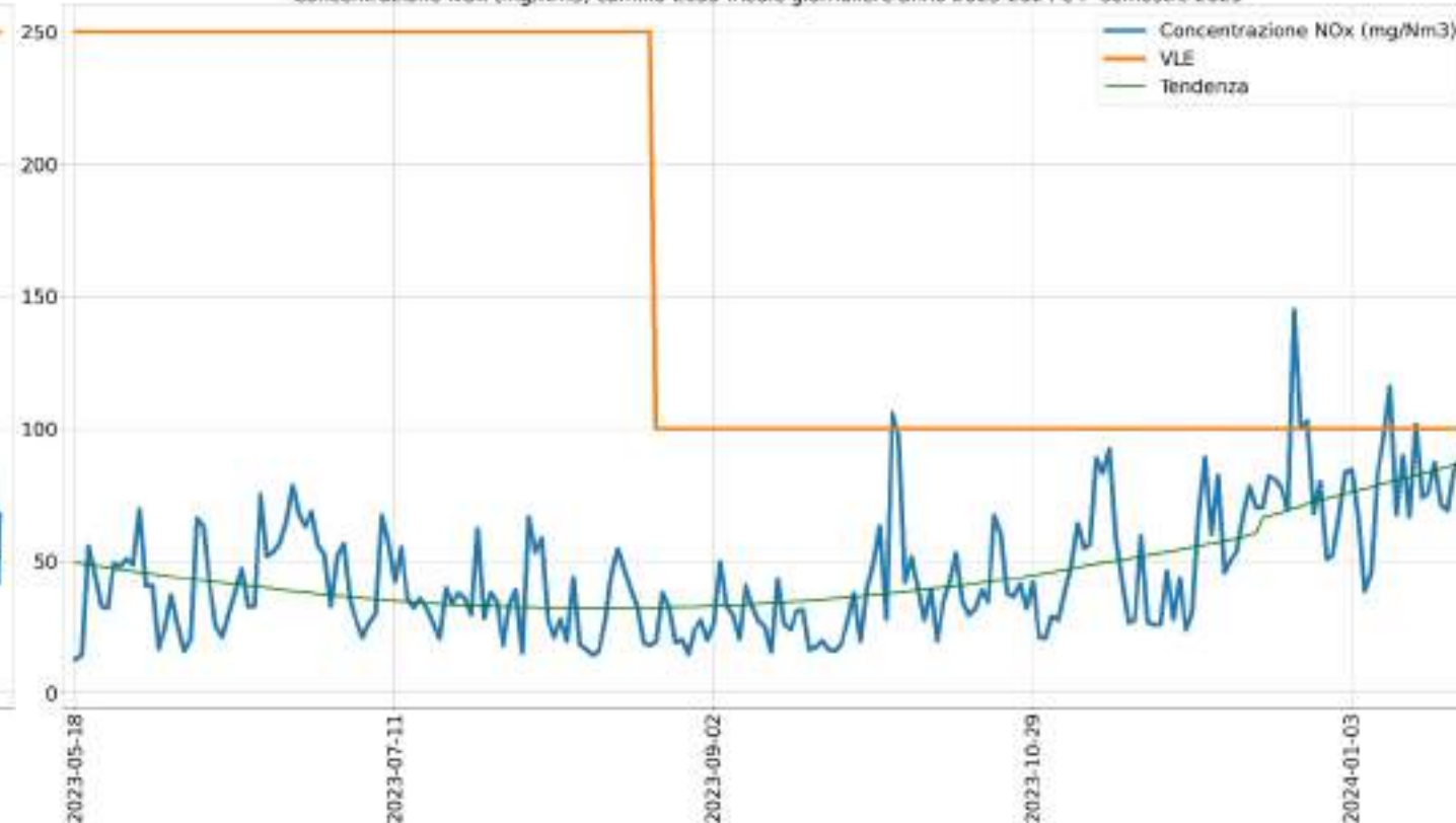
Concentrazione NO x (mg/Nm 3 ) camino E135 medie giornaliere anno 2023-2024 e I° semestre 2025
