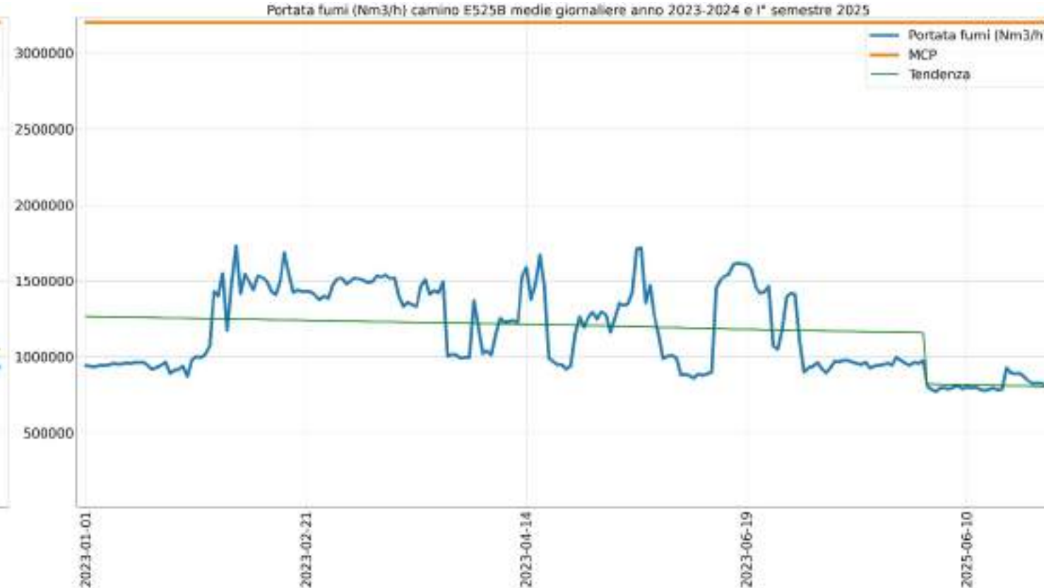
Portata fumi (Nm3/h) camino E525B medie giornaliere anno 2023-2024 e I° semestre 2025
