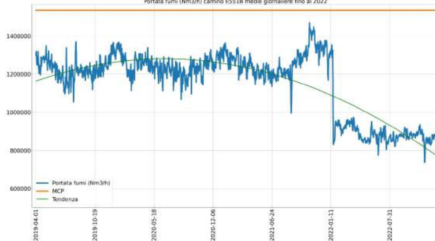
Portata fumi (Nm3/h) camino E551B medie giornaliere fino al 2022
