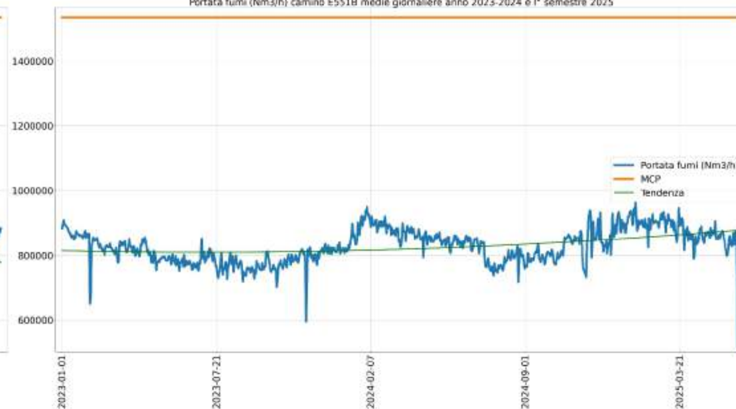
Portata fumi (Nm3/h) camino E551B medie giornaliere anno 2023-2024 e I° semestre 2025
