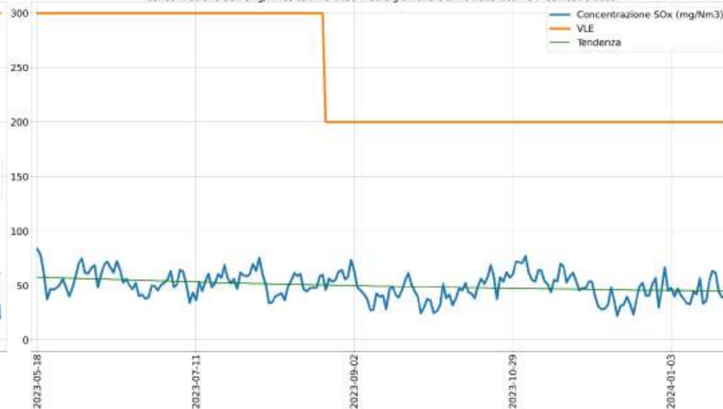
Concentrazione SO x (mg/Nm 3 ) camino E135 medie giornaliere anno 2023-2024 e I° semestre 2025
