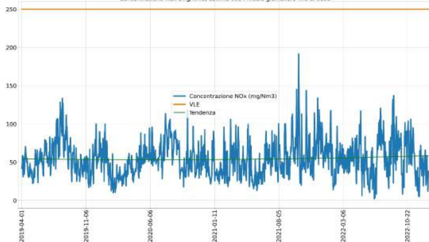
Concentrazione NOx (mg/Nm3) camino E134 medie giornaliere fino al 2022
