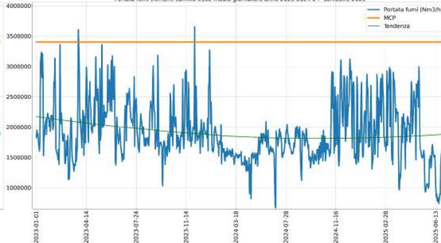
Portata fumi (Nm3/h) camino E312 medie giornaliere anno 2023-2024 e I° semestre 2025
