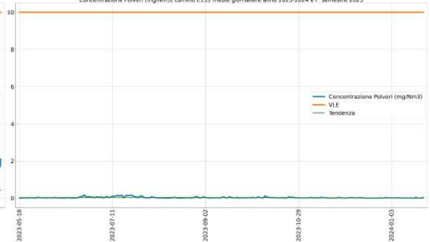
Concentrazione Polveri (mg/Nm 3 ) camino E135 medie giornaliere anno 2023-2024 e 1° semestre 2025
