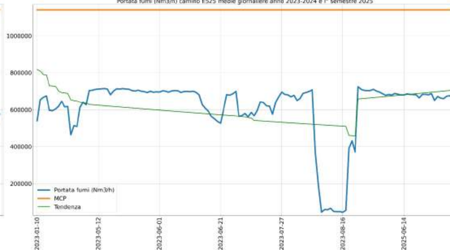
Portata fumi (Nm 3 /h) camino E525 medie giornaliere anno 2023-2024 e 1° semestre 2025
