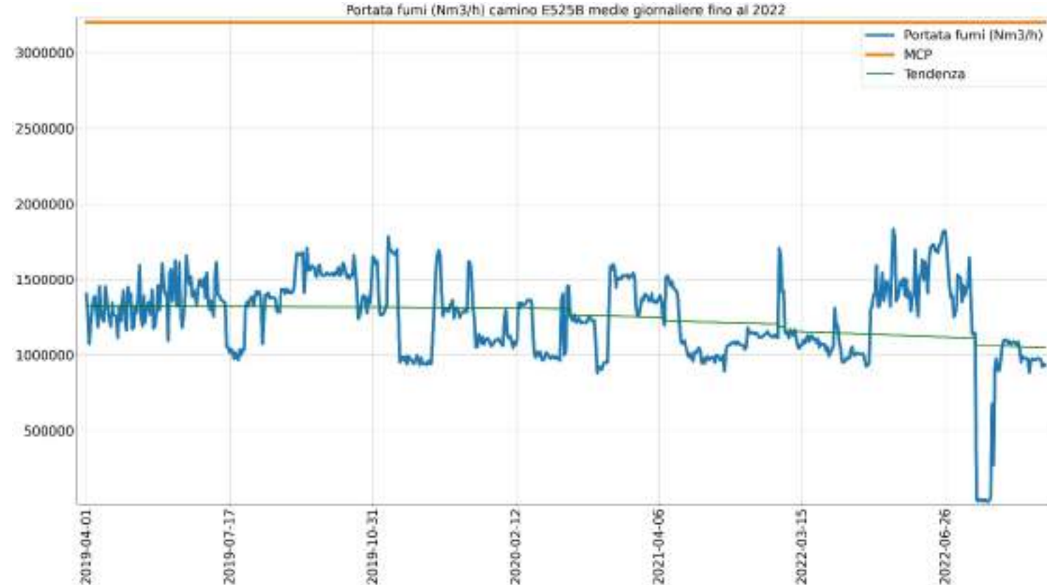
Portata fumi (Nm3/h) camino E525B medie giornaliere fino al 2022
