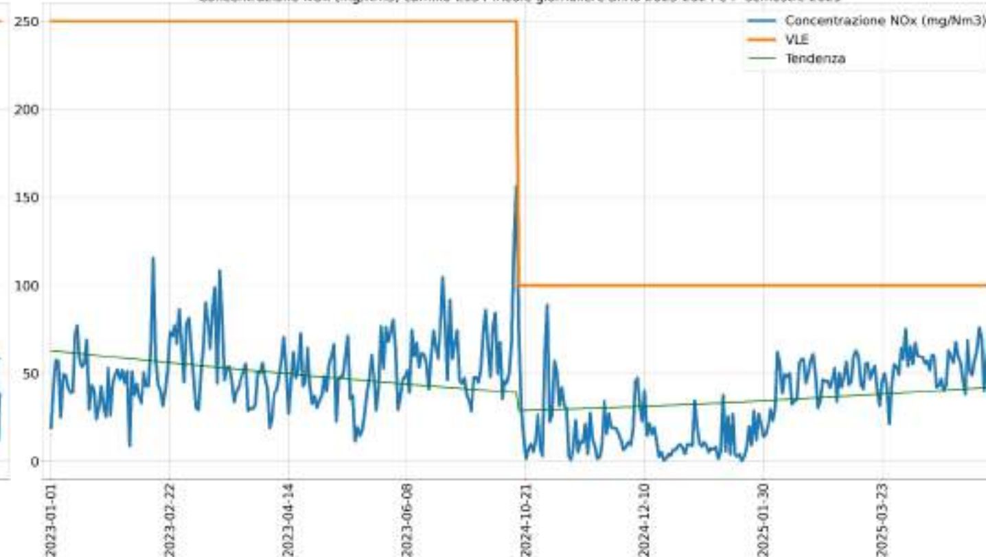
Concentrazione NOx (mg/Nm3) camino E134 medie giornaliere anno 2023-2024 e I° semestre 2025
