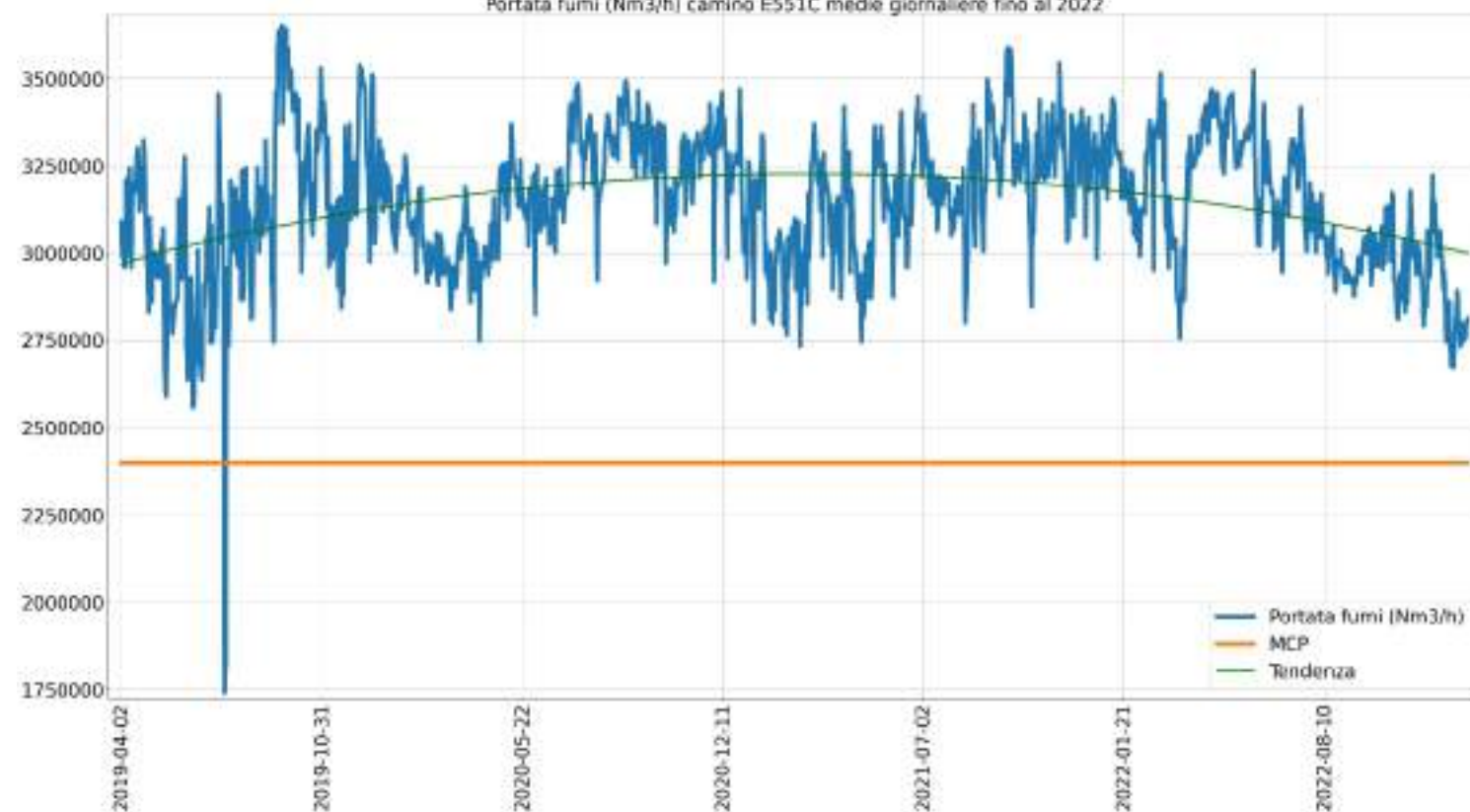
Portata fumi (Nm 3 /h) camino E551C medie giornaliere fino al 2022
