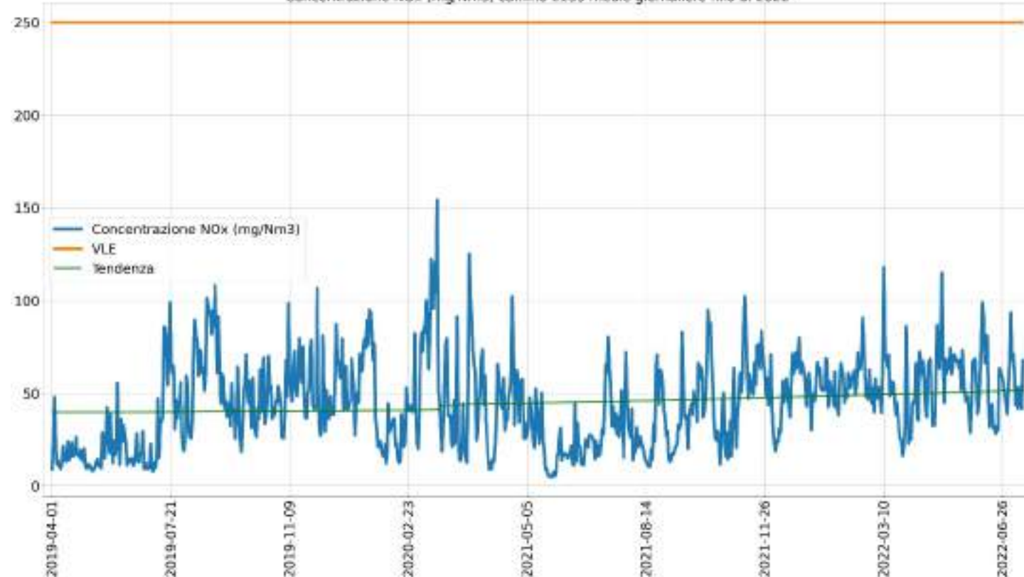
Concentrazione NO x (mg/Nm 3 ) camino E135 medie giornaliere fino al 2022
