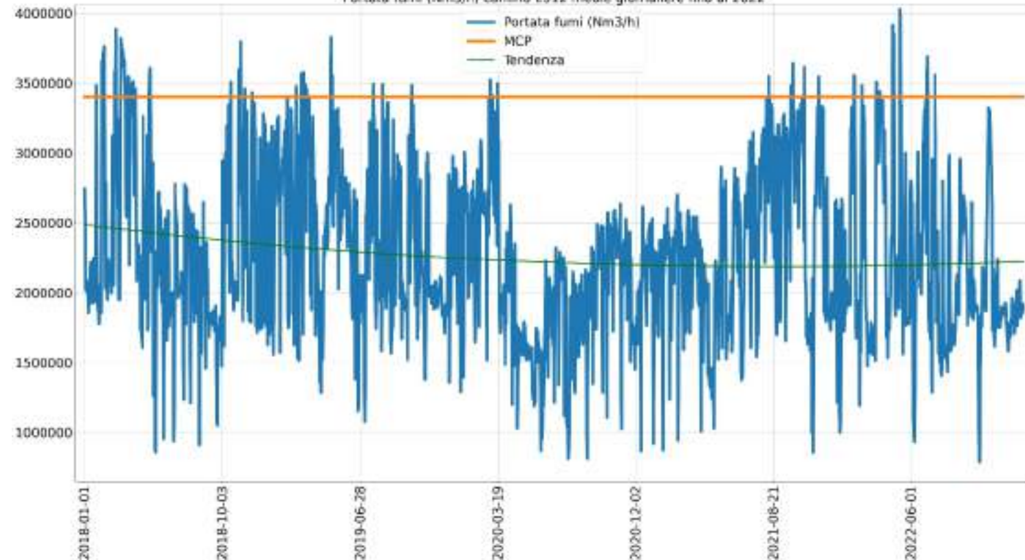
Portata fumi (Nm3/h) camino E312 medie giornaliere fino al 2022
