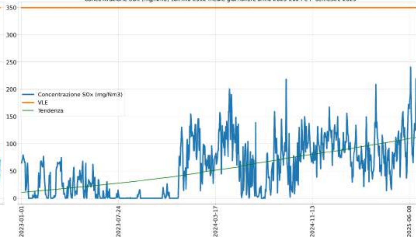
Concentrazione SOx (mg/Nm3) camino E312 medie giornaliere anno 2023-2024 e I° semestre 2025
