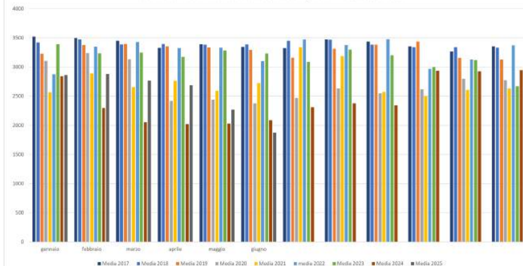
Produzione media mensile cokeria (tonnellate) 2017 - I° semestre 2025
