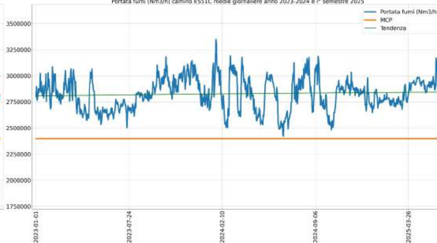
Portata fumi (Nm 3 /h) camino E551C medie giornaliere anno 2023-2024 e 1° semestre 2025
