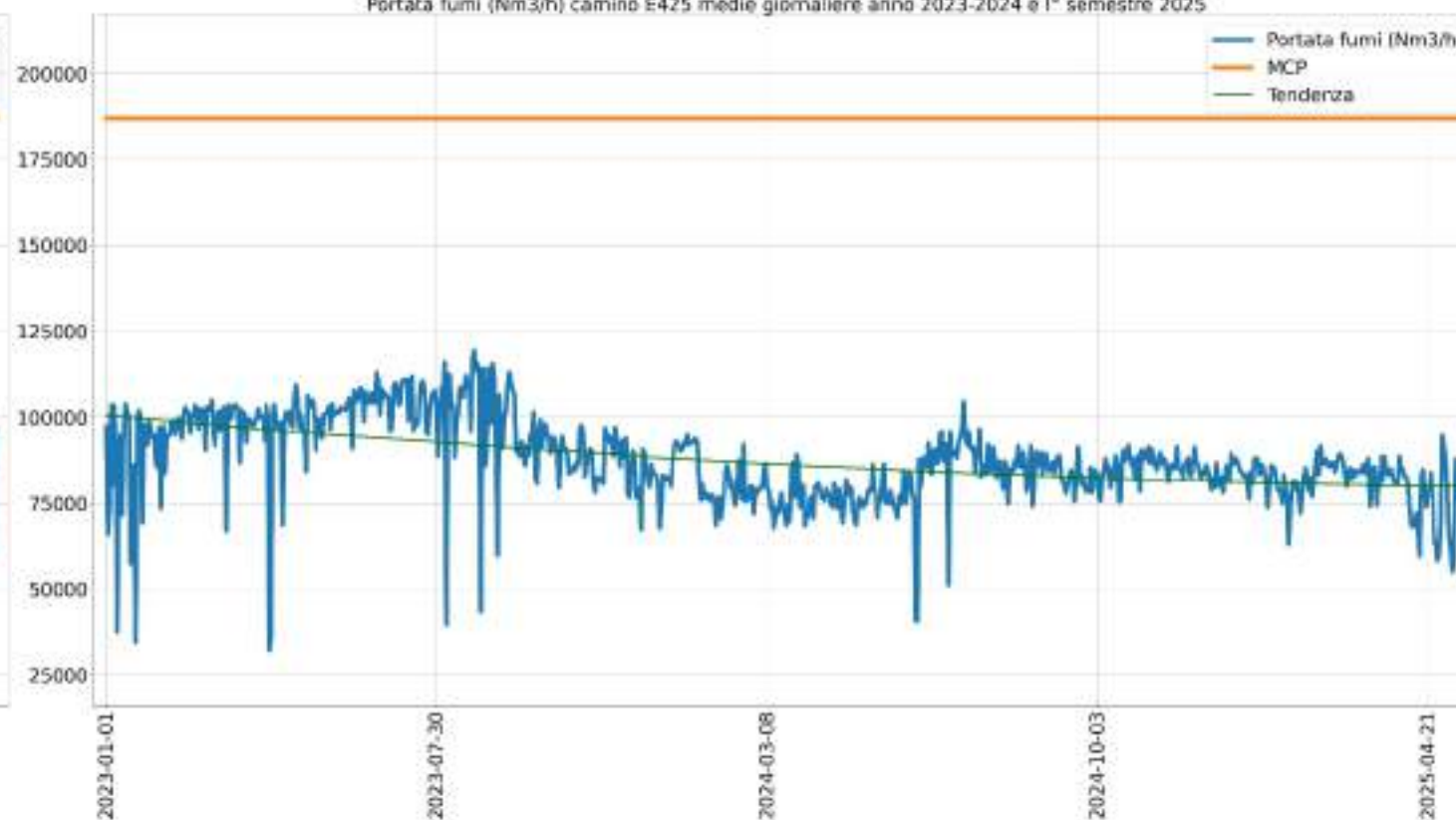
Portata fumi (Nm 3 /h) camino E425 medie giornaliere anno 2023-2024 e I° semestre 2025
