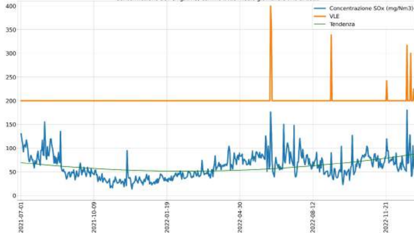
Concentrazione SOx (mg/Nm3) camino E425 medie giornaliere fino al 2022
