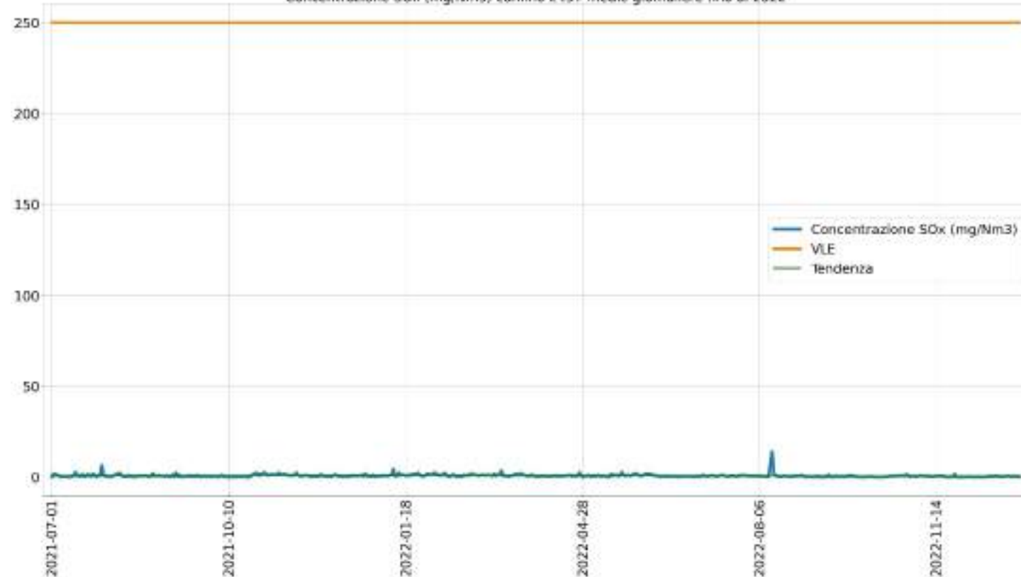
Concentrazione SOx (mg/Nm3) camino E437 medie giornaliere fino al 2022
