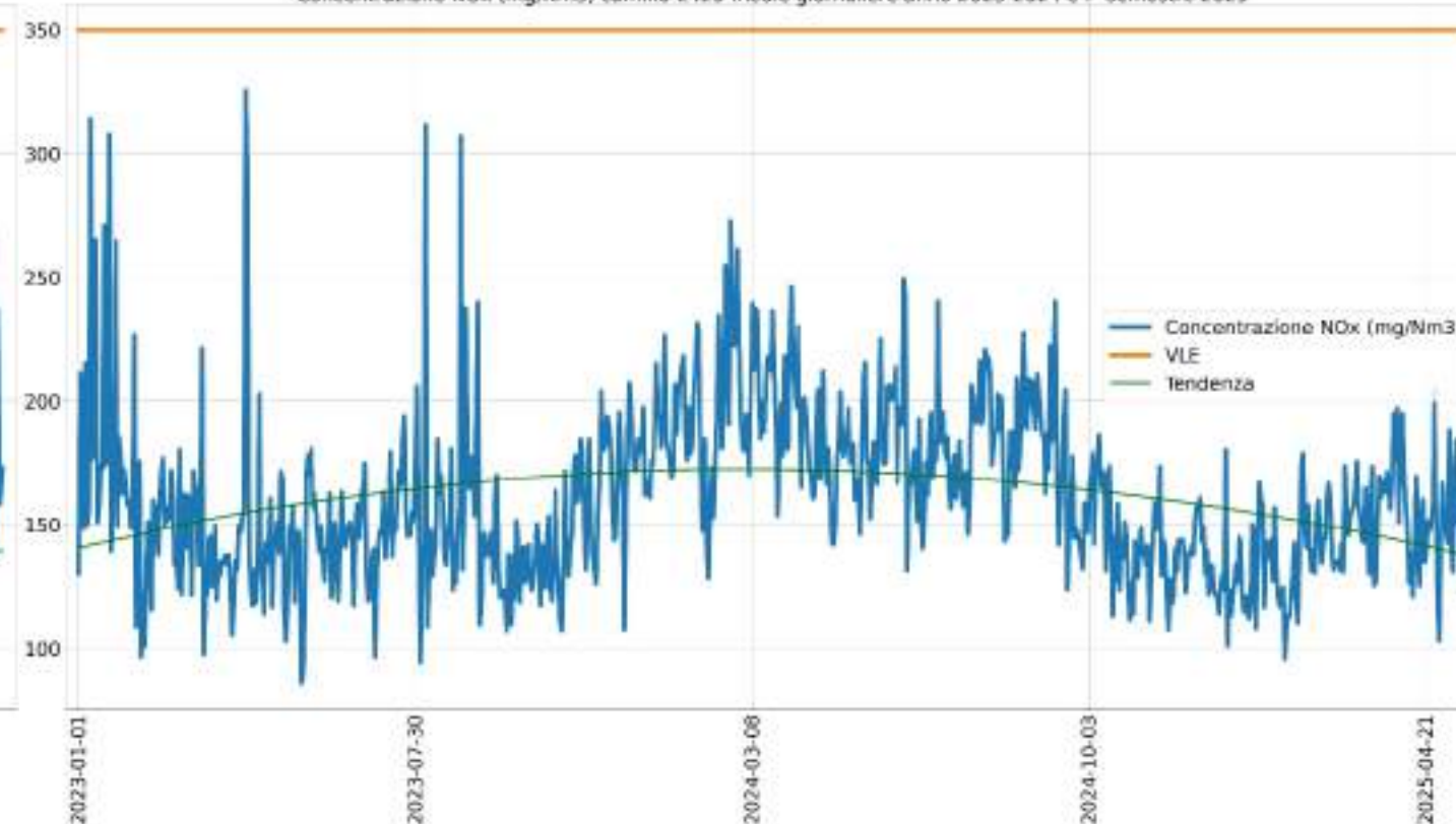
Concentrazione NOx (mg/Nm3) camino E425 medie giornaliere anno 2023-2024 e I° semestre 2025
