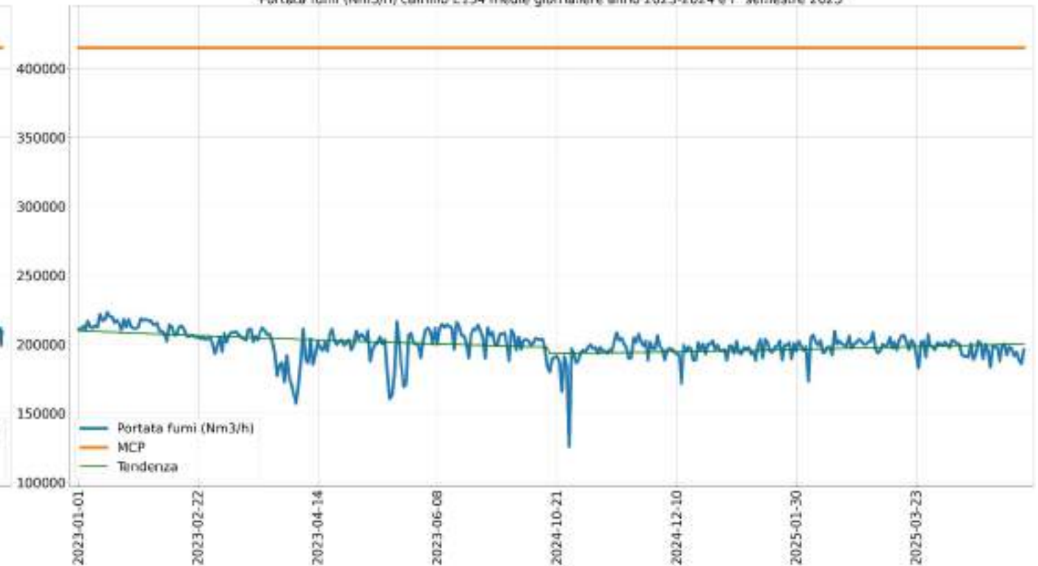
Portata fumi (Nm 3 /h) camino E134 medie giornaliere anno 2023-2024 e 1° semestre 2025
