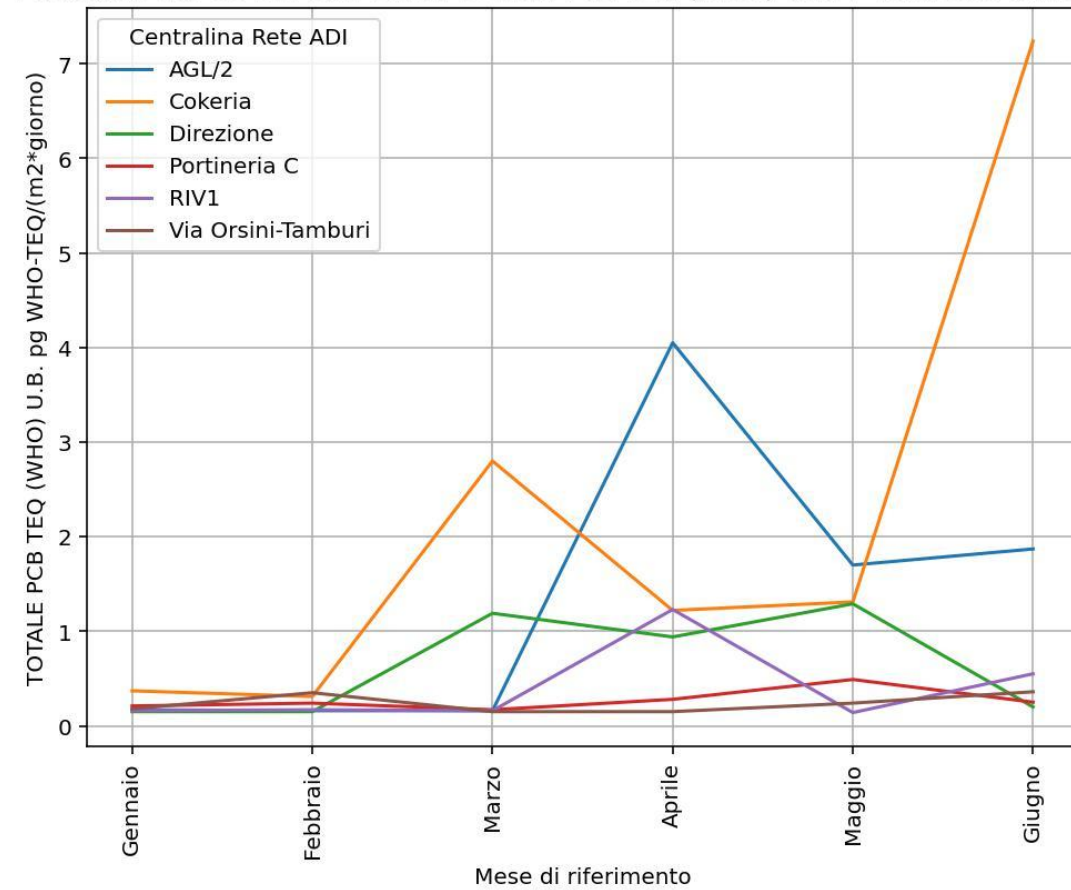
PCBdioxin-like SU DEPOSIMETRI: TOTALE PCB TEQ (WHO) U.B. I° semestre anno 2025
