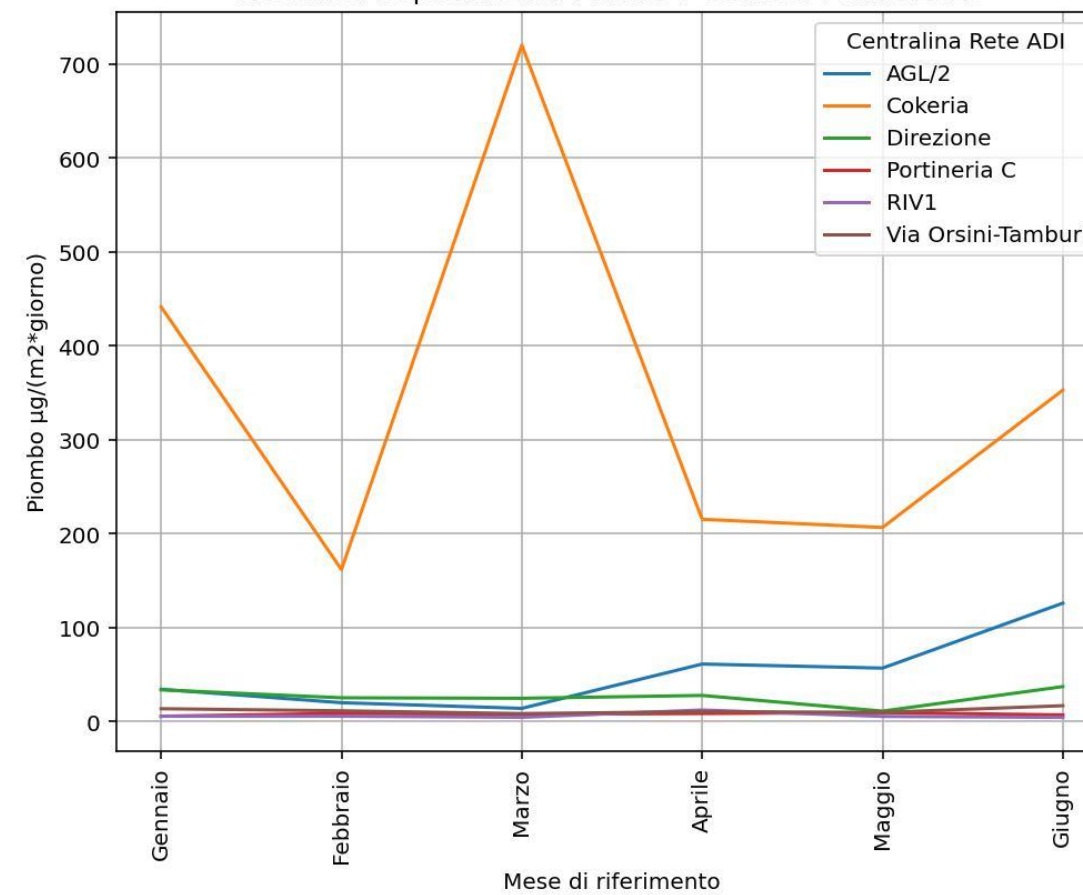
Metalli su Deposimetria: Piombo I° semestre anno 2025
