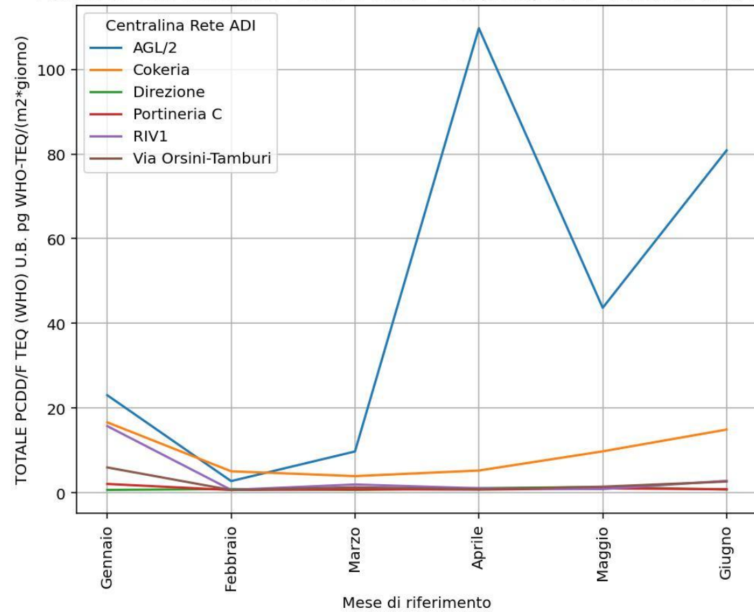
PCDD/F SU DEPOSIMETRI:: TOTALE PCDD/F TEQ (WHO) U.B. I° semestre anno 2025
