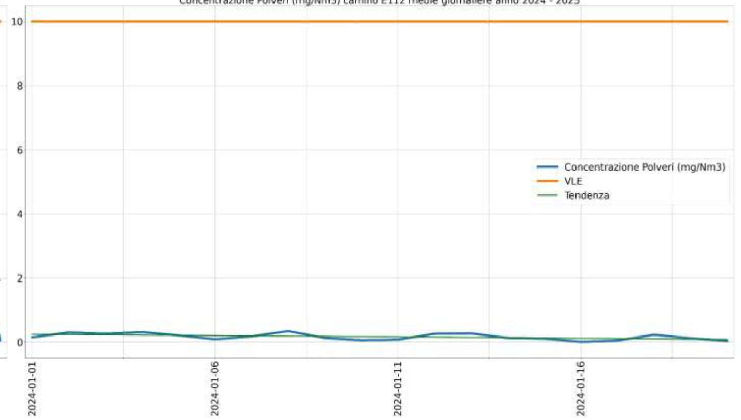
Concentrazione Polveri (mg/Nm 3 ) camino E112 medie giornaliere anno 2024 - 2025
