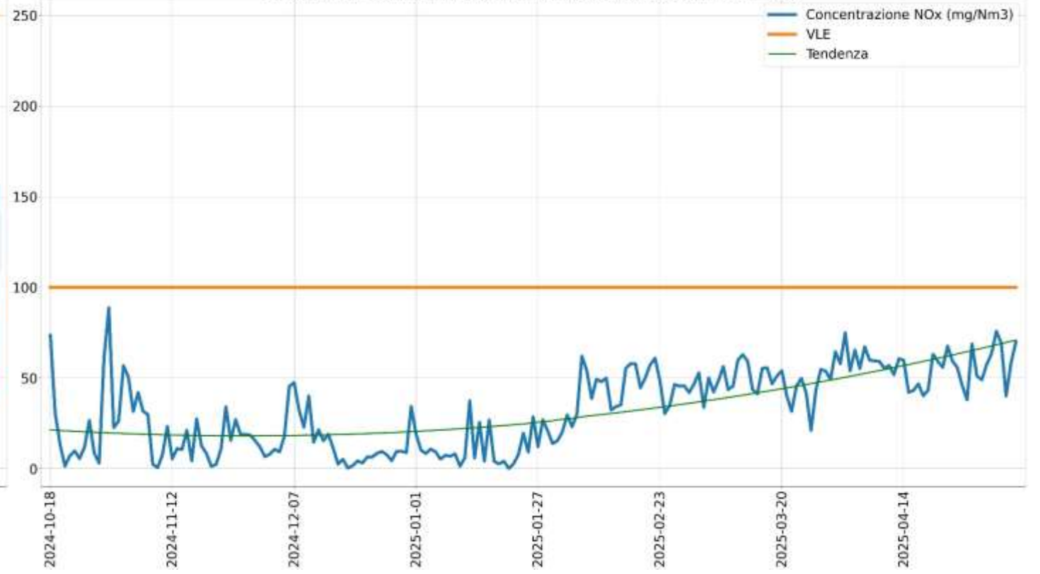
Concentrazione NOx (mg/Nm3) camino E134 medie giornaliere anno 2024 - 2025
