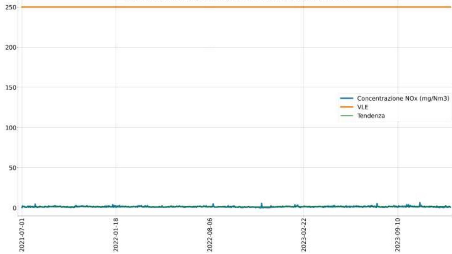
Concentrazione NOx (mg/Nm3) camino E437 medie giornaliere fino al 2023
