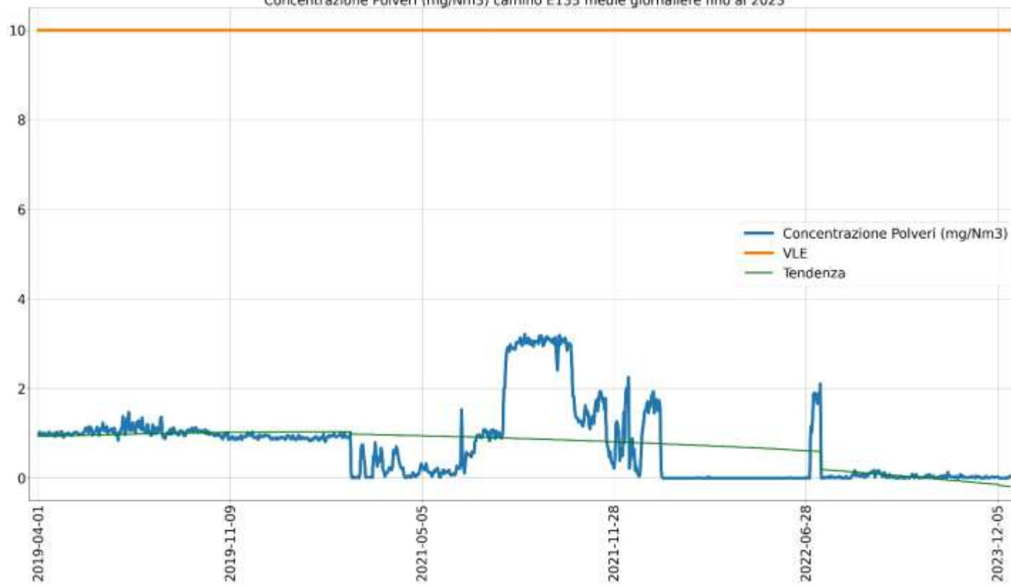
Concentrazione Polveri (mg/Nm 3 ) camino E135 medie giornaliere fino al 2023
