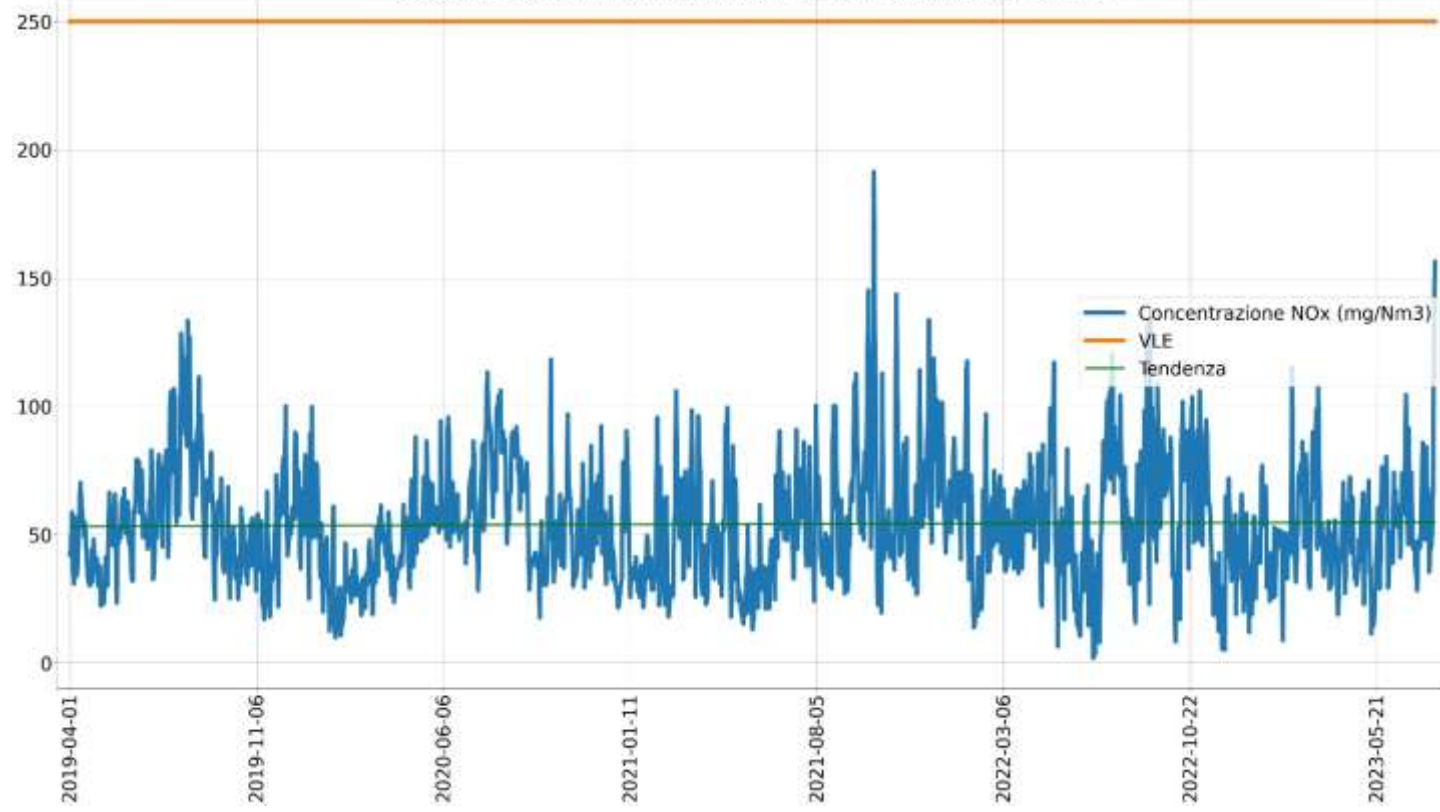
Concentrazione NOx (mg/Nm3) camino E134 medie giornaliere fino al 2023
