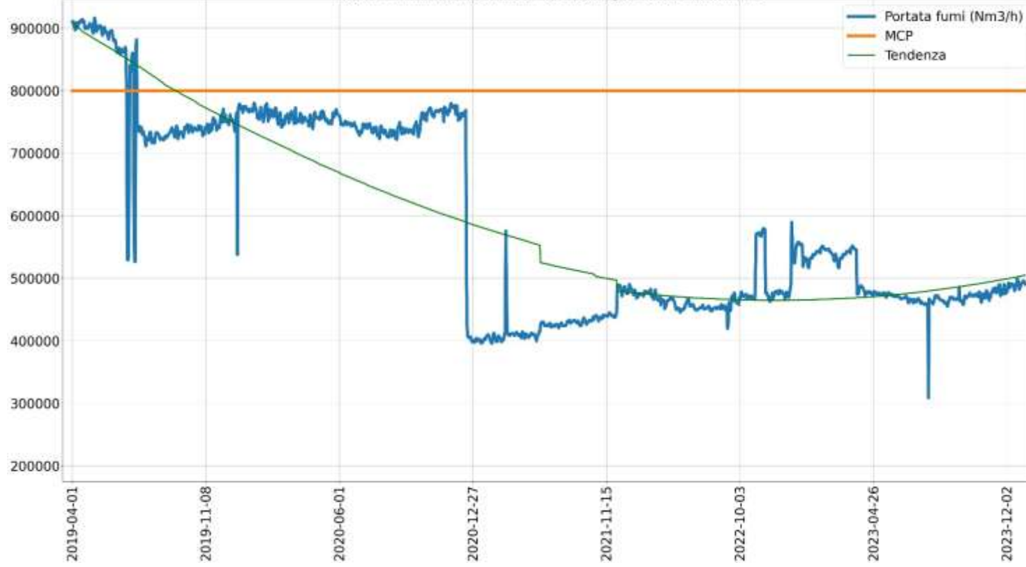
Portata fumi (Nm3/h) camino E109 medie giornaliere fino al 2023
