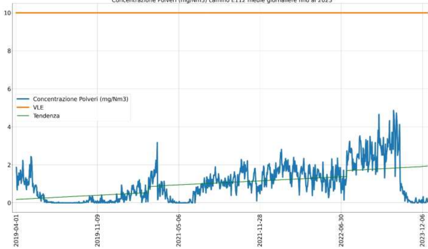
Concentrazione Polveri (mg/Nm 3 ) camino E112 medie giornaliere fino al 2023
