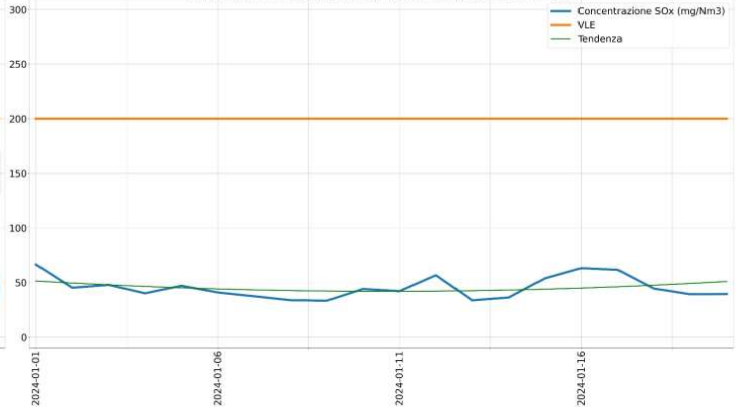
Concentrazione SOx (mg/Nm3) camino E135 medie giornaliere anno 2024 - 2025
