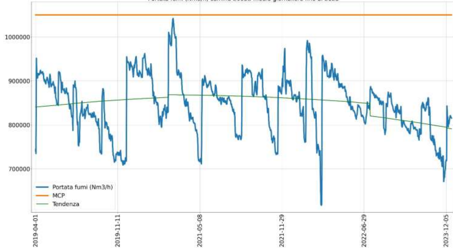
Portata fumi (Nm3/h) camino E103B medie giornaliere fino al 2023
