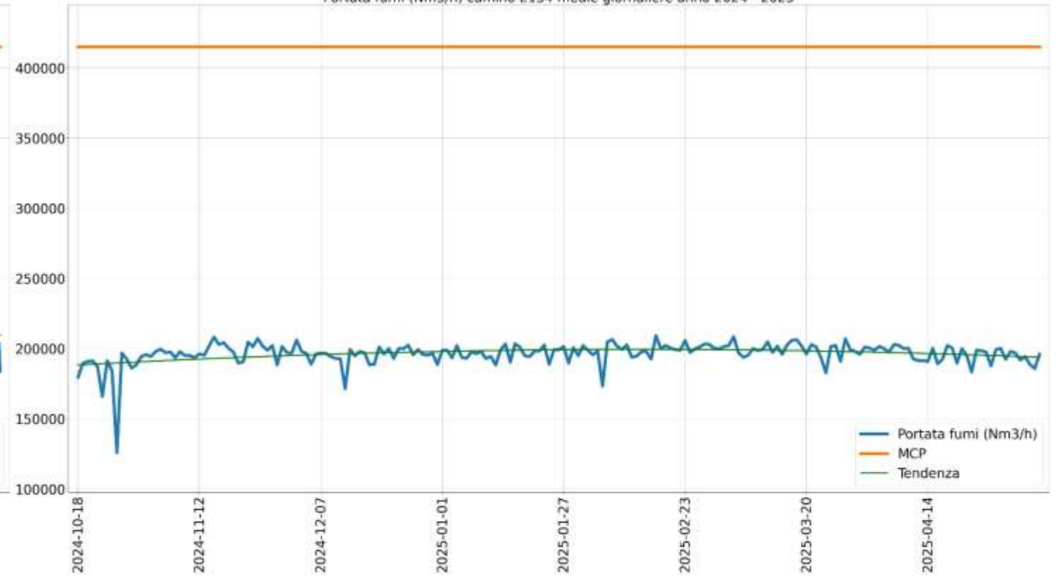
Portata fumi (Nm 3 /h) camino E134 medie giornaliere anno 2024 - 2025
