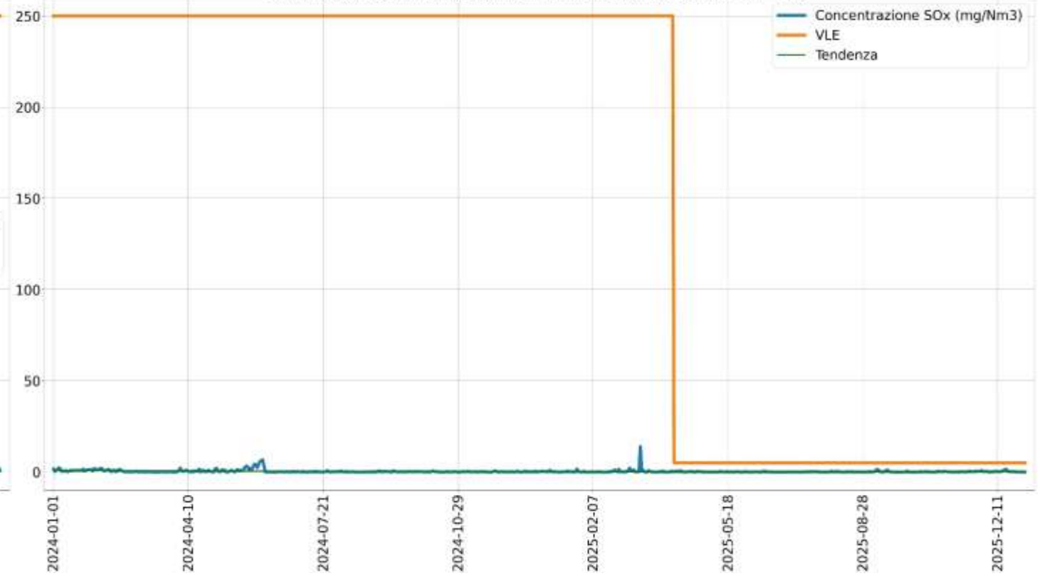
Concentrazione SOx (mg/Nm3) camino E437 medie giornaliere anno 2024 - 2025
