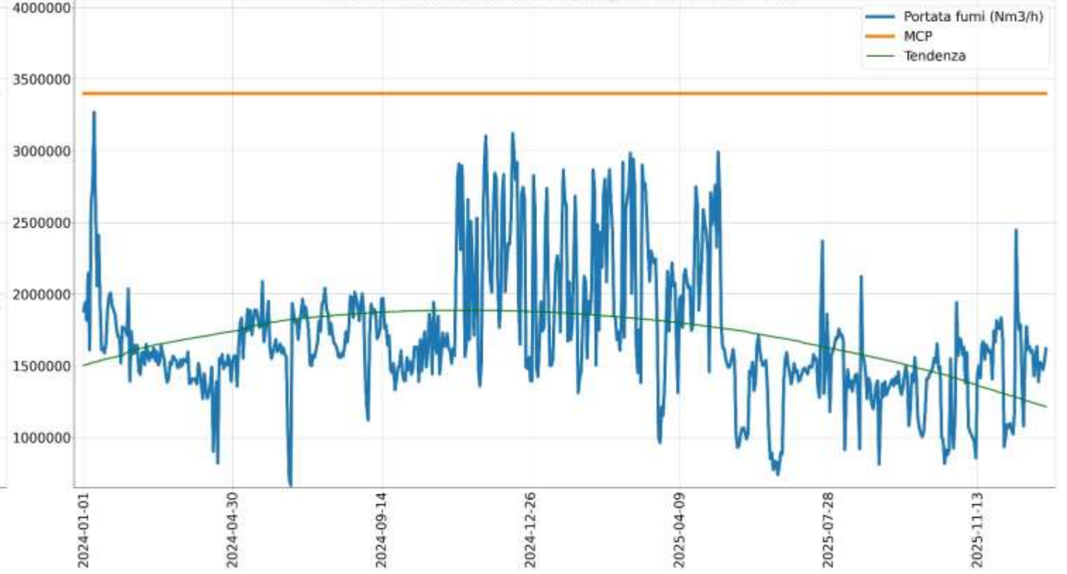
Portata fumi (Nm3/h) camino E312 medie giornaliere anno 2024 - 2025
