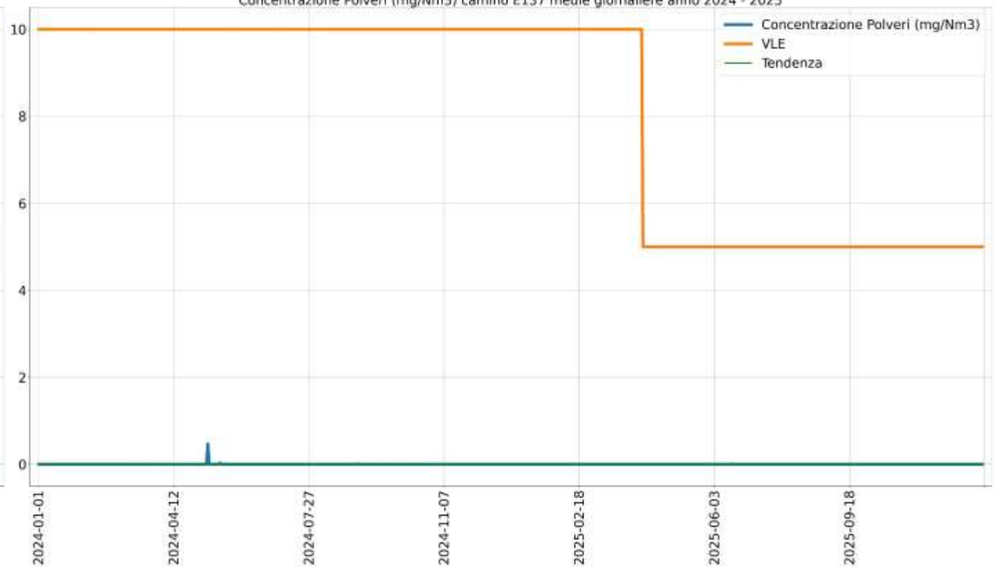
Concentrazione Polveri (mg/Nm3) camino E137 medie giornaliere anno 2024 - 2025
