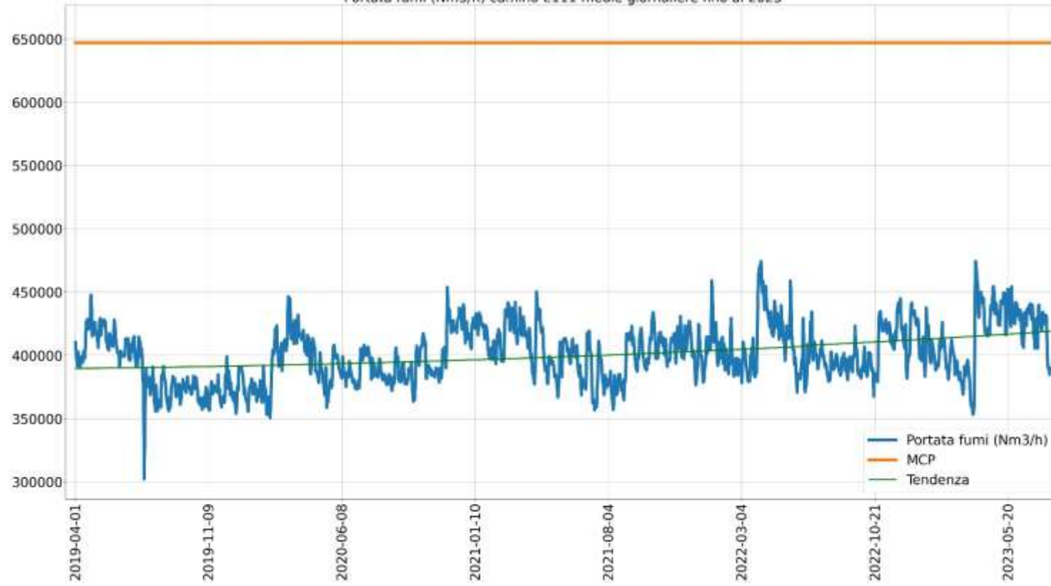
Portata fumi (Nm 3 /h) camino E111 medie giornaliere fino al 2023
