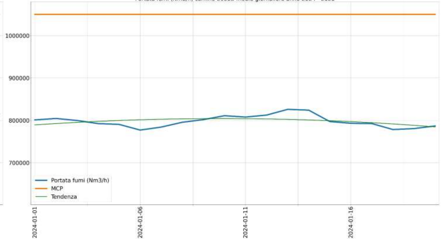
Portata fumi (Nm3/h) camino E103B medie giornaliere anno 2024 - 2025
