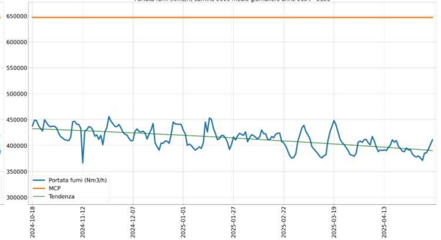
Portata fumi (Nm 3 /h) camino E111 medie giornaliere anno 2024 - 2025
