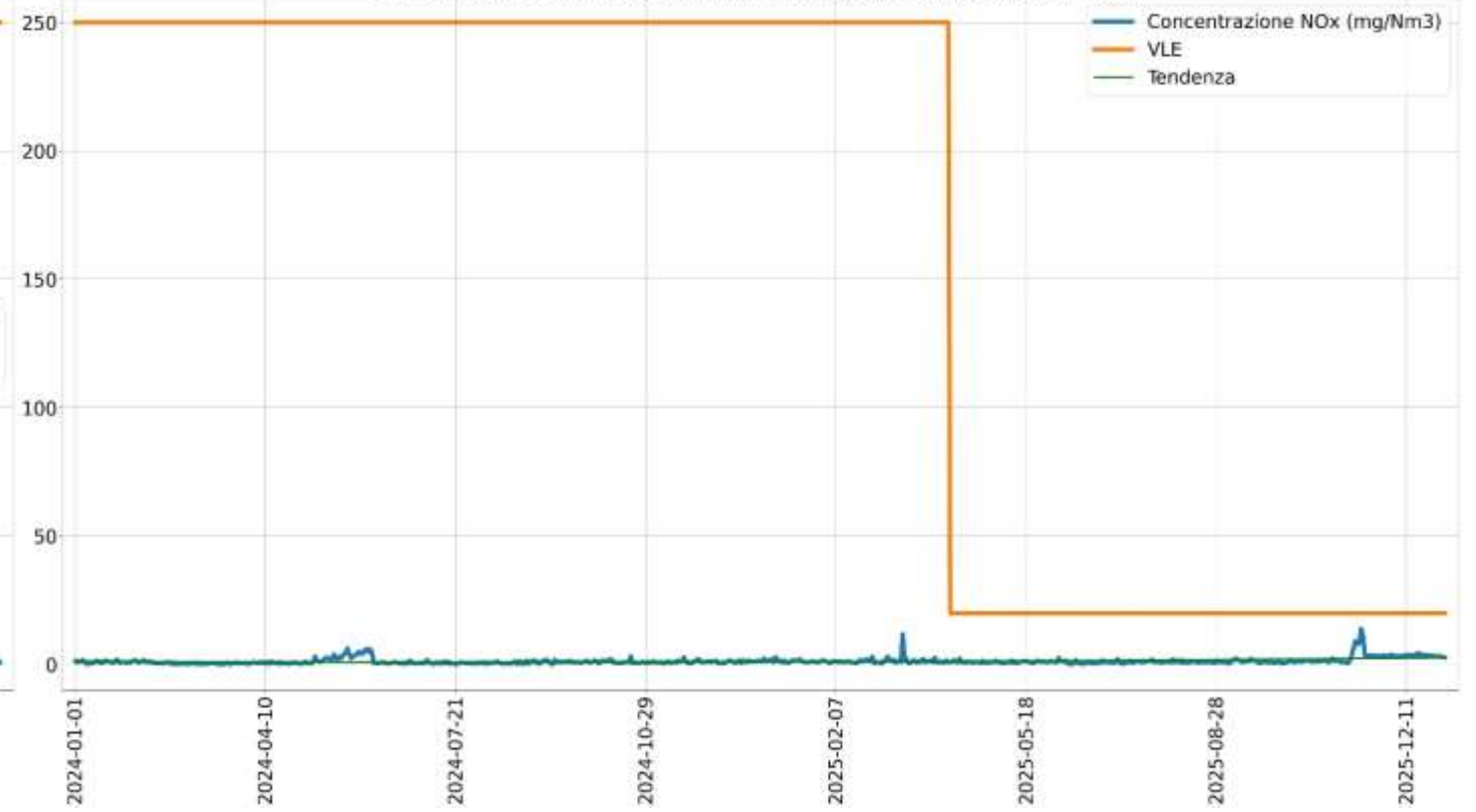
Concentrazione NOx (mg/Nm3) camino E437 medie giornaliere anno 2024 - 2025
