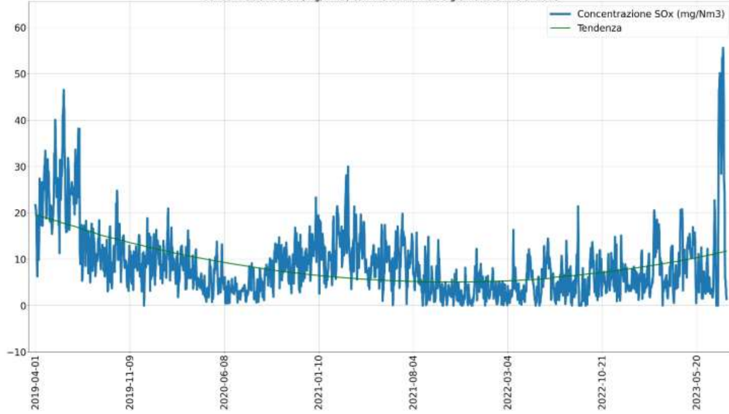
Concentrazione SO x (mg/Nm 3 ) camino E111 medie giornaliere fino al 2023
