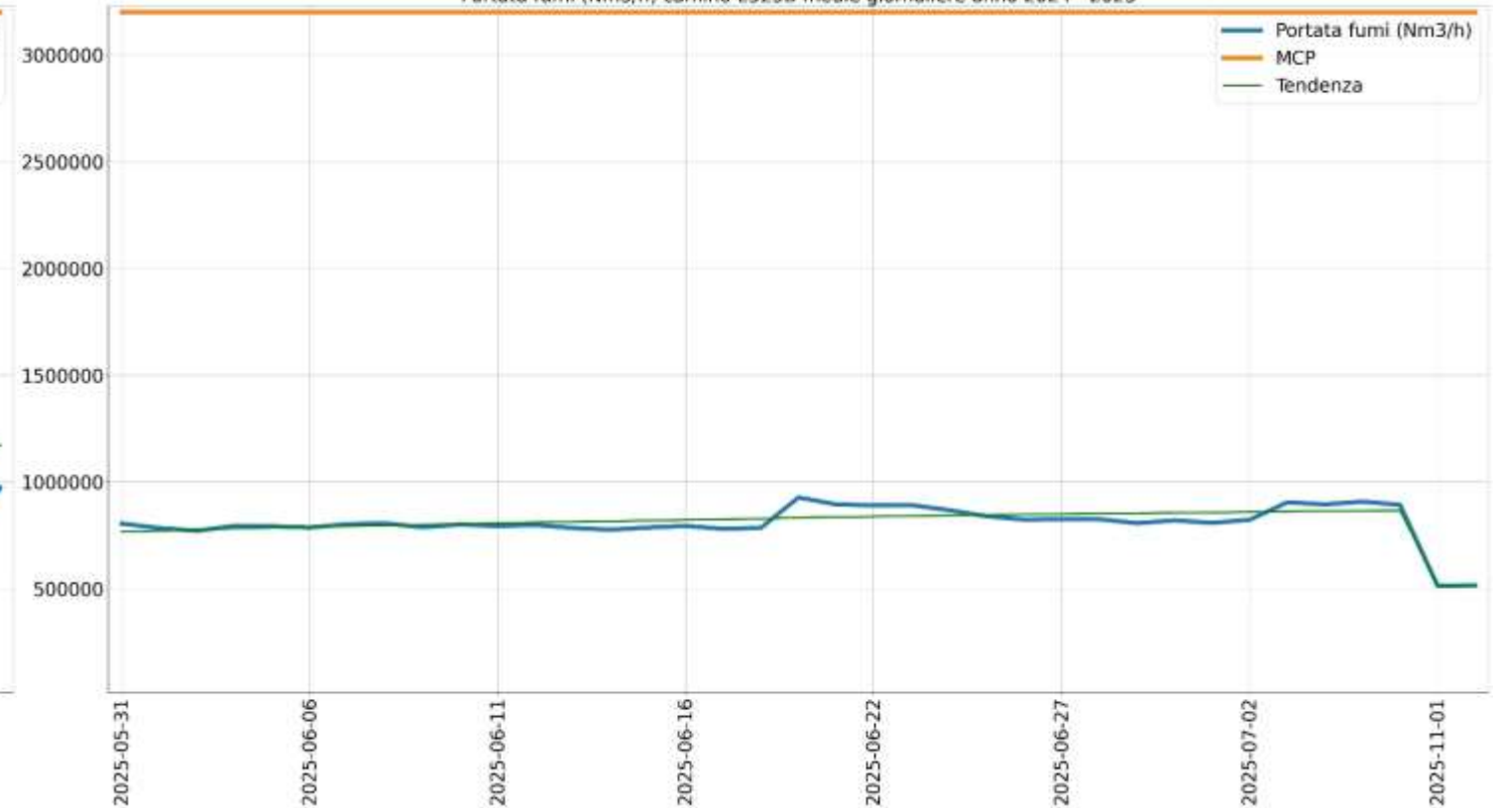
Portata fumi (Nm3/h) camino E525B medie giornaliere anno 2024 - 2025
