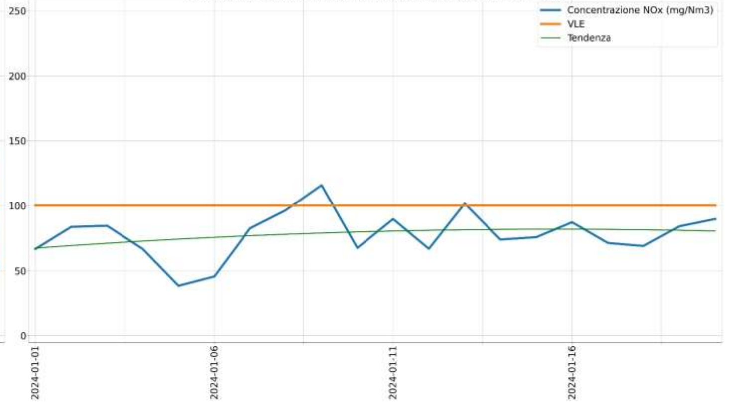
Concentrazione NOx (mg/Nm3) camino E135 medie giornaliere anno 2024 - 2025
