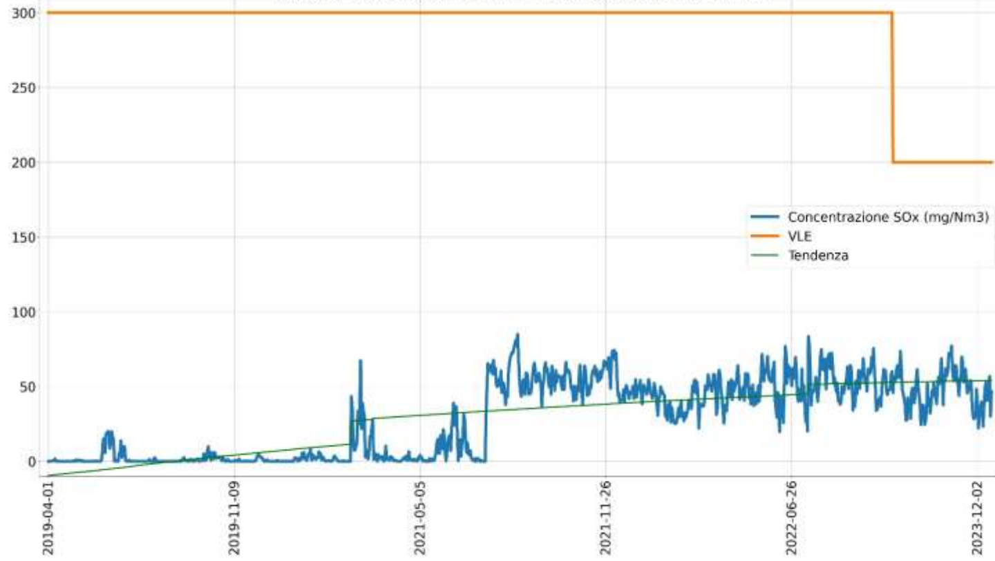
Concentrazione SOx (mg/Nm3) camino E135 medie giornaliere fino al 2023
