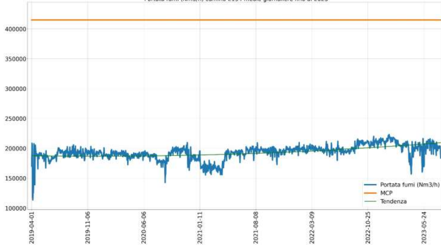
Portata fumi (Nm 3 /h) camino E134 medie giornaliere fino al 2023
