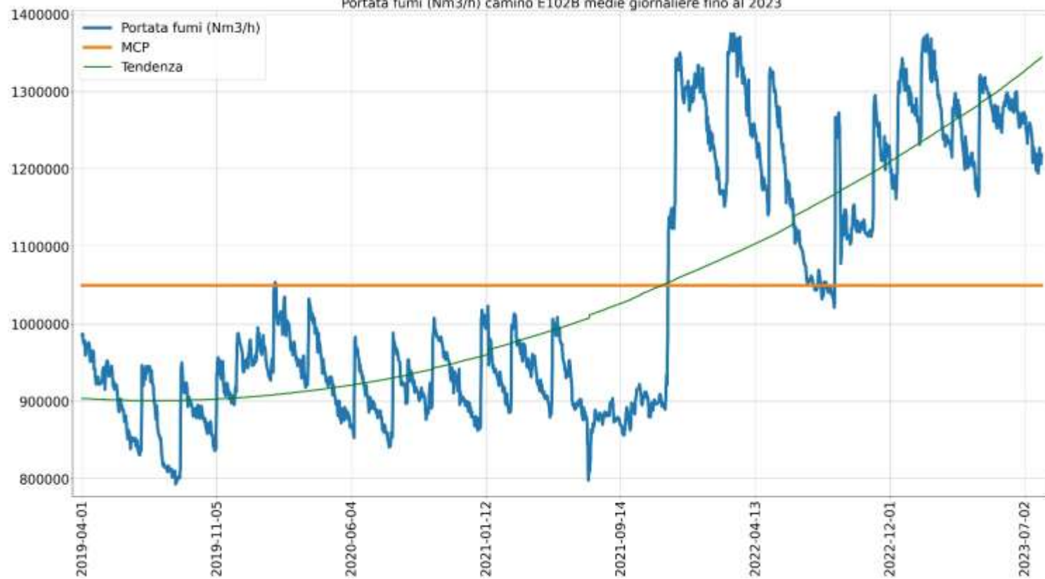
Portata fumi (Nm3/h) camino E102B medie giornaliere fino al 2023
