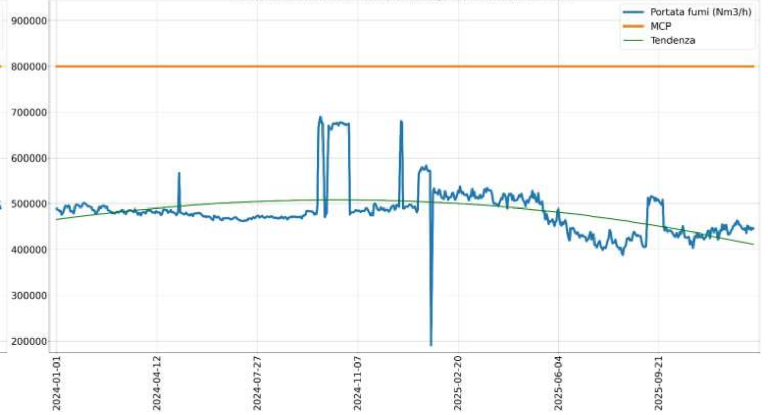
Portata fumi (Nm3/h) camino E109 medie giornaliere anno 2024 - 2025
