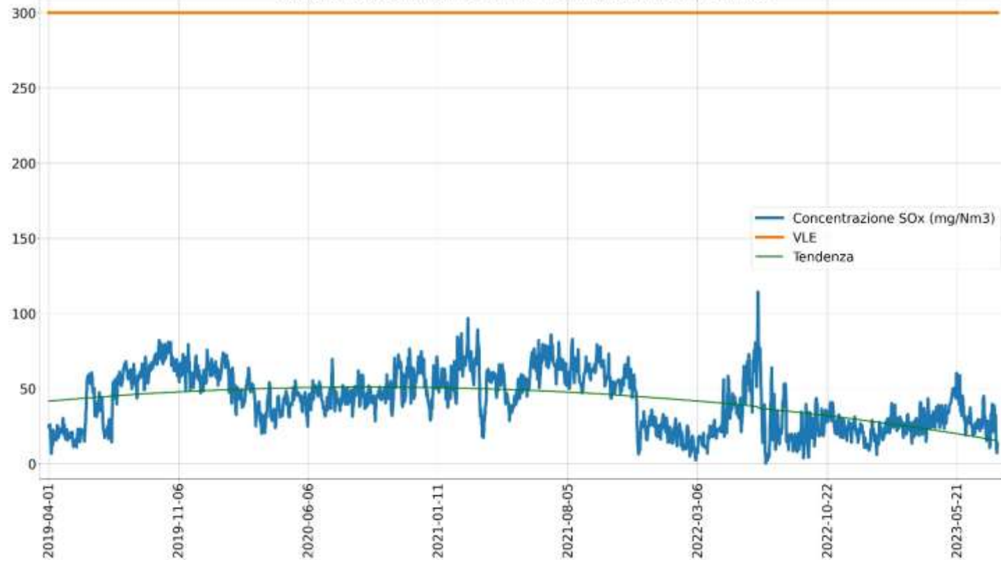
Concentrazione SOx (mg/Nm3) camino E134 medie giornaliere fino al 2023
