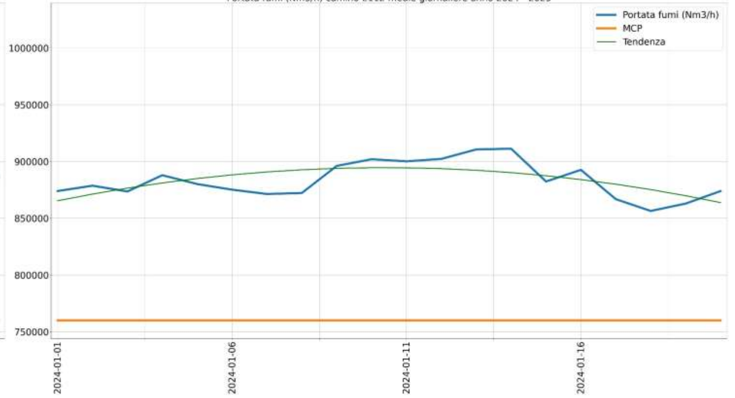
Portata fumi (Nm3/h) camino E112 medie giornaliere anno 2024 - 2025
