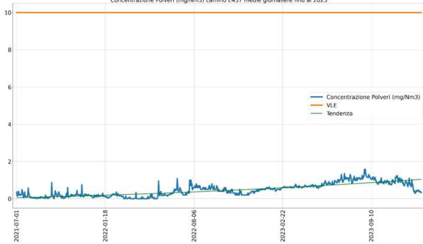
Concentrazione Polveri (mg/Nm3) camino E437 medie giornaliere fino al 2023
