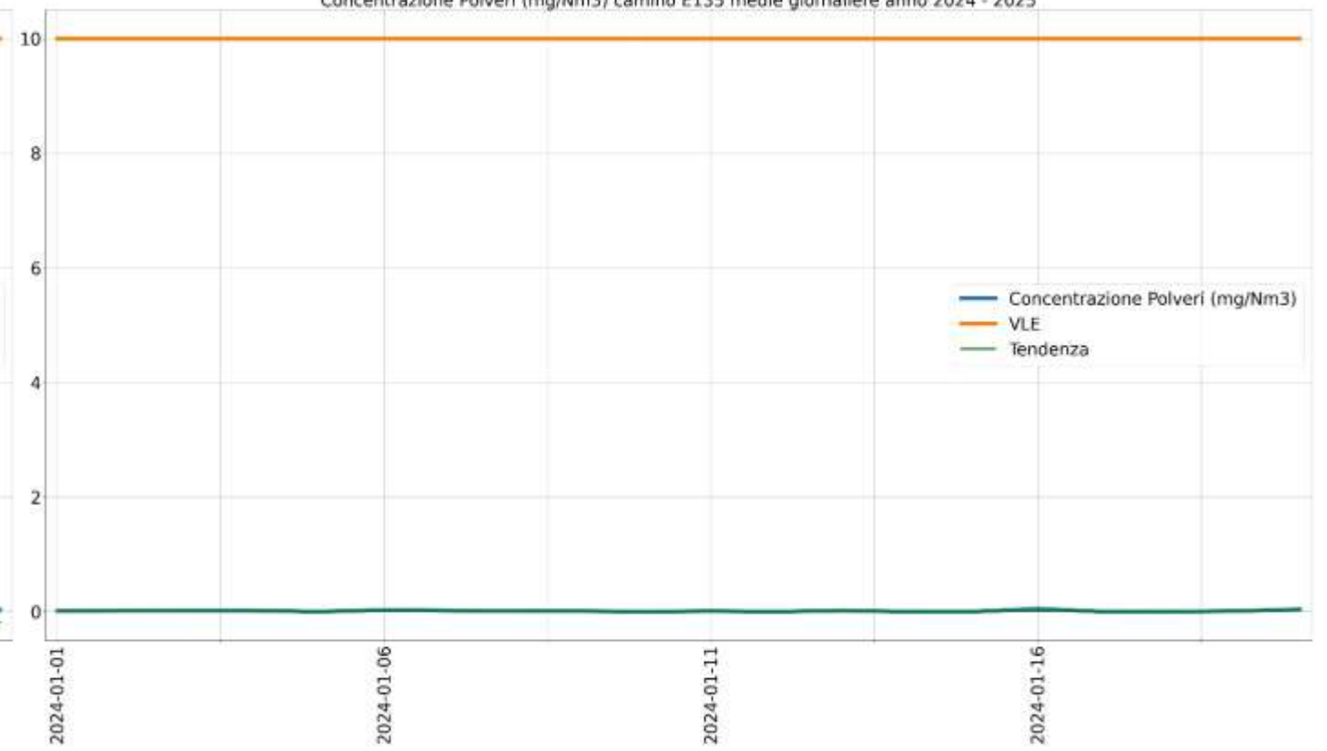
Concentrazione Polveri (mg/Nm 3 ) camino E135 medie giornaliere anno 2024 - 2025
