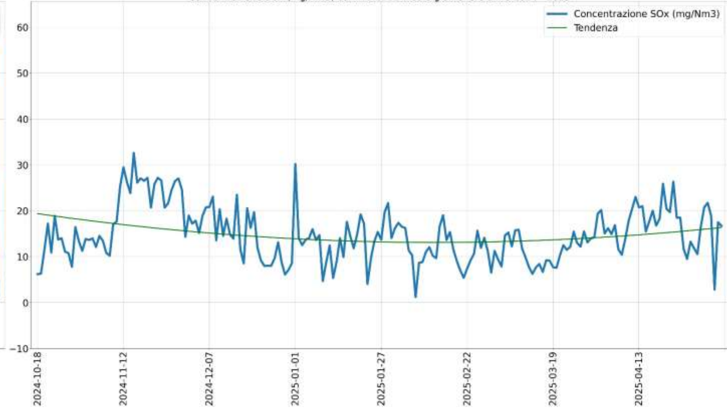
Concentrazione SO x (mg/Nm 3 ) camino E111 medie giornaliere anno 2024 - 2025
