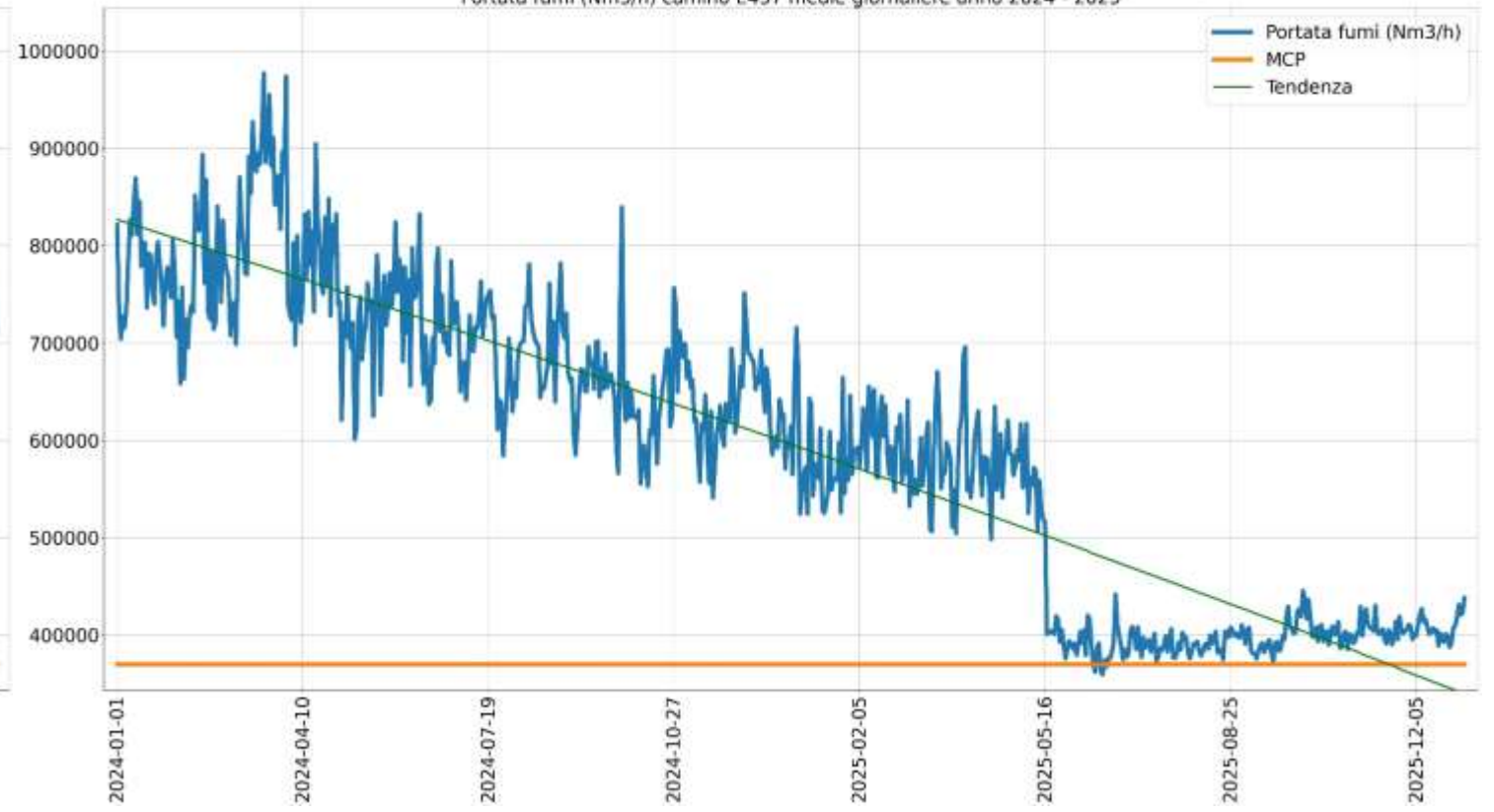
Portata fumi (Nm 3 /h) camino E437 medie giornaliere anno 2024 - 2025
