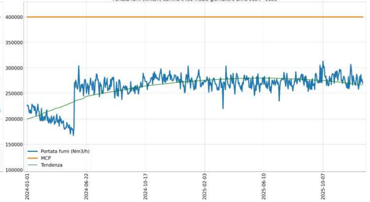
Portata fumi (Nm3/h) camino E435 medie giornaliere anno 2024 - 2025
