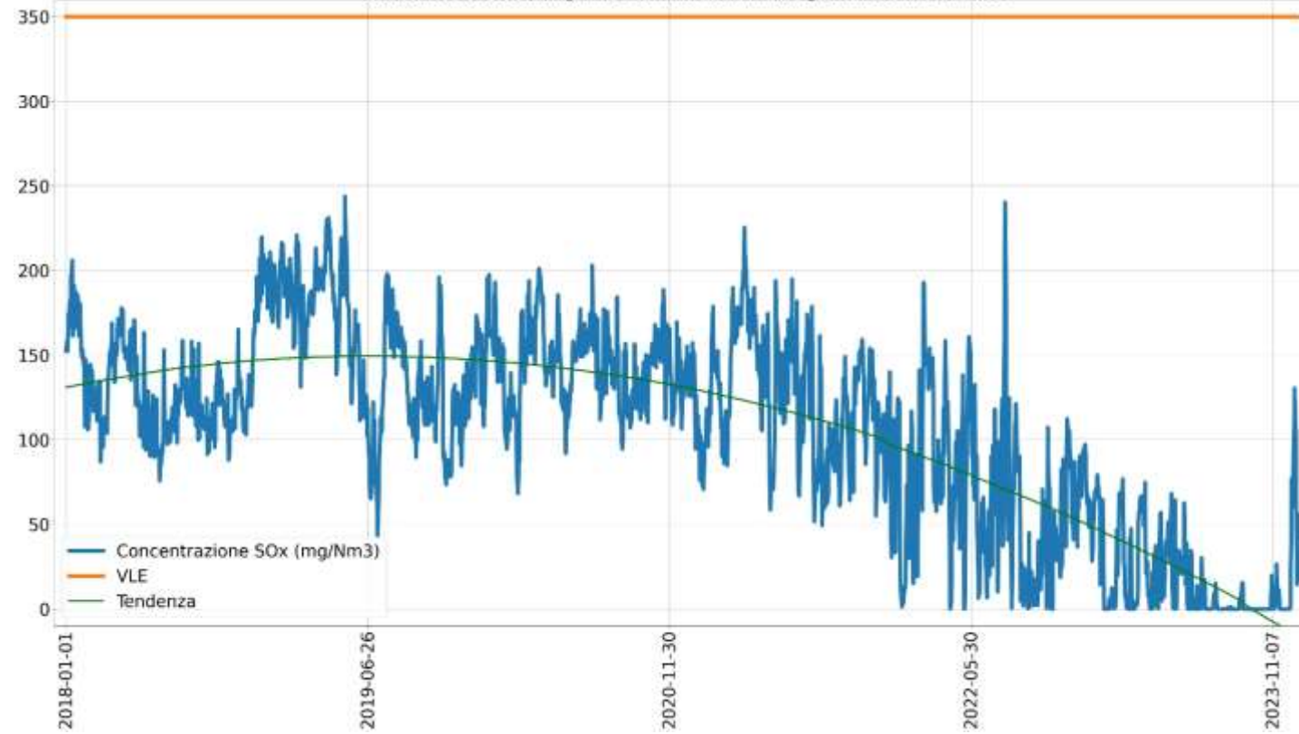
Concentrazione SOx (mg/Nm3) camino E312 medie giornaliere fino al 2023
