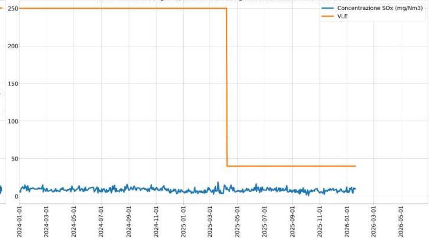
Concentrazione SO x (mg/Nm 3 ) camino E435 medie giornaliere anno 2024 - I° semestre 2026
