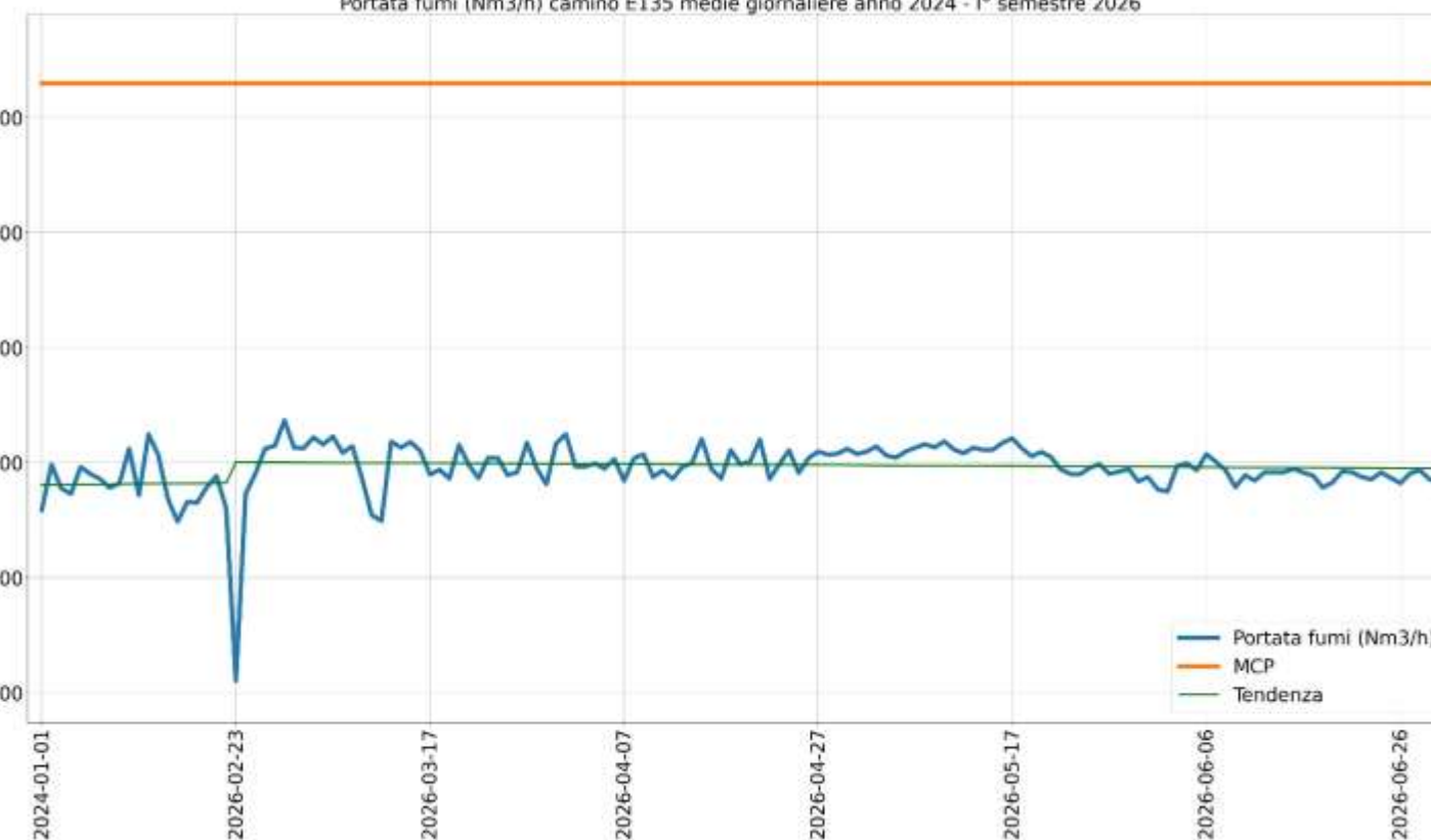
Portata fumi (Nm 3 /h) camino E135 medie giornaliere anno 2024 - I° semestre 2026
