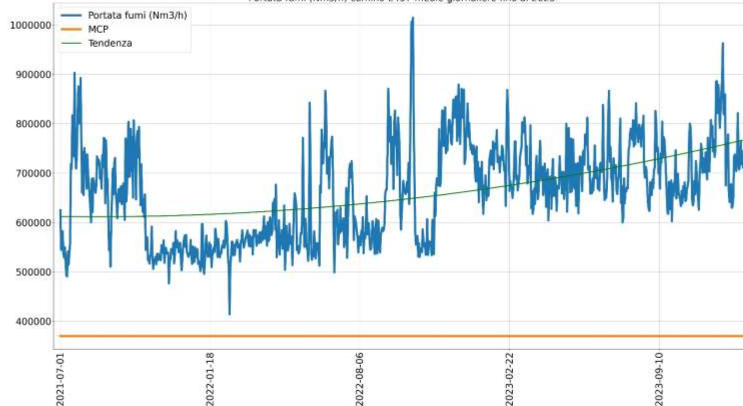
Portata fumi (Nm3/h) camino E437 medie giornaliere fino al 2023
