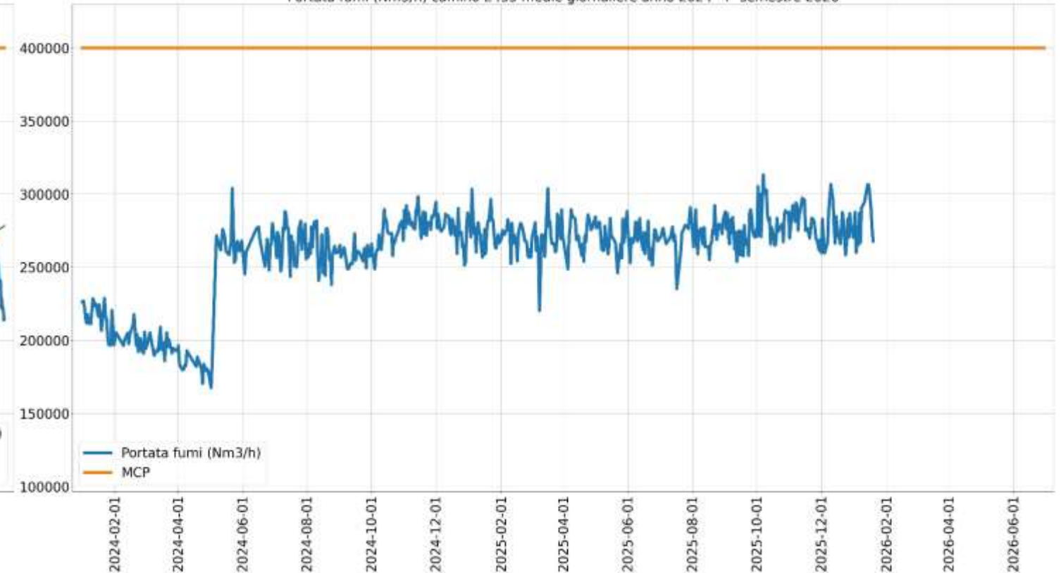
Portata fumi (Nm 3 /h) camino E435 medie giornaliere anno 2024 - I° semestre 2026
