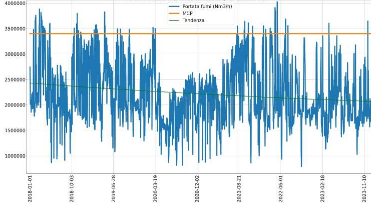
Portata fumi (Nm3/h) camino E312 medie giornaliere fino al 2023
