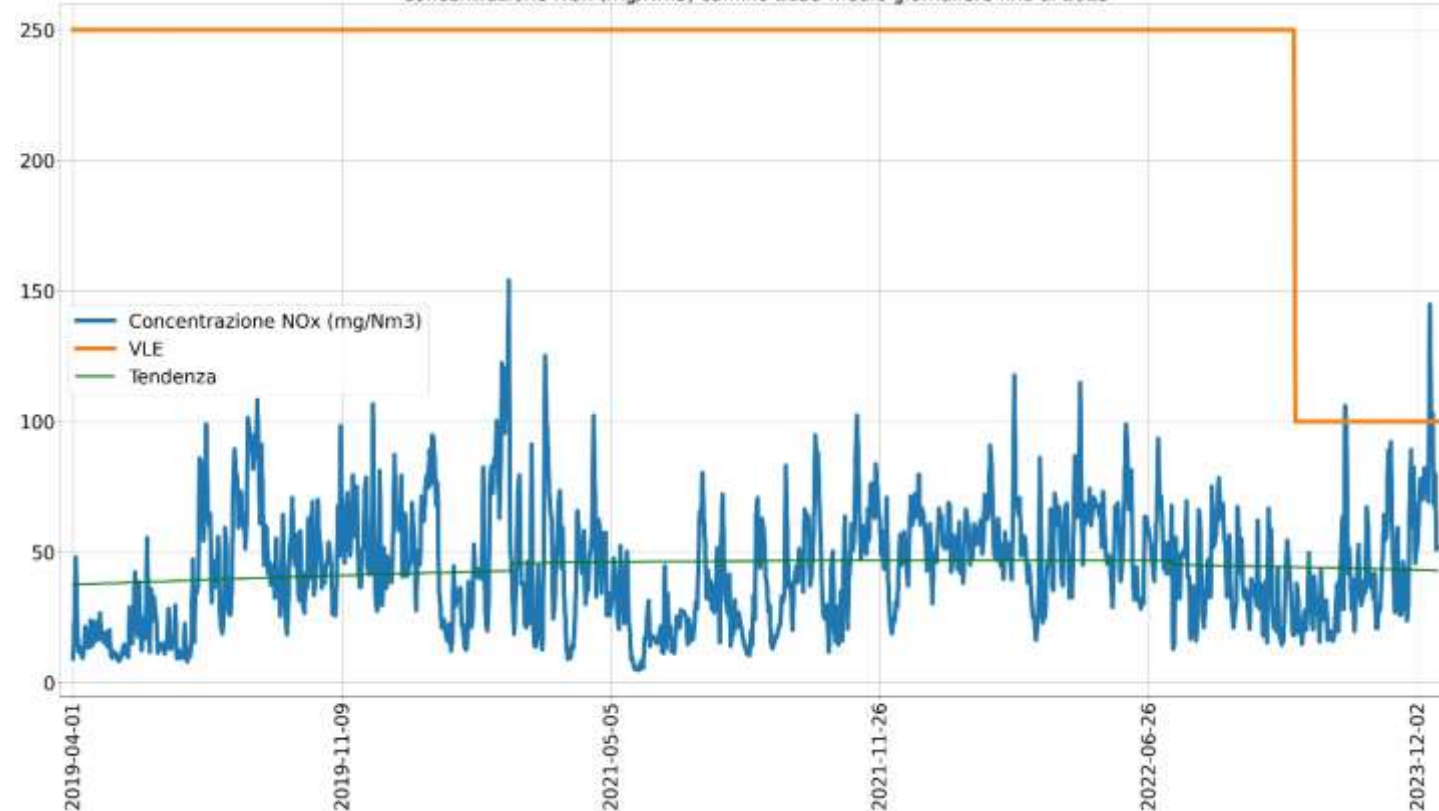
Concentrazione NOx (mg/Nm3) camino E135 medie giornaliere fino al 2023
