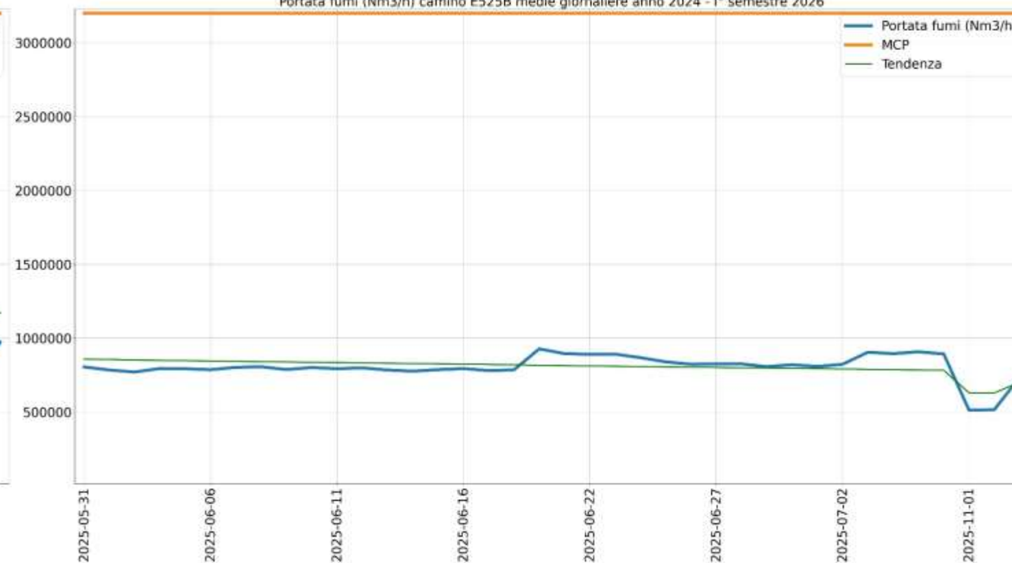
Portata fumi (Nm3/h) camino E525B medie giornaliere anno 2024 - I° semestre 2026
