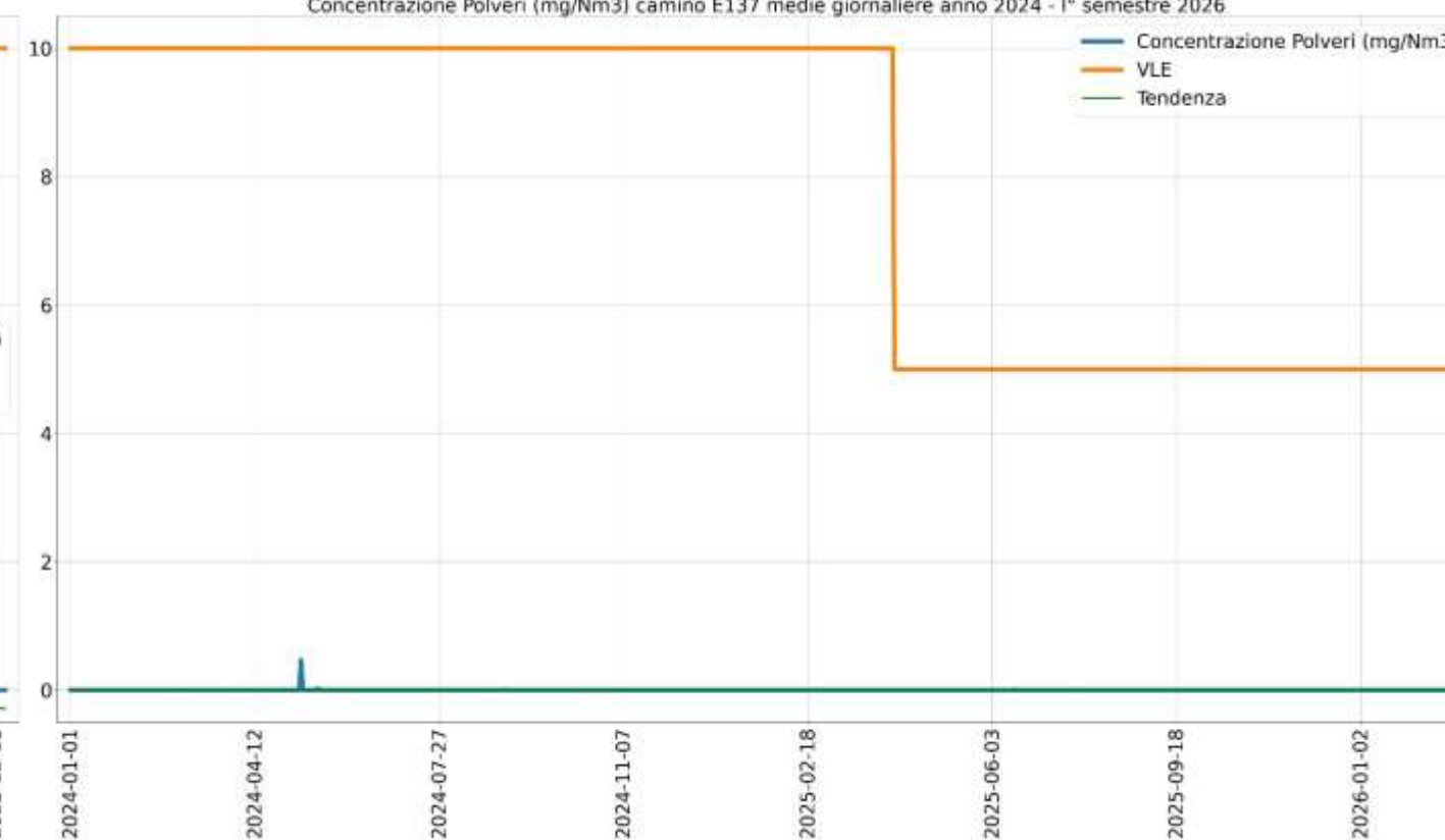
Concentrazione Polveri (mg/Nm 3 ) camino E137 medie giornaliere anno 2024 - I° semestre 2026
