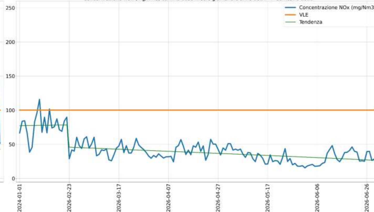
Concentrazione NOx (mg/Nm3) camino E135 medie giornaliere anno 2024 - I° semestre 2026
