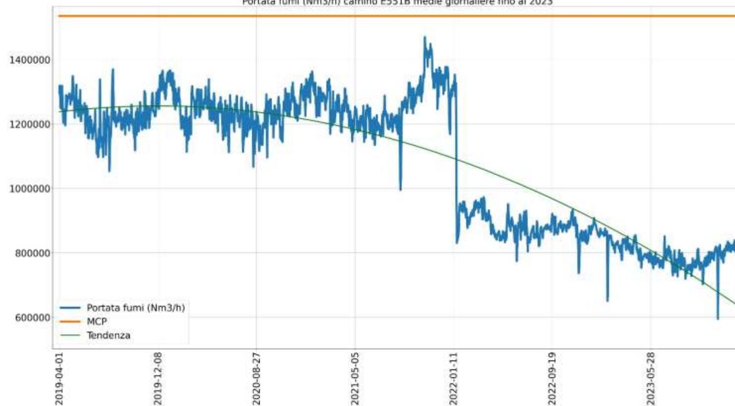
Portata fumi (Nm3/h) camino E551B medie giornaliere fino al 2023
