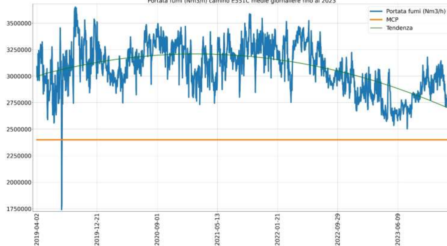
Portata fumi (Nm 3 /h) camino E551C medie giornaliere fino al 2023
