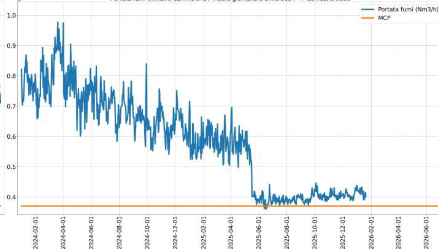
Portata fumi (Nm3/h) camino E437 medie giornaliere anno 2024 - I° semestre 2026
