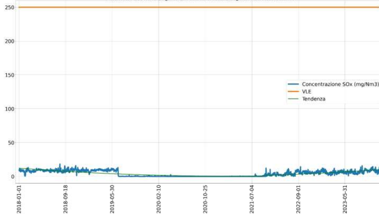
Concentrazione SO x (mg/Nm 3 ) camino E435 medie giornaliere fino al 2023
