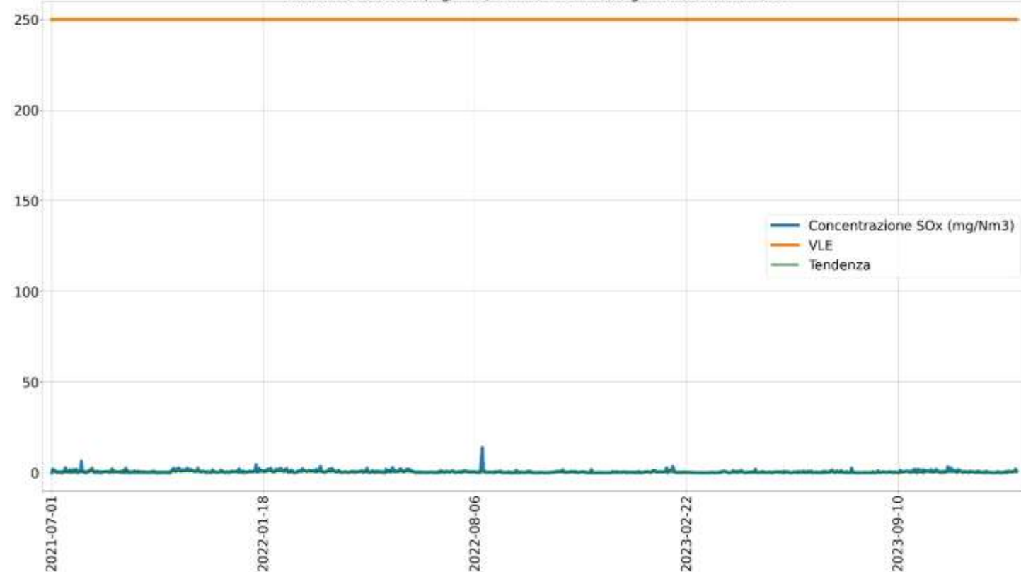
Concentrazione SOx (mg/Nm3) camino E437 medie giornaliere fino al 2023
