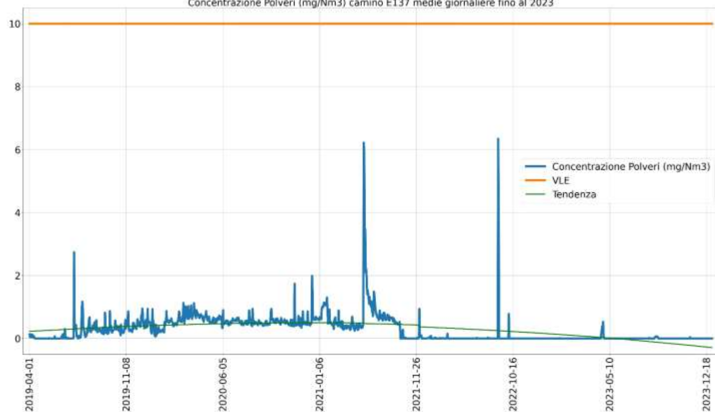
Concentrazione Polveri (mg/Nm 3 ) camino E137 medie giornaliere fino al 2023
