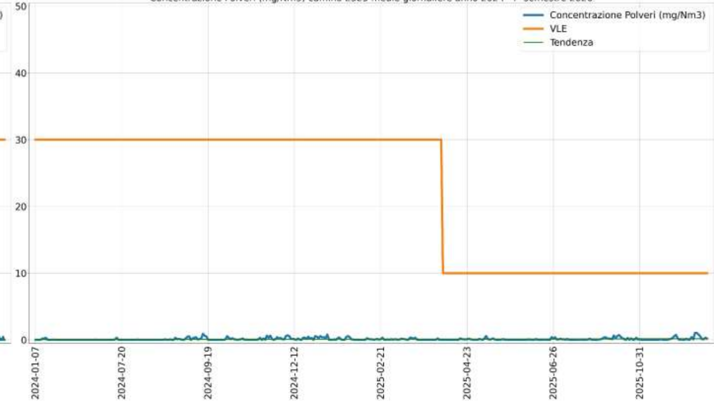
Concentrazione Polveri (mg/Nm 3 ) camino E325 medie giornaliere anno 2024 - I° semestre 2026
