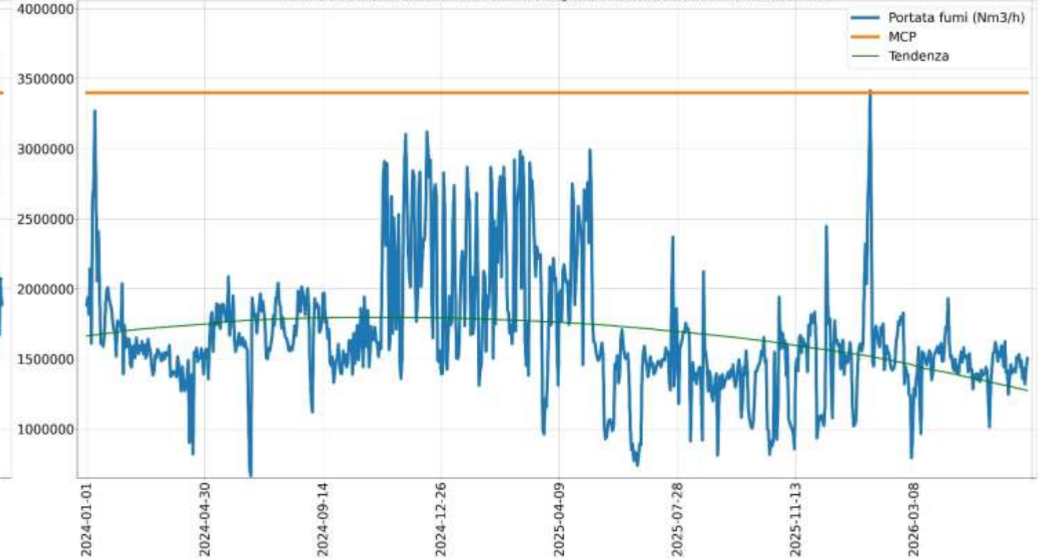
Portata fumi (Nm3/h) camino E312 medie giornaliere anno 2024 - I° semestre 2026
