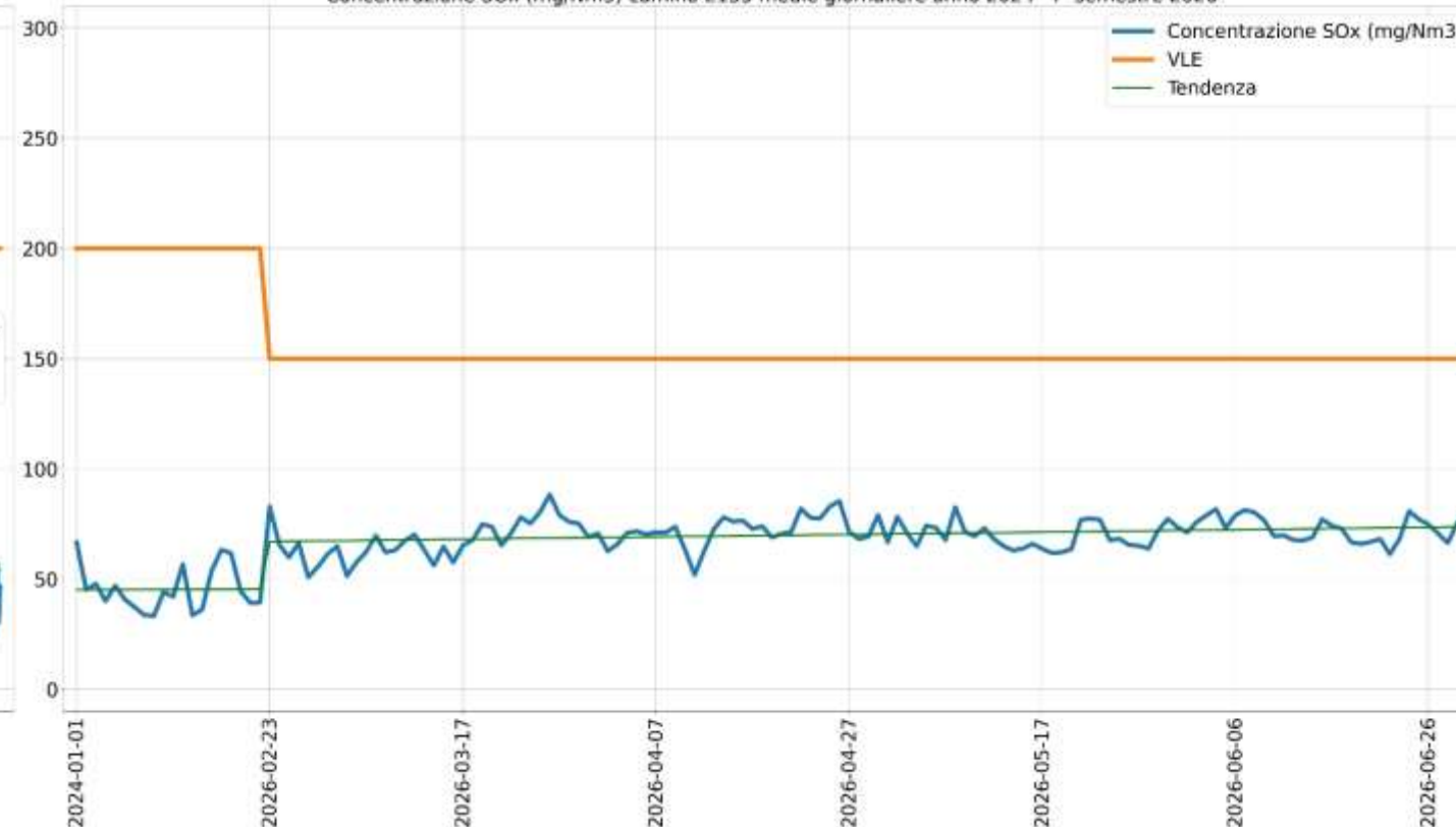
Concentrazione SOx (mg/Nm3) camino E135 medie giornaliere anno 2024 - I° semestre 2026
