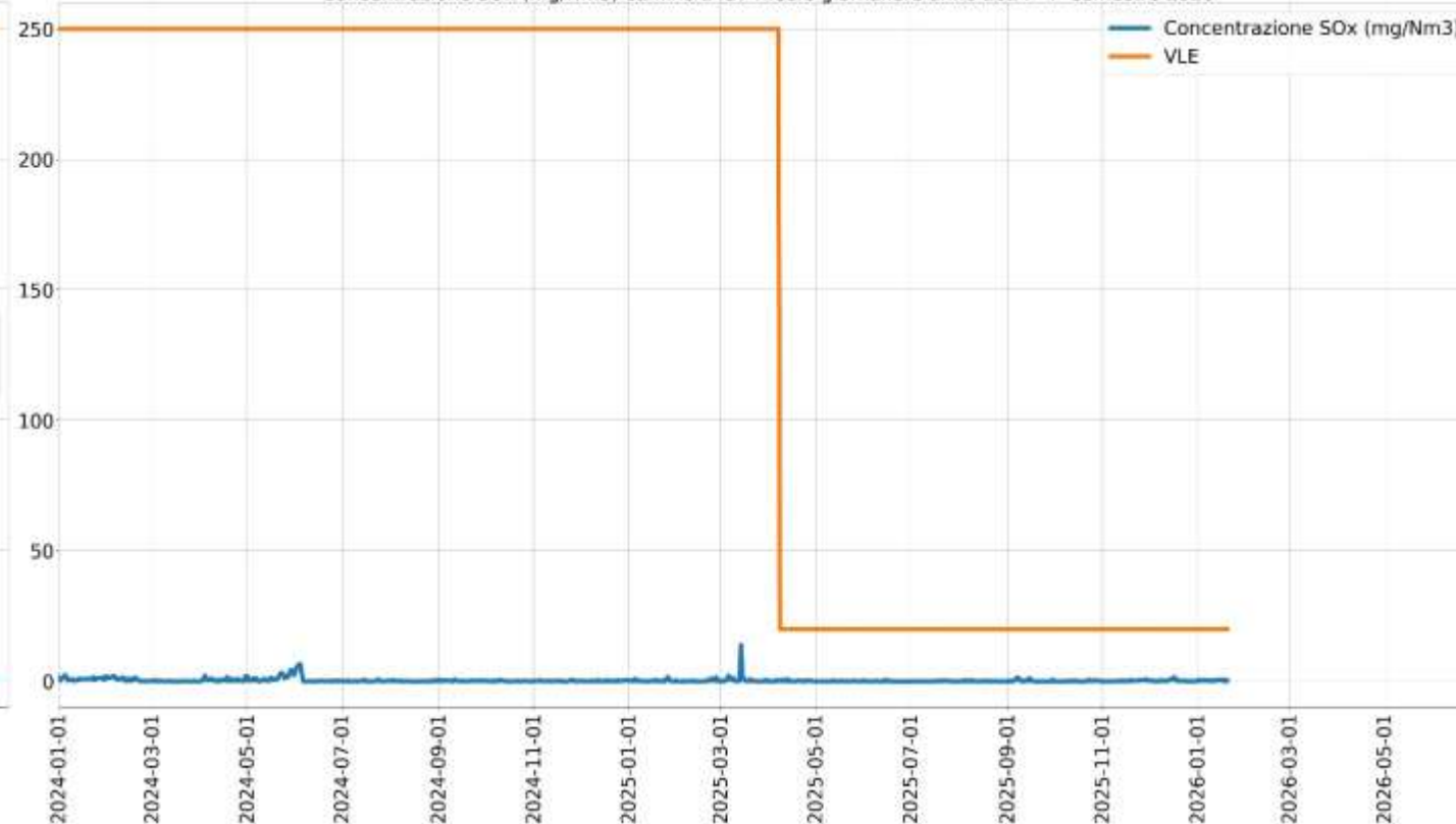
Concentrazione SOx (mg/Nm3) camino E437 medie giornaliere anno 2024 - I° semestre 2026
