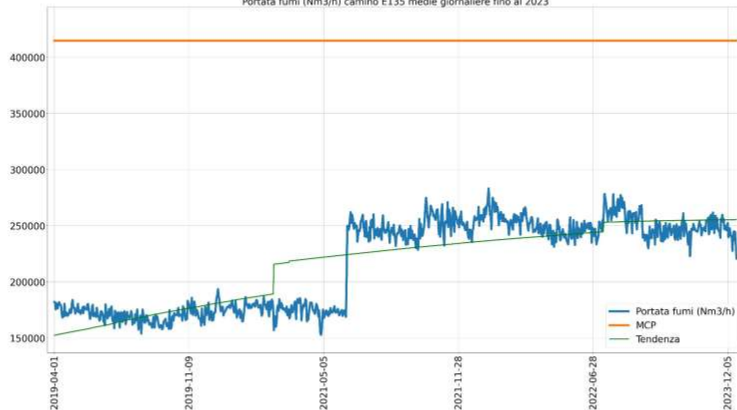
Portata fumi (Nm 3 /h) camino E135 medie giornaliere fino al 2023
