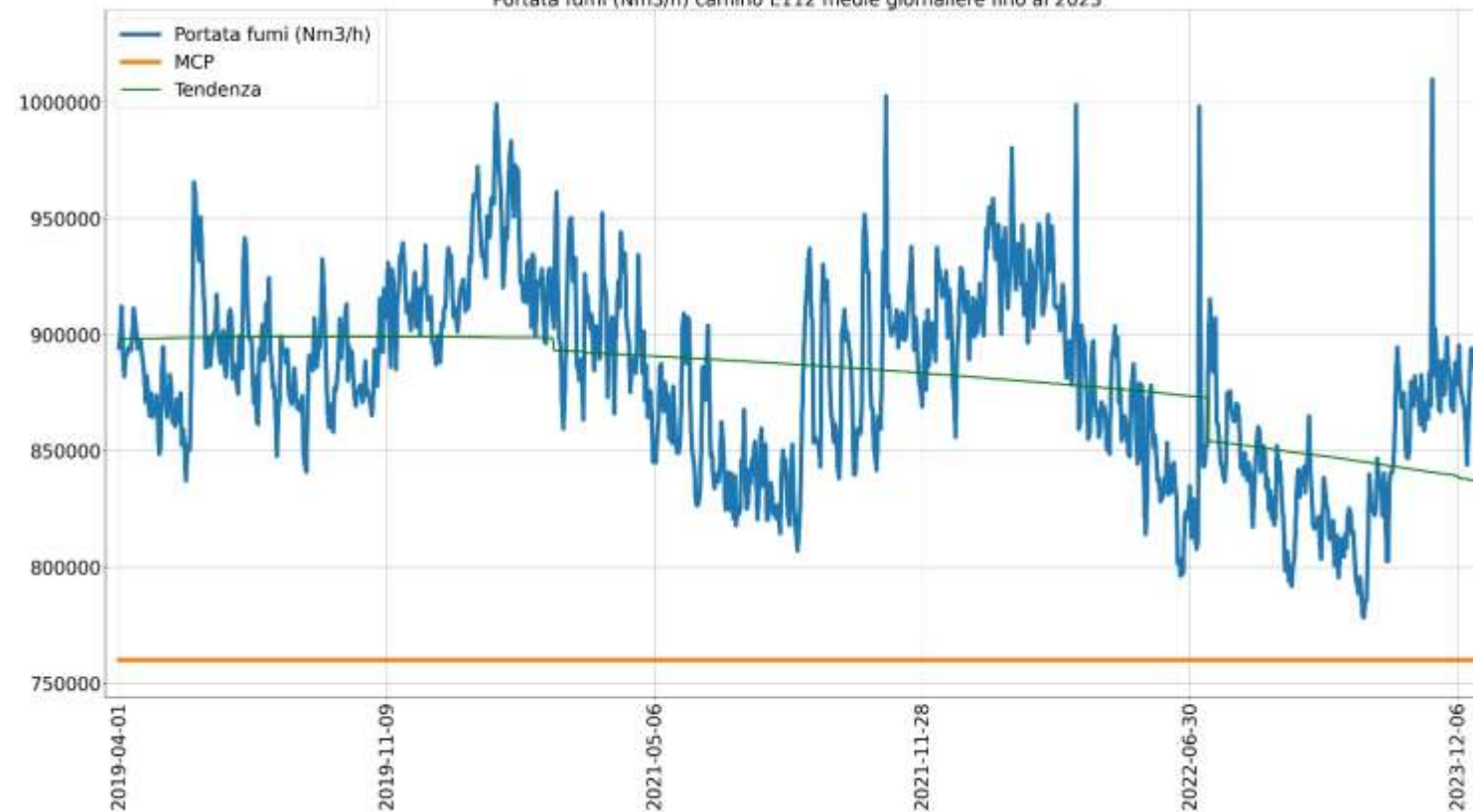
Portata fumi (Nm 3 /h) camino E112 medie giornaliere fino al 2023
