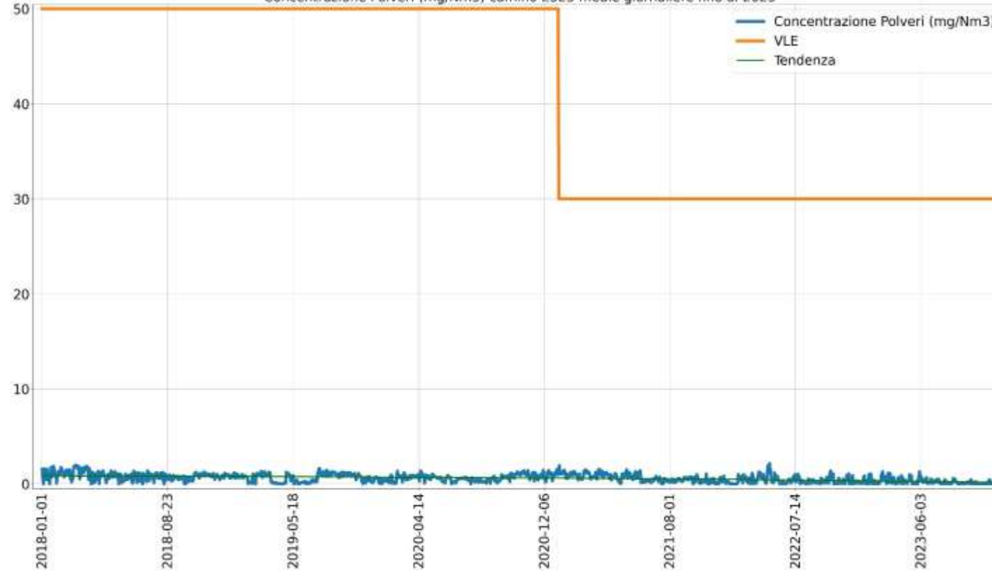
Concentrazione Polveri (mg/Nm 3 ) camino E325 medie giornaliere fino al 2023
