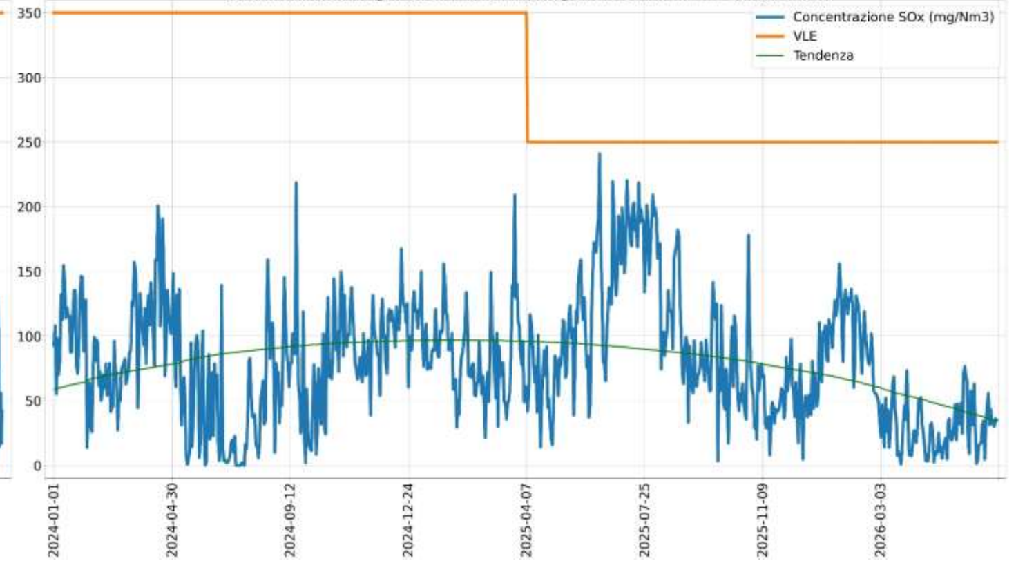
Concentrazione SOx (mg/Nm3) camino E312 medie giornaliere anno 2024 - I° semestre 2026
