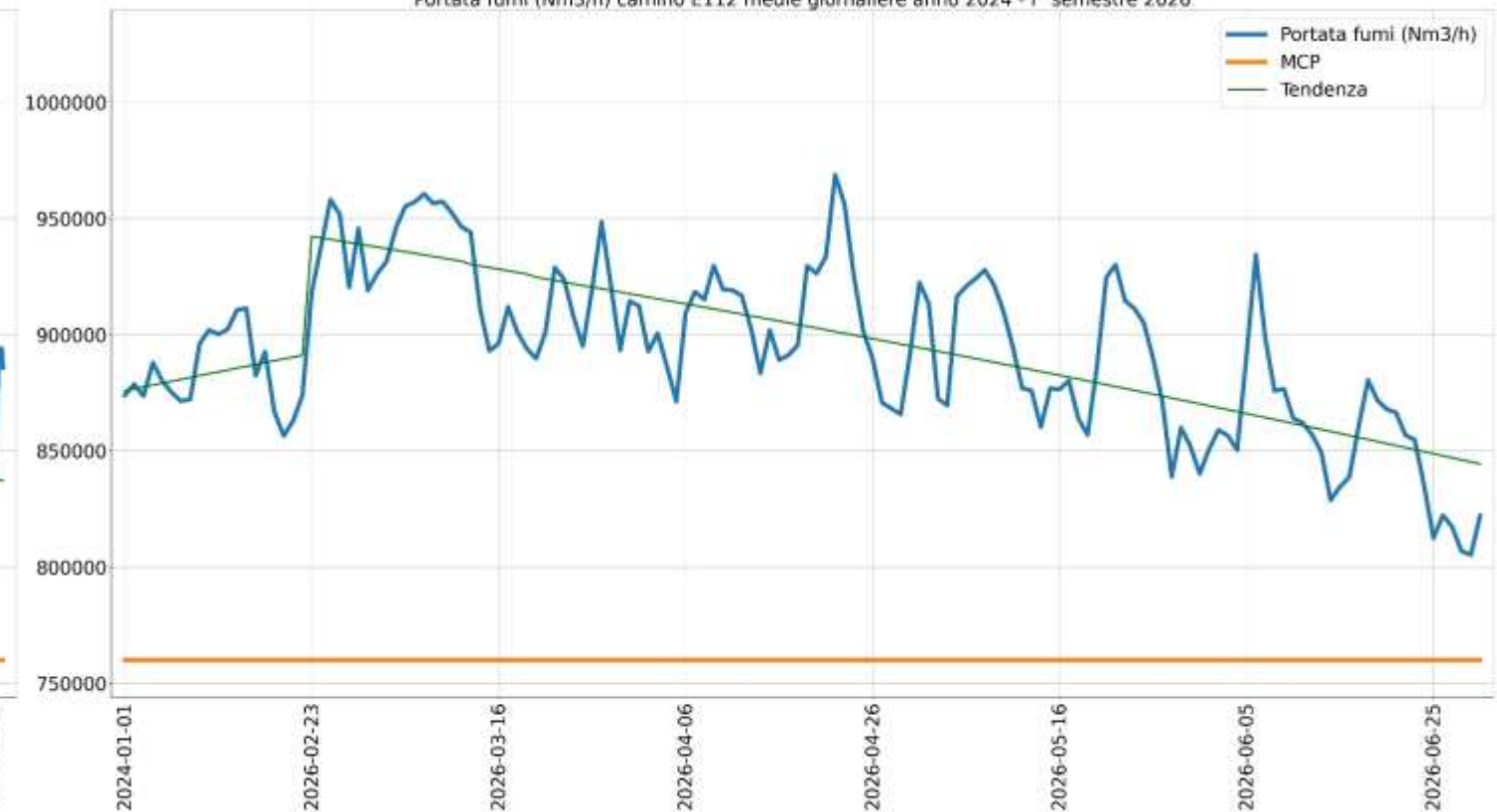
Portata fumi (Nm 3 /h) camino E112 medie giornaliere anno 2024 - I° semestre 2026
