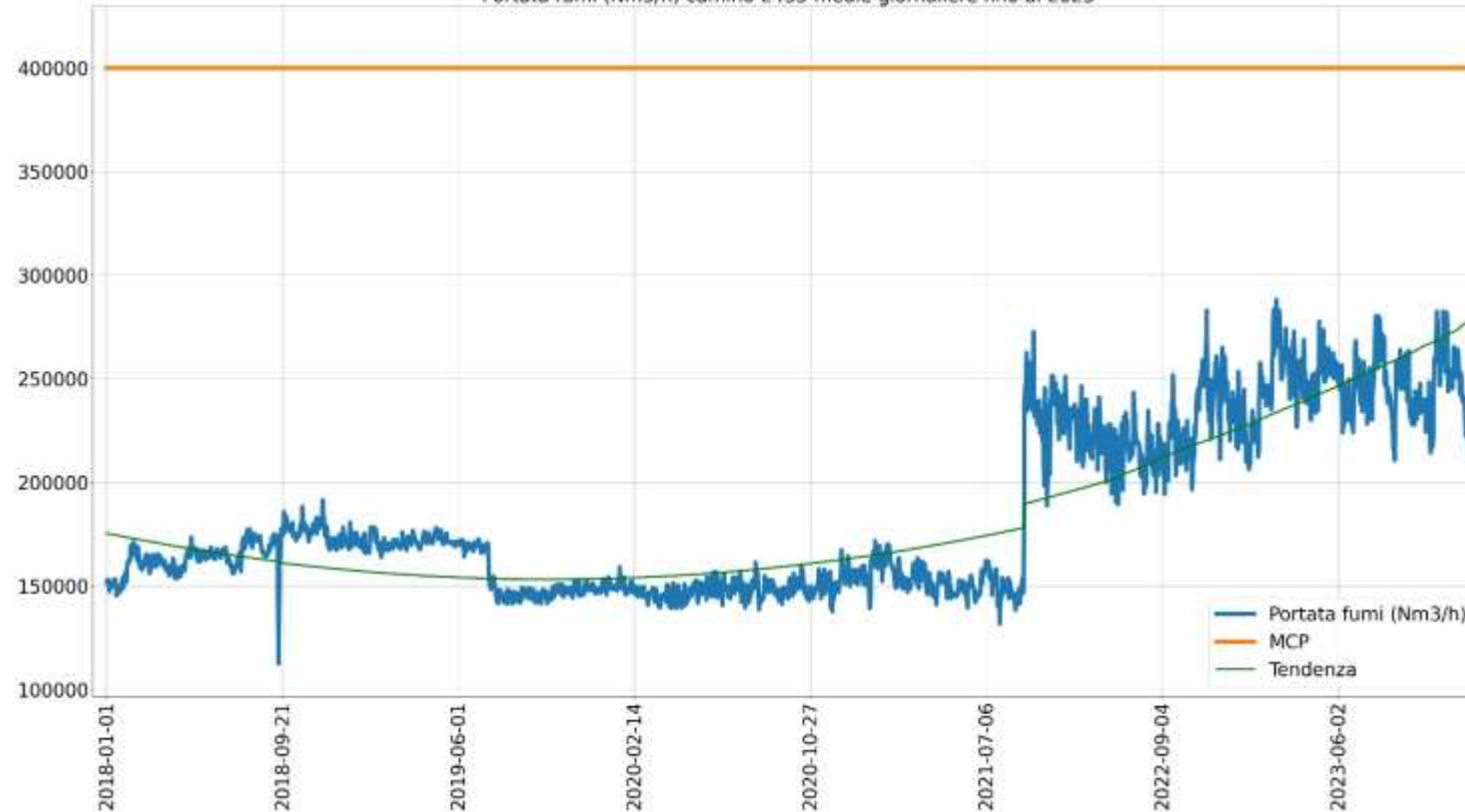
Portata fumi (Nm 3 /h) camino E435 medie giornaliere fino al 2023
