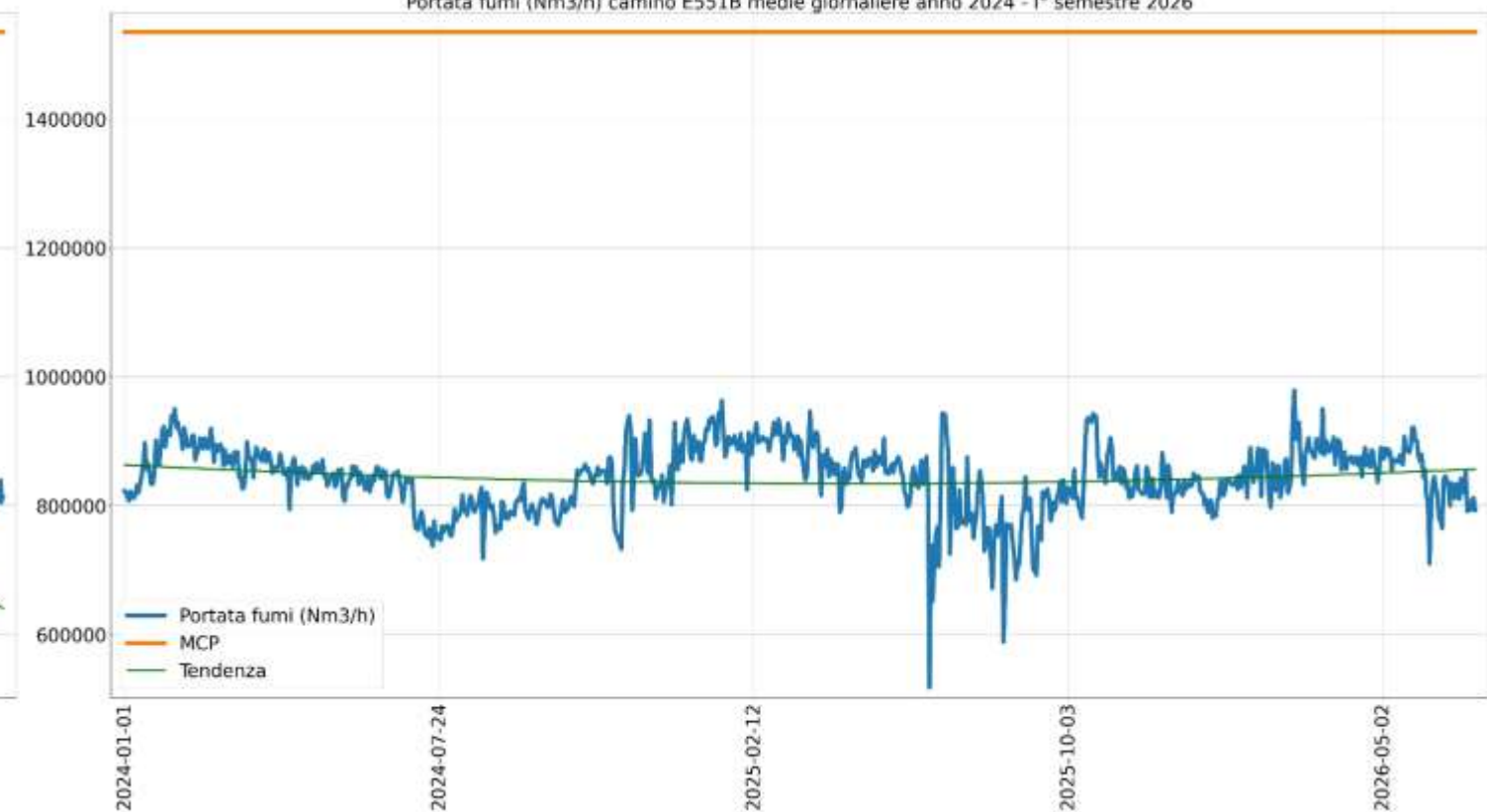
Portata fumi (Nm3/h) camino E551B medie giornaliere anno 2024 - I° semestre 2026
