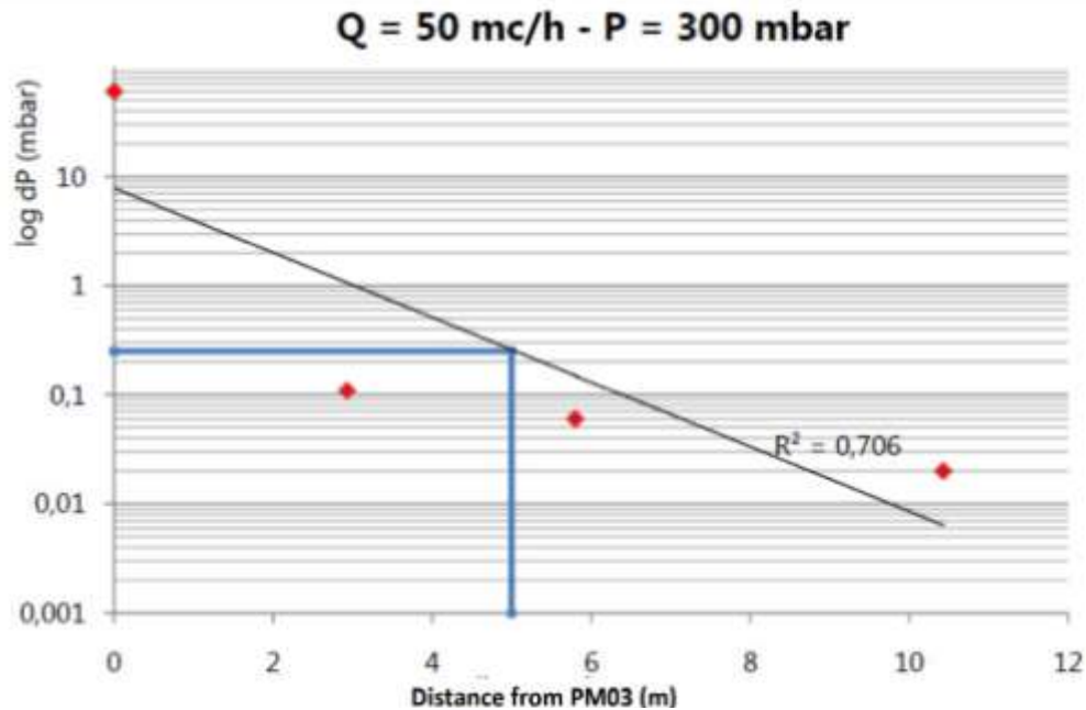
Figura 4.3.: Grafico del test ROI (per gentile concessione di Ing. Caldera F., Mares Italia)
