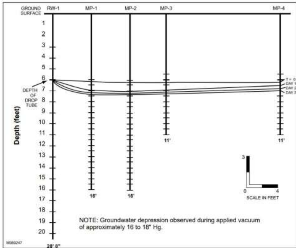
Figura 4.5.: Depressione della falda freatica durante il test pilota di bioslurping [25]
