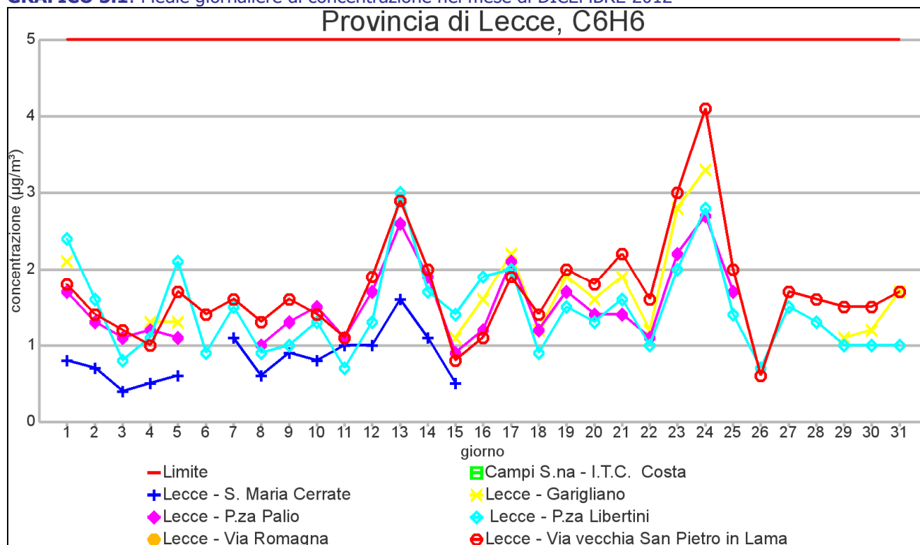
GRAFICO 5.1: Medie giornaliere di concentrazione nel mese di DICEMBRE 2012
