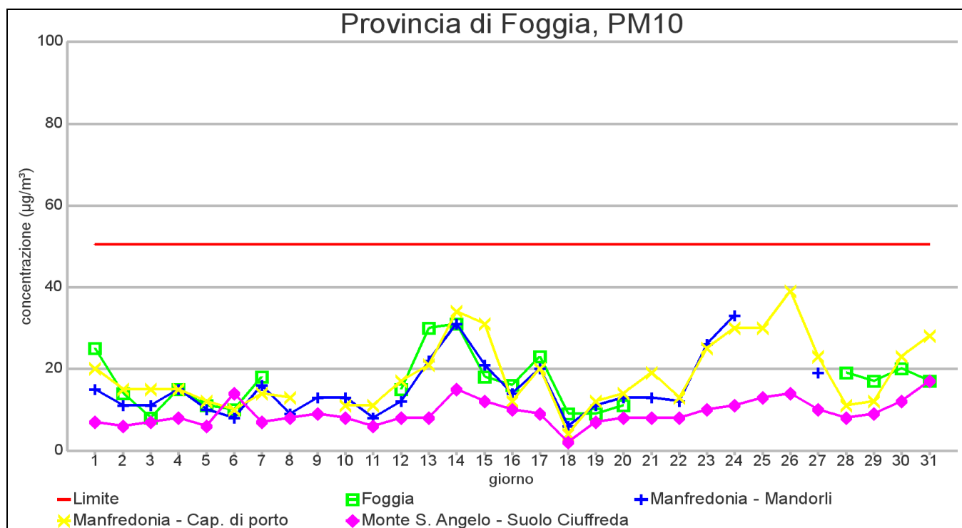
GRAFICO 1.1: Medie giornaliere di concentrazione nel mese di DICEMBRE 2012
