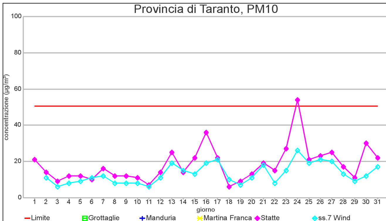
GRAFICO 1.2: Medie giornaliere di concentrazione nel mese di DICEMBRE 2012 – Provincia di Taranto
