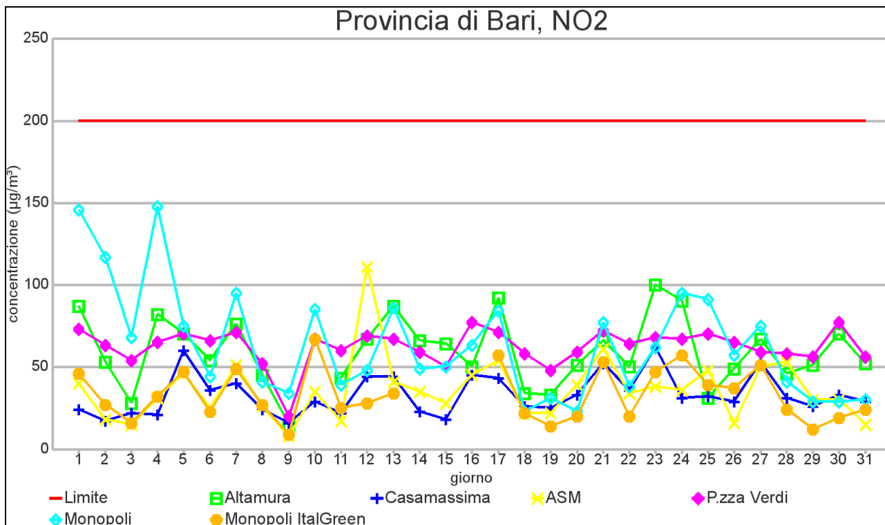
GRAFICO 2.3 PROVINCIA DI BARI: Valore massimo orario NO 2 – DICEMBRE 2012
