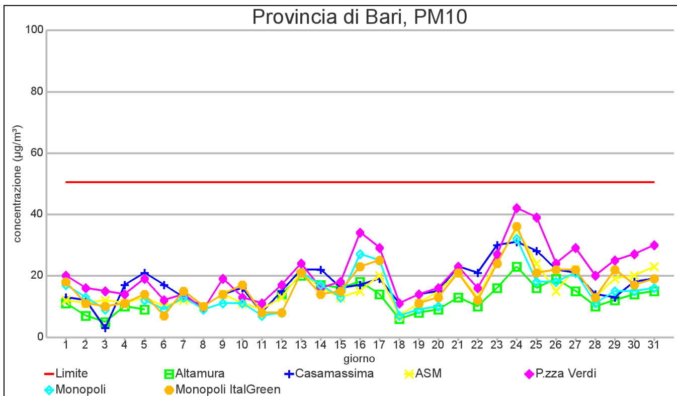
GRAFICO 1.3 PROVINCIA DI BARI: Valori medi giornalieri di concentrazione PM10 – DICEMBRE 2012
