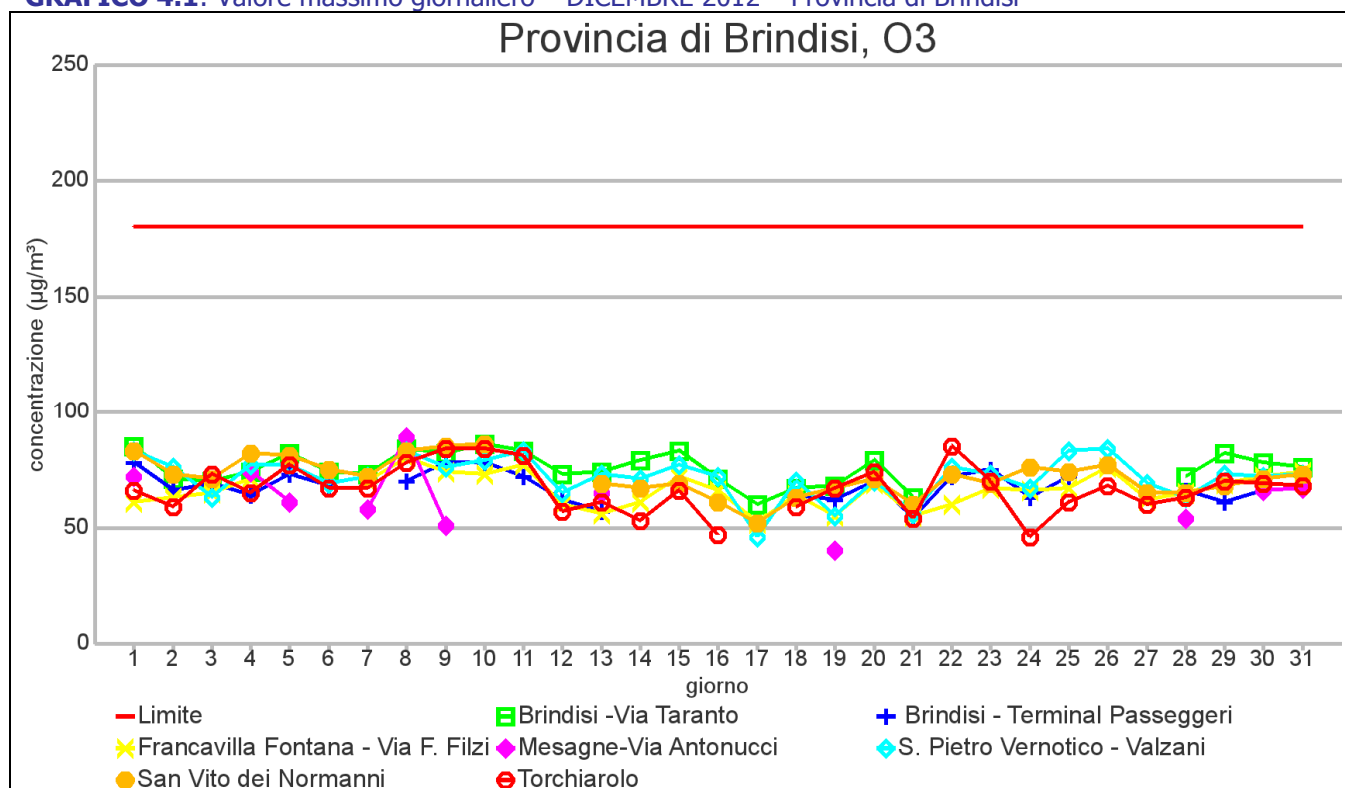
GRAFICO 4.1: Valore massimo giornaliero – DICEMBRE 2012 – Provincia di Brindisi
