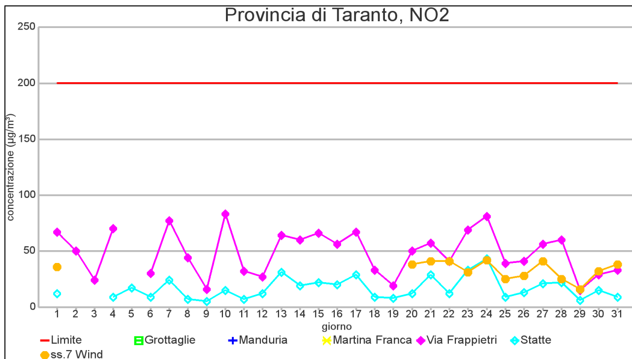
GRAFICO 2.2: Valore massimo giornaliero – mese di DICEMBRE 2012 – Provincia di Taranto
