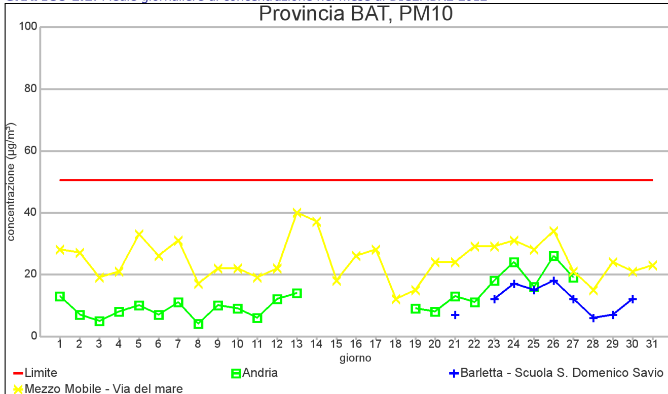
GRAFICO 1.1: Medie giornaliere di concentrazione nel mese di DICEMBRE 2012
