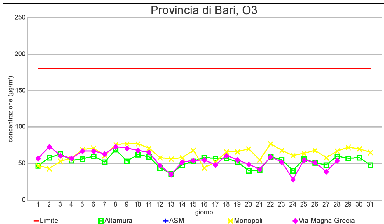
GRAFICO 3.2 PROVINCIA DI BARI: massimo orario –DICEMBRE 2012
