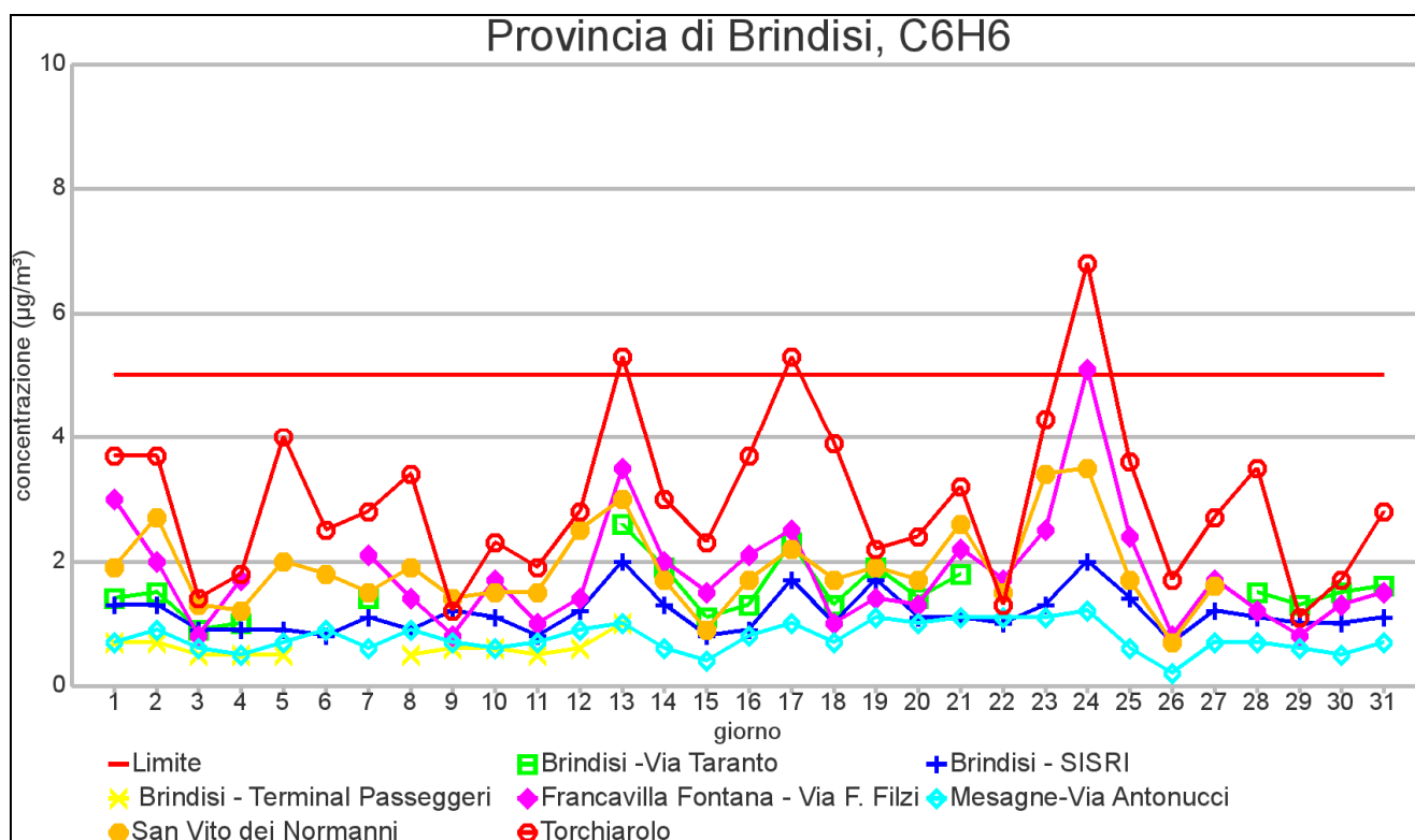
GRAFICO 5.1: Medie giornaliere di concentrazione nel mese di DICEMBRE 2012 (µg/m 3 )
