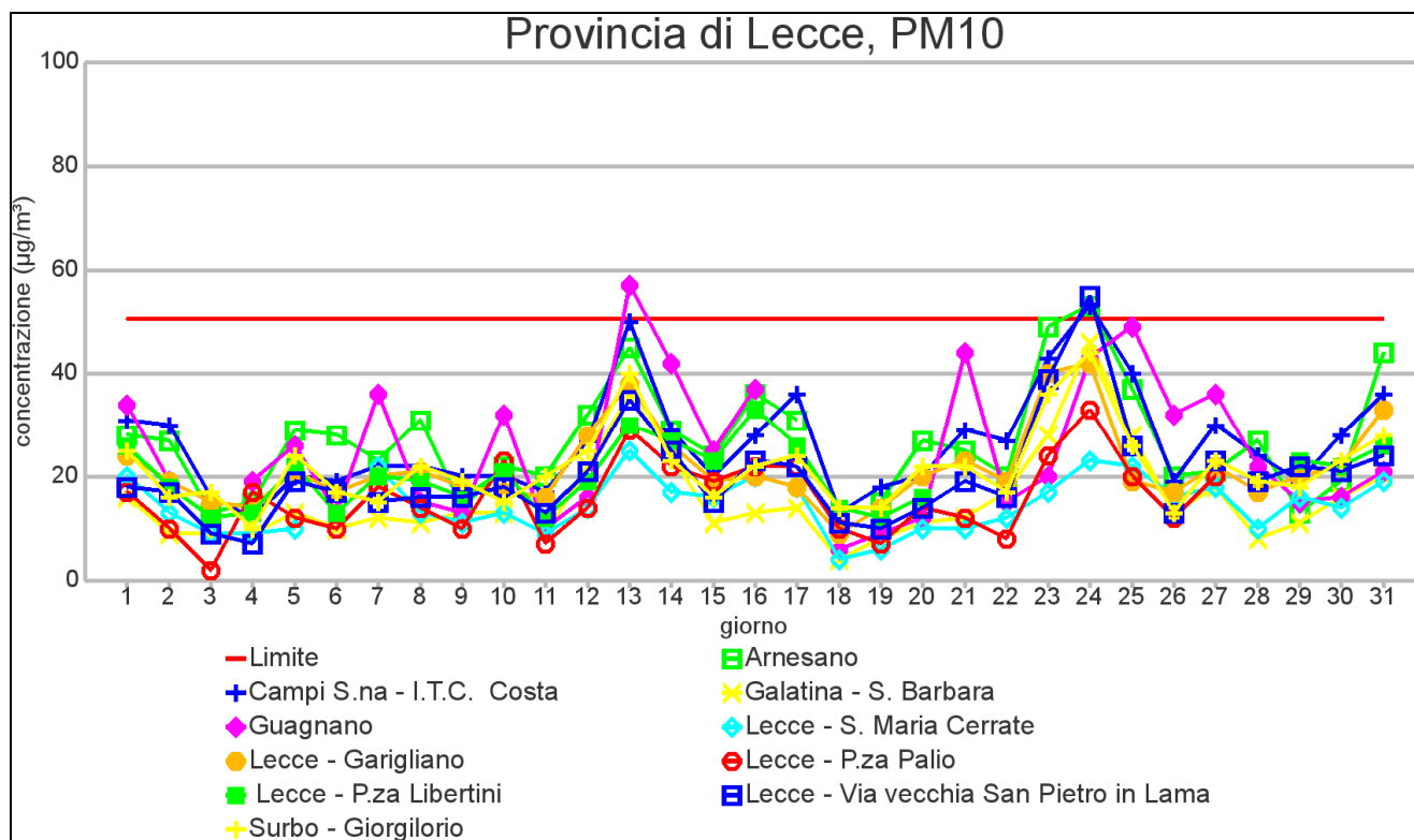
GRAFICO 1.1: Medie giornaliere di concentrazione nel mese di DICEMBRE 2012
