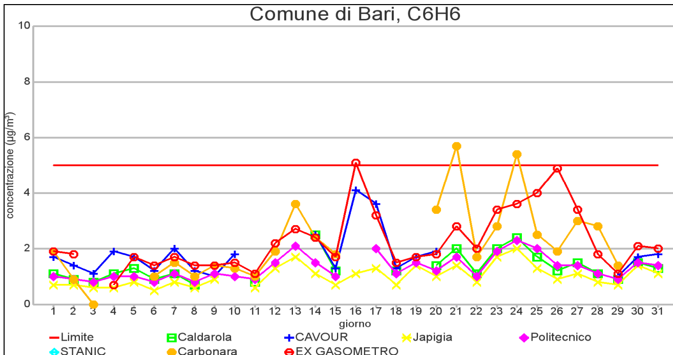
GRAFICO 4.2 PROVINCIA DI BARI: Medie giornaliere di concentrazione Benzene – mese di DICEMBRE 2012
