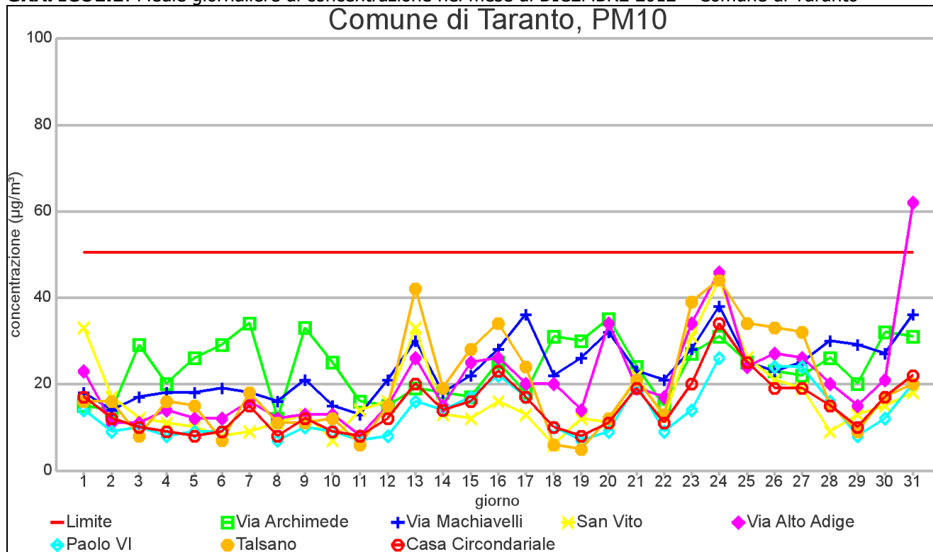
GRAFICO1.1: Medie giornaliere di concentrazione nel mese di DICEMBRE 2012 – Comune di Taranto
