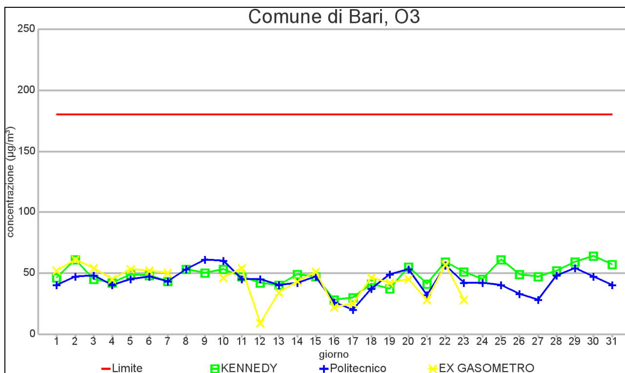
GRAFICO 3.1 COMUNE DI BARI: massimo orario – DICEMBRE 2012
