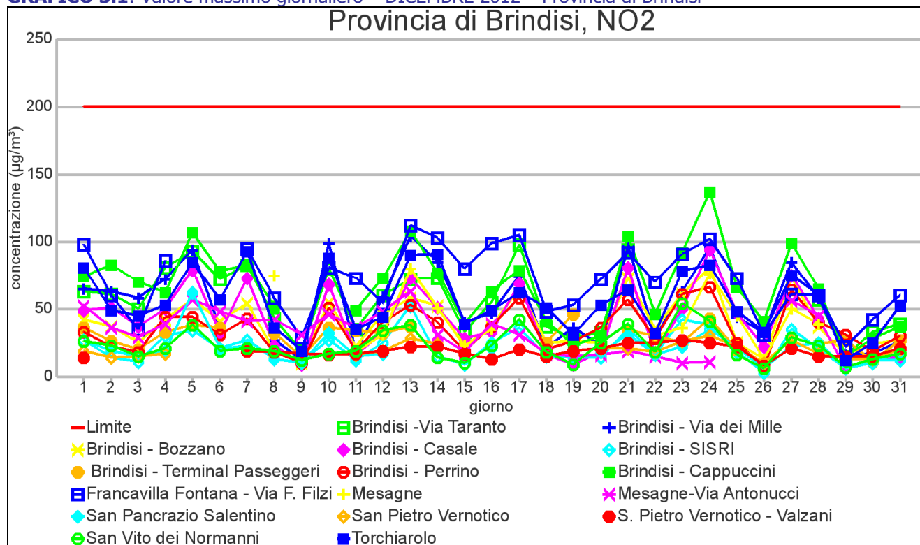
GRAFICO 3.1: Valore massimo giornaliero – DICEMBRE 2012 – Provincia di Brindisi
