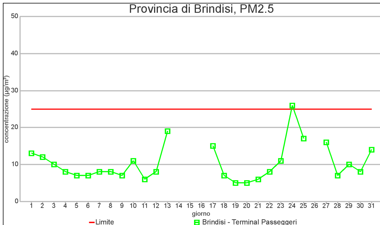
GRAFICO 2.1: Medie giornaliere di concentrazione nel mese di DICEMBRE 2012
