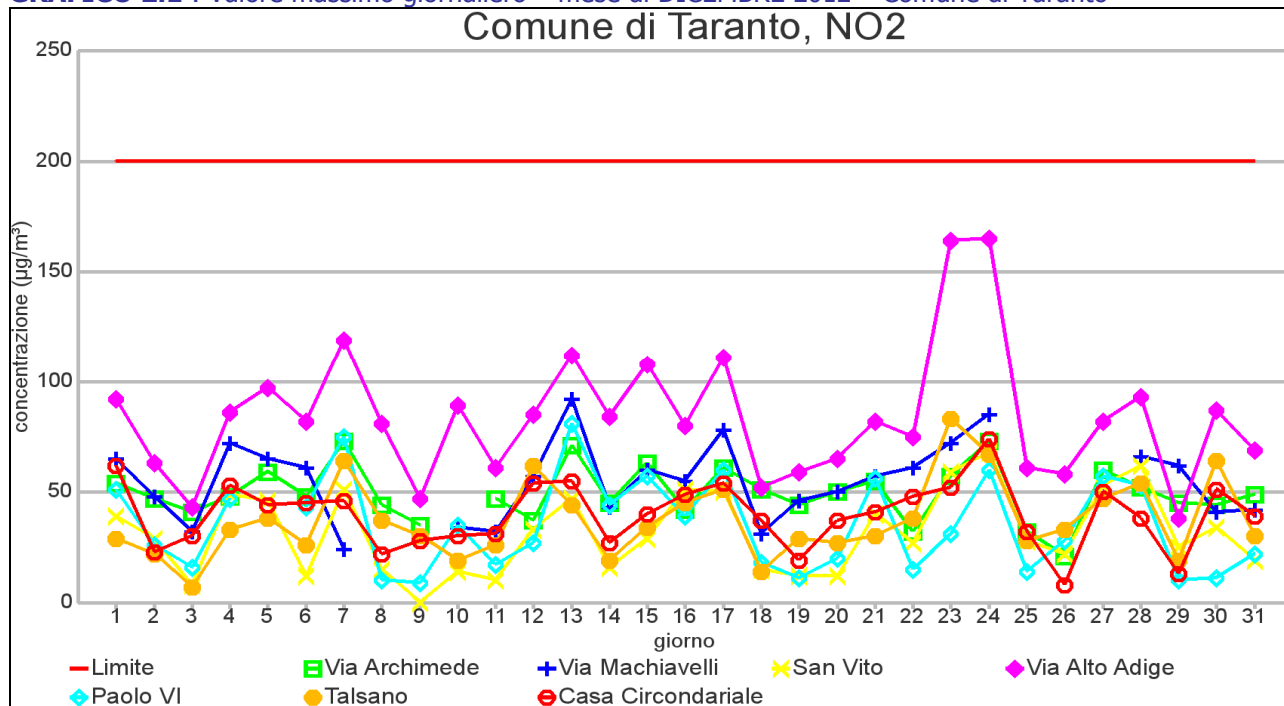
GRAFICO 2.1 : Valore massimo giornaliero – mese di DICEMBRE 2012 – Comune di Taranto
