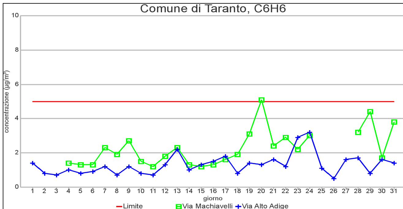
GRAFICO 5.1: Medie giornaliere di concentrazione nel mese di DICEMBRE 2012 – Comune di Taranto
