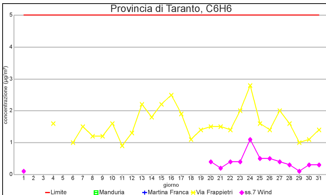
GRAFICO 5.1: Medie giornaliere di concentrazione nel mese di DICEMBRE 2012 – Provincia di Taranto
