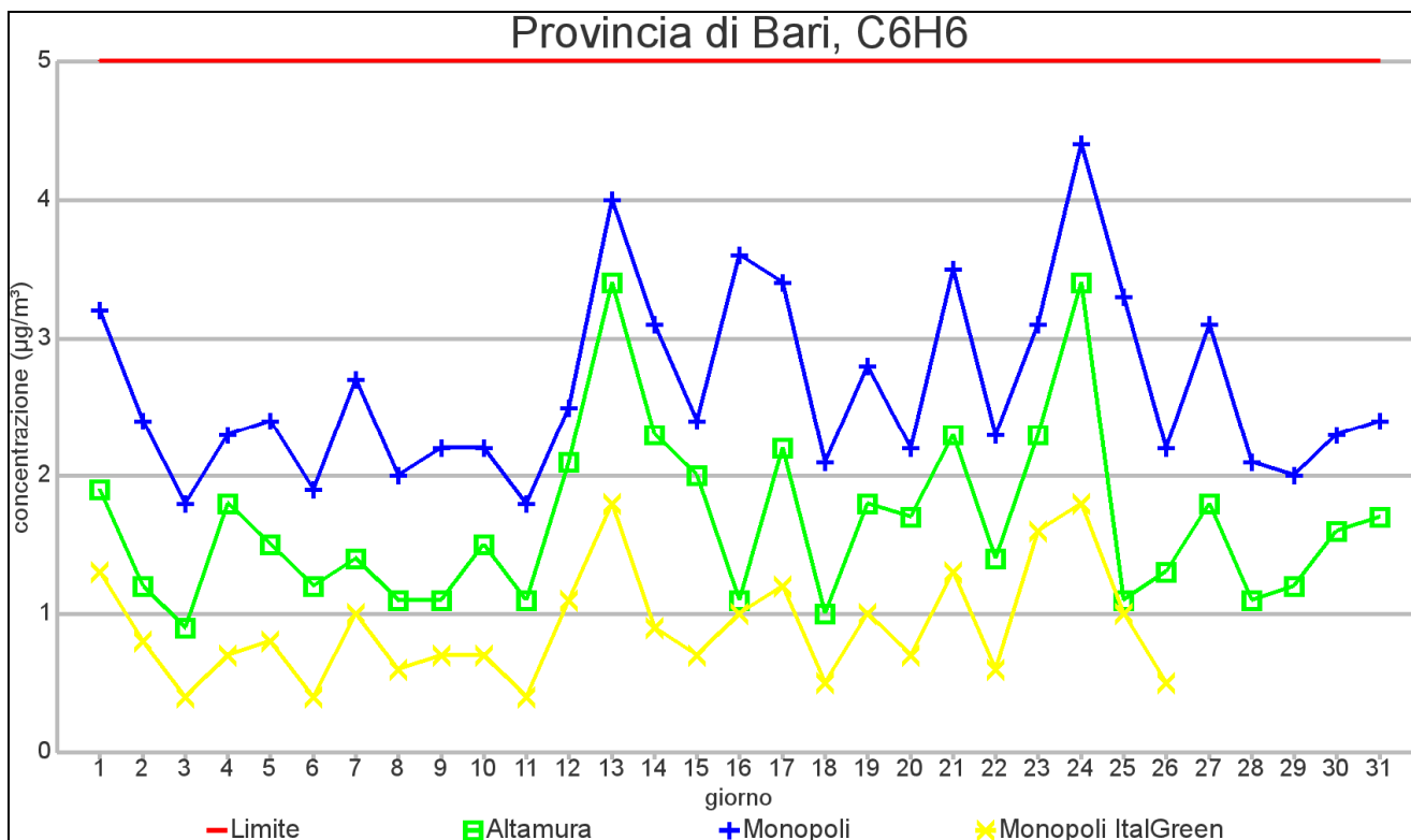
GRAFICO 4.2 PROVINCIA DI BARI: Medie giornaliere di concentrazione Benzene – mese di DICEMBRE 2012
