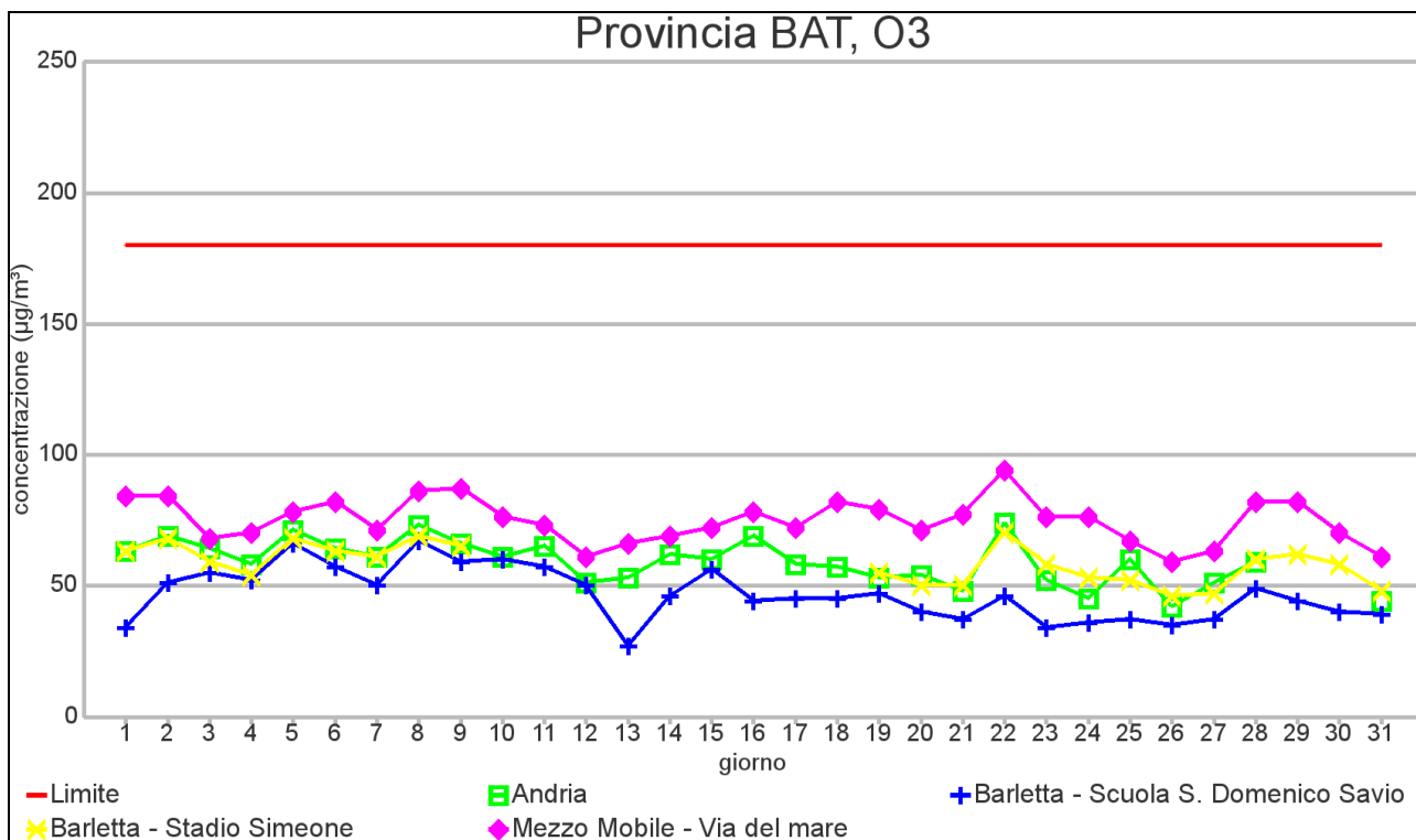
GRAFICO 3.1: massimo orario di O 3 –DICEMBRE 2012
