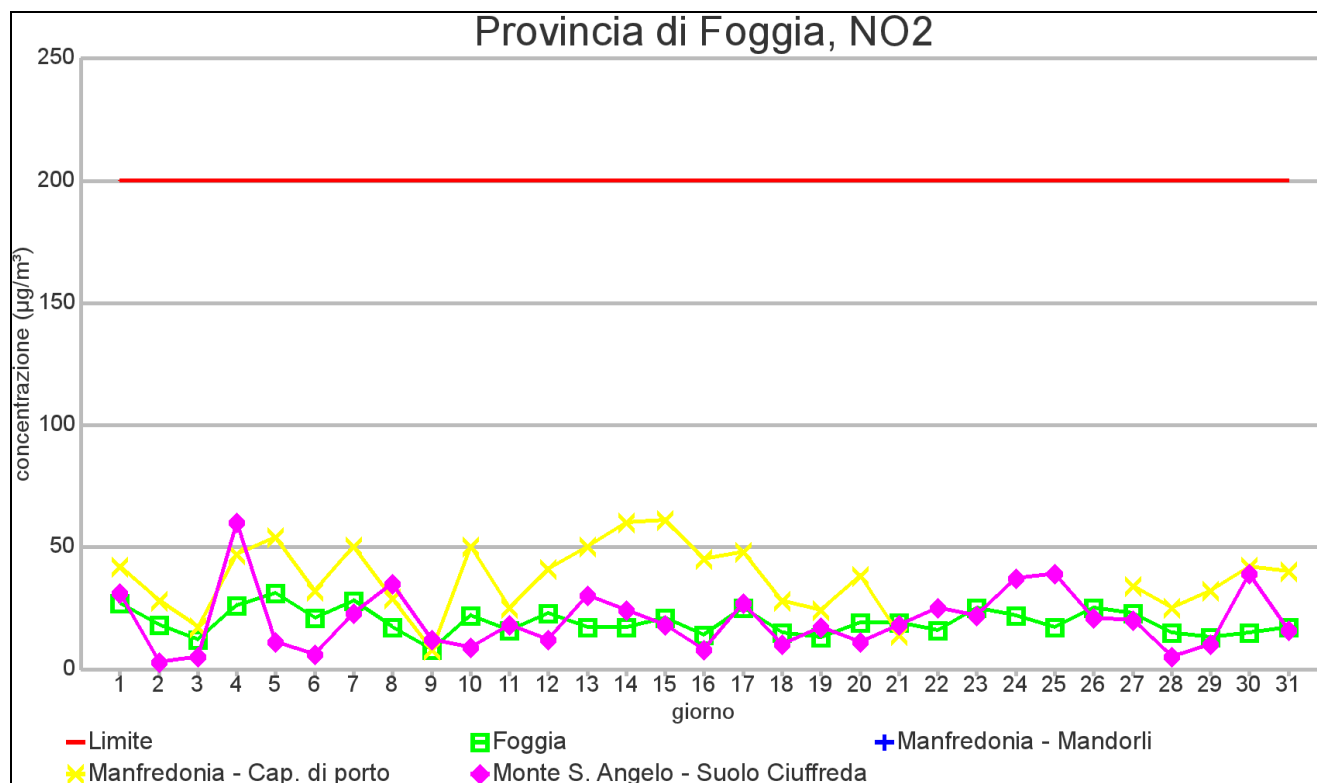
GRAFICO 2.1: Valore massimo orario – mese di DICEMBRE 2012
