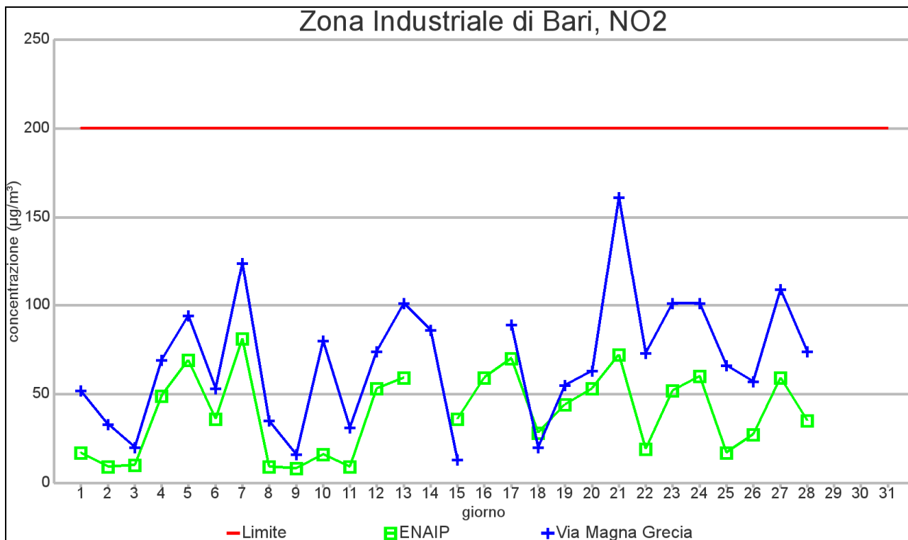
GRAFICO 2.2 AREA INDUSTRIALE BARI: Valore massimo orario NO 2 – DICEMBRE 2012
