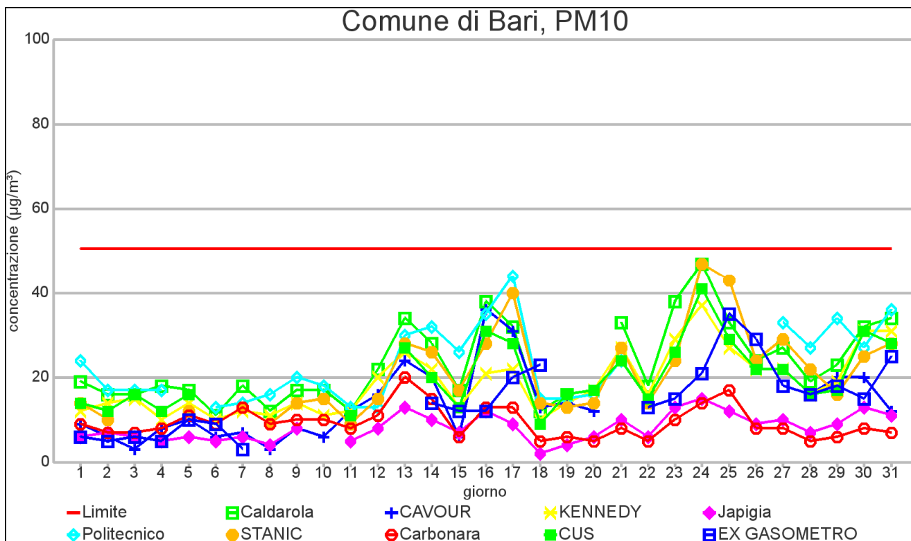
GRAFICO 1.1 COMUNE di BARI: Valori medi giornalieri di concentrazione PM10- mese di DICEMBRE 2012
