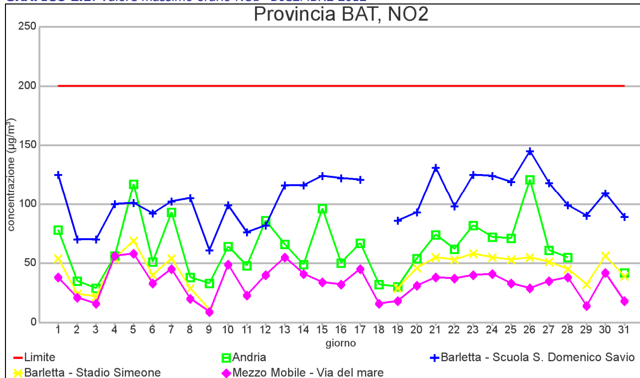
GRAFICO 2.1: Valore massimo orario NO 2 – DICEMBRE 2012
