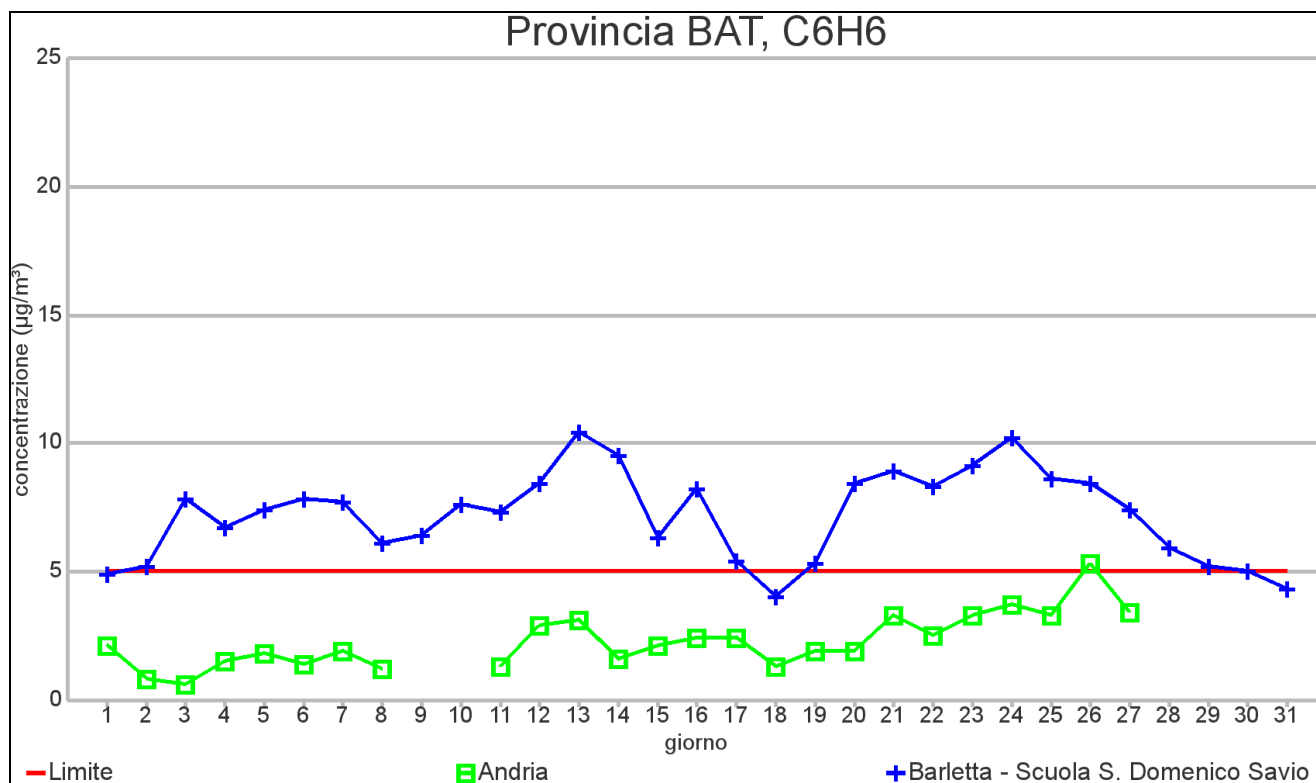
GRAFICO 4.1: Medie giornaliere di concentrazione nel mese di DICEMBRE 2012
