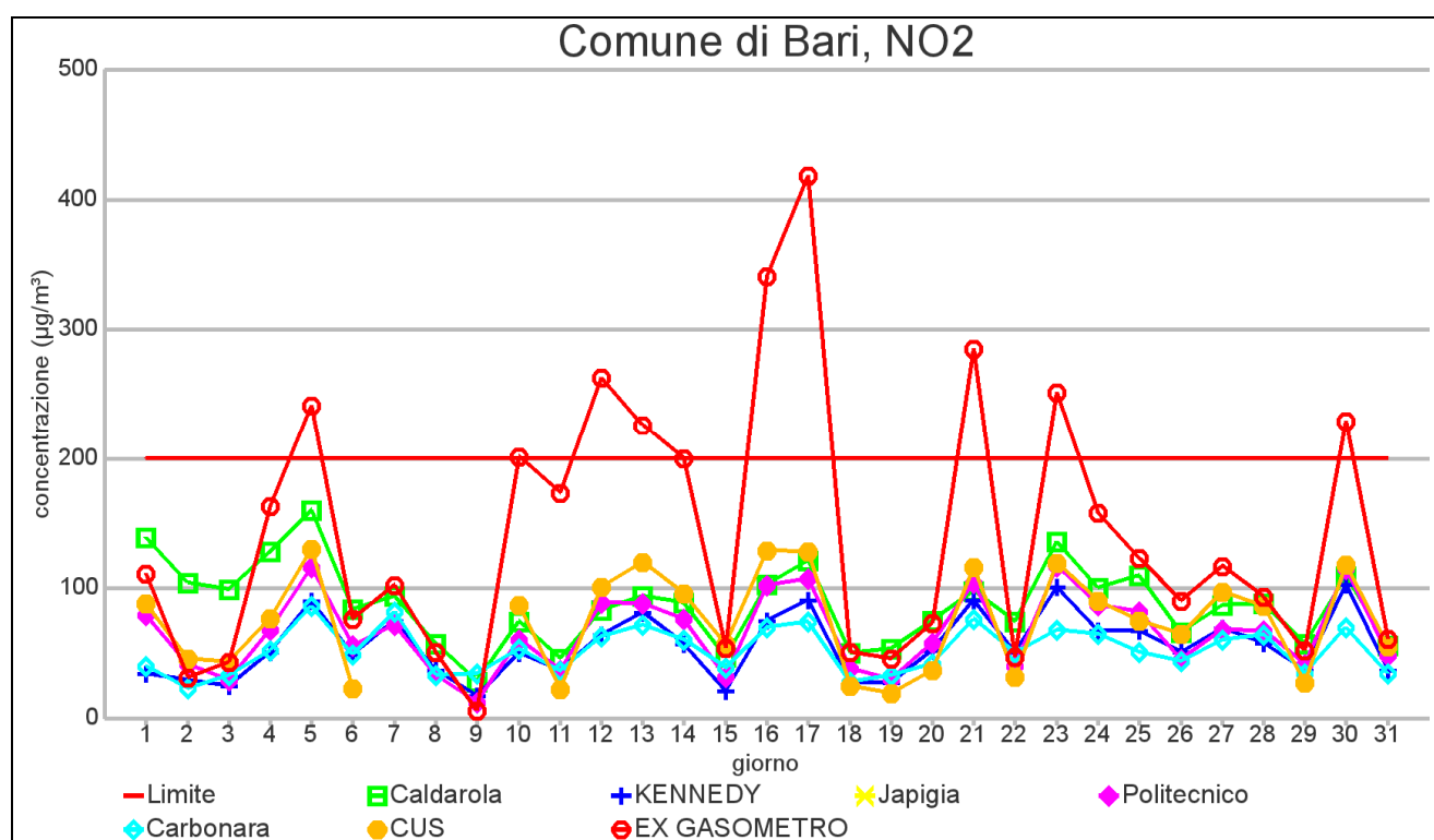
GRAFICO 2.1 COMUNE DI BARI: Valore massimo orario NO 2 – DICEMBRE 2012
