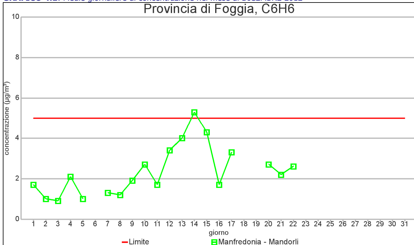
GRAFICO 4.1: Medie giornaliere di concentrazione nel mese di DICEMBRE 2012
