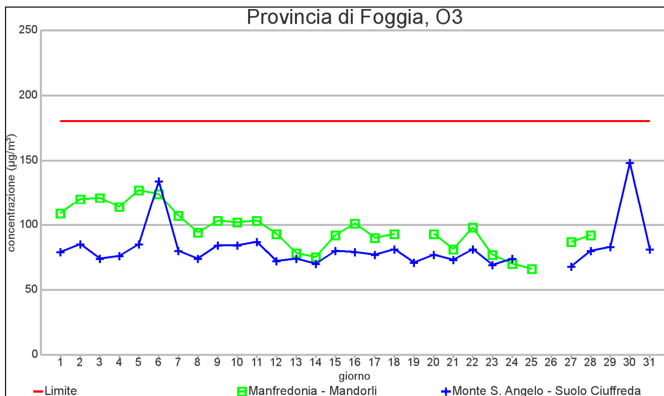
GRAFICO 3.1: massimo orario di O 3 – DICEMBRE 2012
