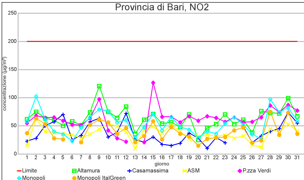
GRAFICO 2.3 PROVINCIA DI BARI: Valore massimo orario NO 2 – GENNAIO 2013
