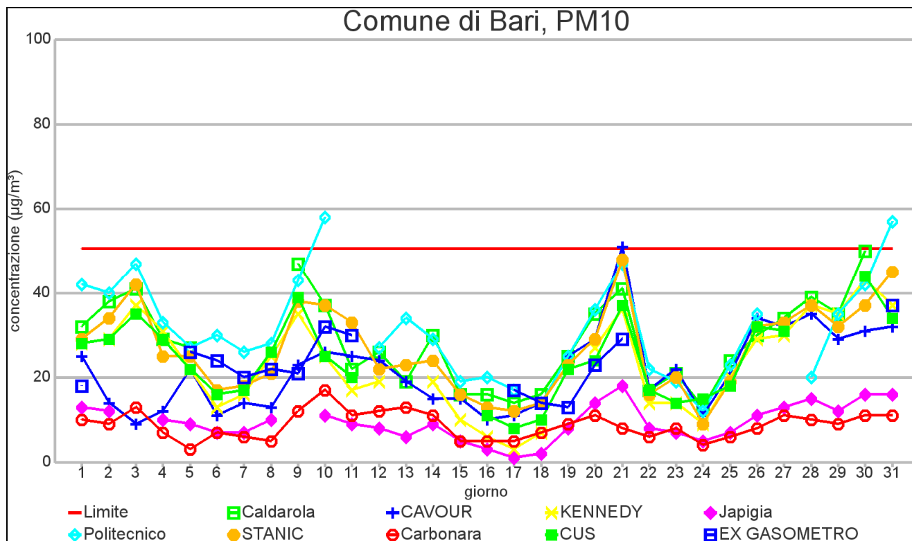
GRAFICO 1.1 COMUNE di BARI: Valori medi giornalieri di concentrazione PM10- mese di GENNAIO 2013
