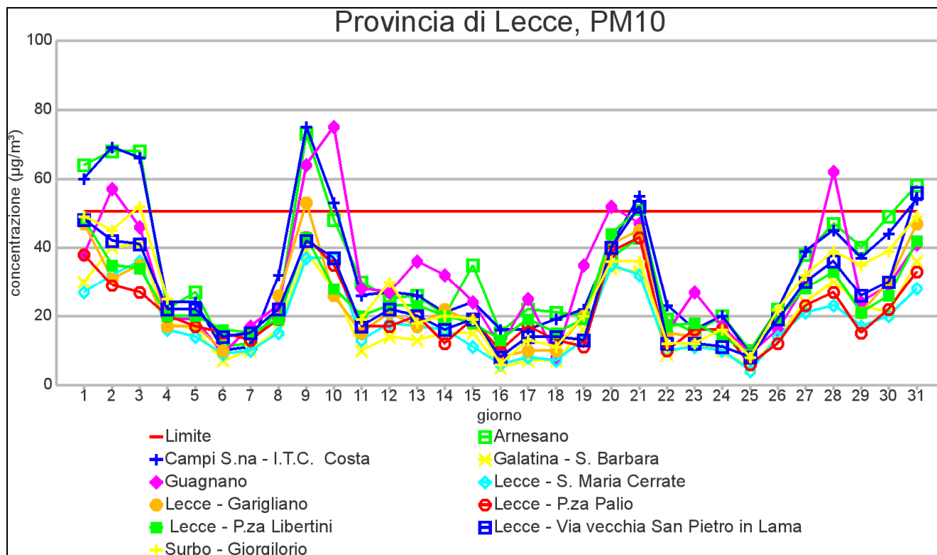
GRAFICO 1.1: Medie giornaliere di concentrazione nel mese di GENNAIO 2013
