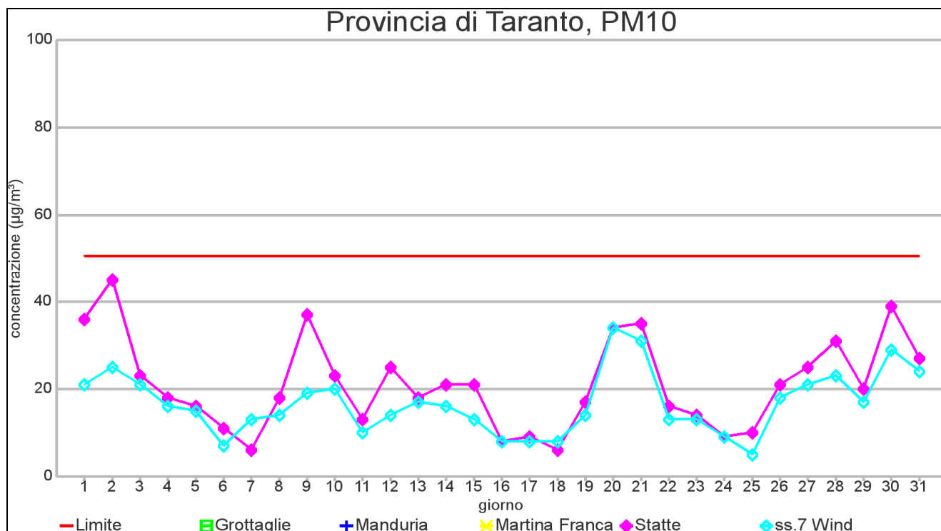
GRAFICO 1.2: Medie giornaliere di concentrazione nel mese di GENNAIO 2013 – Provincia di Taranto
