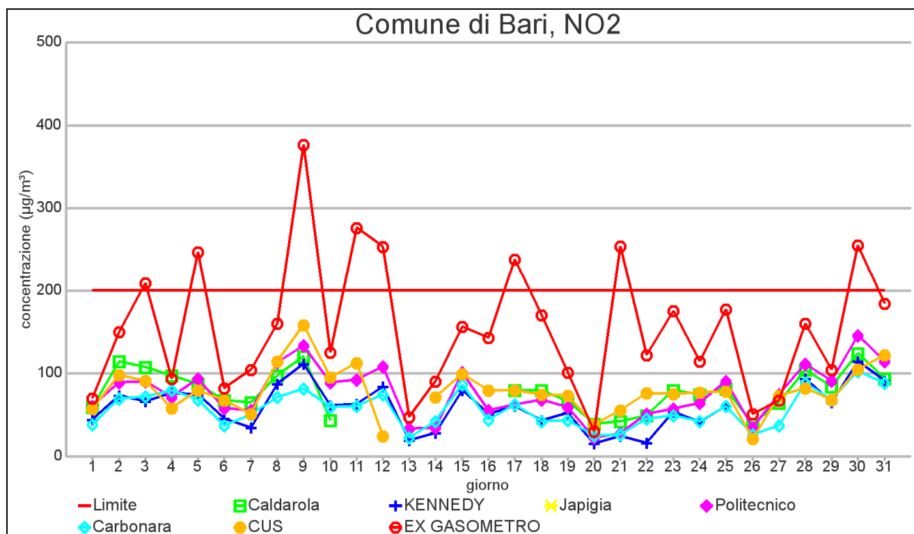
GRAFICO 2.1 COMUNE DI BARI: Valore massimo orario NO 2 – GENNAIO 2013
