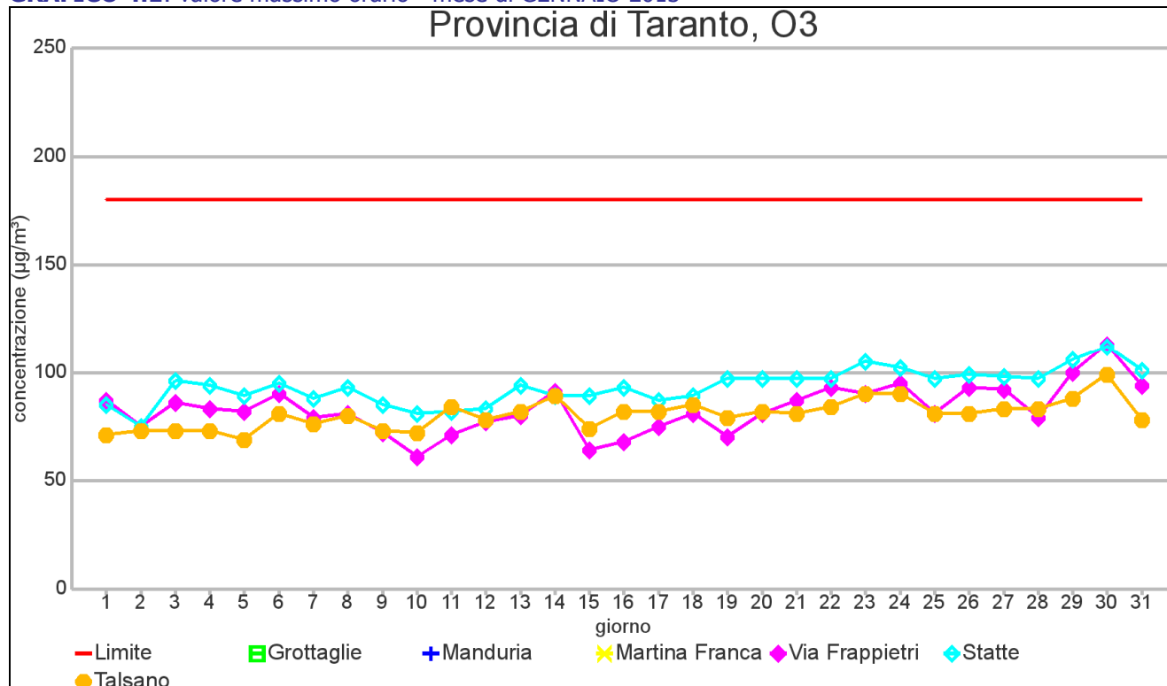
GRAFICO 4.1: valore massimo orario - mese di GENNAIO 2013
