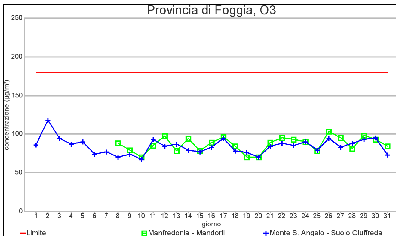
GRAFICO 3.1: massimo orario di O 3 – GENNAIO 2013
