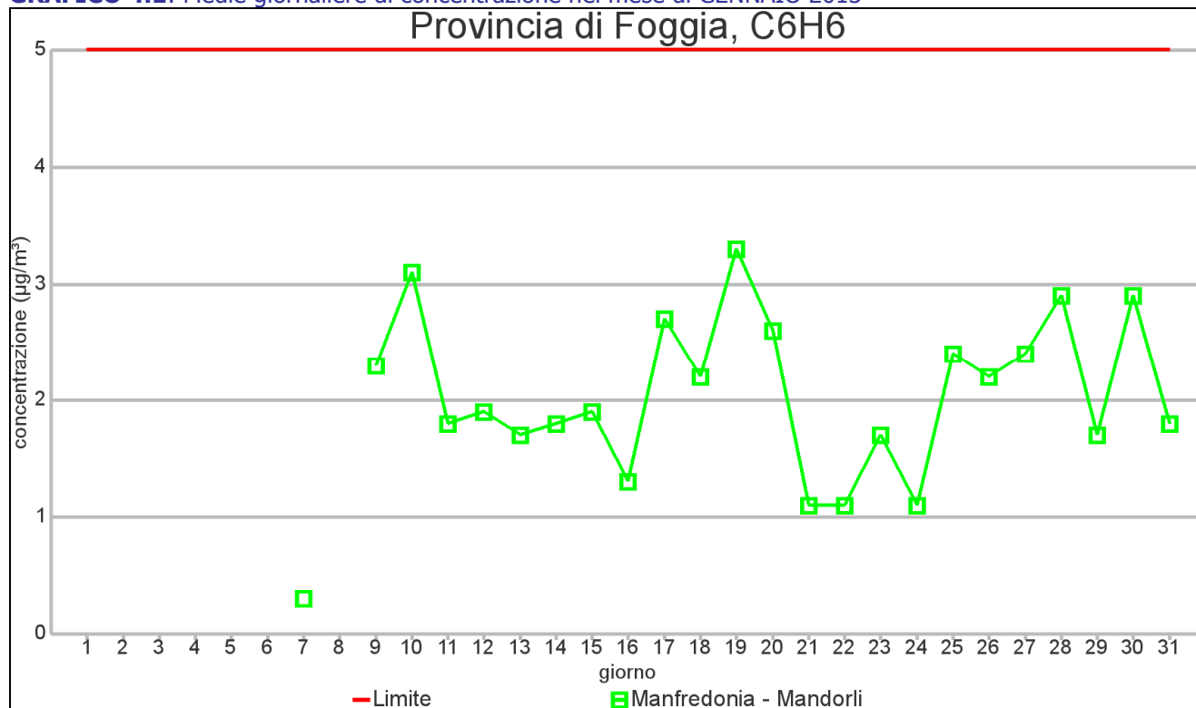
GRAFICO 4.1: Medie giornaliere di concentrazione nel mese di GENNAIO 2013
