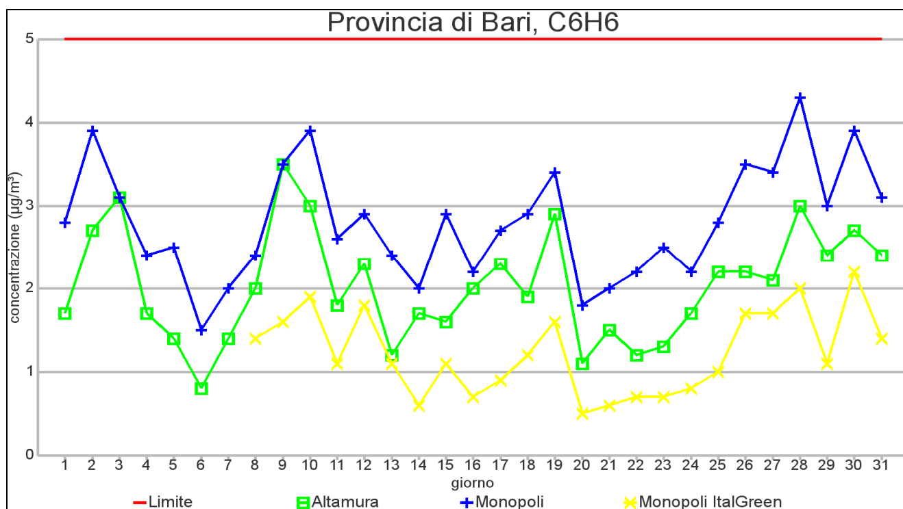
GRAFICO 4.2 PROVINCIA DI BARI: Medie giornaliere di concentrazione Benzene – mese di GENNAIO 2013
