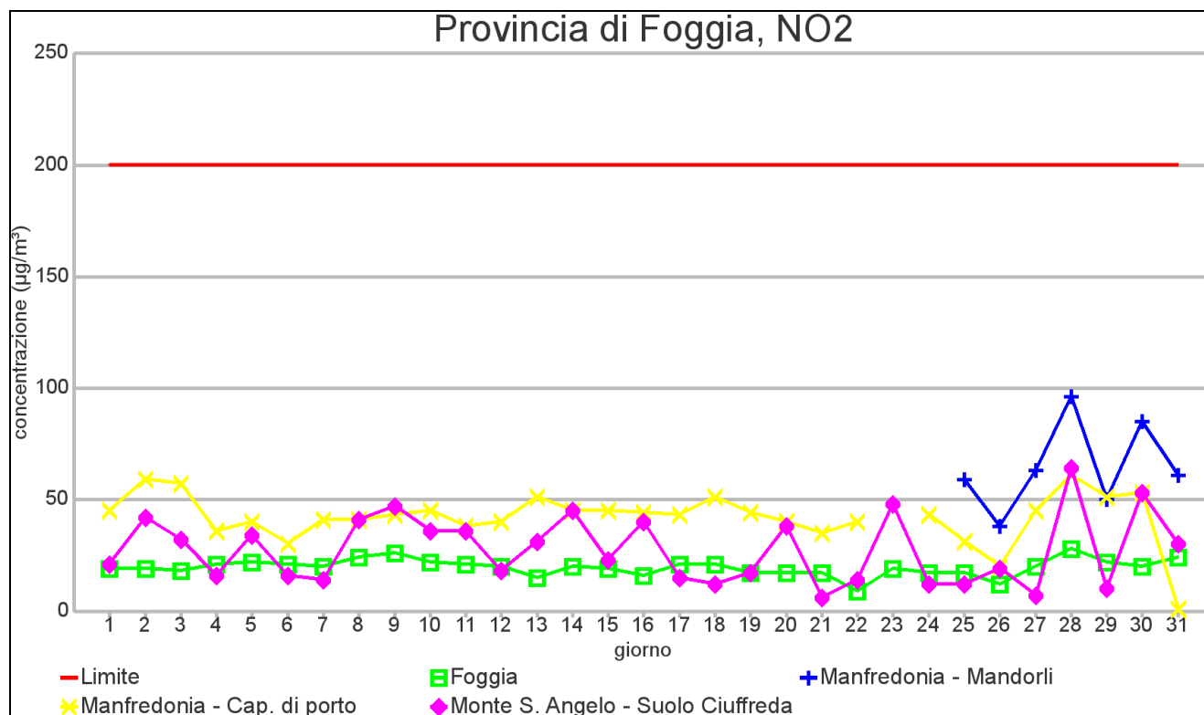
GRAFICO 2.1: Valore massimo orario – mese di GENNAIO 2013
