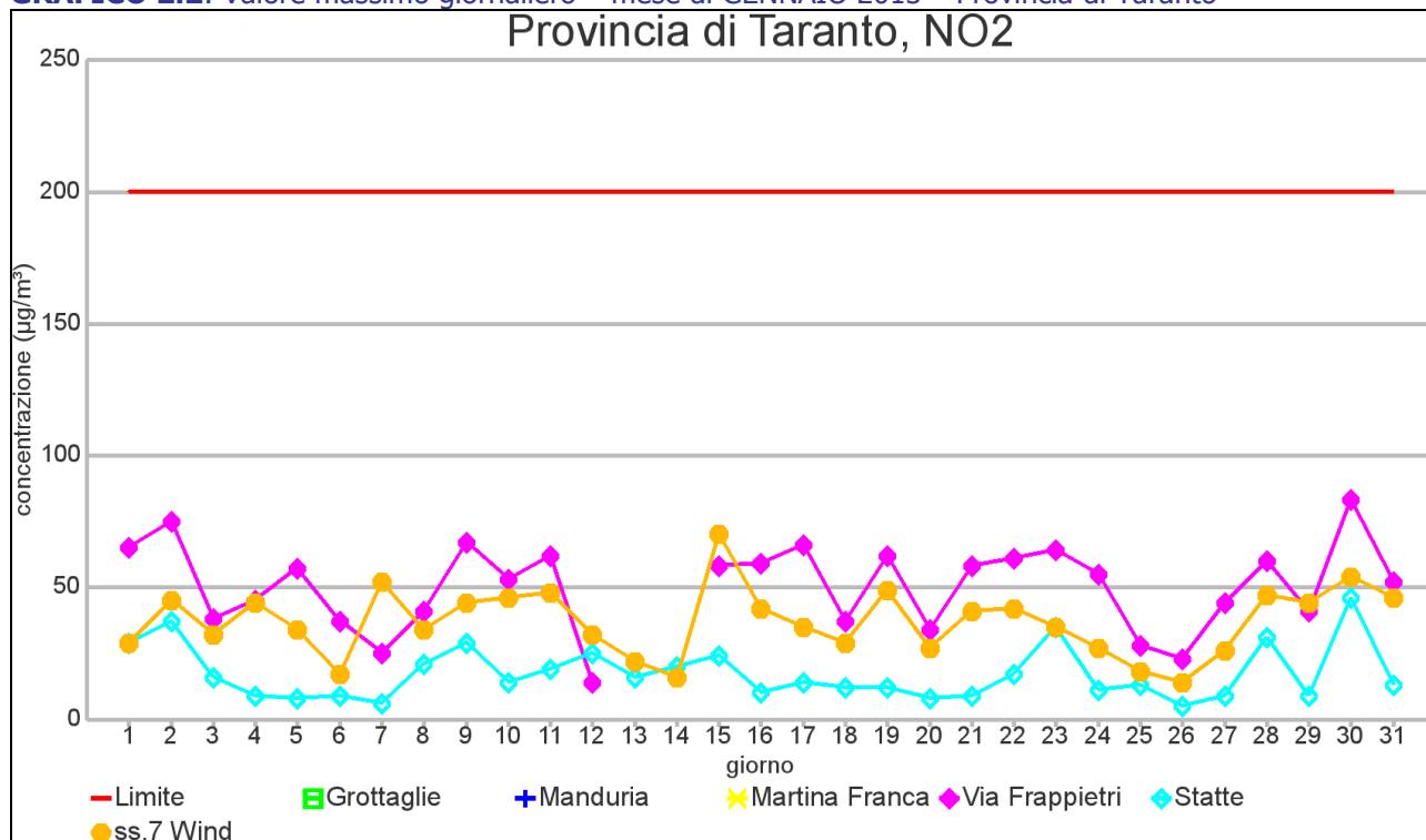
GRAFICO 2.2: Valore massimo giornaliero – mese di GENNAIO 2013 – Provincia di Taranto
