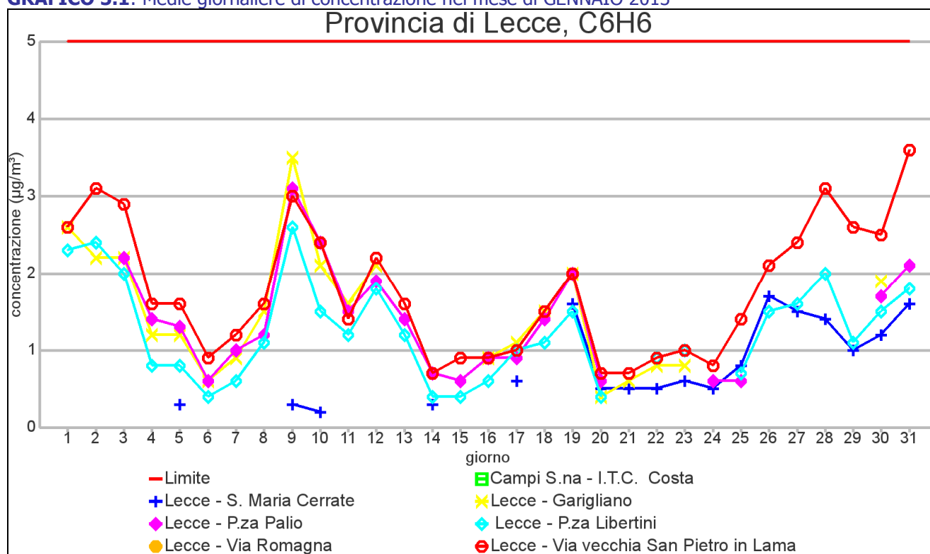
GRAFICO 5.1: Medie giornaliere di concentrazione nel mese di GENNAIO 2013
