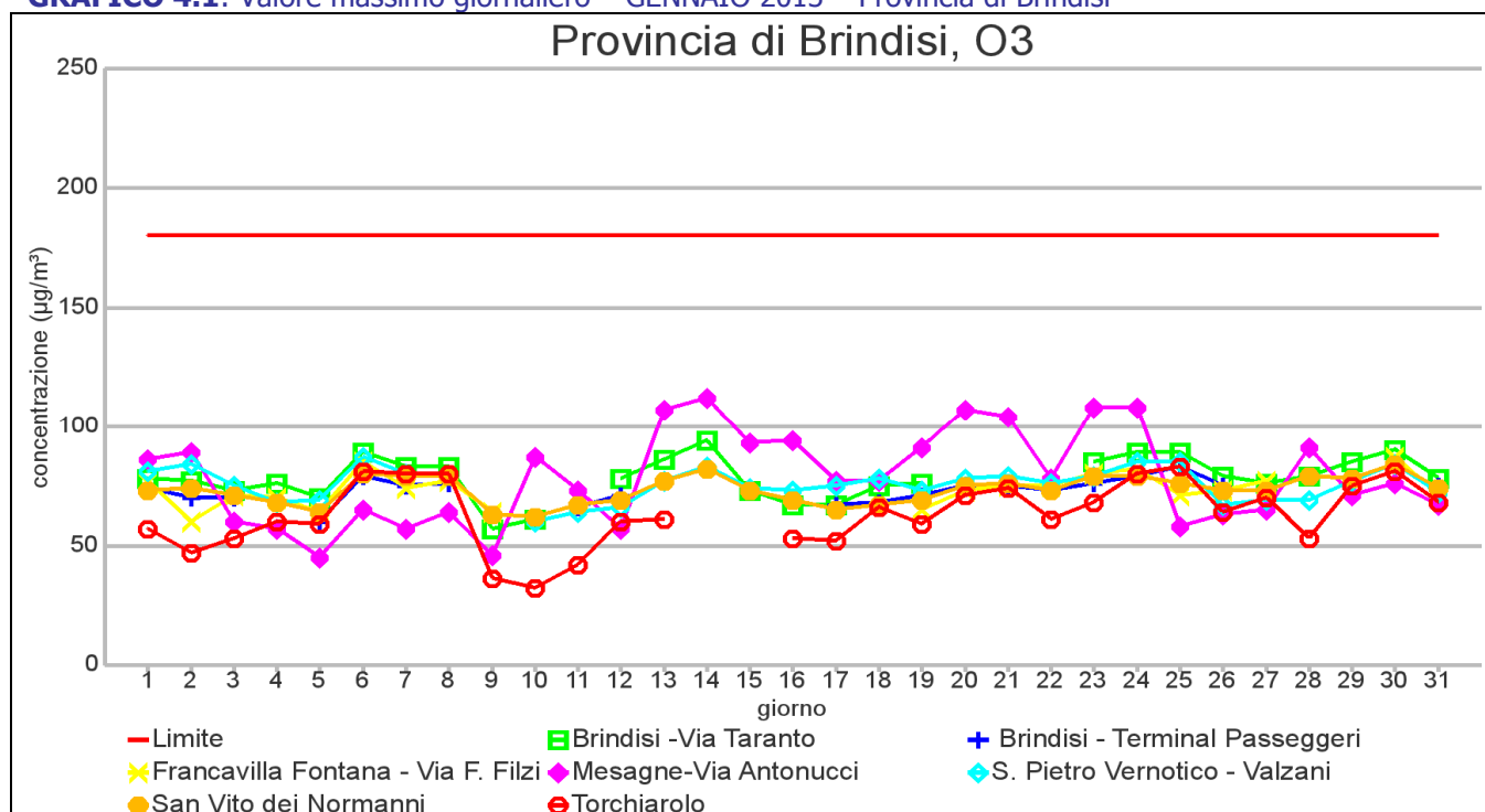
GRAFICO 4.1: Valore massimo giornaliero – GENNAIO 2013 – Provincia di Brindisi
