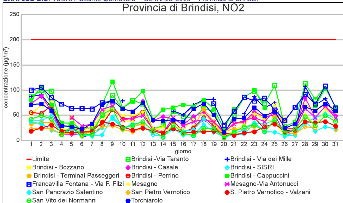
GRAFICO 3.1: Valore massimo giornaliero – GENNAIO 2013 – Provincia di Brindisi
