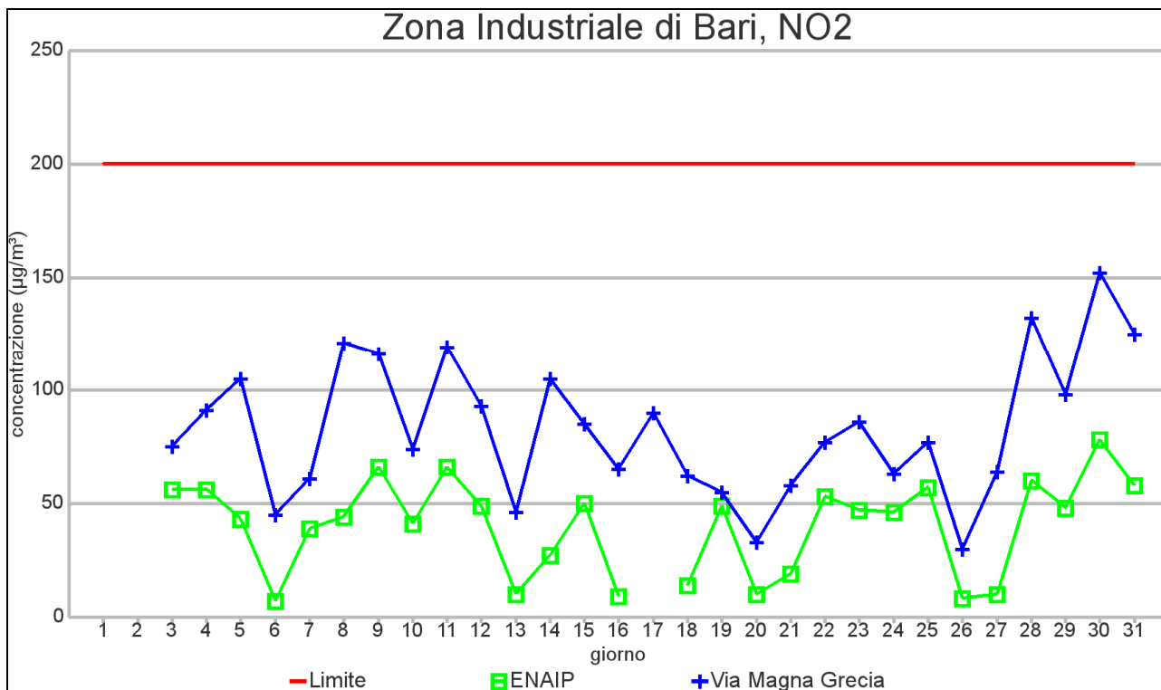
GRAFICO 2.2 AREA INDUSTRIALE BARI: Valore massimo orario NO 2 – GENNAIO 2013
