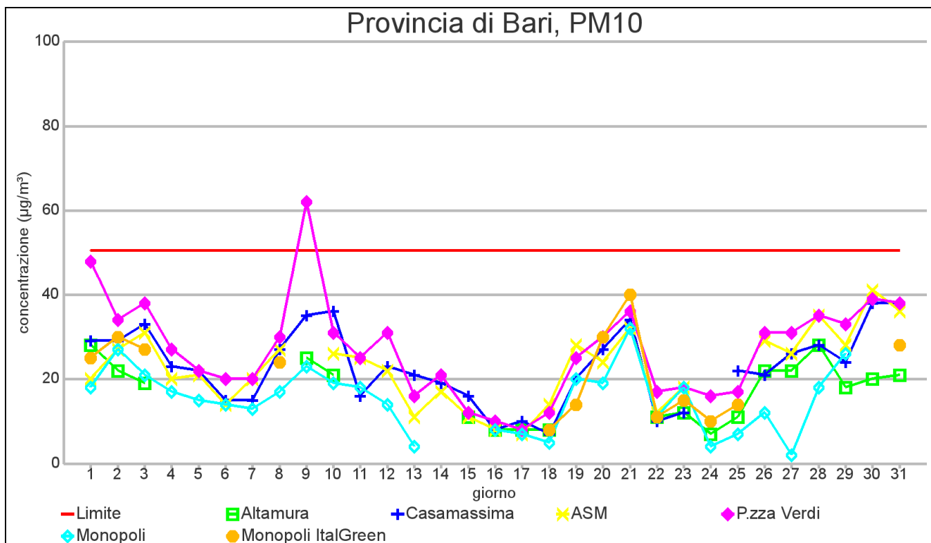
GRAFICO 1.3 PROVINCIA DI BARI: Valori medi giornalieri di concentrazione PM10 – GENNAIO 2013
