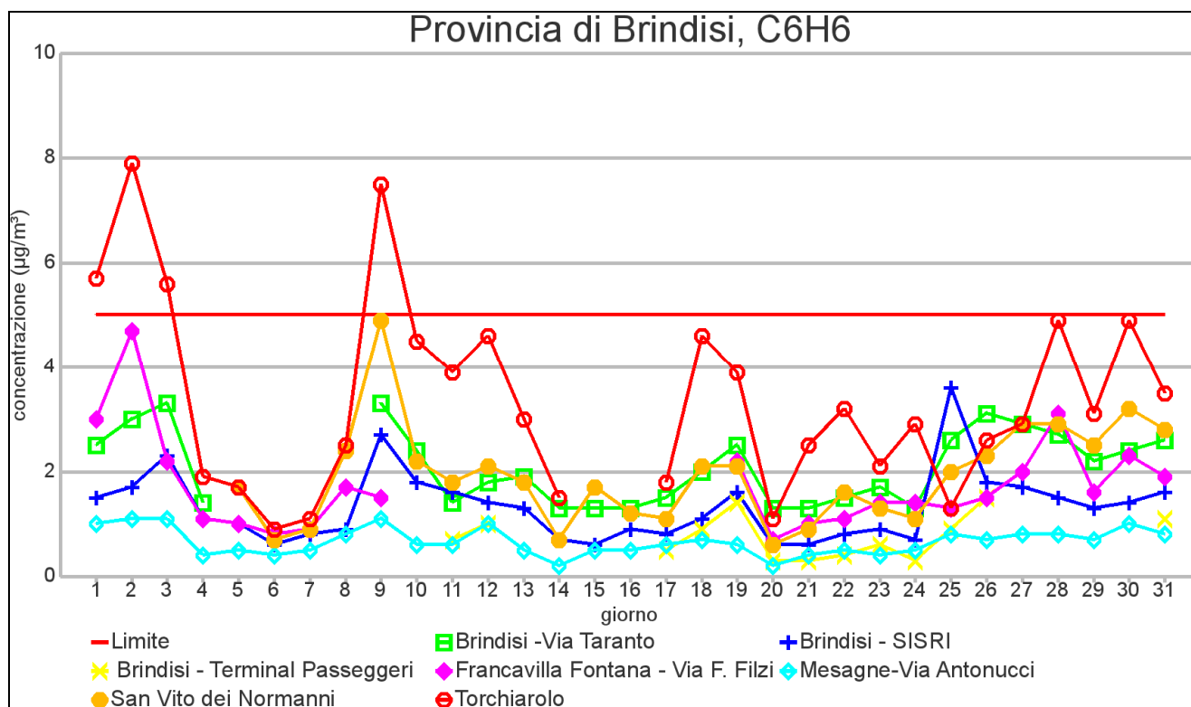
GRAFICO 5.1: Medie giornaliere di concentrazione nel mese di GENNAIO 2013 (µg/m 3 )
