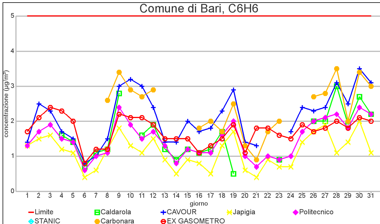
GRAFICO 4.2 PROVINCIA DI BARI: Medie giornaliere di concentrazione Benzene – mese di GENNAIO 2013
