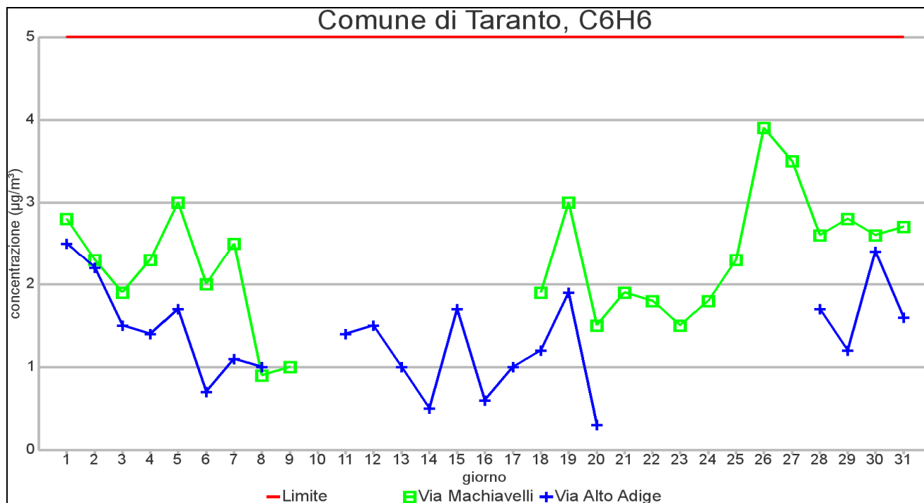
GRAFICO 5.1: Medie giornaliere di concentrazione nel mese di GENNAIO 2013 – Comune di Taranto
