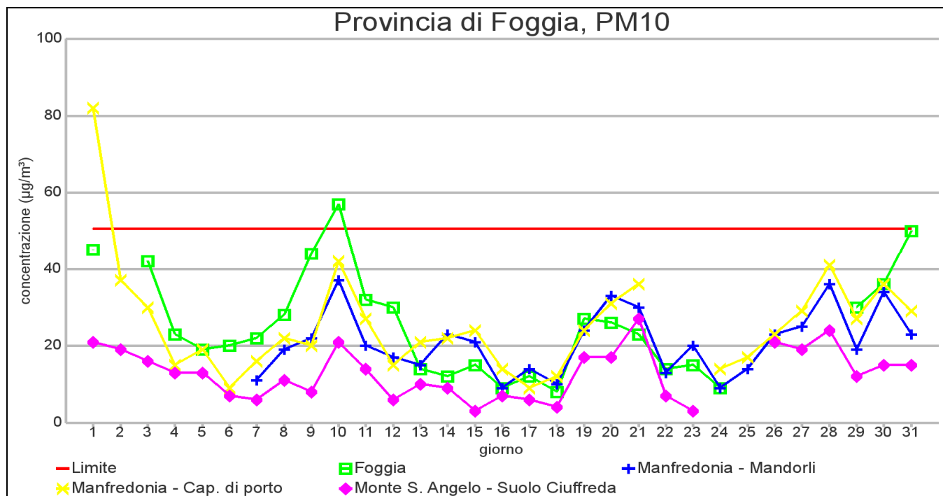
GRAFICO 1.1: Medie giornaliere di concentrazione nel mese di GENNAIO 2013
