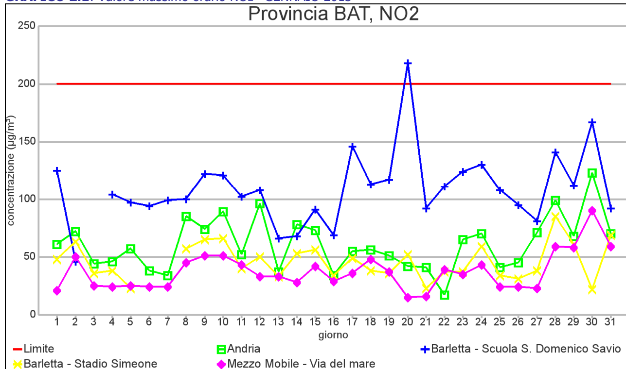
GRAFICO 2.1: Valore massimo orario NO 2 – GENNAIO 2013
