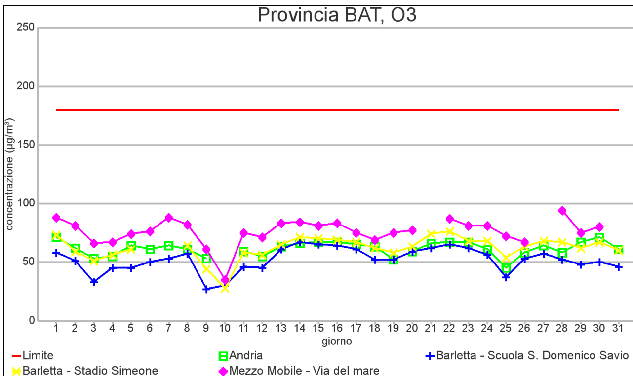
GRAFICO 3.1: massimo orario di O 3 –GENNAIO 2013
