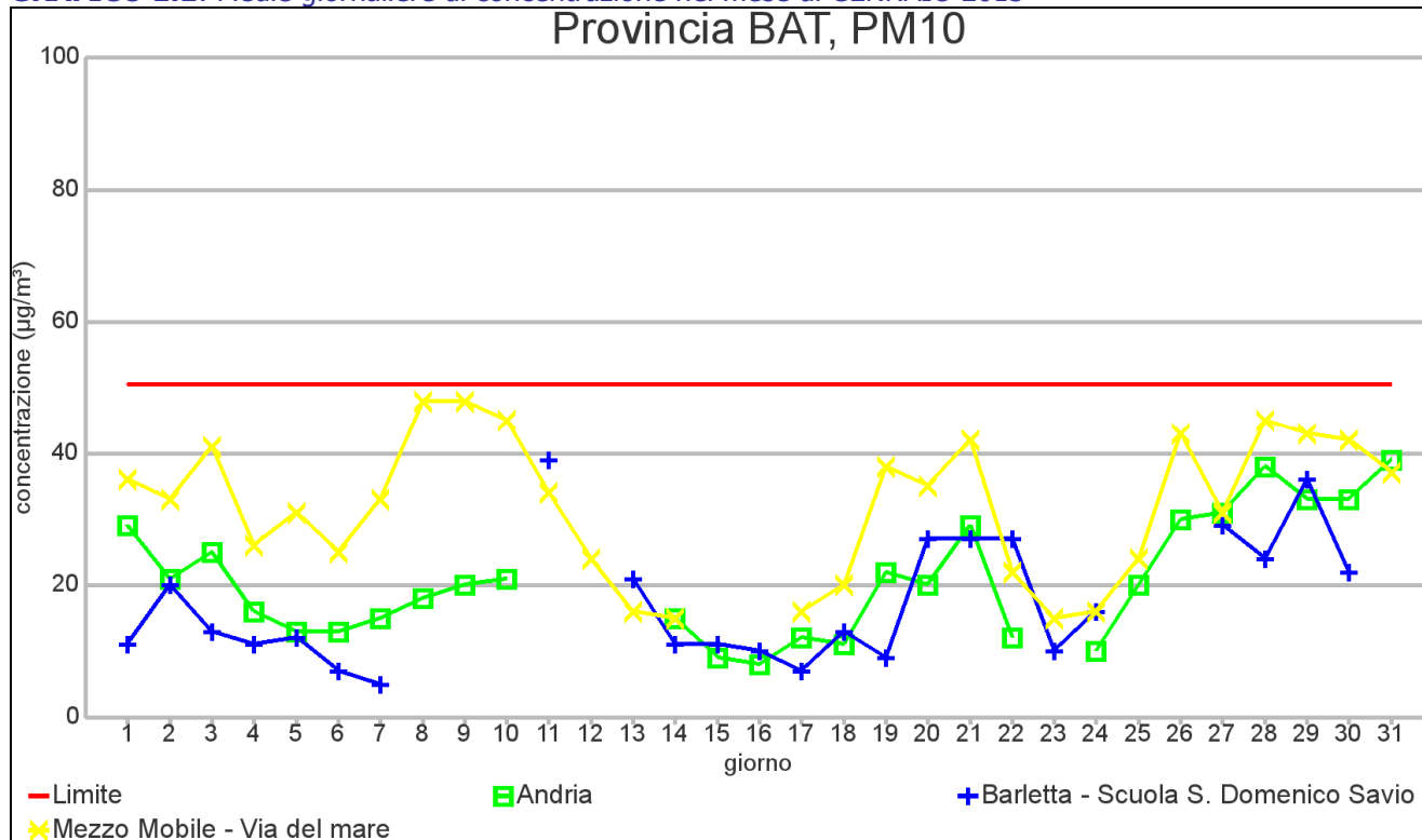
GRAFICO 1.1: Medie giornaliere di concentrazione nel mese di GENNAIO 2013
