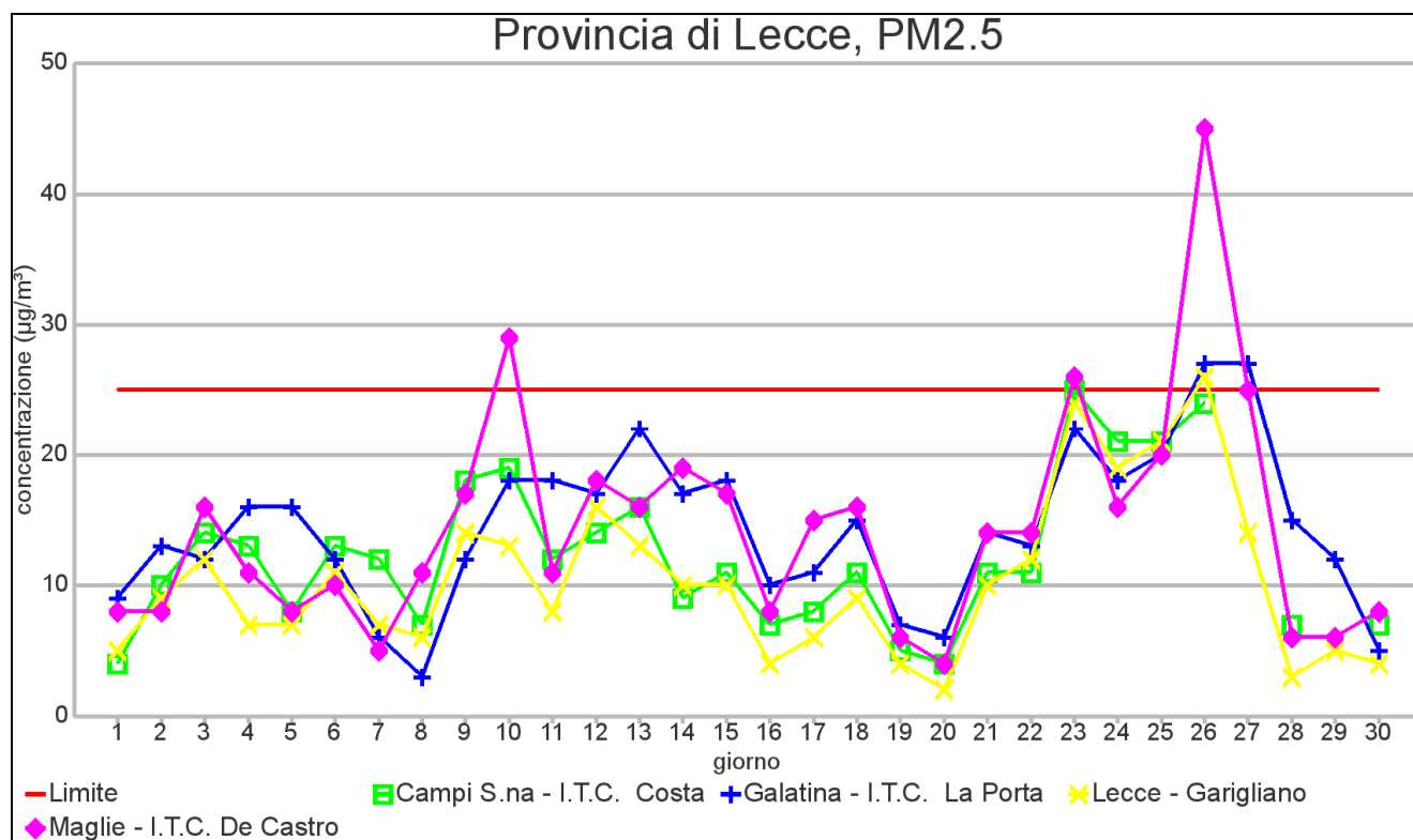
GRAFICO 2.1: Medie giornaliere di concentrazione nel mese di NOVEMBRE 2012
