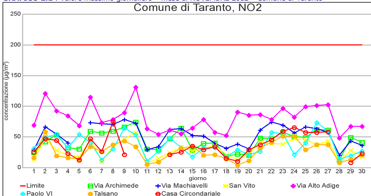
GRAFICO 2.1 : Valore massimo giornaliero – mese di NOVEMBRE 2012 – Comune di Taranto
