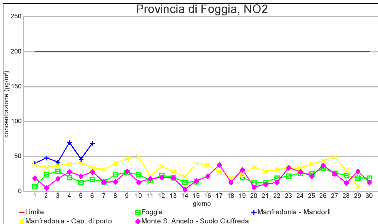
GRAFICO 2.1: Valore massimo orario – mese di NOVEMBRE 2012
