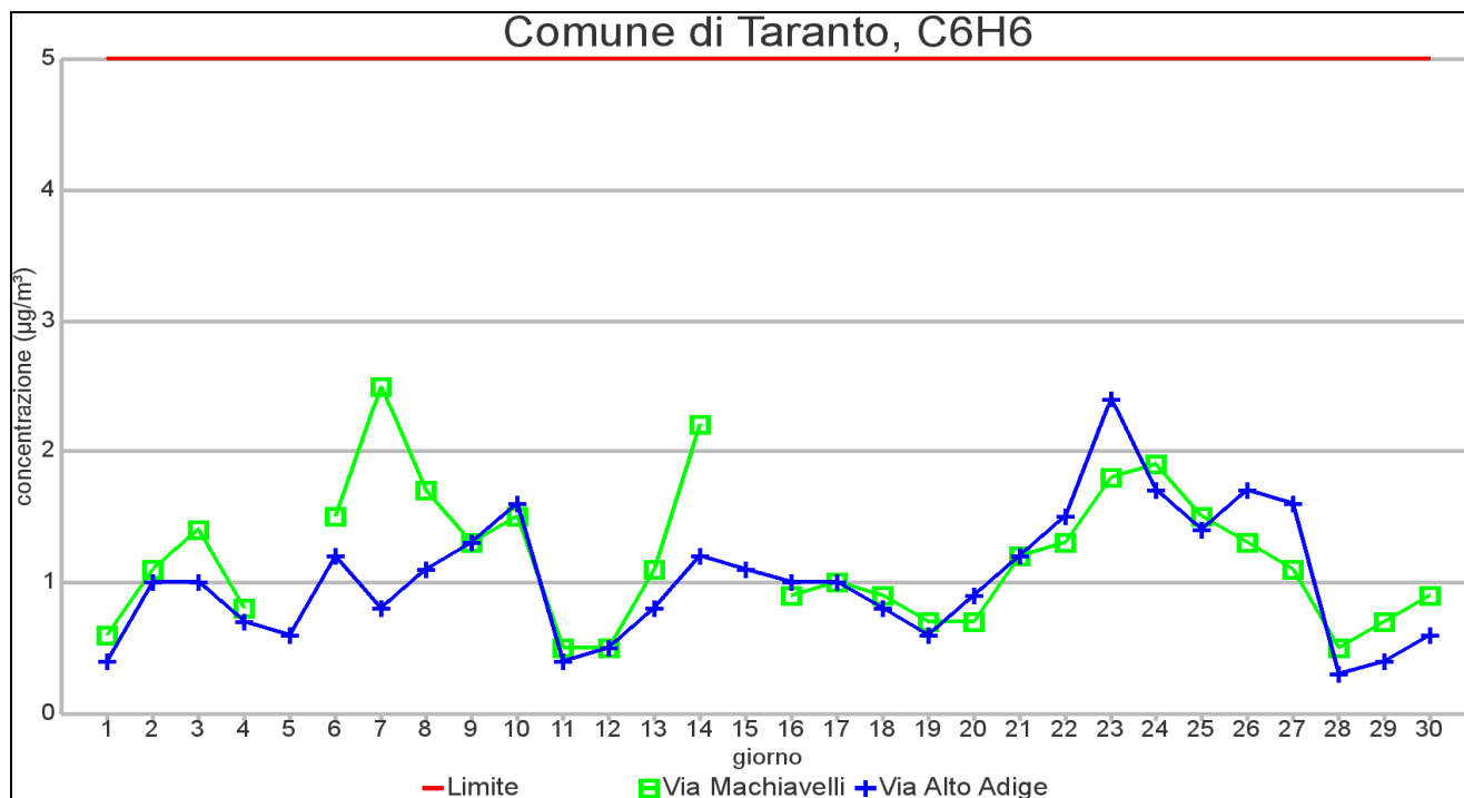
GRAFICO 5.1: Medie giornaliere di concentrazione nel mese di NOVEMBRE 2012 – Comune di Taranto
