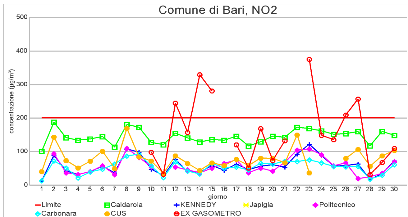
GRAFICO 2.1 COMUNE DI BARI: Valore massimo orario NO 2 – NOVEMBRE 2012
