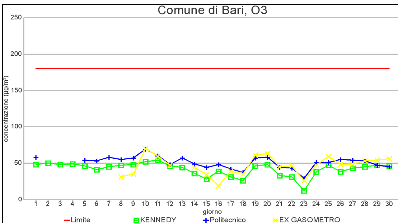
GRAFICO 3.1 COMUNE DI BARI: massimo orario – NOVEMBRE 2012
