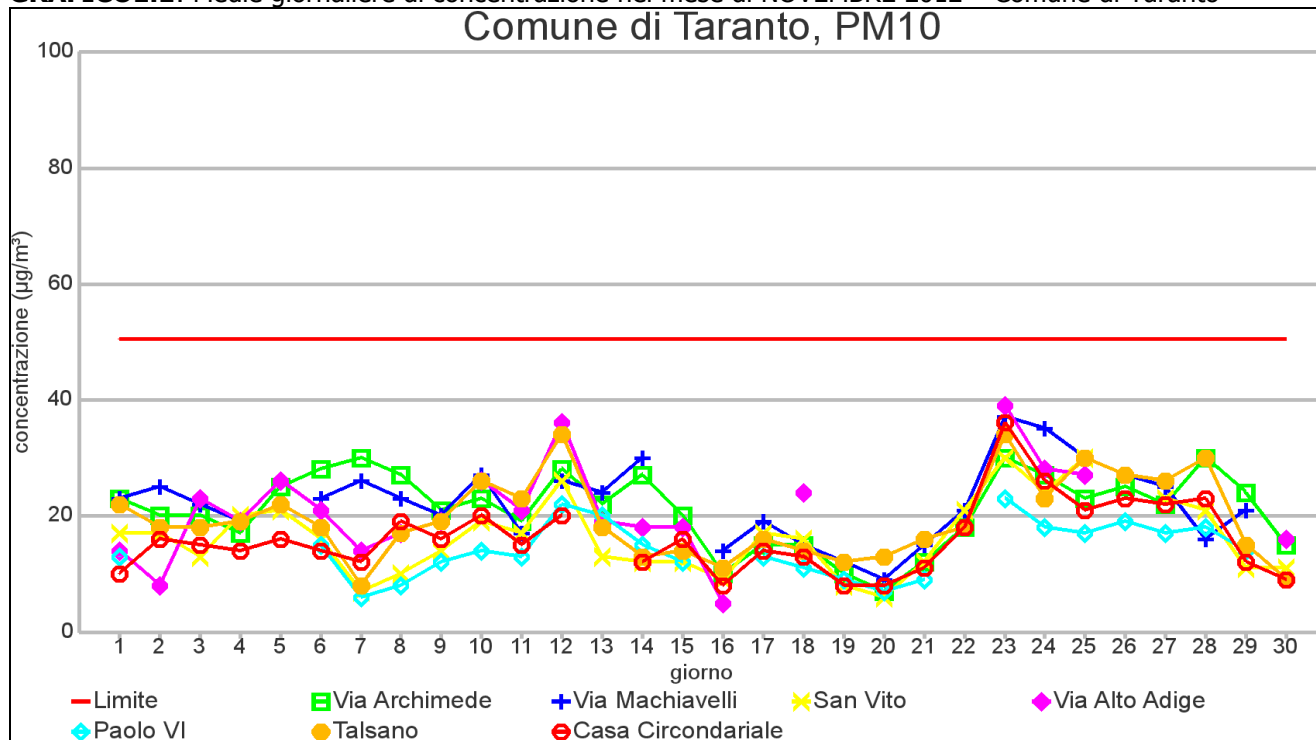
GRAFICO1.1: Medie giornaliere di concentrazione nel mese di NOVEMBRE 2012 – Comune di Taranto
