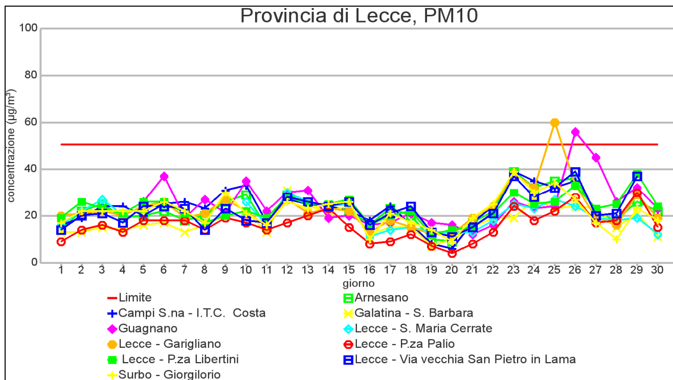
GRAFICO 1.1: Medie giornaliere di concentrazione nel mese di NOVEMBRE 2012
