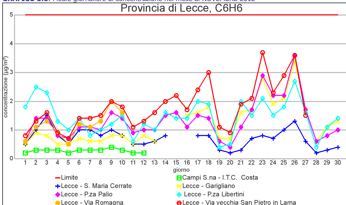
GRAFICO 5.1: Medie giornaliere di concentrazione nel mese di NOVEMBRE 2012
