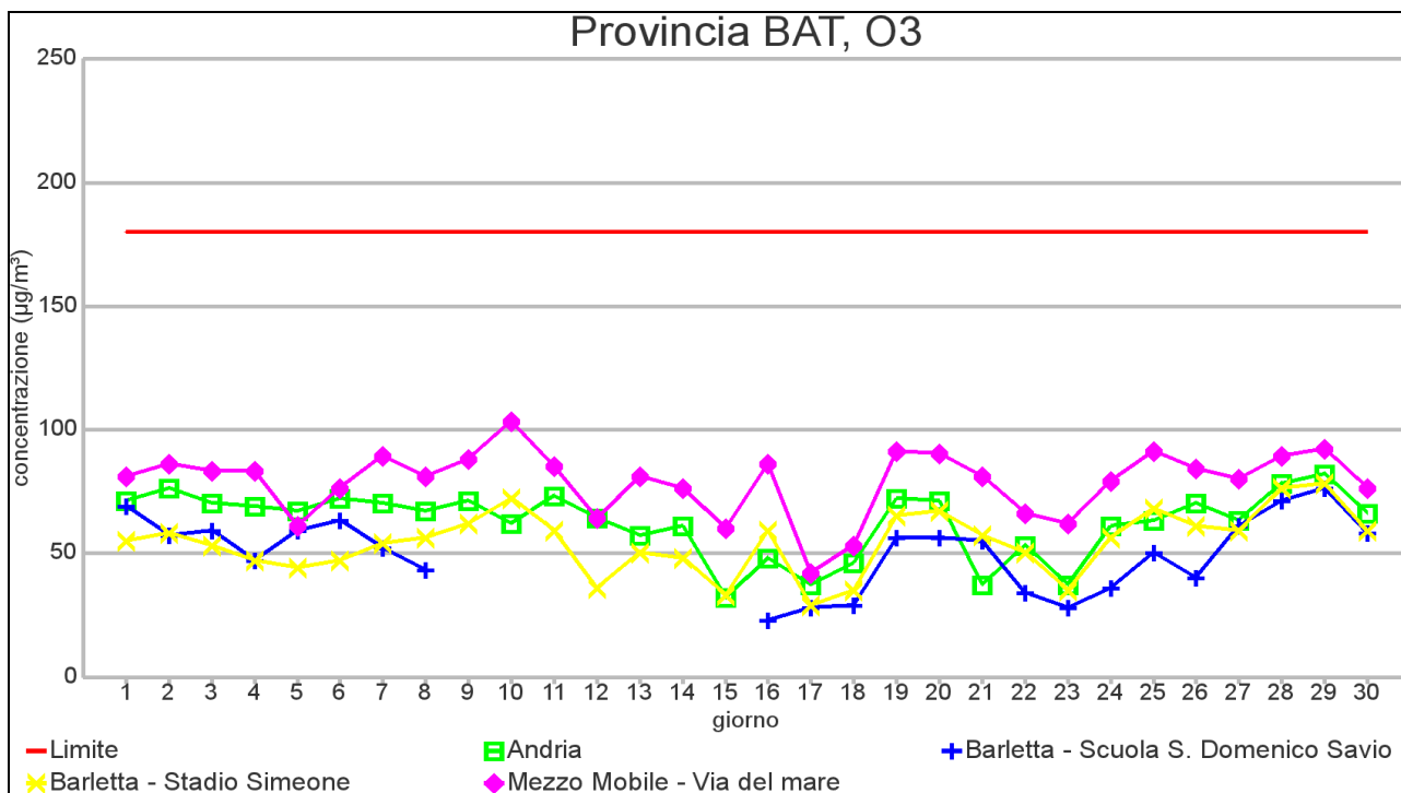
GRAFICO 3.1: massimo orario di O 3 –NOVEMBRE 2012
