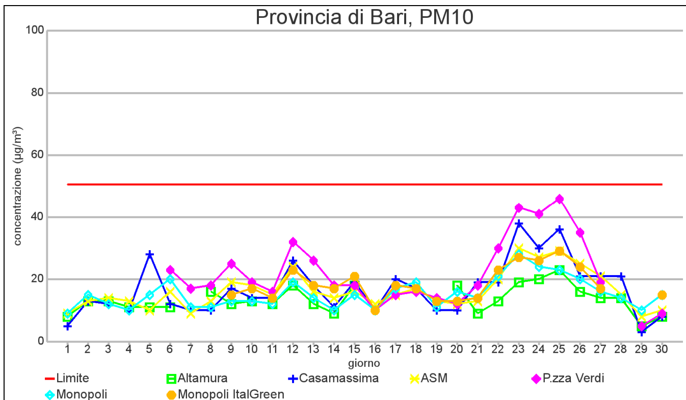
GRAFICO 1.3 PROVINCIA DI BARI: Valori medi giornalieri di concentrazione PM10 – NOVEMBRE 2012
