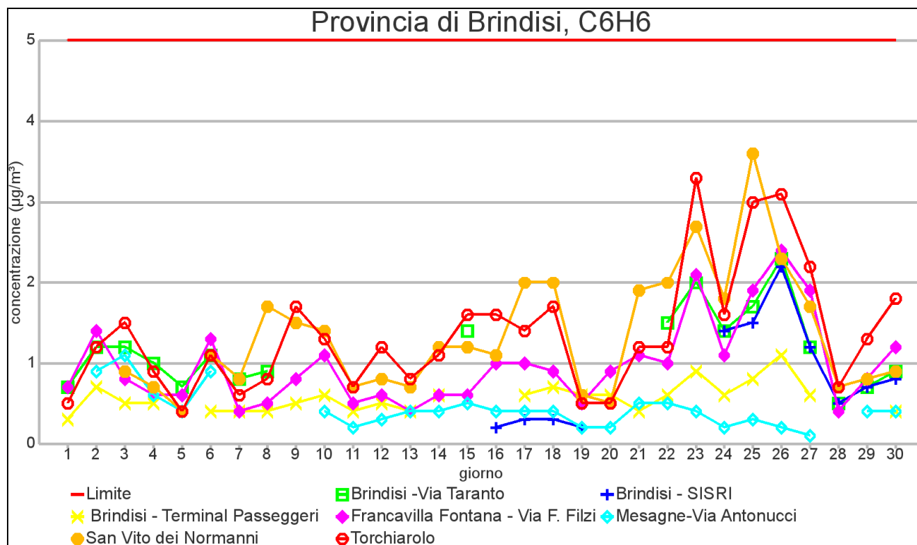
GRAFICO 5.1: Medie giornaliere di concentrazione nel mese di NOVEMBRE 2012 ( \mu\text{g}/\text{m}^3 )
