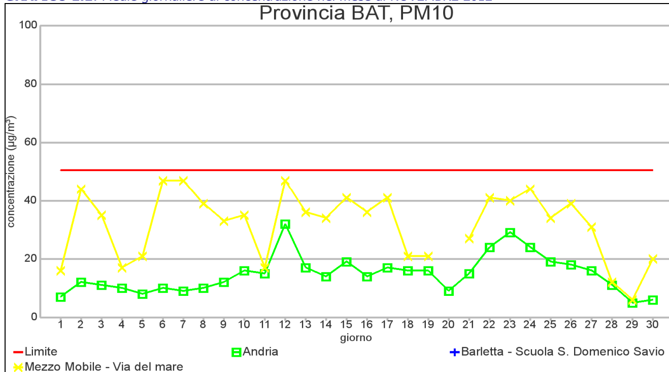
GRAFICO 1.1: Medie giornaliere di concentrazione nel mese di NOVEMBRE 2012
