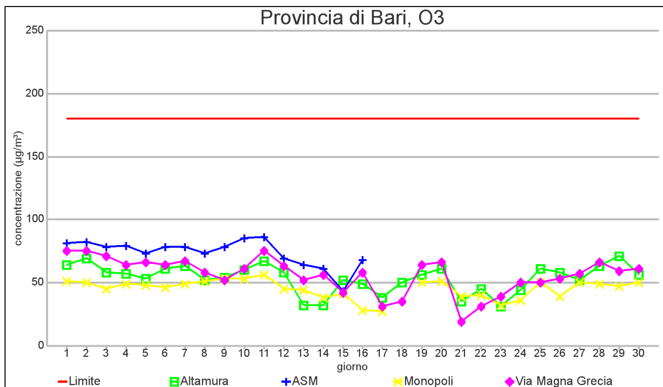
GRAFICO 3.2 PROVINCIA DI BARI: massimo orario –NOVEMBRE 2012
