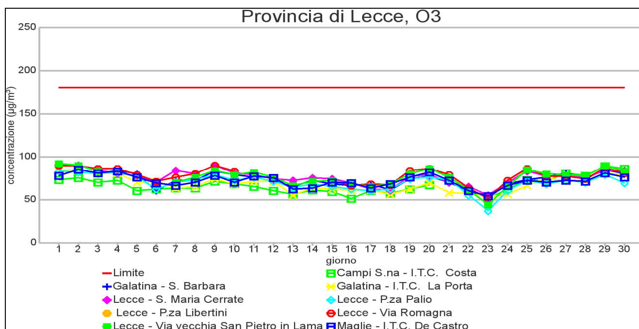
GRAFICO 4.1: massimo orario di O 3 –NOVEMBRE 2012
