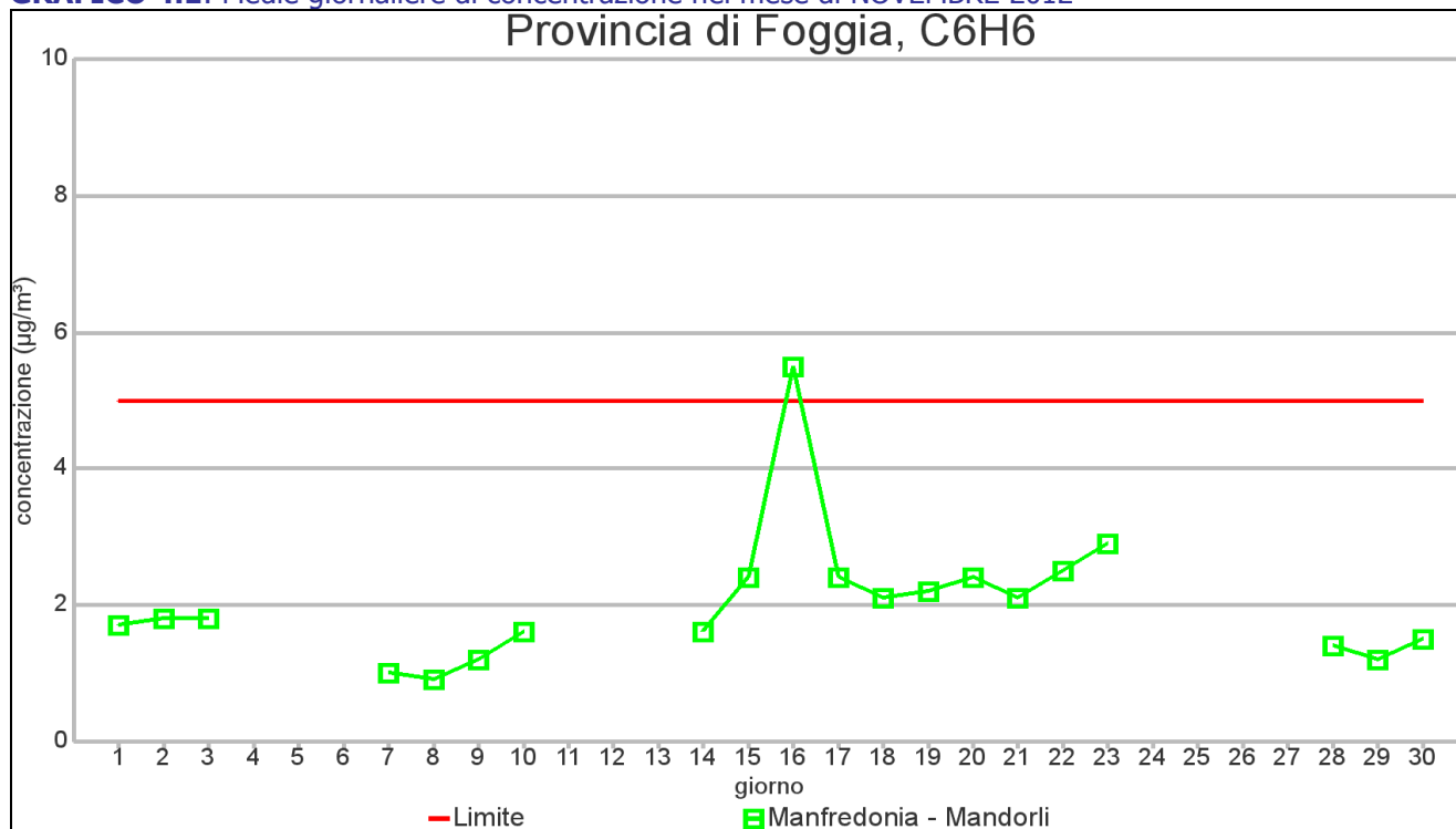
GRAFICO 4.1: Medie giornaliere di concentrazione nel mese di NOVEMBRE 2012
