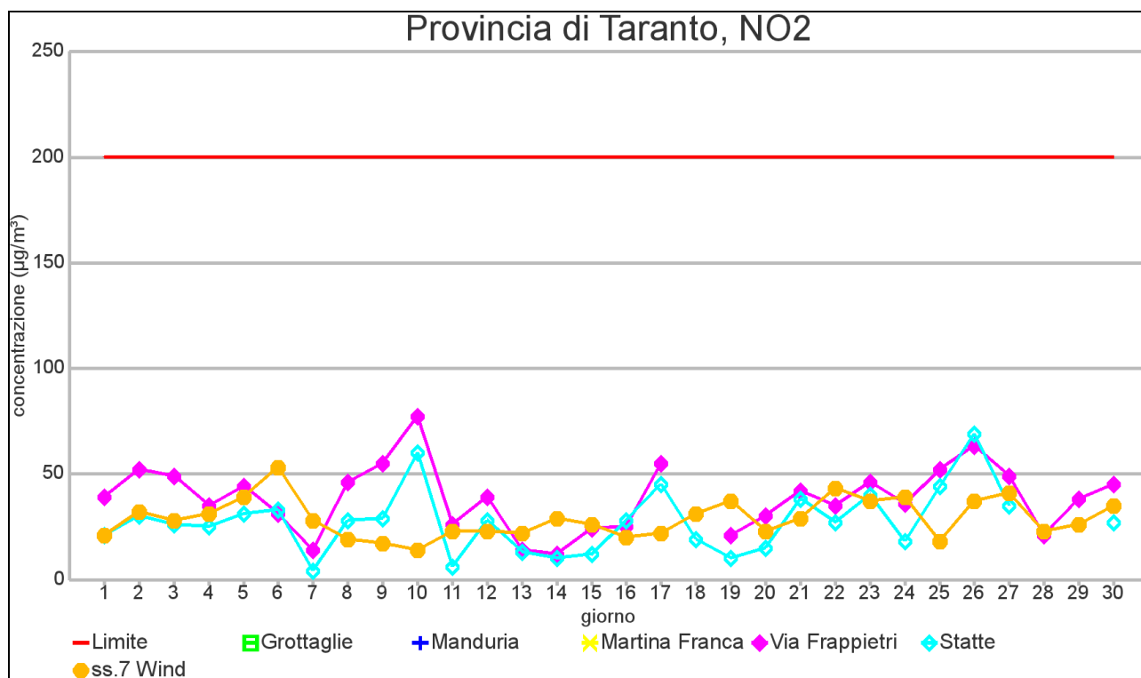
GRAFICO 2.2: Valore massimo giornaliero – mese di NOVEMBRE 2012 – Provincia di Taranto
