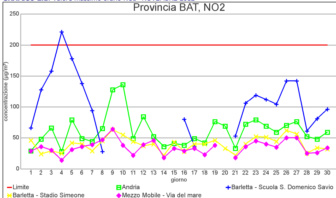
GRAFICO 2.1: Valore massimo orario NO 2 – NOVEMBRE 2012
