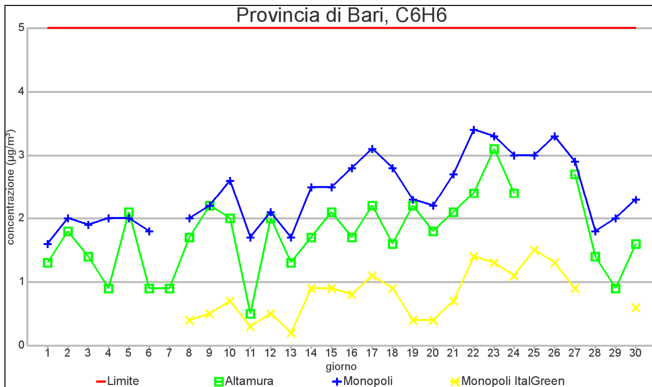
GRAFICO 4.2 PROVINCIA DI BARI: Medie giornaliere di concentrazione Benzene – mese di NOVEMBRE 2012
