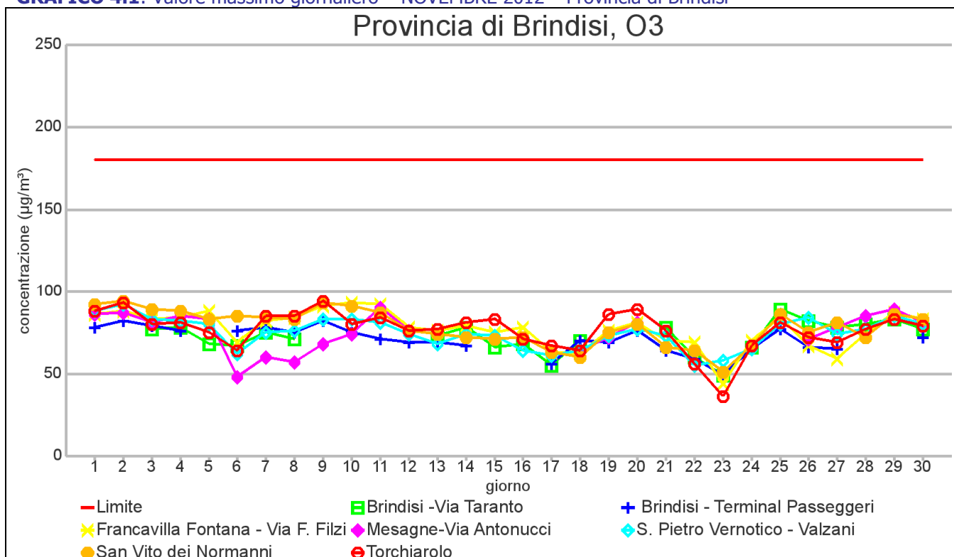
GRAFICO 4.1: Valore massimo giornaliero – NOVEMBRE 2012 – Provincia di Brindisi
