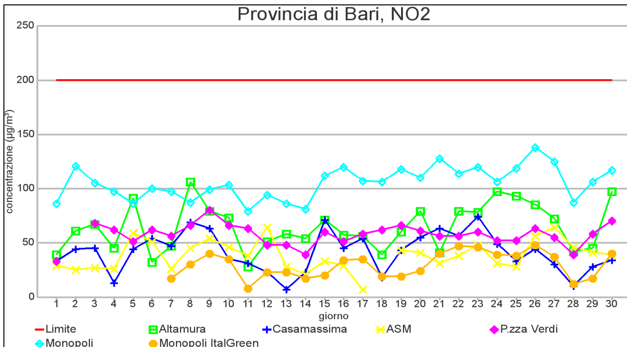
GRAFICO 2.3 PROVINCIA DI BARI: Valore massimo orario NO 2 – NOVEMBRE 2012
