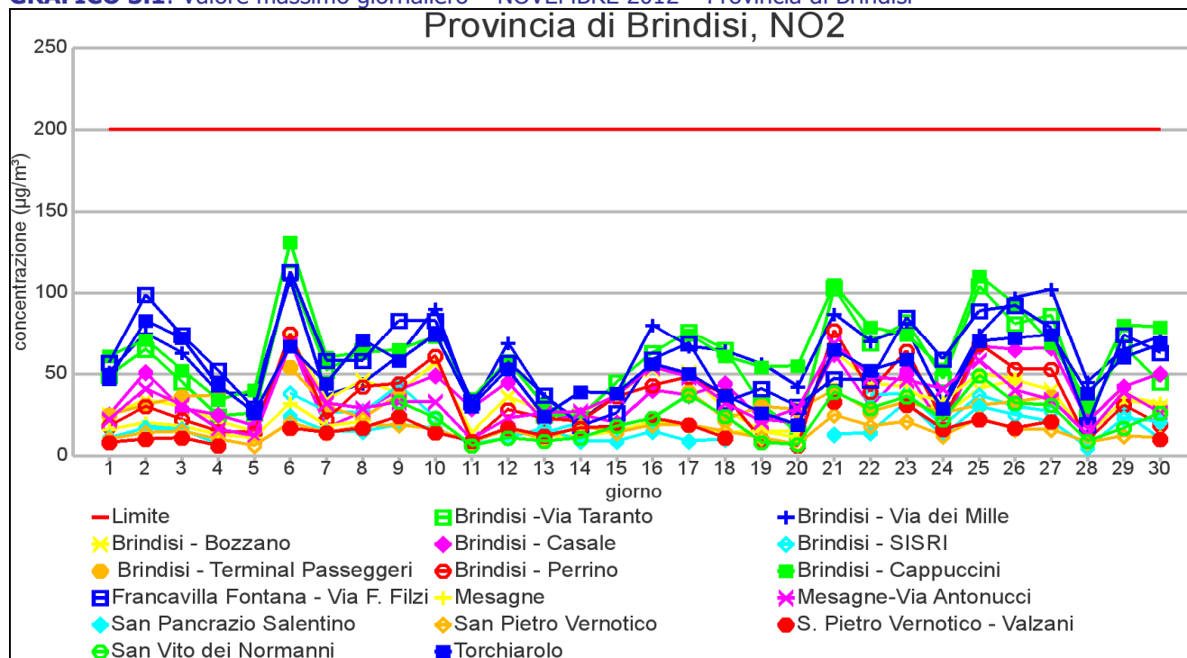
GRAFICO 3.1: Valore massimo giornaliero – NOVEMBRE 2012 – Provincia di Brindisi
