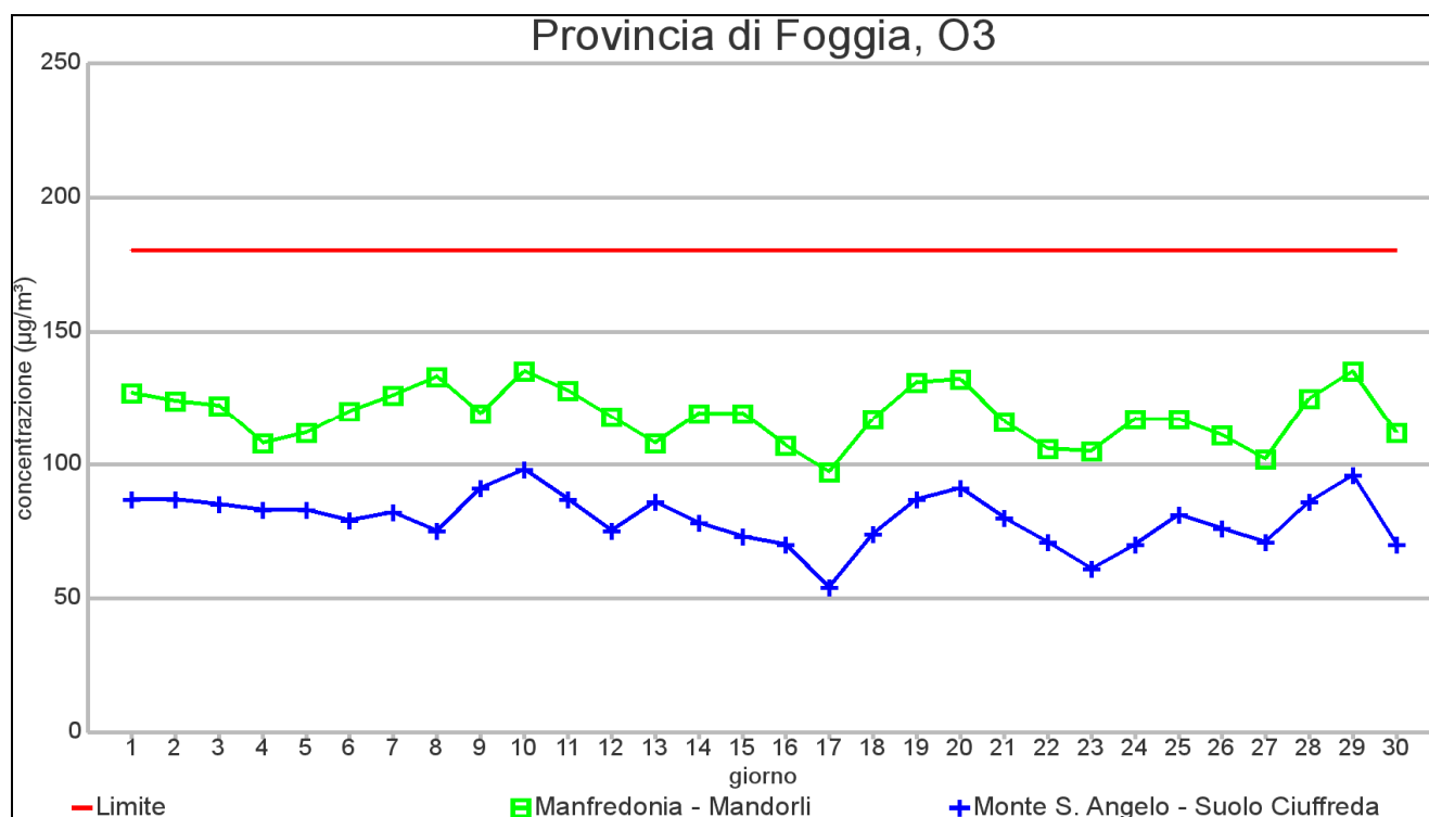
GRAFICO 3.1: massimo orario di O 3 – NOVEMBRE 2012
