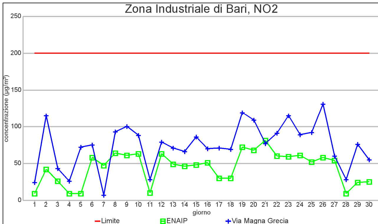
GRAFICO 2.2 AREA INDUSTRIALE BARI: Valore massimo orario NO 2 – NOVEMBRE 2012
