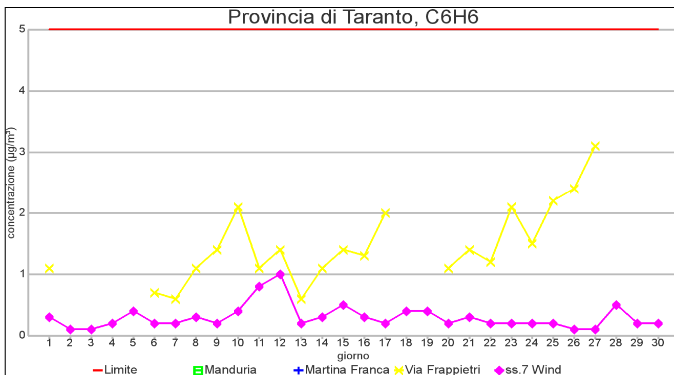
GRAFICO 5.1: Medie giornaliere di concentrazione nel mese di NOVEMBRE 2012 – Provincia di Taranto
