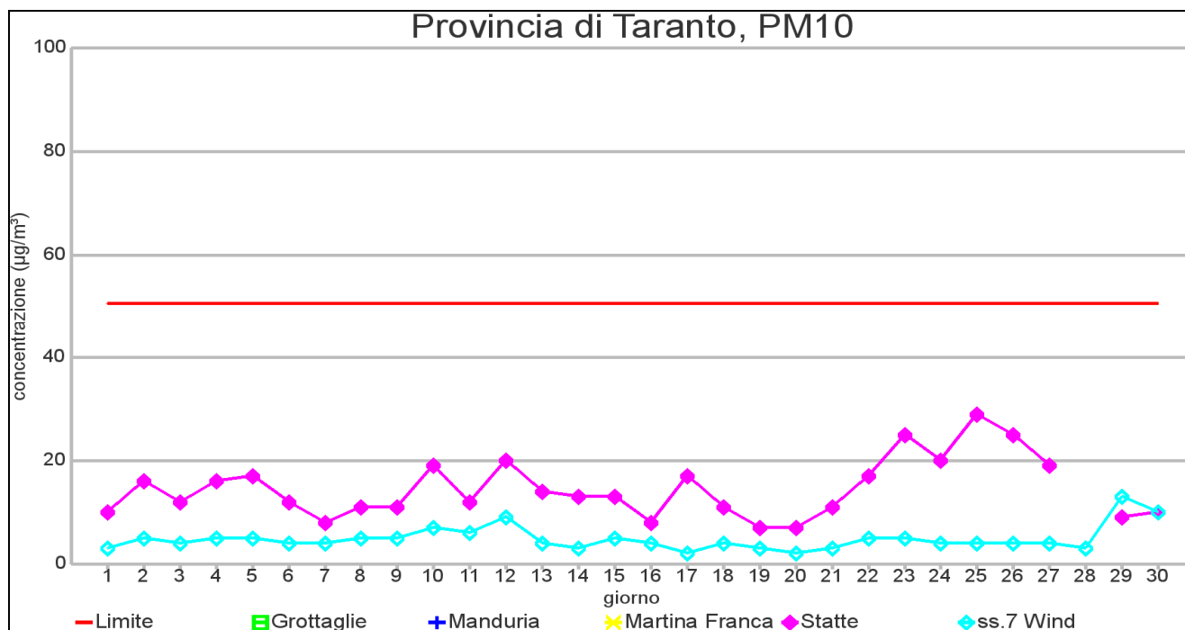
GRAFICO 1.2: Medie giornaliere di concentrazione nel mese di NOVEMBRE 2012 – Provincia di Taranto
