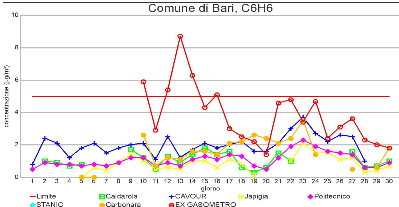
GRAFICO 4.2 PROVINCIA DI BARI: Medie giornaliere di concentrazione Benzene – mese di NOVEMBRE 2012
