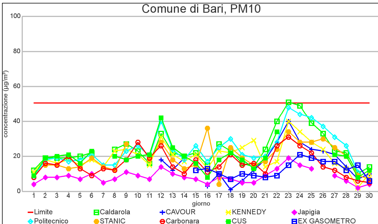
GRAFICO 1.1 COMUNE di BARI: Valori medi giornalieri di concentrazione PM10- mese di NOVEMBRE 2012
