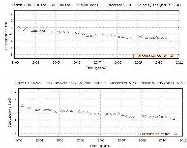
Fig. 8 - Mappa di velocità di deformazione a alta risoluzione relativa ad edifici affetti da subsidenza ubicati a sud della città di Gallipoli (LE), ed esempi di serie storiche di spostamento associate a due punti di misura.
