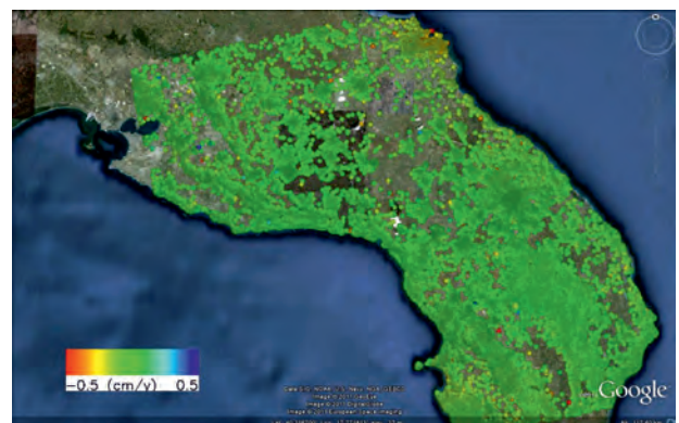
Fig. 5 - Mappa di velocità di deformazione a scala regionale relativa all'area del Salento, Puglia meridionale, ottenuta mediante elaborazione di immagini SAR ENVISAT acquisite in orbita ascendente (intervallo temporale: 2003-2010). - Ground deformation velocity map at regional scale relevant to the Salento area, Apulia region (ENVISAT ascending dataset, time interval 2003-2010).
